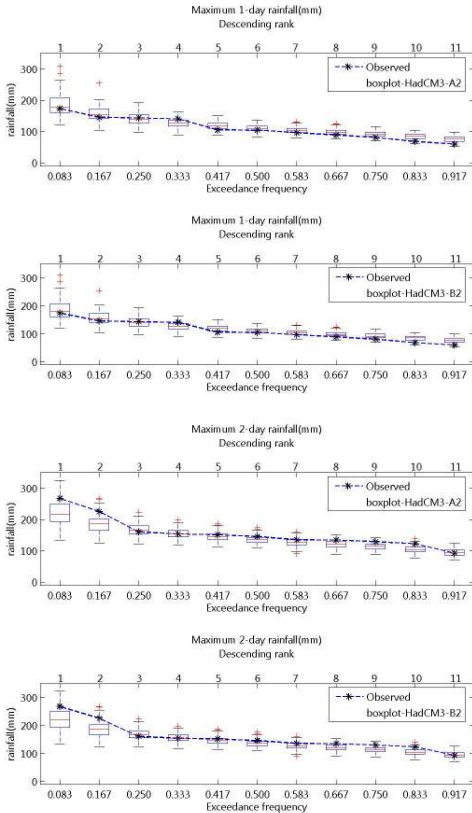
ภาพที่ จ.53 ความถี่ส่วนเกินของฝนรายวันสูงสุด 1- และ 2 วัน ของฝนรายวันอดีตและที่สังเคราะห์ได้จากภาพฉาย HadCM3-A2 และ HadCM3-B2 สำหรับสถานี 406004 (ปี ค.ศ.1991-2001)
