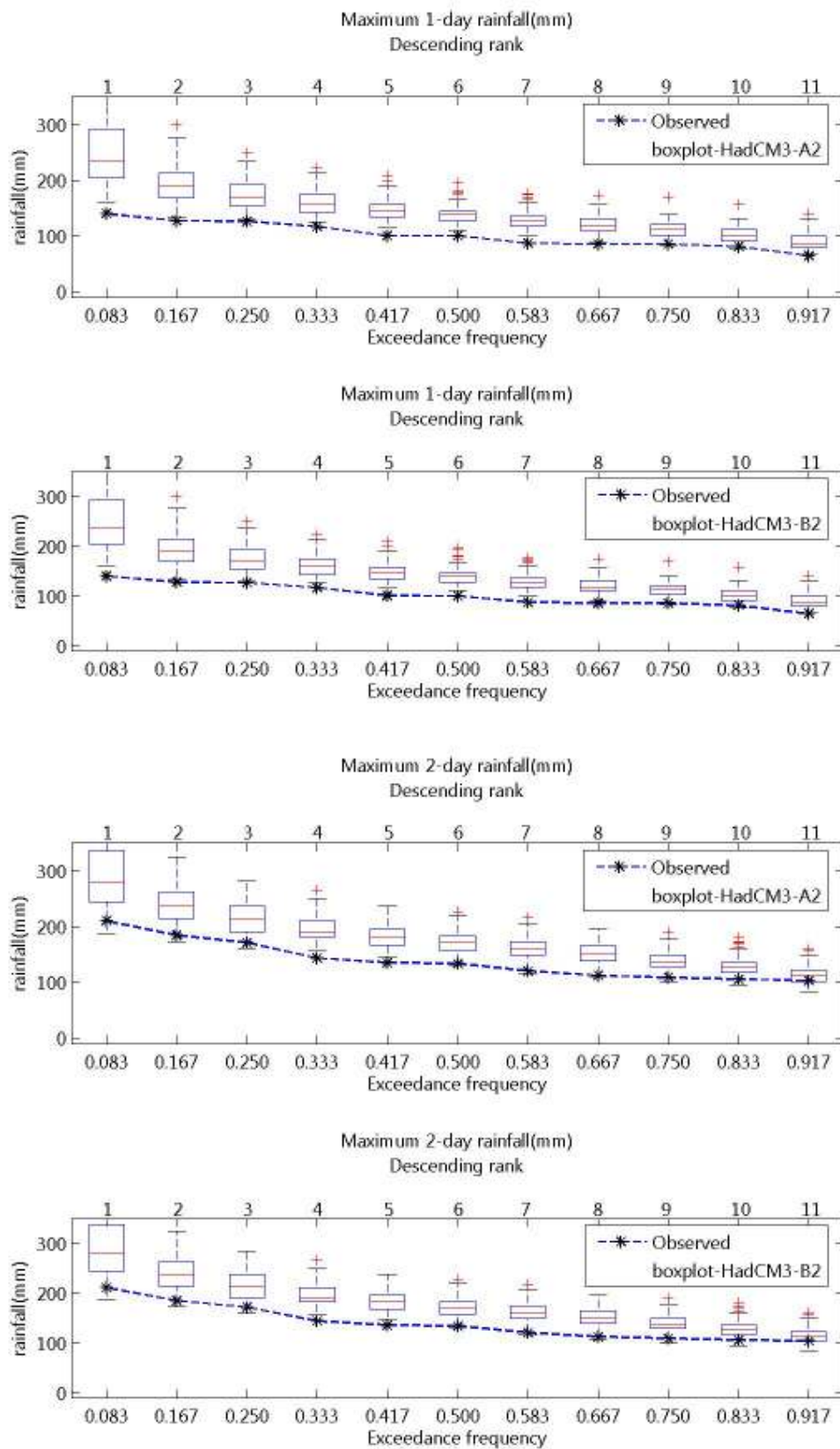
ภาพที่ จ.47 ความถี่ส่วนเกินของฝนรายวันสูงสุด 1- และ 2 วัน ของฝนรายวันอดีตและที่สังเคราะห์ได้จากภาพฉาย HadCM3-A2 และ HadCM3-B2 สำหรับสถานี 405002 (ปี ค.ศ.1991-2001)
