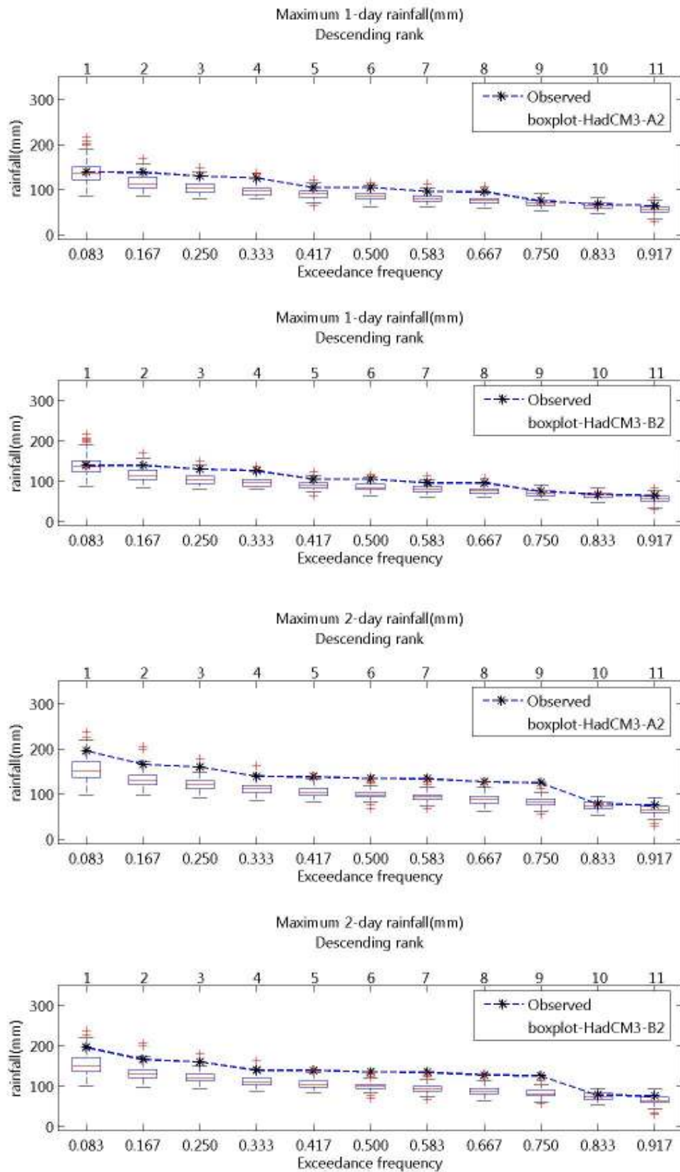
ภาพที่ จ.79 ความถี่ส่วนเกินของฝนรายวันสูงสุด 1- และ 2 วัน ของฝนรายวันอดีตและที่สังเคราะห์ได้จากภาพฉาย HadCM3-A2 และ HadCM3-B2 สำหรับสถานี 436006 (ปี ค.ศ.1991-2001)
