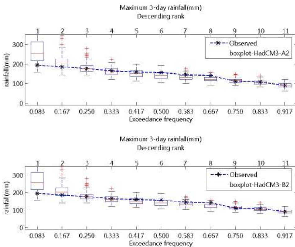
ภาพที่ จ.30 ความถี่ส่วนเกินของฝนรายวันสูงสุด 3 วัน ของฝนรายวันอดีตและที่สังเคราะห์ได้จาก ภาพฉาย HadCM3-A2 และ HadCM3-B2 สำหรับสถานี 21190 (ปี ค.ศ.1991-2001)
