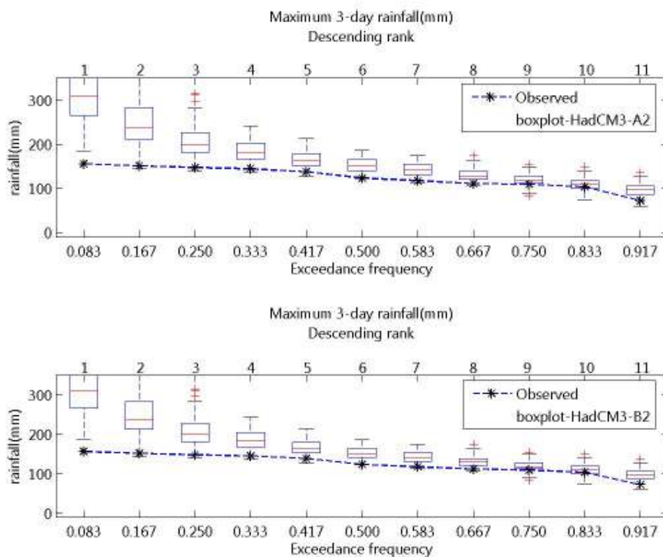
ภาพที่ จ.82 ความถี่ส่วนเกินของฝนรายวันสูงสุด 3 วัน ของฝนรายวันอดีตและที่สังเคราะห์ได้จาก ภาพฉาย HadCM3-A2 และ HadCM3-B2 สำหรับสถานี 436007 (ปี ค.ศ.1991-2001)
