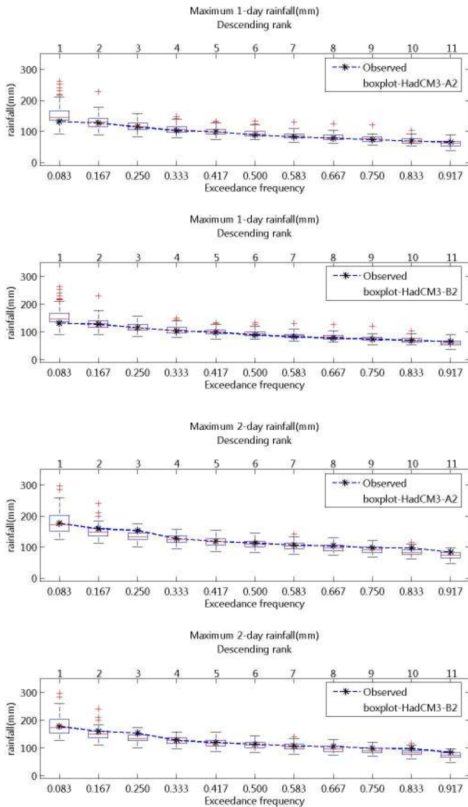
ภาพที่ จ.49 ความถี่ส่วนเกินของฝนรายวันสูงสุด 1- และ 2 วัน ของฝนรายวันอดีตและที่สังเคราะห์ได้จากภาพฉาย HadCM3-A2 และ HadCM3-B2 สำหรับสถานี 405008 (ปี ค.ศ.1991-2001)
