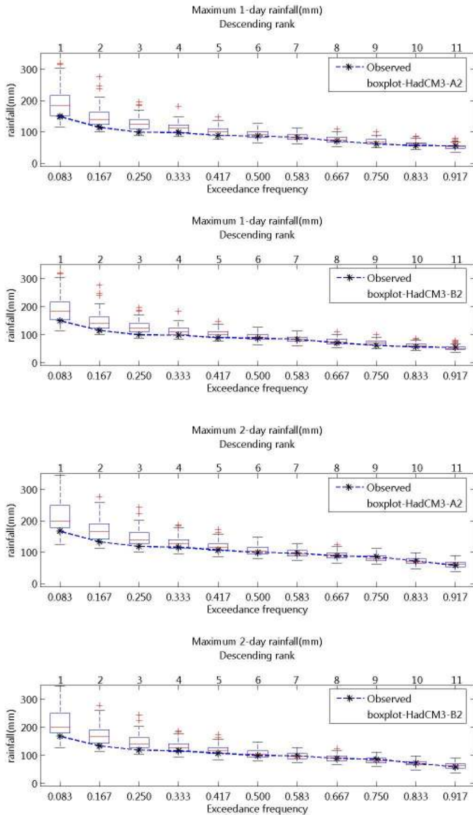
ภาพที่ จ.9 ความถี่ส่วนเกินของฝนรายวันสูงสุด 1- และ 2 วัน ของฝนรายวันอดีตและที่สังเคราะห์ได้จากภาพฉาย HadCM3-A2 และ HadCM3-B2 สำหรับสถานี 05171 (ปี ค.ศ.1991-2001)
