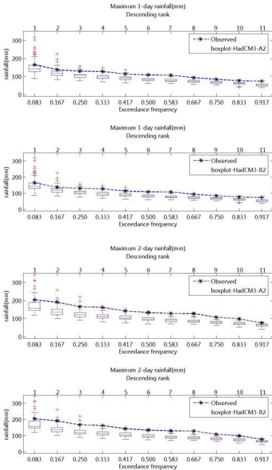
ภาพที่ จ.67 ความถี่ส่วนเกินของฝนรายวันสูงสุด 1- และ 2 วัน ของฝนรายวันอดีตและที่สังเคราะห์ได้จากภาพฉาย HadCM3-A2 และ HadCM3-B2 สำหรับสถานี 432001 (ปี ค.ศ.1991-2001)
