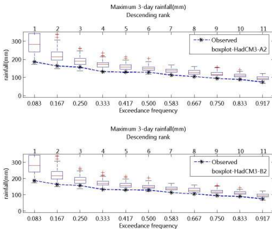
ภาพที่ จ.16 ความถี่ส่วนเกินของฝนรายวันสูงสุด 3 วัน ของฝนรายวันอดีตและที่สังเคราะห์ได้จาก ภาพฉาย HadCM3-A2 และ HadCM3-B2 สำหรับสถานี 11202 (ปี ค.ศ.1991-2001)
