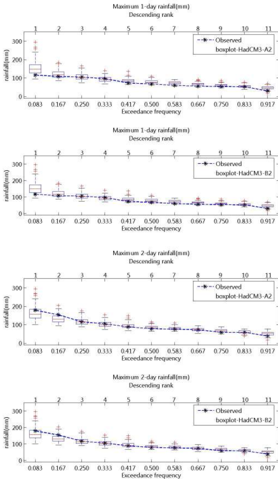
ภาพที่ ๗.7 ความถี่ส่วนเกินของฝนรายวันสูงสุด 1- และ 2 วัน ของฝนรายวันอดีตและที่สังเคราะห์ได้จากภาพฉาย HadCM3-A2 และ HadCM3-B2 สำหรับ 05092 (ปี ค.ศ.1991-2001)
