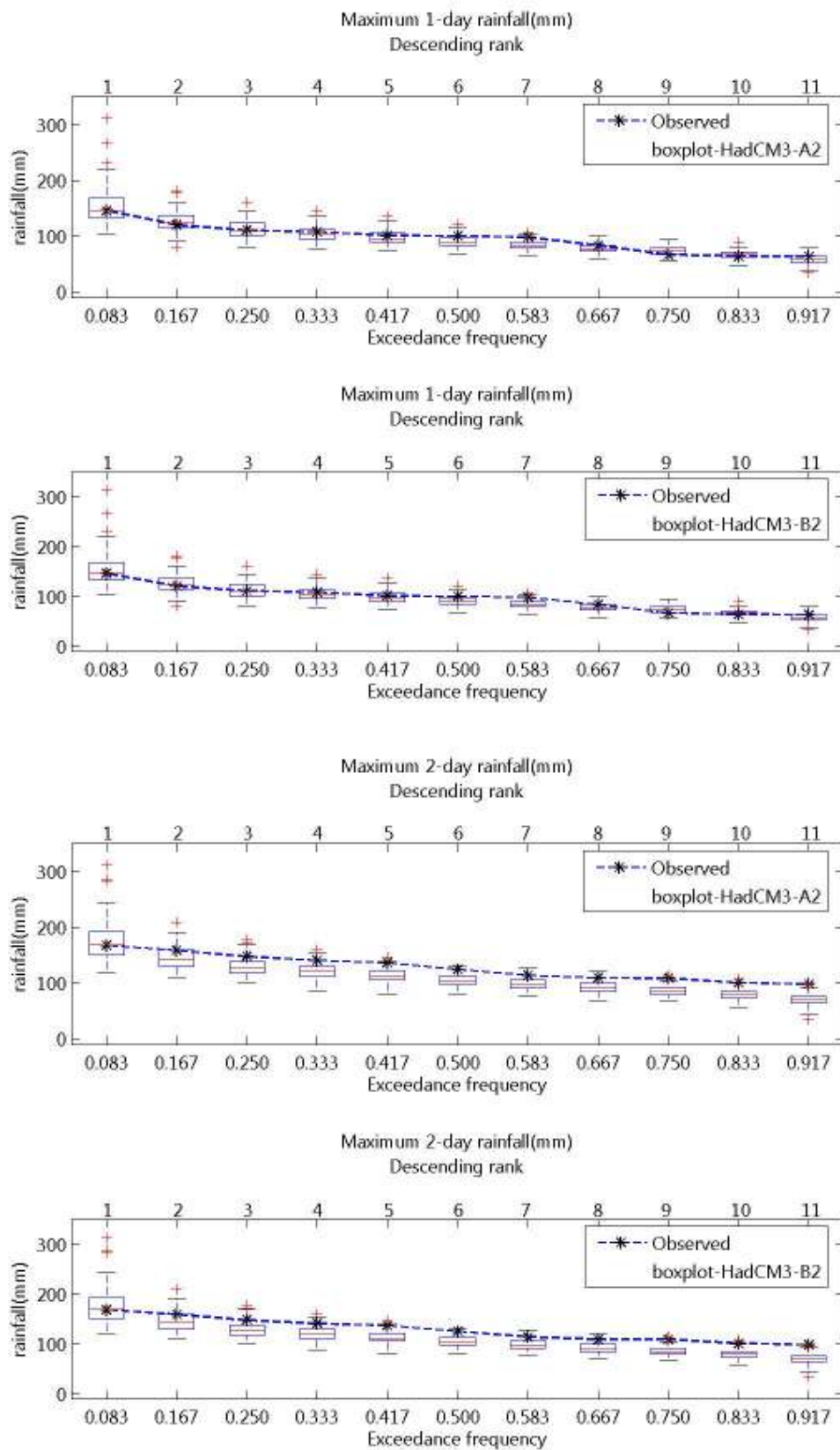
ภาพที่ จ.69 ความถี่ส่วนเกินของฝนรายวันสูงสุด 1- และ 2 วัน ของฝนรายวันอดีตและที่สังเคราะห์ได้จากภาพฉาย HadCM3-A2 และ HadCM3-B2 สำหรับสถานี 432004 (ปี ค.ศ.1991-2001)
