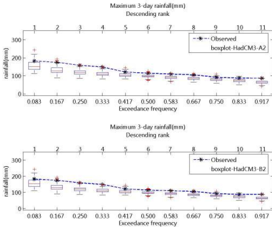
ภาพที่ ๑.6 ความถี่ส่วนเกินของฝนรายวันสูงสุด 3 วัน ของฝนรายวันอดีตและที่สังเคราะห์ได้จากภาพฉาย HadCM3-A2 และ HadCM3-B2 สำหรับสถานี 05032 (ปี ค.ศ.1991-2001)
