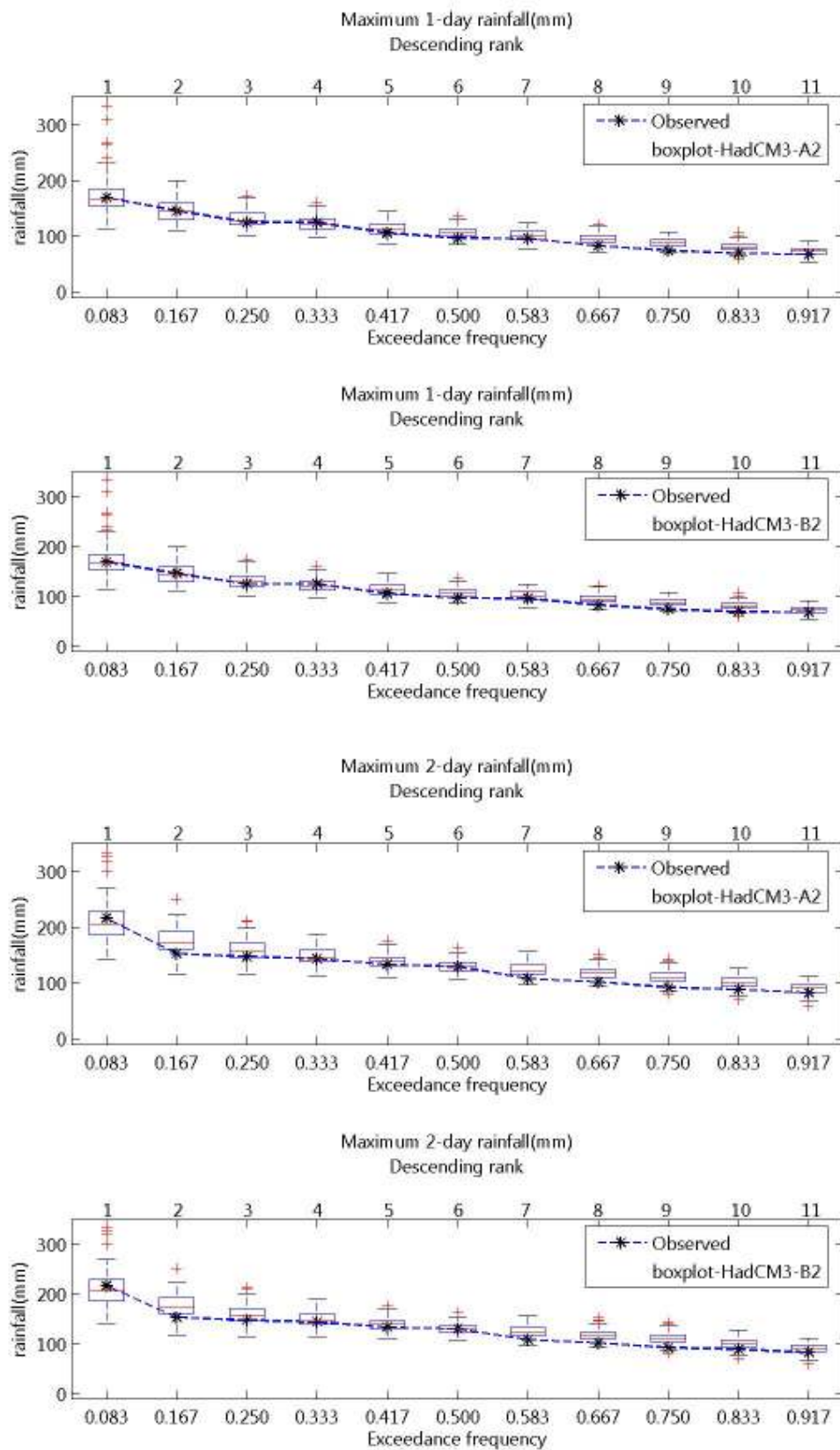
ภาพที่ จ.61 ความถี่ส่วนเกินของฝนรายวันสูงสุด 1- และ 2 วัน ของฝนรายวันอดีตและที่สังเคราะห์ได้จากภาพฉาย HadCM3-A2 และ HadCM3-B2 สำหรับสถานี 407009 (ปี ค.ศ.1991-2001)
