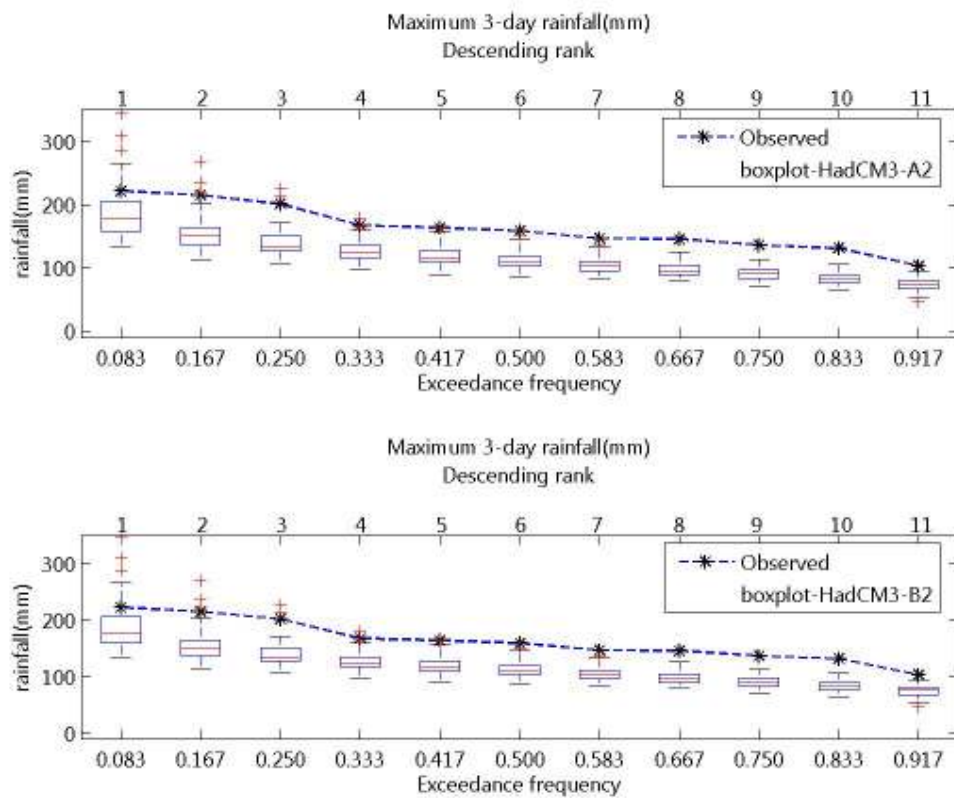
ภาพที่ ๑.68 ความถี่ส่วนเกินของฝนรายวันสูงสุด 3 วัน ของฝนรายวันอดีตและที่สังเคราะห์ได้จาก ภาพฉาย HadCM3-A2 และ HadCM3-B2 สำหรับสถานี 432001 (ปี ค.ศ.1991-2001)
