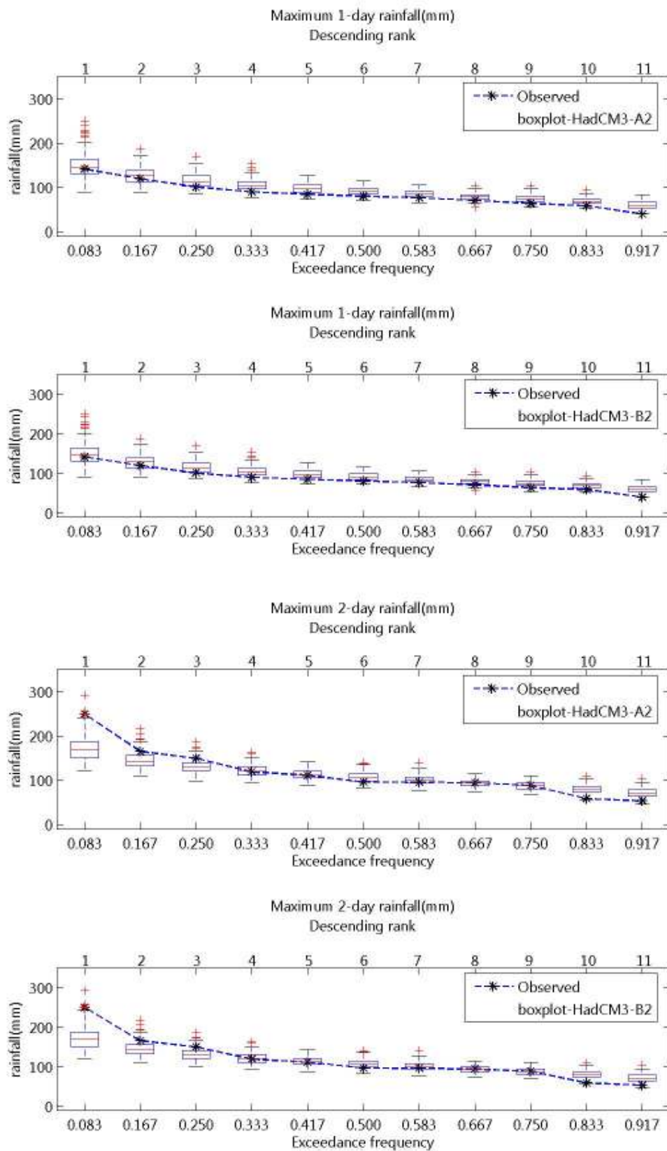
ภาพที่ จ.13 ความถี่ส่วนเกินของฝนรายวันสูงสุด 1- และ 2 วัน ของฝนรายวันอดีตและที่สังเคราะห์ได้จากภาพฉาย HadCM3-A2 และ HadCM3-B2 สำหรับสถานี 11170 (ปี ค.ศ.1991-2001)
