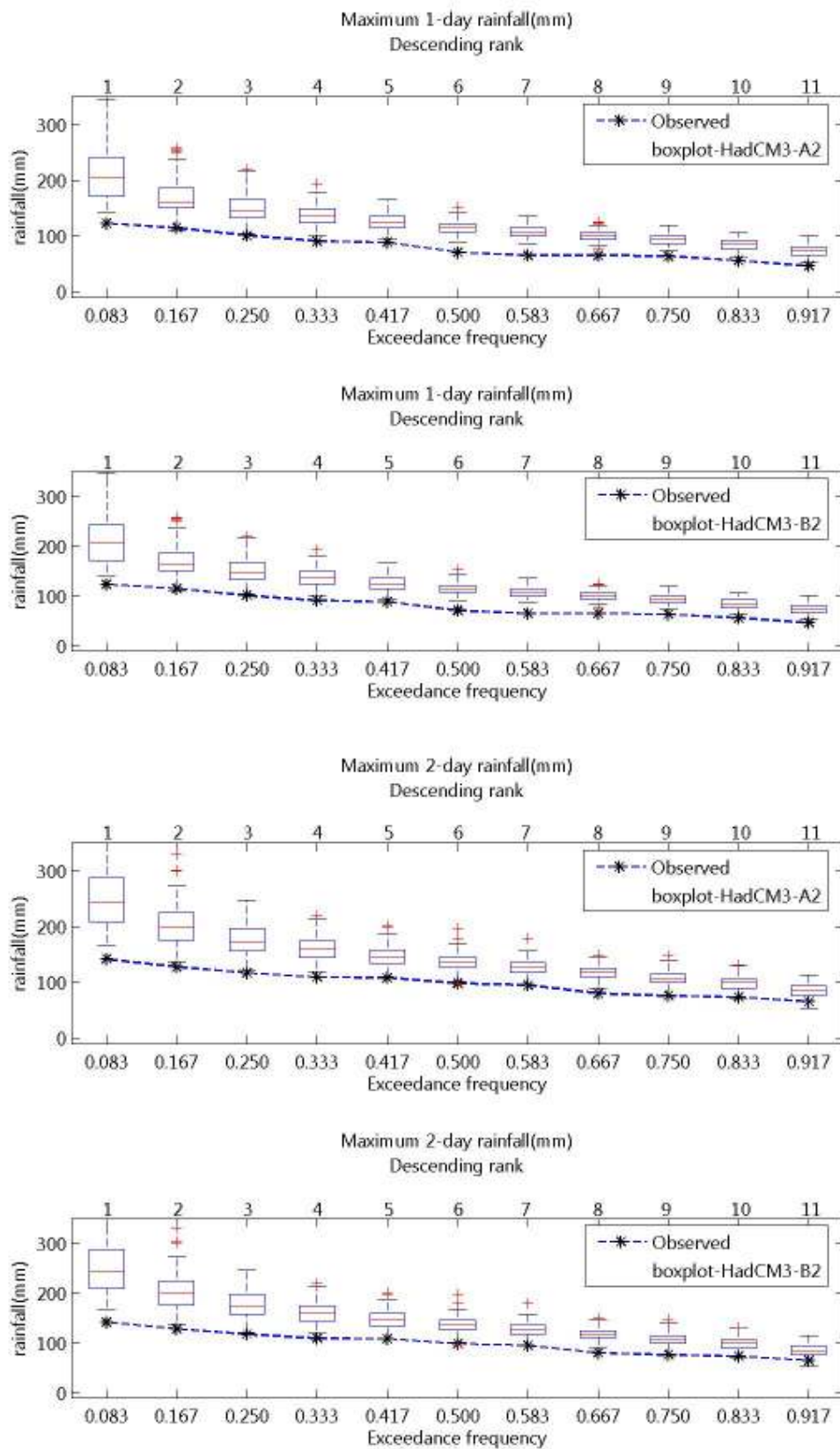
ภาพที่ จ.33 ความถี่ส่วนเกินของฝนรายวันสูงสุด 1- และ 2 วัน ของฝนรายวันอดีตและที่สังเคราะห์ได้จากภาพฉาย HadCM3-A2 และ HadCM3-B2 สำหรับสถานี 49062 (ปี ค.ศ.1991-2001)
