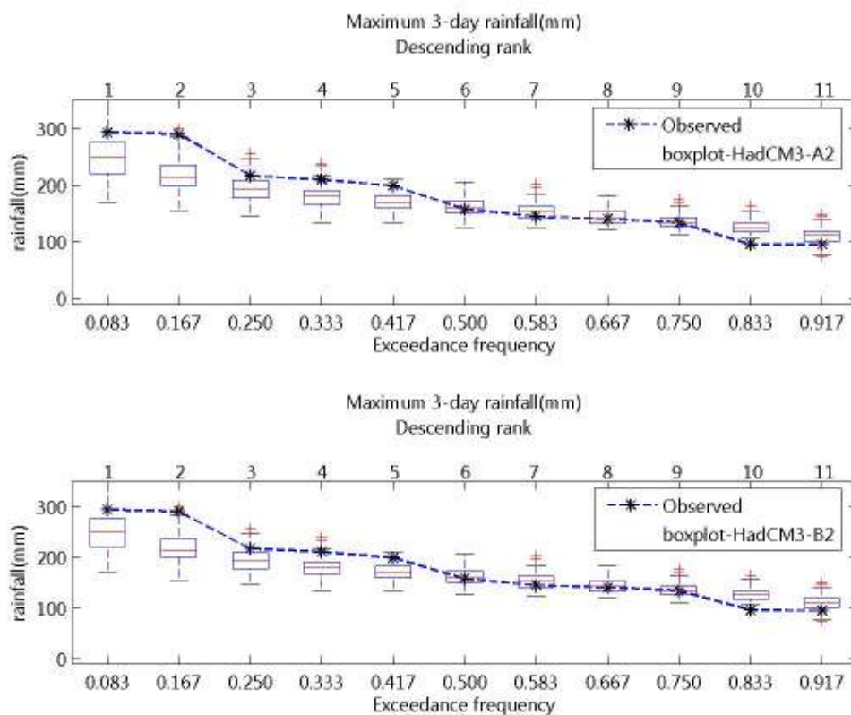
ภาพที่ จ.60 ความถี่ส่วนเกินของฝนรายวันสูงสุด 3 วัน ของฝนรายวันอดีตและที่สังเคราะห์ได้จาก ภาพฉาย HadCM3-A2 และ HadCM3-B2 สำหรับสถานี 407006 (ปี ค.ศ.1991-2001)
