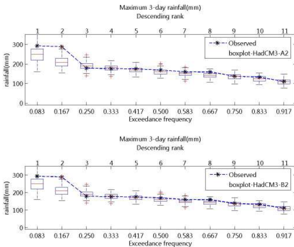
ภาพที่ จ.54 ความถี่ส่วนเกินของฝนรายวันสูงสุด 3 วัน ของฝนรายวันอดีตและที่สังเคราะห์ได้จาก ภาพฉาย HadCM3-A2 และ HadCM3-B2 สำหรับสถานี 406004 (ปี ค.ศ.1991-2001)
