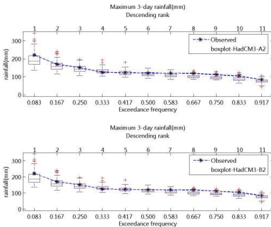
ภาพที่ จ.32 ความถี่ส่วนเกินของฝนรายวันสูงสุด 3 วัน ของฝนรายวันอดีตและที่สังเคราะห์ได้จาก ภาพฉาย HadCM3-A2 และ HadCM3-B2 สำหรับสถานี 49013 (ปี ค.ศ.1991-2001)
