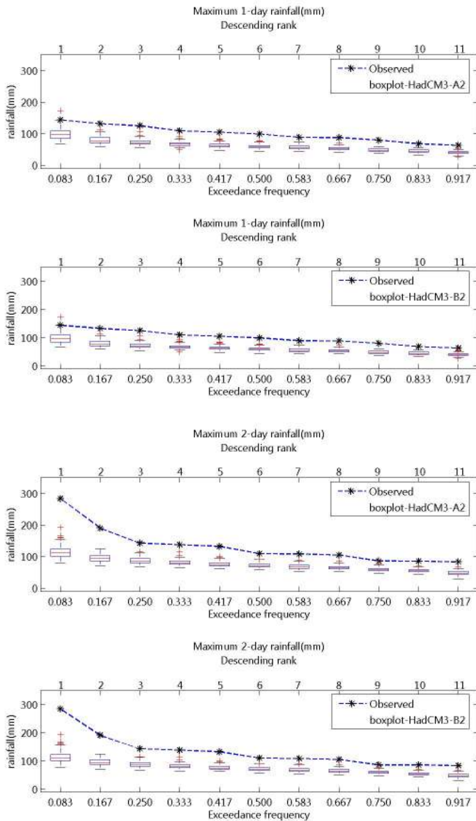
ภาพที่ จ.71 ความถี่ส่วนเกินของฝนรายวันสูงสุด 1- และ 2 วัน ของฝนรายวันอดีตและที่สังเคราะห์ได้จากภาพฉาย HadCM3-A2 และ HadCM3-B2 สำหรับสถานี 432005 (ปี ค.ศ.1991-2001)
