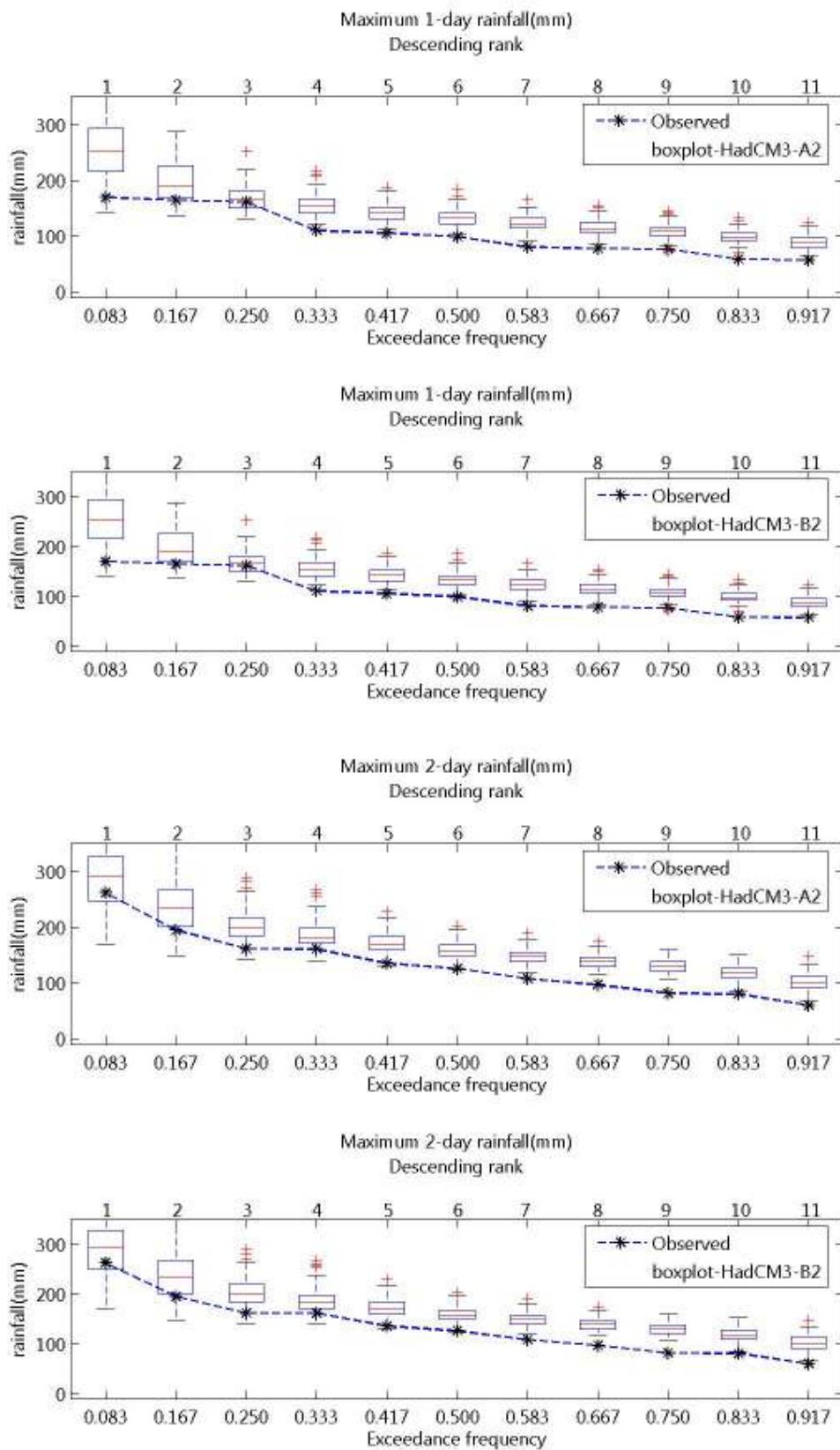
ภาพที่ จ.73 ความถี่ส่วนเกินของฝนรายวันสูงสุด 1- และ 2 วัน ของฝนรายวันอดีตและที่สังเคราะห์ได้จากภาพฉาย HadCM3-A2 และ HadCM3-B2 สำหรับสถานี 432006 (ปี ค.ศ.1991-2001)
