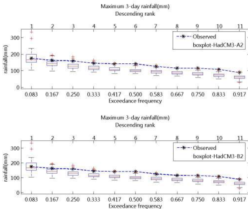
ภาพที่ จ.28 ความถี่ส่วนเกินของฝนรายวันสูงสุด 3 วัน ของฝนรายวันอดีตและที่สังเคราะห์ได้จาก ภาพถ่าย HadCM3-A2 และ HadCM3-B2 สถานี 21043 (ปี ค.ศ.1991-2001)
