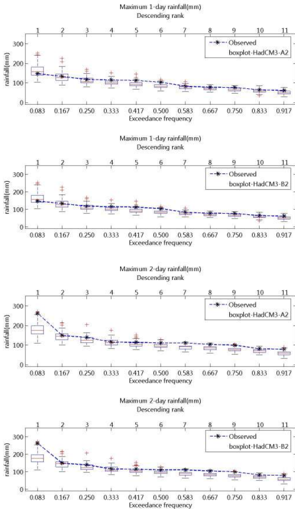
ภาพที่ จ.23 ความถี่ส่วนเกินของฝนรายวันสูงสุด 1- และ 2 วัน ของฝนรายวันอดีตและที่สังเคราะห์ได้จากภาพฉาย HadCM3-A2 และ HadCM3-B2 สำหรับสถานี 14112 (ปี ค.ศ.1991-2001)
