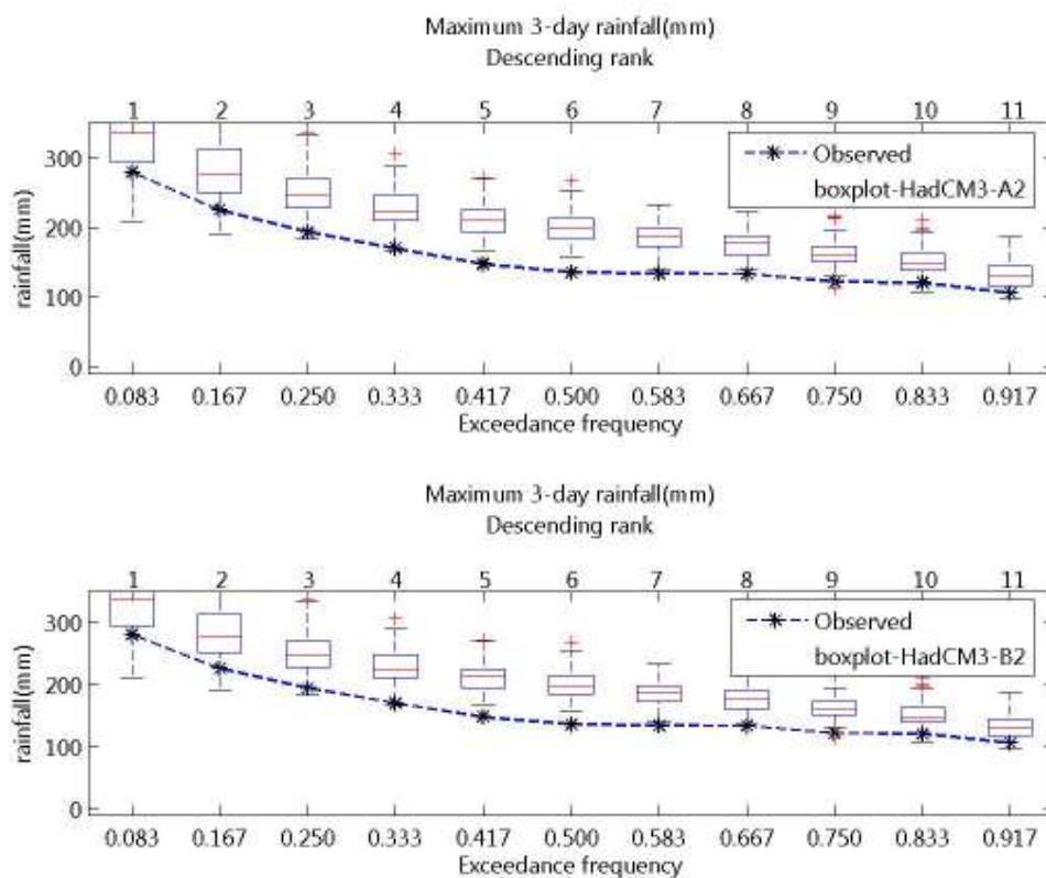
ภาพที่ จ.48 ความถี่ส่วนเกินของฝนรายวันสูงสุด 3 วัน ของฝนรายวันอดีตและที่สังเคราะห์ได้จาก ภาพฉาย HadCM3-A2 และ HadCM3-B2 สำหรับสถานี 405002 (ปี ค.ศ.1991-2001)
