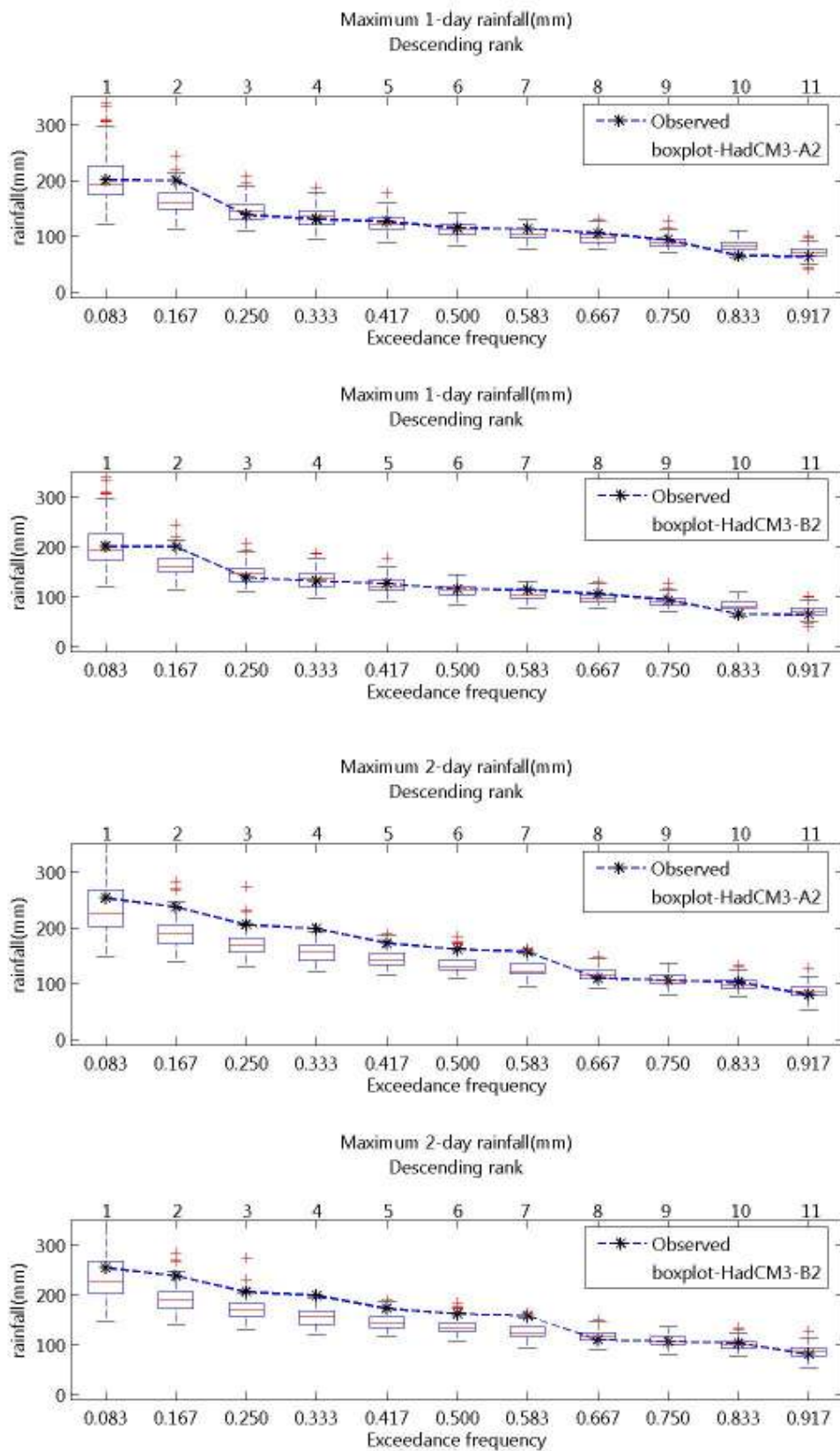
ภาพที่ จ.39 ความถี่ส่วนเกินของฝนรายวันสูงสุด 1- และ 2 วัน ของฝนรายวันอดีตและที่สังเคราะห์ได้จากภาพฉาย HadCM3-A2 และ HadCM3-B2 สำหรับสถานี 72022 (ปี ค.ศ.1991-2001)
