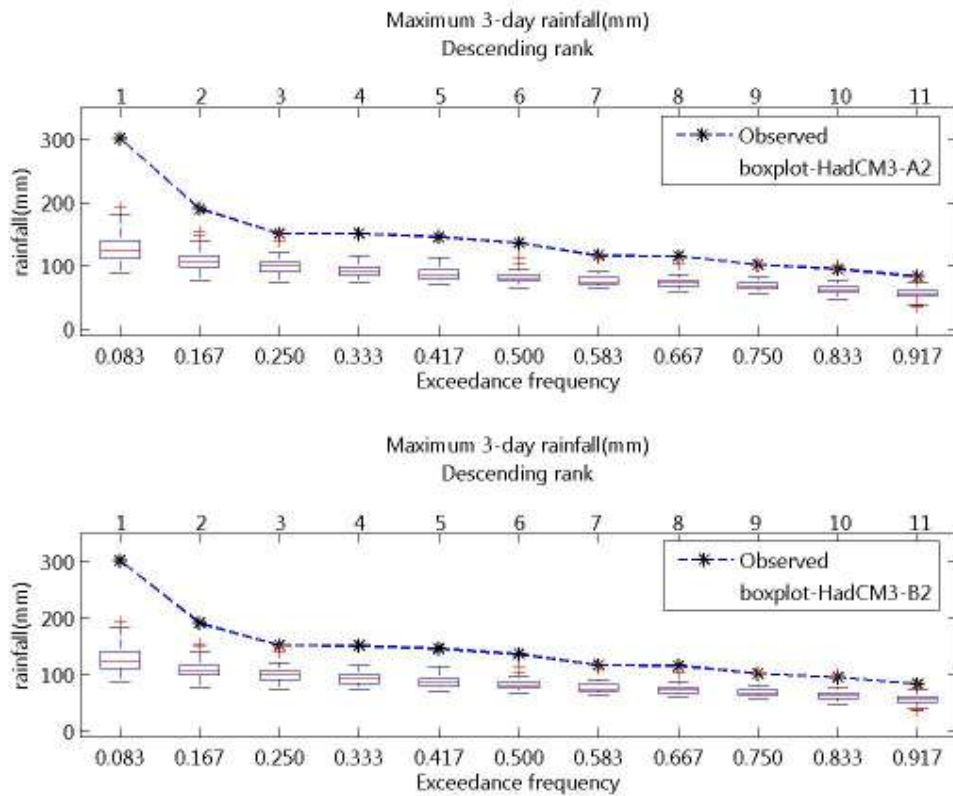
ภาพที่ จ.72 ความถี่ส่วนเกินของฝนรายวันสูงสุด 3 วัน ของฝนรายวันอดีตและที่สังเคราะห์ได้จาก ภาพฉาย HadCM3-A2 และ HadCM3-B2 สำหรับสถานี 432005 (ปี ค.ศ.1991-2001)
