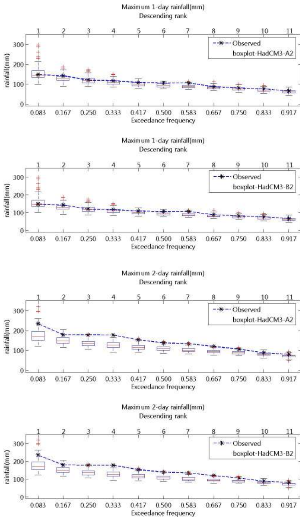
ภาพที่ จ.35 ความถี่ส่วนเกินของฝนรายวันสูงสุด 1- และ 2 วัน ของฝนรายวันอดีตและที่สังเคราะห์ได้จากภาพฉาย HadCM3-A2 และ HadCM3-B2 สำหรับสถานี 49301 (ปี ค.ศ.1991-2001)
