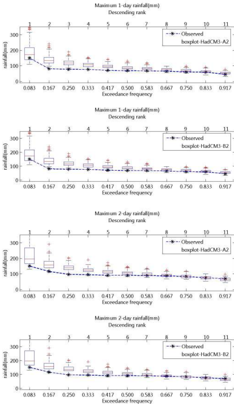
ภาพที่ จ.3 ความถี่ส่วนเกินของฝนรายวันสูงสุด 1- และ 2 วัน ของฝนรายวันอดีตและที่สังเคราะห์ได้ จากภาพฉาย HadCM3-A2 และ HadCM3-B2 สำหรับสถานี 05023 (ปี ค.ศ.1991-2001)
