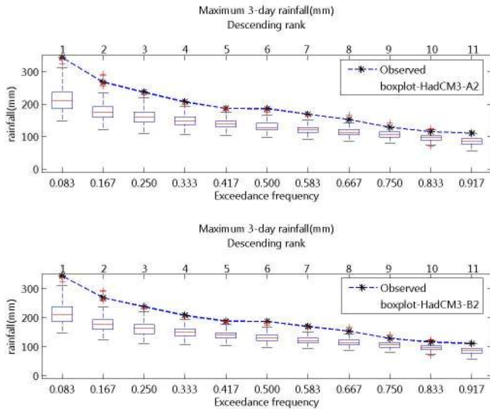
ภาพที่ จ.64 ความถี่ส่วนเกินของฝนรายวันสูงสุด 3 วัน ของฝนรายวันอดีตและที่สังเคราะห์ได้จาก ภาพฉาย HadCM3-A2 และ HadCM3-B2 สำหรับสถานี 407015 (ปี ค.ศ.1991-2001)
