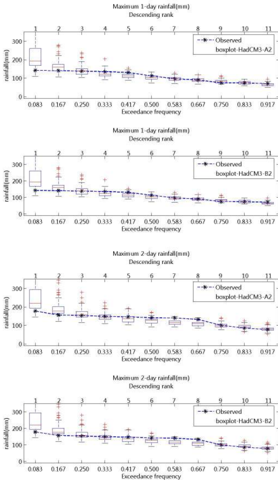
ภาพที่ จ.29 ความถี่ส่วนเกินของฝนรายวันสูงสุด 1- และ 2 วัน ของฝนรายวันอดีตและที่สังเคราะห์ได้จากภาพฉาย HadCM3-A2 และ HadCM3-B2 สำหรับสถานี 21190 (ปี ค.ศ.1991-2001)
