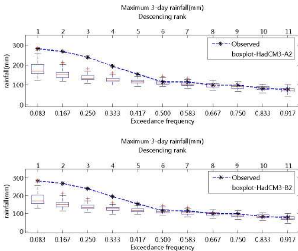
ภาพที่ จ.66 ความถี่ส่วนเกินของฝนรายวันสูงสุด 3 วัน ของฝนรายวันอดีตและที่สังเคราะห์ได้จาก ภาพฉาย HadCM3-A2 และ HadCM3-B2 สำหรับสถานี 409004 (ปี ค.ศ.1991-2001)
