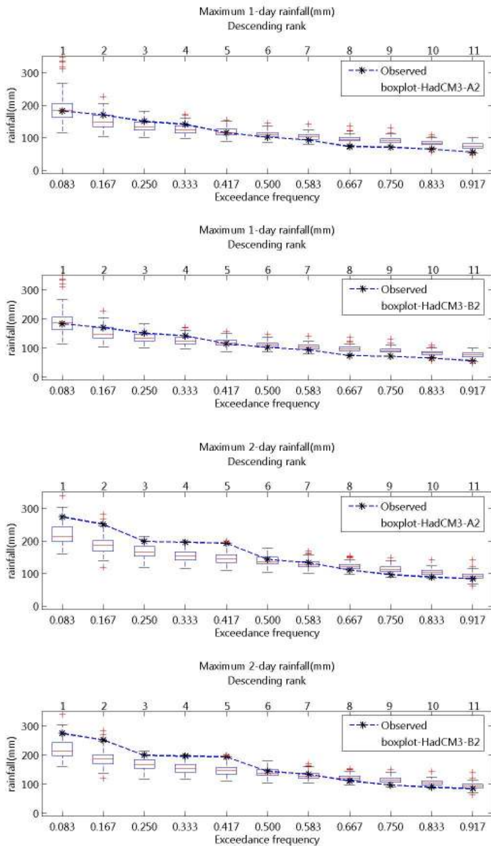
ภาพที่ จ.59 ความถี่ส่วนเกินของฝนรายวันสูงสุด 1- และ 2 วัน ของฝนรายวันอดีตและที่สังเคราะห์ได้จากภาพฉาย HadCM3-A2 และ HadCM3-B2 สำหรับสถานี 407006 (ปี ค.ศ.1991-2001)
