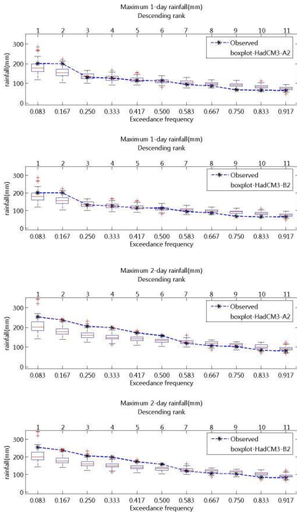
ภาพที่ จ.51 ความถี่ส่วนเกินของฝนรายวันสูงสุด 1- และ 2 วัน ของฝนรายวันอดีตและที่สังเคราะห์ได้จากภาพฉาย HadCM3-A2 และ HadCM3-B2 สำหรับสถานี 406002 (ปี ค.ศ.1991-2001)
