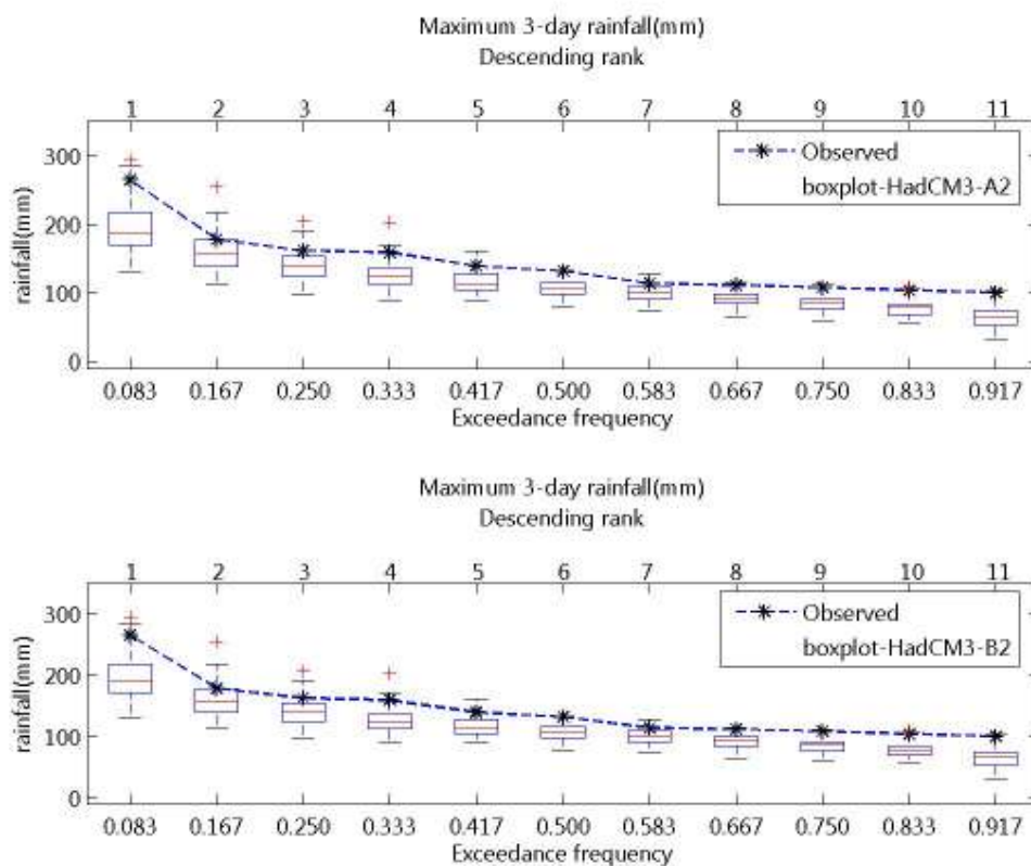
ภาพที่ ๑.๒๔ ความถี่ส่วนเกินของฝนรายวันสูงสุด 3 วัน ของฝนรายวันอดีตและที่สังเคราะห์ได้จาก ภาพฉาย HadCM3-A2 และ HadCM3-B2 สำหรับสถานี 14112 (ปี ค.ศ.1991-2001)
