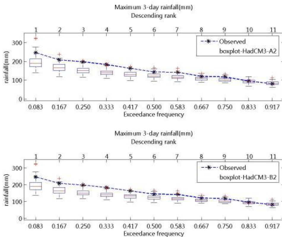
ภาพที่ ๑.36 ความถี่ส่วนเกินของฝนรายวันสูงสุด 3 วัน ของฝนรายวันอดีตและที่สังเคราะห์ได้จาก ภาพฉาย HadCM3-A2 และ HadCM3-B2 สำหรับสถานี 49301 (ปี ค.ศ.1991-2001)
