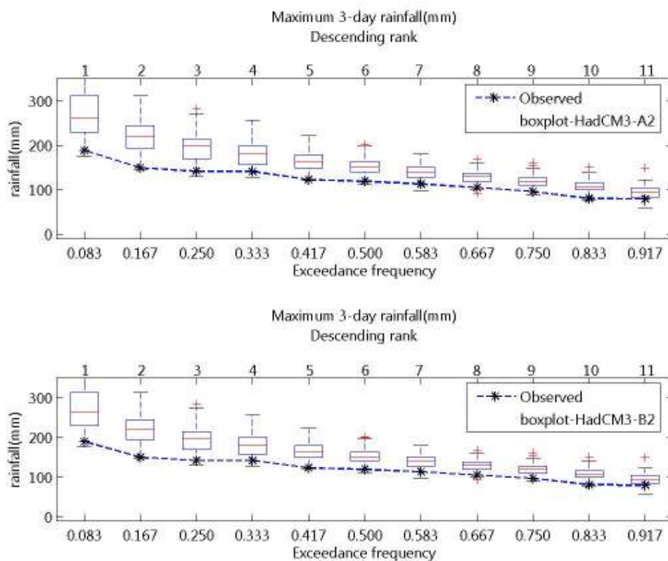
ภาพที่ จ.34 ความถี่ส่วนเกินของฝนรายวันสูงสุด 3 วัน ของฝนรายวันอดีตและที่สังเคราะห์ได้จาก ภาพฉาย HadCM3-A2 และ HadCM3-B2 สำหรับสถานี 49062 (ปี ค.ศ.1991-2001)
