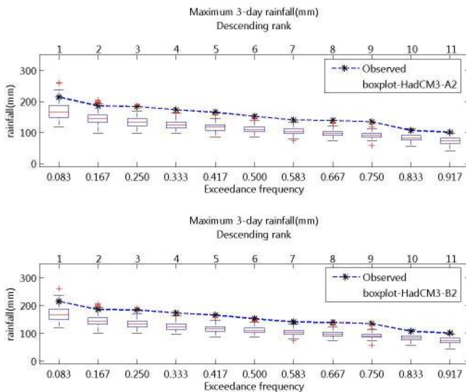
ภาพที่ จ.80 ความถี่ส่วนเกินของฝนรายวันสูงสุด 3 วัน ของฝนรายวันอดีตและที่สังเคราะห์ได้จาก ภาพฉาย HadCM3-A2 และ HadCM3-B2 สำหรับสถานี 436006 (ปี ค.ศ.1991-2001)
