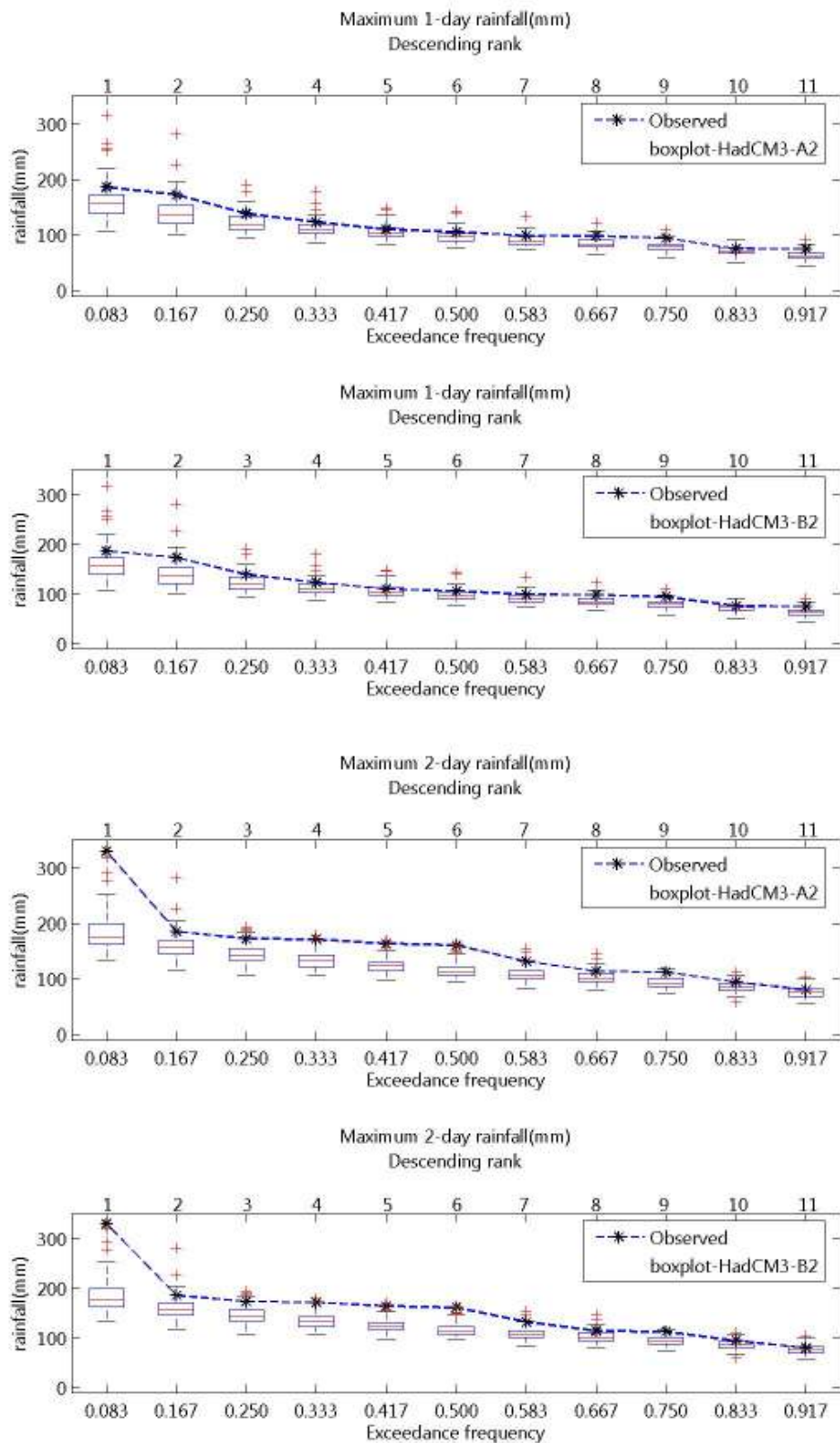
ภาพที่ จ.83 ความถี่ส่วนเกินของฝนรายวันสูงสุด 1- และ 2 วัน ของฝนรายวันอดีตและที่สังเคราะห์ได้จากภาพฉาย HadCM3-A2 และ HadCM3-B2 สำหรับสถานี 436013 (ปี ค.ศ.1991-2001)
