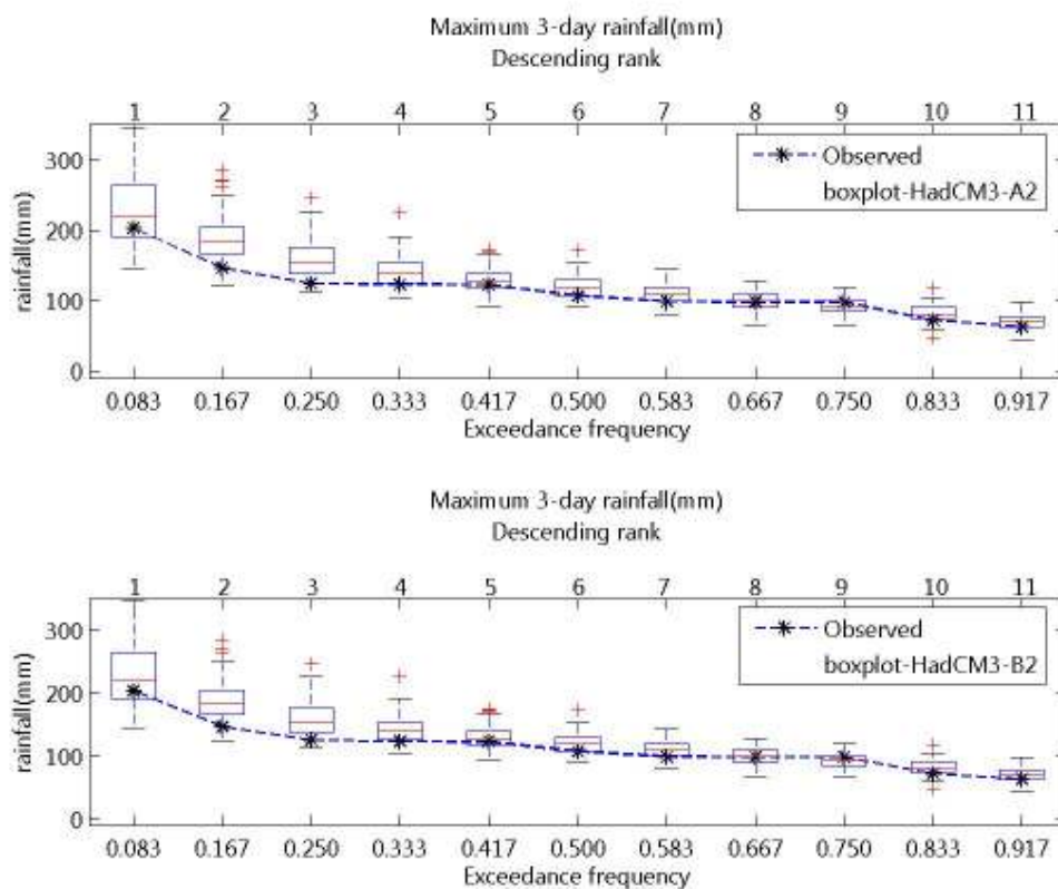
ภาพที่ จ.10 ความถี่ส่วนเกินของฝนรายวันสูงสุด 3 วัน ของฝนรายวันอดีตและที่สังเคราะห์ได้จาก ภาพฉาย HadCM3-A2 และ HadCM3-B2 สำหรับสถานี 05171 (ปี ค.ศ.1991-2001)
