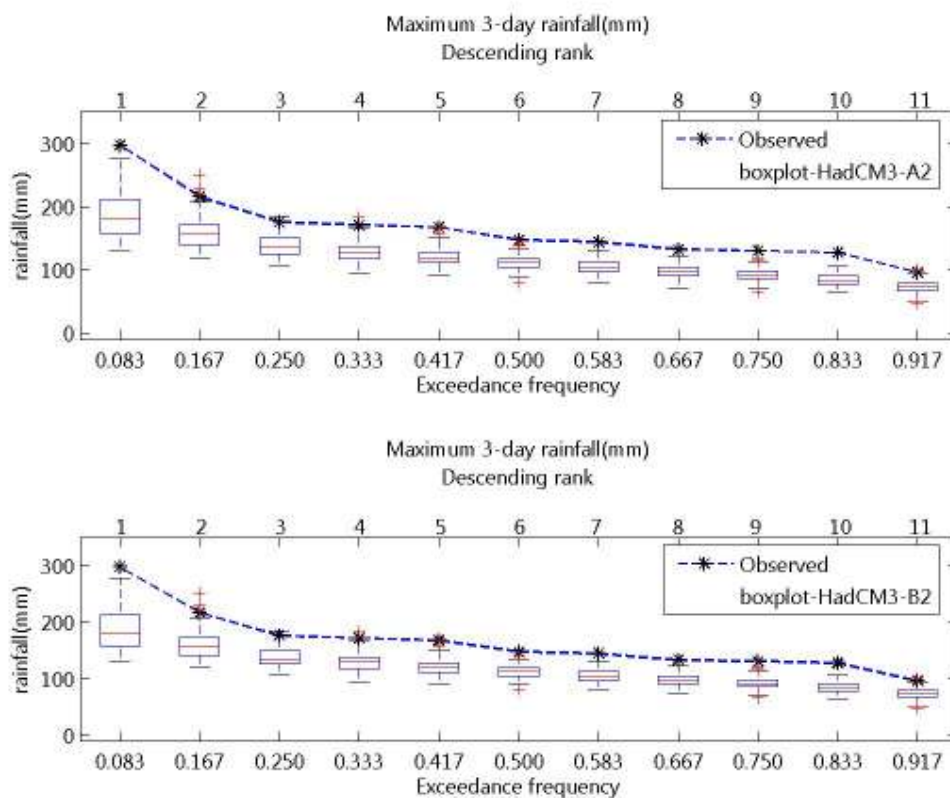
ภาพที่ จ.58 ความถี่ส่วนเกินของฝนรายวันสูงสุด 3 วัน ของฝนรายวันอดีตและที่สังเคราะห์ได้จาก ภาพฉาย HadCM3-A2 และ HadCM3-B2 สำหรับสถานี 407002 (ปี ค.ศ.1991-2001)
