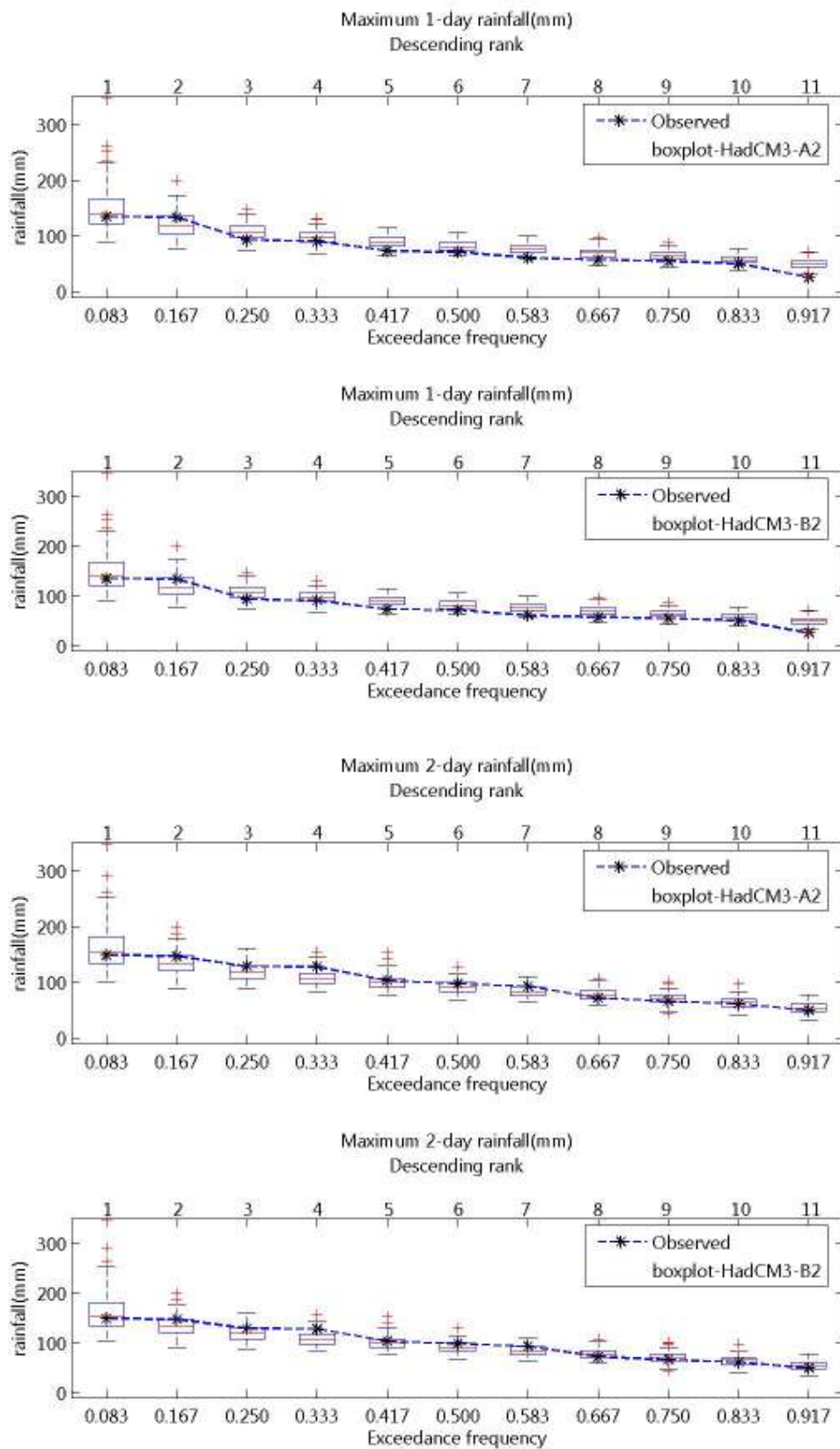
ภาพที่ จ.43 ความถี่ส่วนเกินของฝนรายวันสูงสุด 1- และ 2 วัน ของฝนรายวันอดีตและที่สังเคราะห์ได้จากภาพฉาย HadCM3-A2 และ HadCM3-B2 สำหรับสถานี 75052 (ปี ค.ศ.1991-2001)
