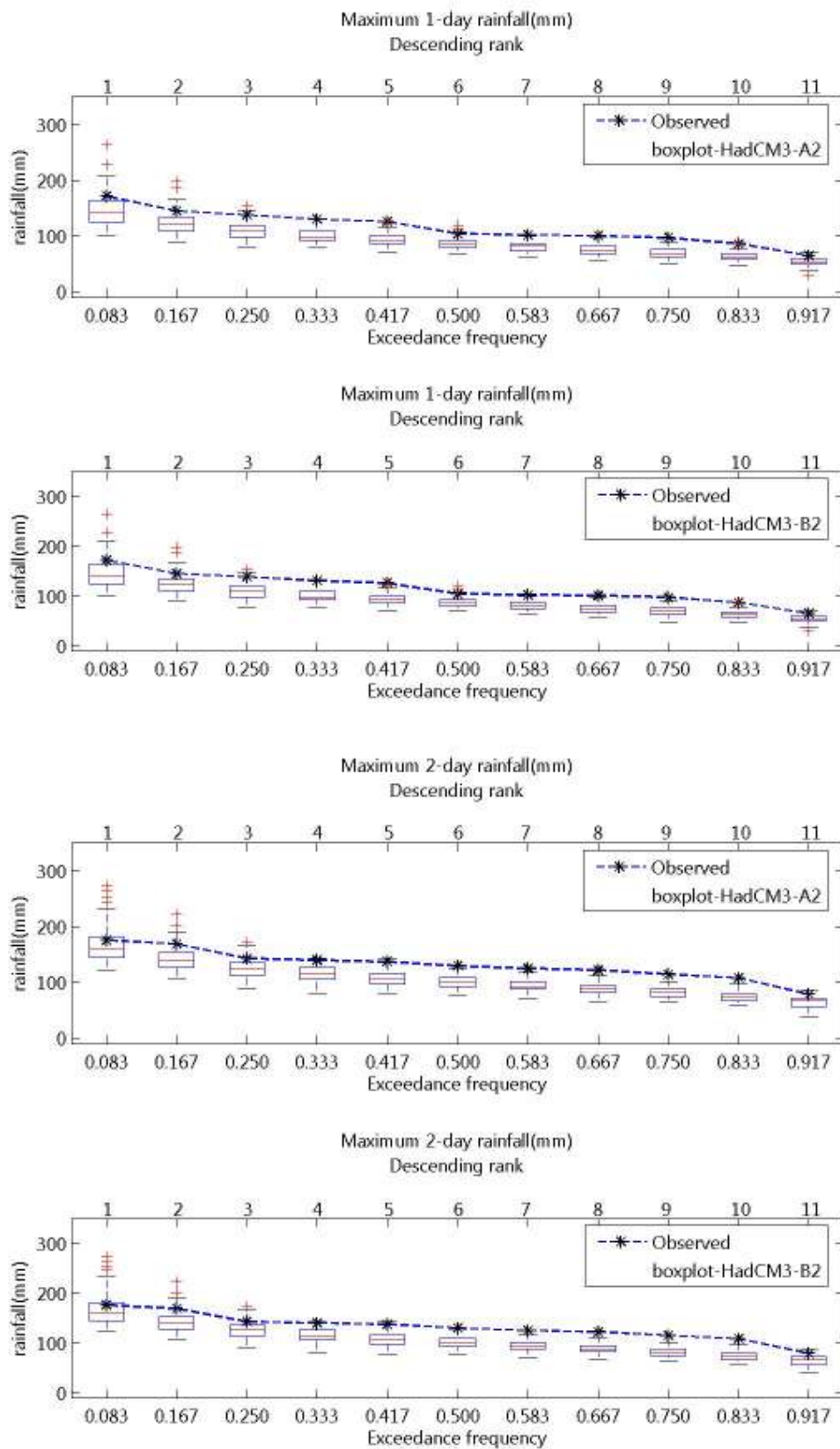
ภาพที่ จ.57 ความถี่ส่วนเกินของฝนรายวันสูงสุด 1- และ 2 วัน ของฝนรายวันอดีตและที่สังเคราะห์ได้จากภาพฉาย HadCM3-A2 และ HadCM3-B2 สำหรับสถานี 407002 (ปี ค.ศ.1991-2001)
