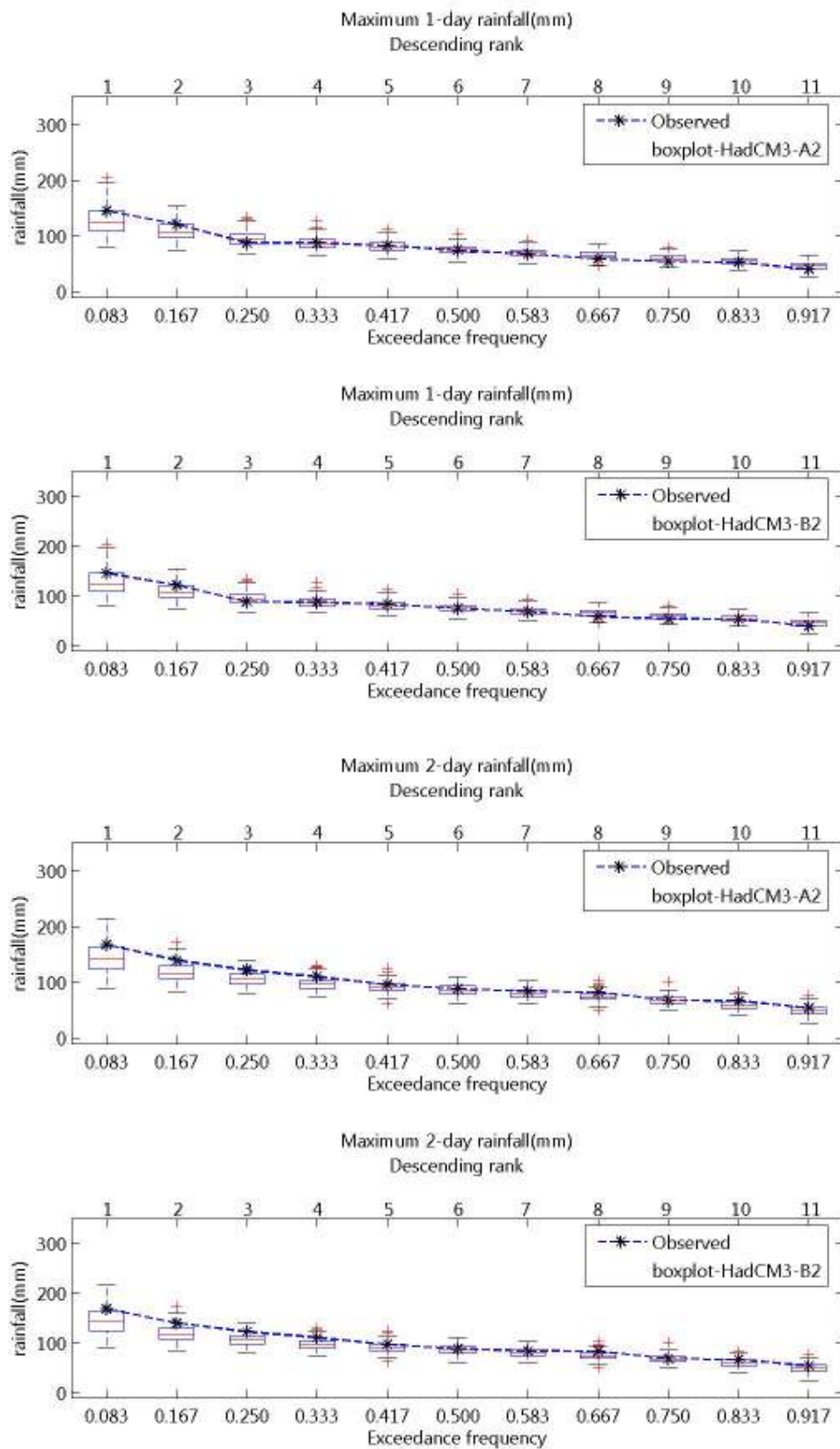
ภาพที่ จ.21 ความถี่ส่วนเกินของฝนรายวันสูงสุด 1- และ 2 วัน ของฝนรายวันอดีตและที่สังเคราะห์ได้จากภาพฉาย HadCM3-A2 และ HadCM3-B2 สำหรับสถานี 14062 (ปี ค.ศ.1991-2001)
