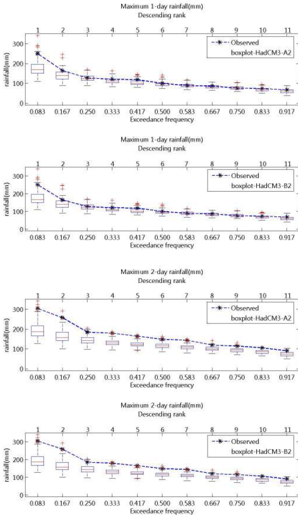
ภาพที่ จ.63 ความถี่ส่วนเกินของฝนรายวันสูงสุด 1- และ 2 วัน ของฝนรายวันอดีตและที่สังเคราะห์ได้จากภาพฉาย HadCM3-A2 และ HadCM3-B2 สำหรับสถานี 407015 (ปี ค.ศ.1991-2001)
