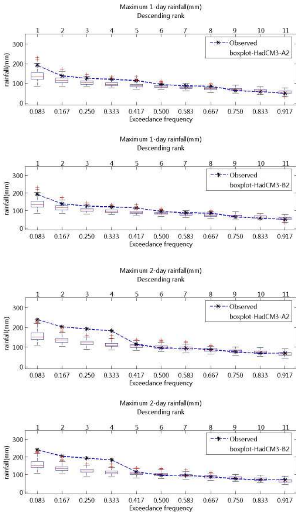
ภาพที่ จ.65 ความถี่ส่วนเกินของฝนรายวันสูงสุด 1- และ 2 วัน ของฝนรายวันอดีตและที่สังเคราะห์ได้จากภาพฉาย HadCM3-A2 และ HadCM3-B2 สำหรับสถานี 409004 (ปี ค.ศ.1991-2001)
