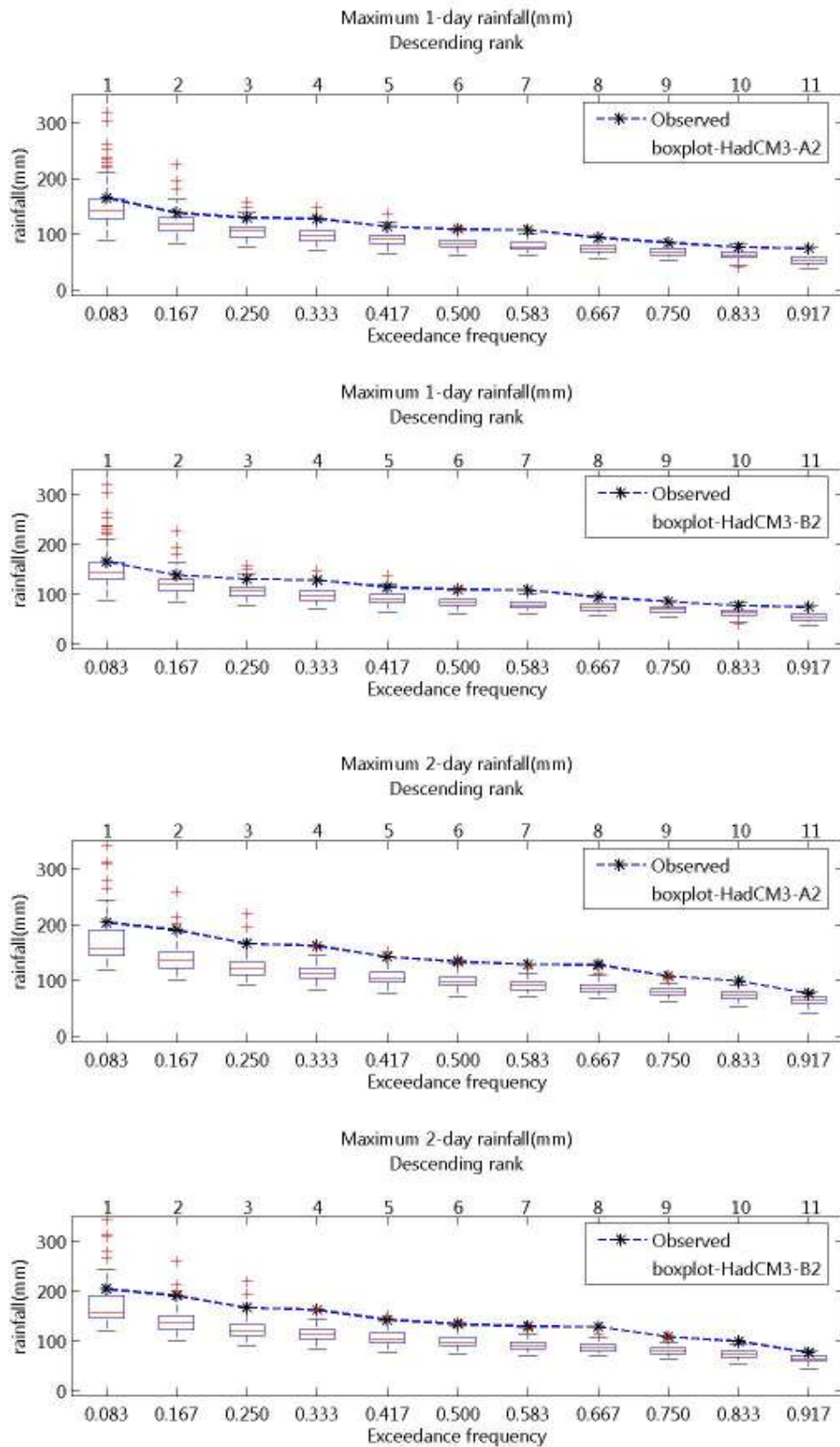
ภาพที่ จ.77 ความถี่ส่วนเกินของฝนรายวันสูงสุด 1- และ 2 วัน ของฝนรายวันอดีตและที่สังเคราะห์ได้จากภาพฉาย HadCM3-A2 และ HadCM3-B2 สำหรับสถานี 436005 (ปี ค.ศ.1991-2001)
