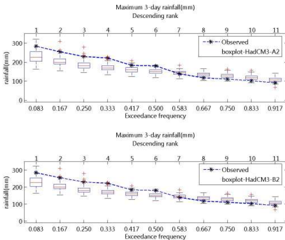
ภาพที่ จ.52 ความถี่ส่วนเกินของฝนรายวันสูงสุด 3 วัน ของฝนรายวันอดีตและที่สังเคราะห์ได้จาก ภาพฉาย HadCM3-A2 และ HadCM3-B2 สำหรับสถานี 406002 (ปี ค.ศ.1991-2001)
