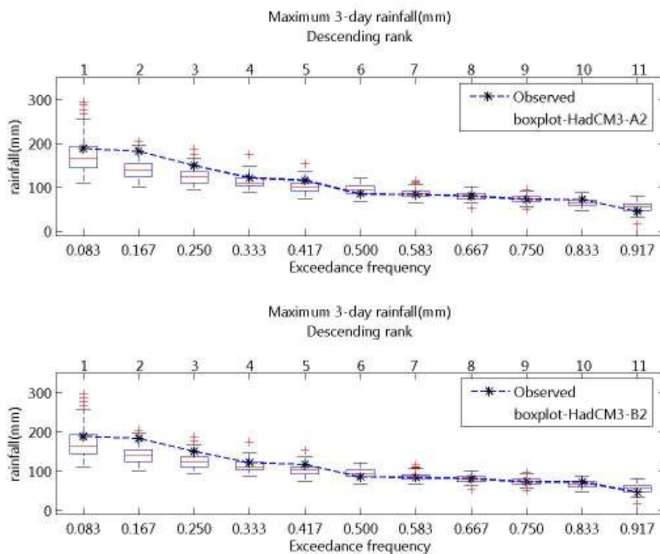
ภาพที่ ๑.๘ ความถี่ส่วนเกินของฝนรายวันสูงสุด 3 วัน ของฝนรายวันอดีตและที่สังเคราะห์ได้จากภาพฉาย HadCM3-A2 และ HadCM3-B2 สำหรับ 05092 (ปี ค.ศ.1991-2001)
