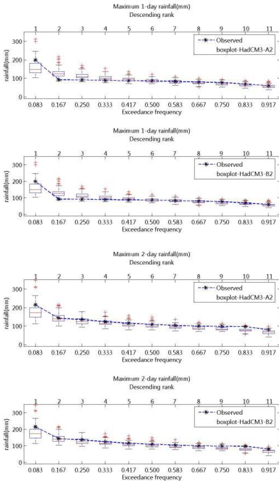
ภาพที่ จ.31 ความถี่ส่วนเกินของฝนรายวันสูงสุด 1- และ 2 วัน ของฝนรายวันอดีตและที่สังเคราะห์ได้จากภาพฉาย HadCM3-A2 และ HadCM3-B2 สำหรับสถานี 49013 (ปี ค.ศ.1991-2001)
