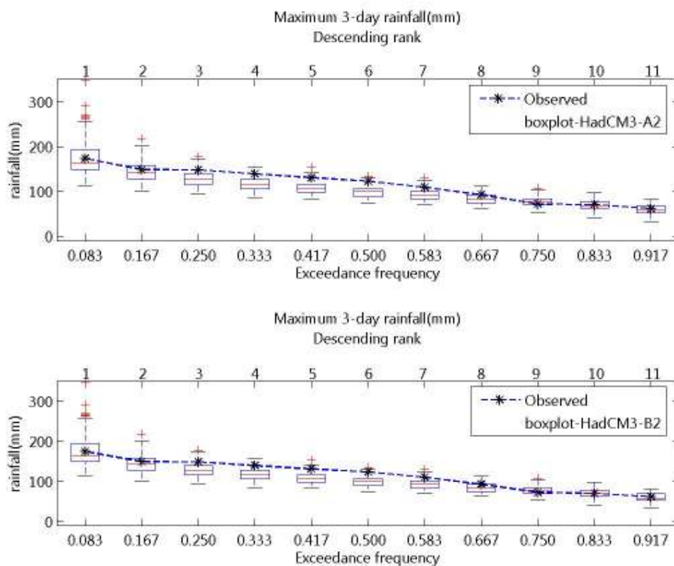
ภาพที่ จ.44 ความถี่ส่วนเกินของฝนรายวันสูงสุด 3 วัน ของฝนรายวันอดีตและที่สังเคราะห์ได้จาก ภาพฉาย HadCM3-A2 และ HadCM3-B2 สำหรับสถานี 75052 (ปี ค.ศ.1991-2001)
