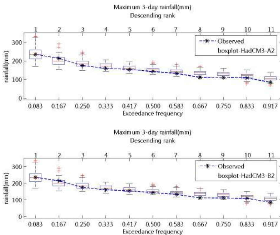
ภาพที่ จ.62 ความถี่ส่วนเกินของฝนรายวันสูงสุด 3 วัน ของฝนรายวันอดีตและที่สังเคราะห์ได้จาก ภาพฉาย HadCM3-A2 และ HadCM3-B2 สำหรับสถานี 407009 (ปี ค.ศ.1991-2001)
