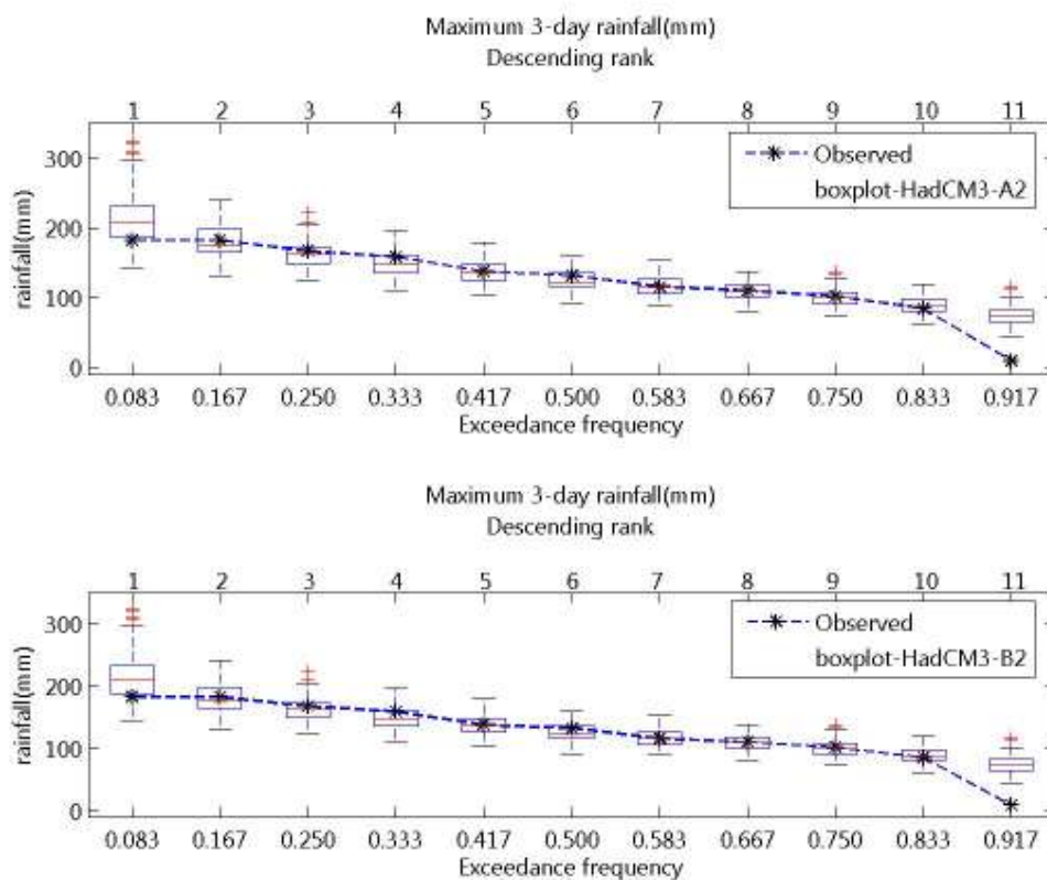
ภาพที่ จ.38 ความถี่ส่วนเกินของฝนรายวันสูงสุด 3 วัน ของฝนรายวันอดีตและที่สังเคราะห์ได้จาก ภาพถ่าย HadCM3-A2 และ HadCM3-B2 สำหรับสถานี 68150 (ปี ค.ศ.1991-2001)
