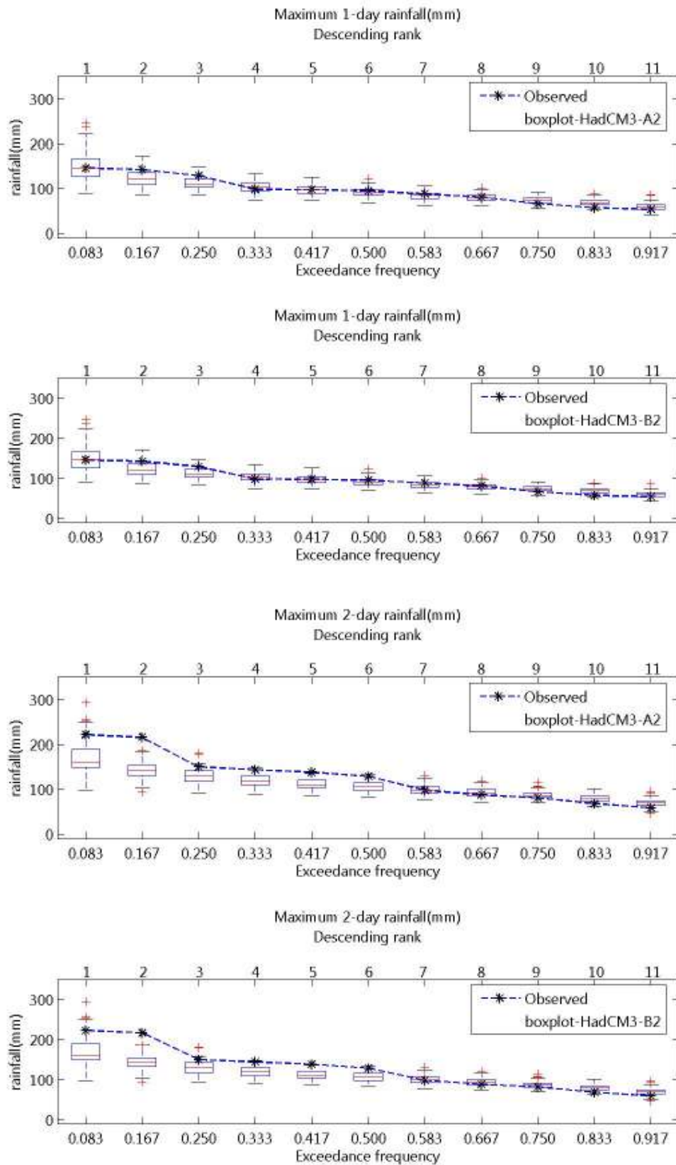
ภาพที่ จ.75 ความถี่ส่วนเกินของฝนรายวันสูงสุด 1- และ 2 วัน ของฝนรายวันอดีตและที่สังเคราะห์ได้จากภาพฉาย HadCM3-A2 และ HadCM3-B2 สำหรับสถานี 436004 (ปี ค.ศ.1991-2001)
