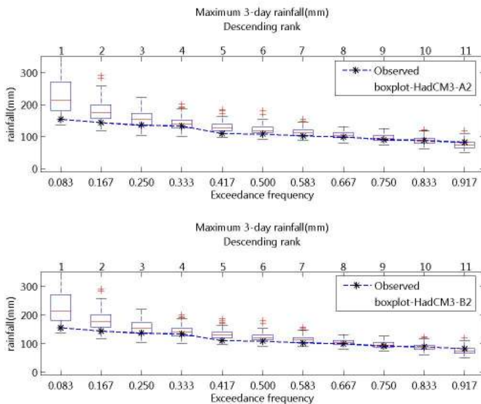
ภาพที่ ๑.๔ ความถี่ส่วนเกินของฝนรายวันสูงสุด 3 วัน ของฝนรายวันอดีตและที่สังเคราะห์ได้จากภาพถ่าย HadCM3-A2 และ HadCM3-B2 สำหรับสถานี 05023 (ปี ค.ศ.1991-2001)
