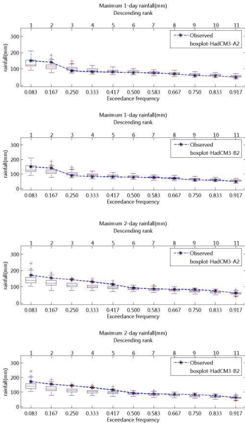
ภาพที่ จ.5 ความถี่ส่วนเกินของฝนรายวันสูงสุด 1- และ 2 วัน ของฝนรายวันอดีตและที่สังเคราะห์ได้ จากภาพฉาย HadCM3-A2 และ HadCM3-B2 สำหรับสถานี 05032 (ปี ค.ศ.1991-2001)
