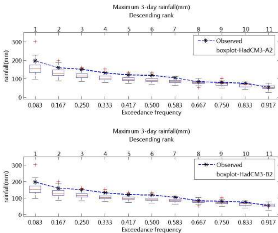
ภาพที่ จ.22 ความถี่ส่วนเกินของฝนรายวันสูงสุด 3 วัน ของฝนรายวันอดีตและที่สังเคราะห์ได้จาก ภาพฉาย HadCM3-A2 และ HadCM3-B2 สำหรับสถานี 14062 (ปี ค.ศ.1991-2001)
