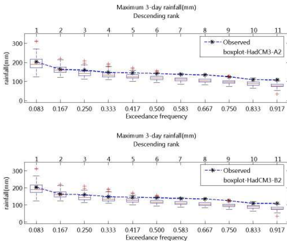
ภาพที่ จ.70 ความถี่ส่วนเกินของฝนรายวันสูงสุด 3 วัน ของฝนรายวันอดีตและที่สังเคราะห์ได้จาก ภาพฉาย HadCM3-A2 และ HadCM3-B2 สำหรับสถานี 432004 (ปี ค.ศ.1991-2001)
