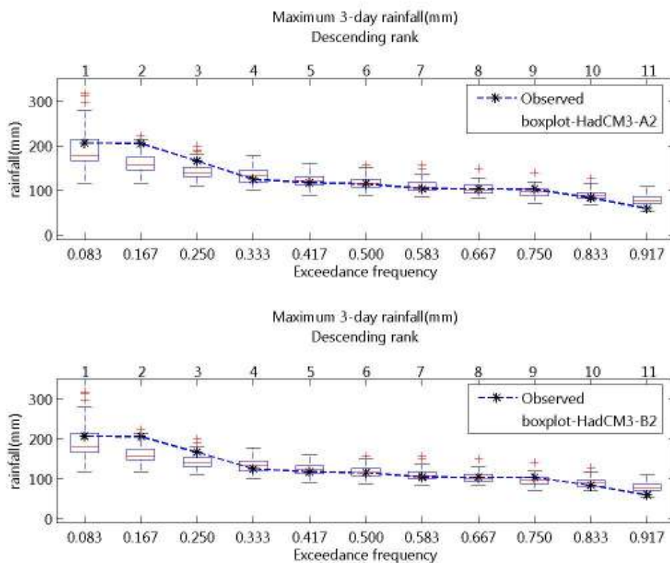
ภาพที่ จ.26 ความถี่ส่วนเกินของฝนรายวันสูงสุด 3 วัน ของฝนรายวันอดีตและที่สังเคราะห์ได้จาก ภาพฉาย HadCM3-A2 และ HadCM3-B2 สถานี 18073 (ปี ค.ศ.1991-2001)
