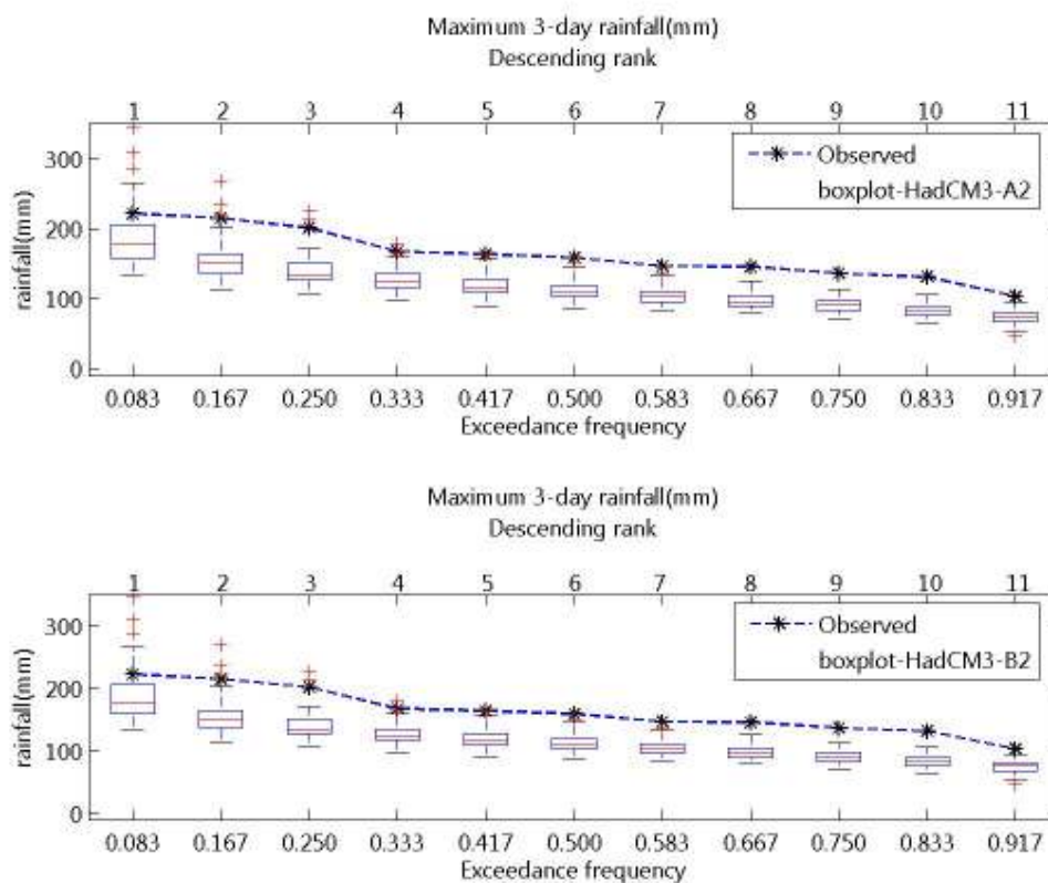
ภาพที่ จ.78 ความถี่ส่วนเกินของฝนรายวันสูงสุด 3 วัน ของฝนรายวันอดีตและที่สังเคราะห์ได้จาก ภาพฉาย HadCM3-A2 และ HadCM3-B2 สำหรับสถานี 436005 (ปี ค.ศ.1991-2001)
