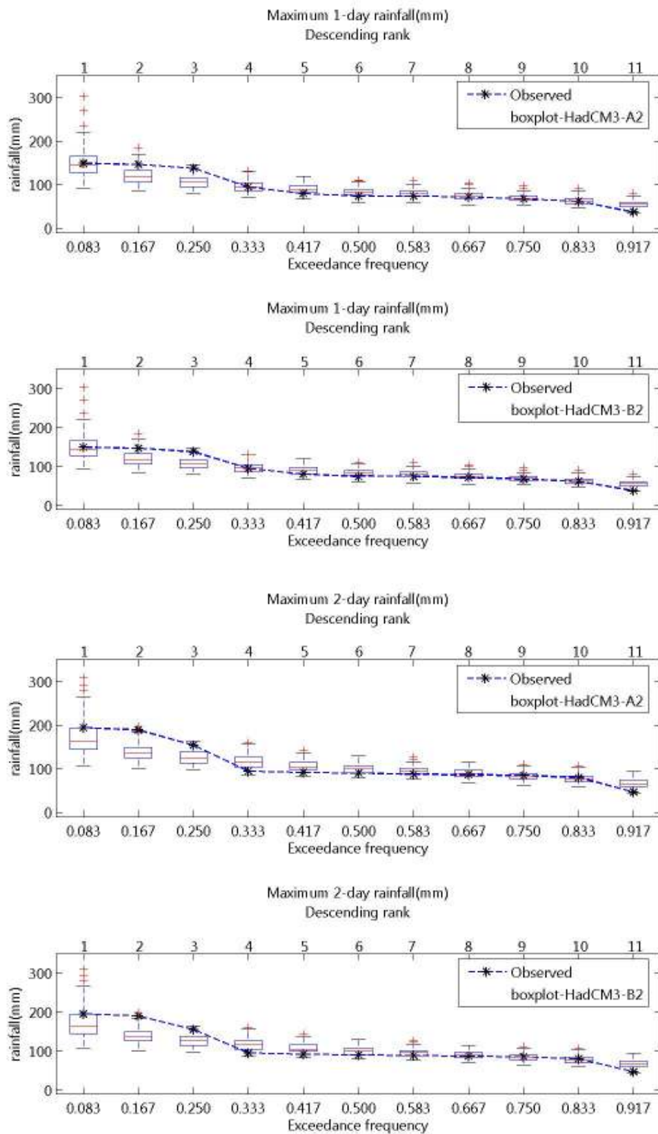
ภาพที่ จ.25 ความถี่ส่วนเกินของฝนรายวันสูงสุด 1- และ 2 วัน ของฝนรายวันอดีตและที่สังเคราะห์ได้จากภาพฉาย HadCM3-A2 และ HadCM3-B2 สถานี 18073 (ปี ค.ศ.1991-2001)
