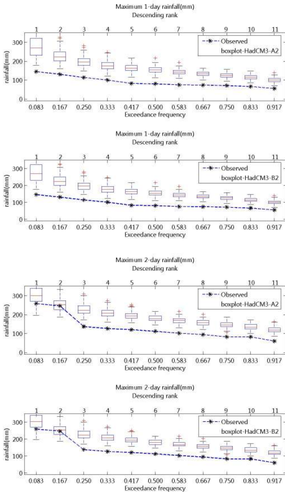
ภาพที่ จ.55 ปริมาณฝนสูงสุด 1 วัน และ 2 วัน ของฝนรายวันอดีตและที่สังเคราะห์ได้จากภาพถ่าย HadCM3-A2 และ HadCM3-B2 สำหรับสถานี 406005 (ปี ค.ศ.1991-2001)
