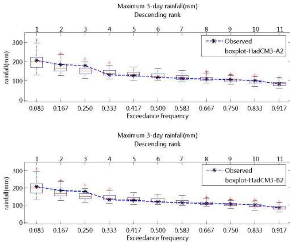
ภาพที่ จ.50 ความถี่ส่วนเกินของฝนรายวันสูงสุด 3 วัน ของฝนรายวันอดีตและที่สังเคราะห์ได้จาก ภาพฉาย HadCM3-A2 และ HadCM3-B2 สำหรับสถานี 405008 (ปี ค.ศ.1991-2001)
