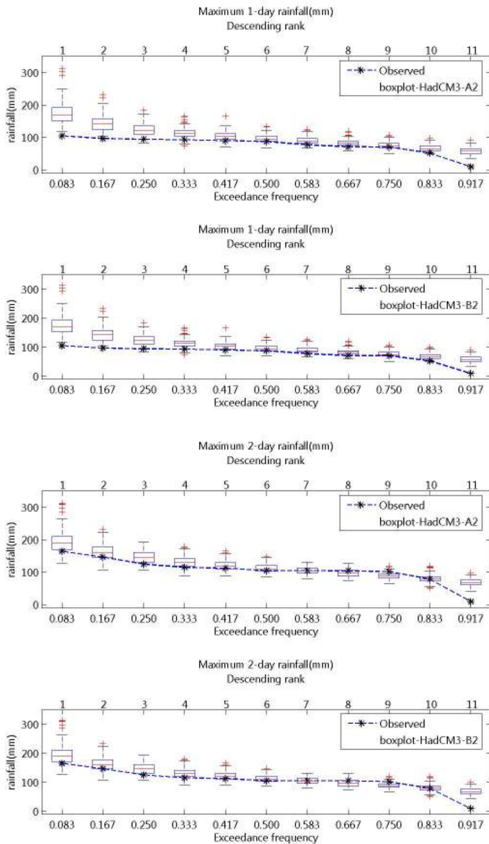
ภาพที่ จ.37 ความถี่ส่วนเกินของฝนรายวันสูงสุด 1- และ 2 วัน ของฝนรายวันอดีตและที่สังเคราะห์ได้จากภาพฉาย HadCM3-A2 และ HadCM3-B2 สำหรับสถานี 68150 (ปี ค.ศ.1991-2001)
