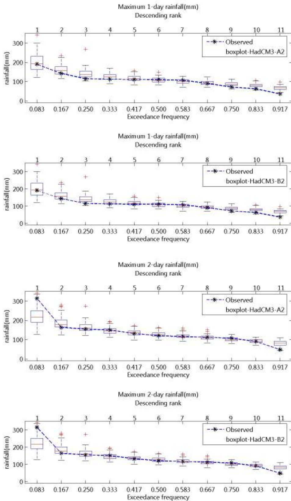
ภาพที่ จ.17 ความถี่ส่วนเกินของฝนรายวันสูงสุด 1- และ 2 วัน ของฝนรายวันอดีตและที่สังเคราะห์ได้จากภาพฉาย HadCM3-A2 และ HadCM3-B2 สำหรับสถานี 11210 (ปี ค.ศ.1991-2001)
