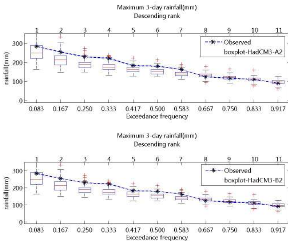
ภาพที่ จ.40 ความถี่ส่วนเกินของฝนรายวันสูงสุด 3 วัน ของฝนรายวันอดีตและที่สังเคราะห์ได้จาก ภาพฉาย HadCM3-A2 และ HadCM3-B2 สำหรับสถานี 72022 (ปี ค.ศ.1991-2001)
