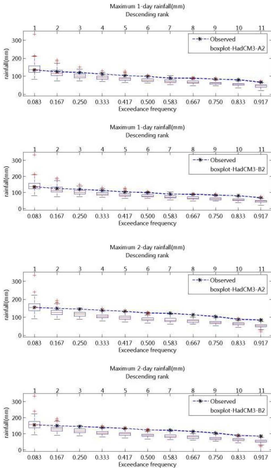
ภาพที่ จ.27 ความถี่ส่วนเกินของฝนรายวันสูงสุด 1- และ 2 วัน ของฝนรายวันอดีตและที่สังเคราะห์ได้จากภาพฉาย HadCM3-A2 และ HadCM3-B2 สถานี 21043 (ปี ค.ศ.1991-2001)
