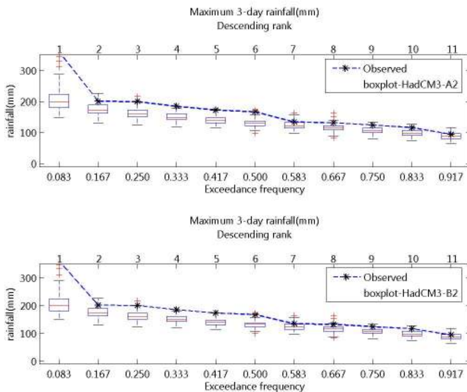
ภาพที่ ๑.๘๔ ความถี่ส่วนเกินของฝนรายวันสูงสุด 3 วัน ของฝนรายวันอดีตและที่สังเคราะห์ได้จาก ภาพฉาย HadCM3-A2 และ HadCM3-B2 สำหรับสถานี 436013 (ปี ค.ศ.1991-2001)
