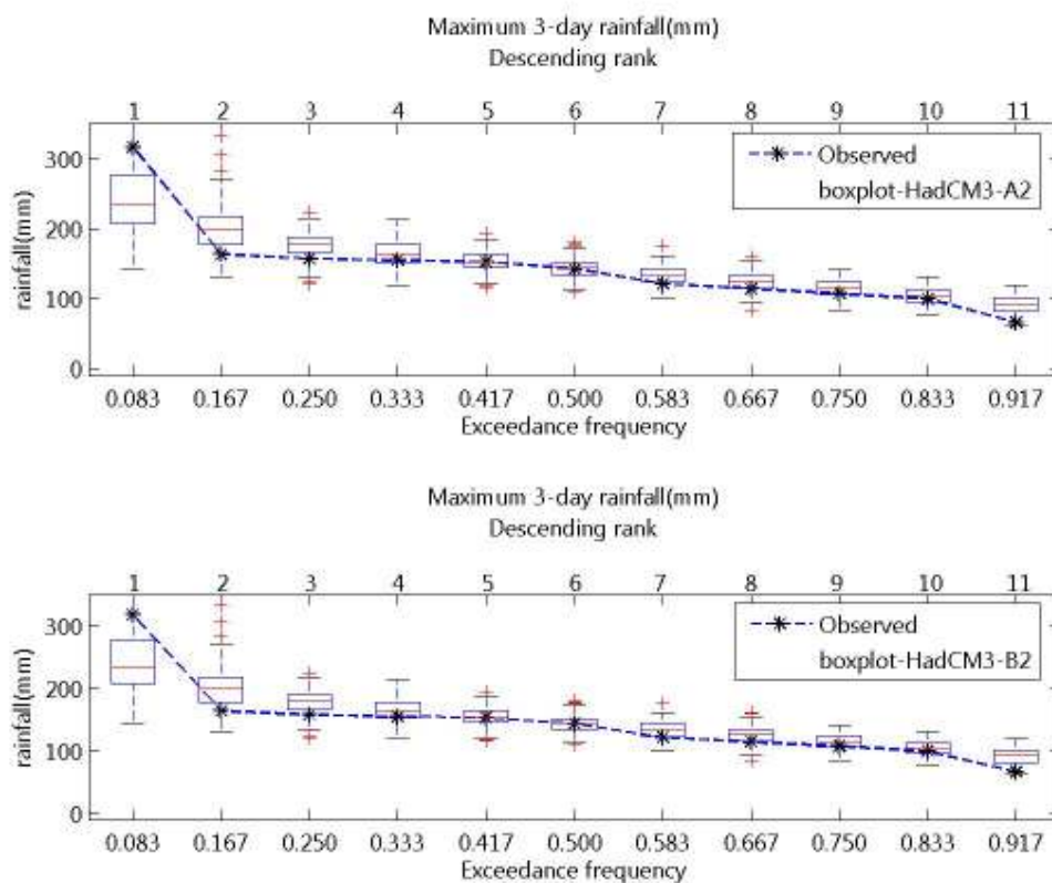
ภาพที่ จ.18 ความถี่ส่วนเกินของฝนรายวันสูงสุด 3 วัน ของฝนรายวันอดีตและที่สังเคราะห์ได้จาก ภาพฉาย HadCM3-A2 และ HadCM3-B2 สำหรับสถานี 11210 (ปี ค.ศ.1991-2001)
