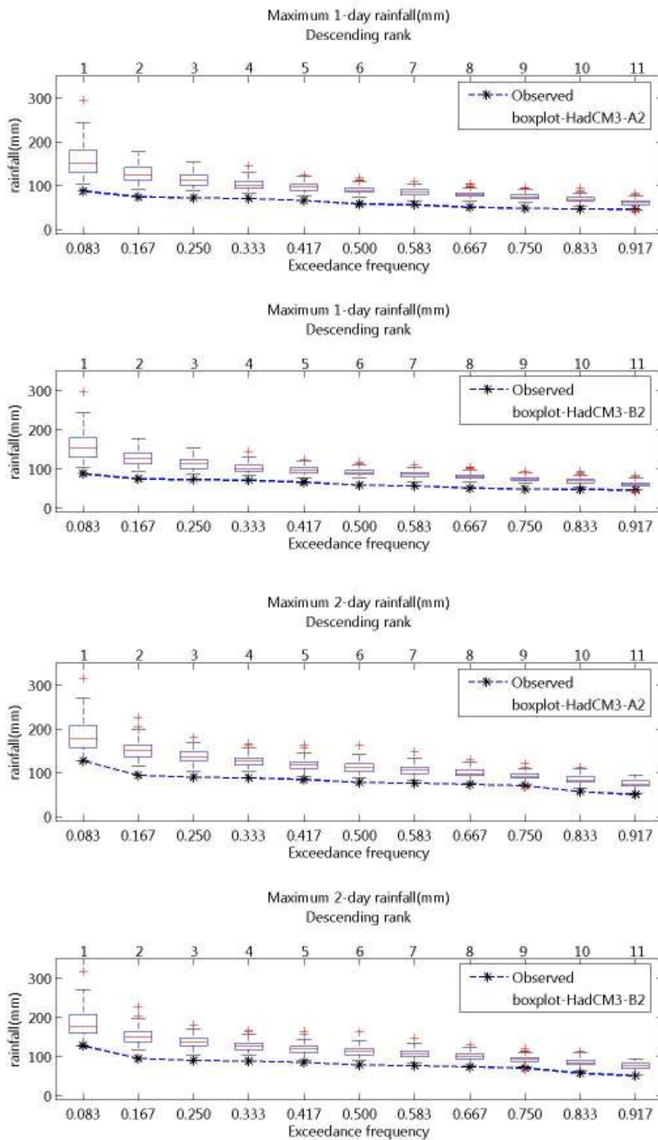
ภาพที่ จ.41 ความถี่ส่วนเกินของฝนรายวันสูงสุด 1- และ 2 วัน ของฝนรายวันอดีตและที่สังเคราะห์ได้จากภาพฉาย HadCM3-A2 และ HadCM3-B2 สถานี 75032 (ปี ค.ศ.1991-2001)
