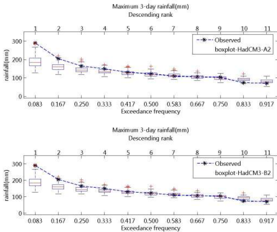
ภาพที่ จ.14 ความถี่ส่วนเกินของฝนรายวันสูงสุด 3 วัน ของฝนรายวันอดีตและที่สังเคราะห์ได้จาก ภาพฉาย HadCM3-A2 และ HadCM3-B2 สำหรับสถานี 11170 (ปี ค.ศ.1991-2001)
