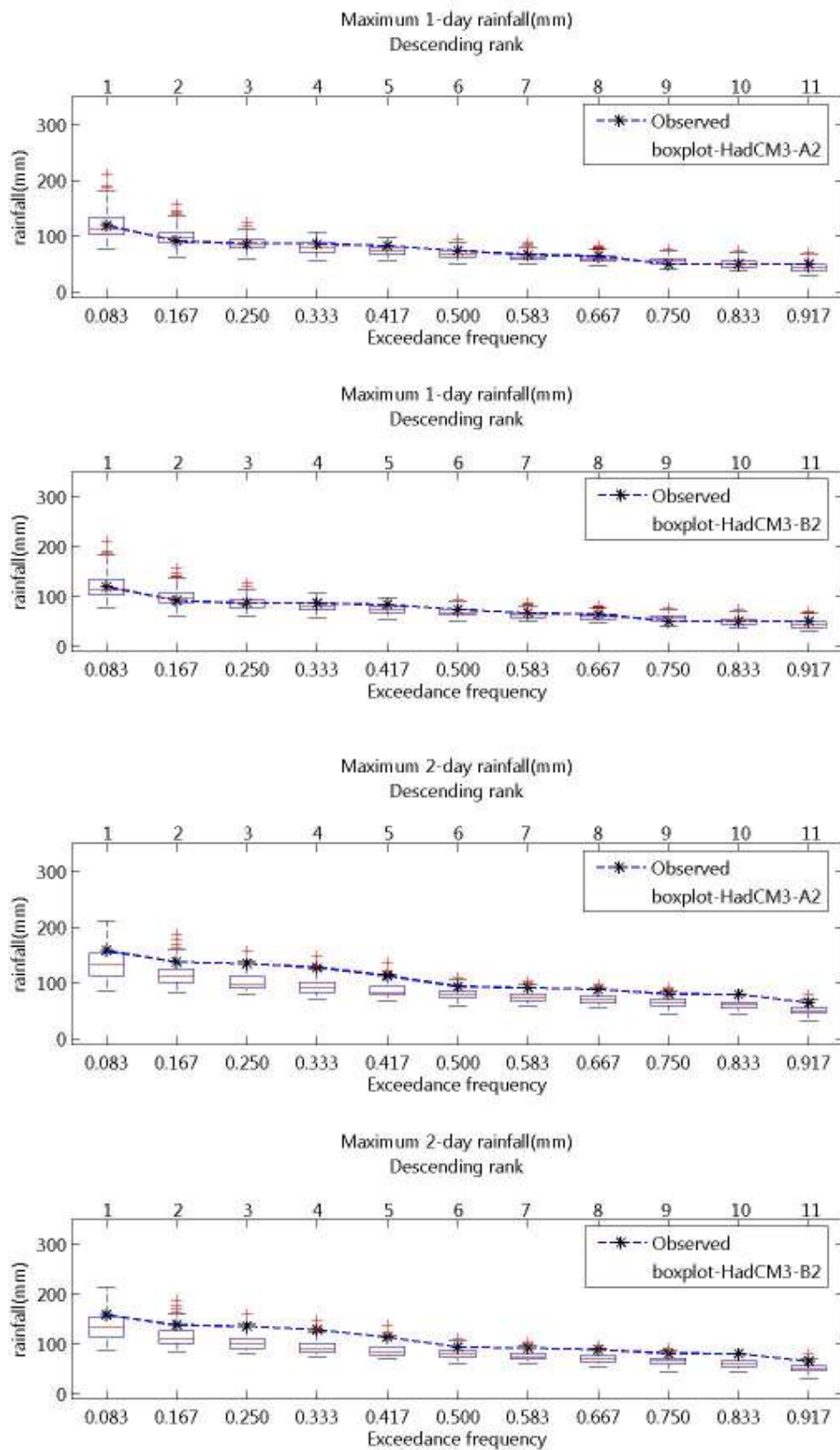
ภาพที่ จ.19 ความถี่ส่วนเกินของฝนรายวันสูงสุด 1- และ 2 วัน ของฝนรายวันอดีตและที่สังเคราะห์ได้จากภาพฉาย HadCM3-A2 และ HadCM3-B2 สำหรับสถานี 14052 (ปี ค.ศ.1991-2001)
