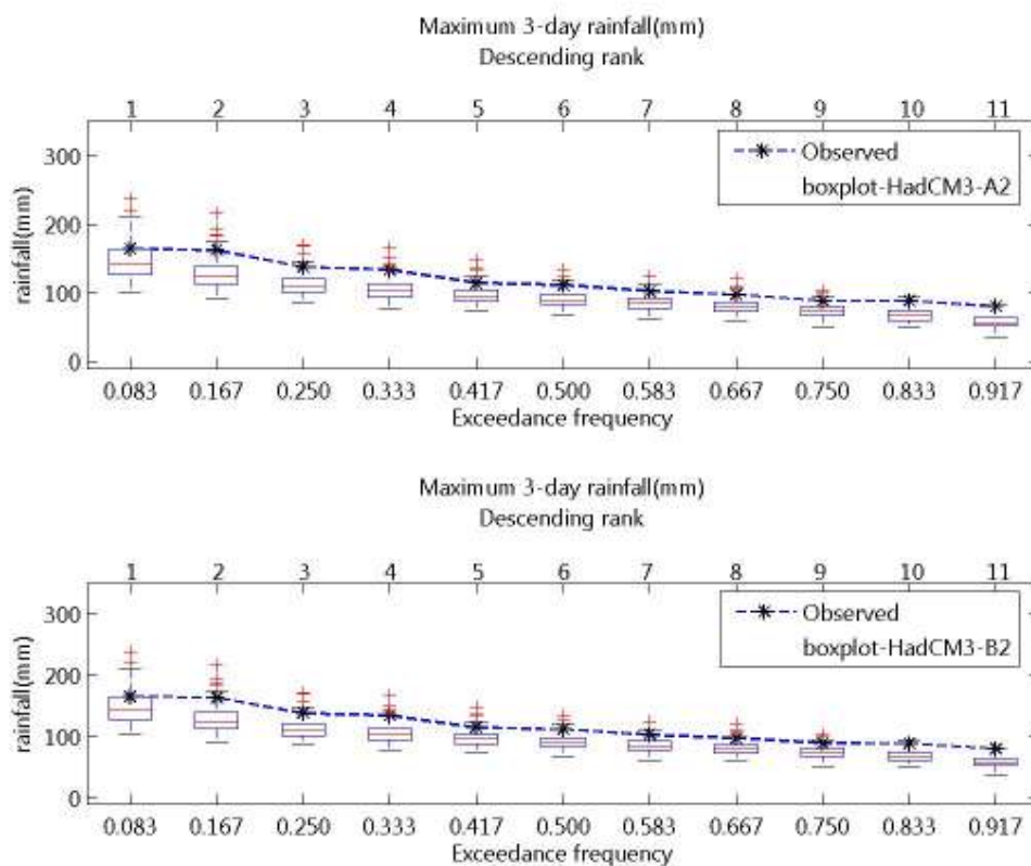
ภาพที่ จ.20 ความถี่ส่วนเกินของฝนรายวันสูงสุด 3 วัน ของฝนรายวันอดีตและที่สังเคราะห์ได้จาก ภาพฉาย HadCM3-A2 และ HadCM3-B2 สำหรับสถานี 14052 (ปี ค.ศ.1991-2001)
