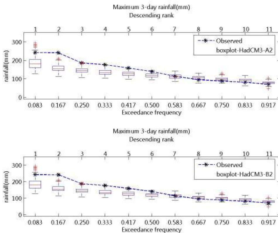
ภาพที่ จ.76 ความถี่ส่วนเกินของฝนรายวันสูงสุด 3 วัน ของฝนรายวันอดีตและที่สังเคราะห์ได้จาก ภาพฉาย HadCM3-A2 และ HadCM3-B2 สำหรับสถานี 436004 (ปี ค.ศ.1991-2001)
