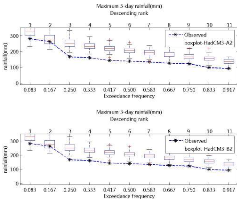
ภาพที่ จ.56 ความถี่ส่วนเกินของฝนรายวันสูงสุด 3 วัน ของฝนรายวันอดีตและที่สังเคราะห์ได้จาก ภาพฉาย HadCM3-A2 และ HadCM3-B2 สำหรับสถานี 406005 (ปี ค.ศ.1991-2001)
