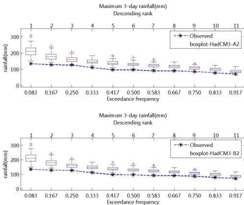
ภาพที่ จ.42ความถี่ส่วนเกินของฝนรายวันสูงสุด 3 วัน ของฝนรายวันอดีตและที่สังเคราะห์ได้จาก ภาพฉาย HadCM3-A2 และ HadCM3-B2 สถานี 75032 (ปี ค.ศ.1991-2001)
