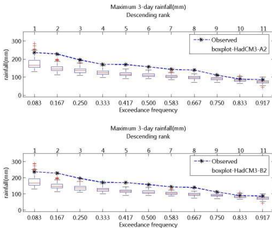
ภาพที่ จ.46 ความถี่ส่วนเกินของฝนรายวันสูงสุด 3 วัน ของฝนรายวันอดีตและที่สังเคราะห์ได้จาก ภาพถ่าย HadCM3-A2 และ HadCM3-B2 สถานี 404003 (ปี ค.ศ.1991-2001)
