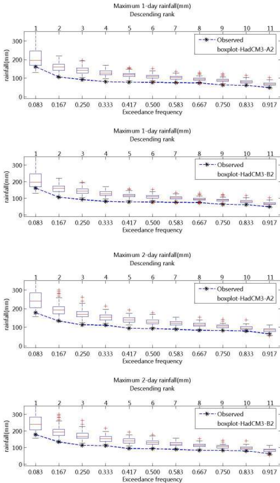
ภาพที่ จ.15 ความถี่ส่วนเกินของฝนรายวันสูงสุด 1- และ 2 วัน ของฝนรายวันอดีตและที่สังเคราะห์ได้จากภาพฉาย HadCM3-A2 และ HadCM3-B2 สำหรับสถานี 11202 (ปี ค.ศ.1991-2001)
