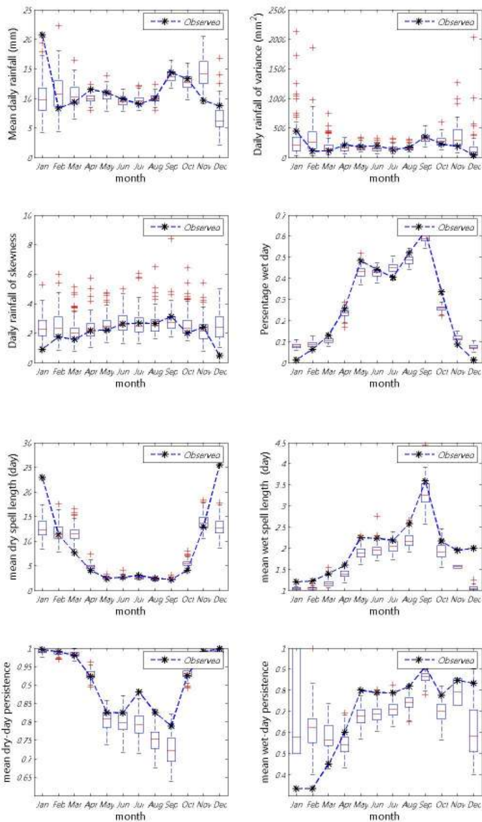
ภาพที่ ข.9 ค่าเฉลี่ย ความแปรปรวน สัมประสิทธิ์ความเบ้ เปอร์เซนต์ที่ฝนตก ช่วงเวลาที่ฝนหยุดและตก และจำนวนครั้งสัมพัทธ์ที่ฝนหยุดและตก ของข้อมูลฝนรายวันอดีตกับข้อมูลสังเคราะห์ สำหรับสถานี 05171 (ปี ค.ศ. 1976-1990)
