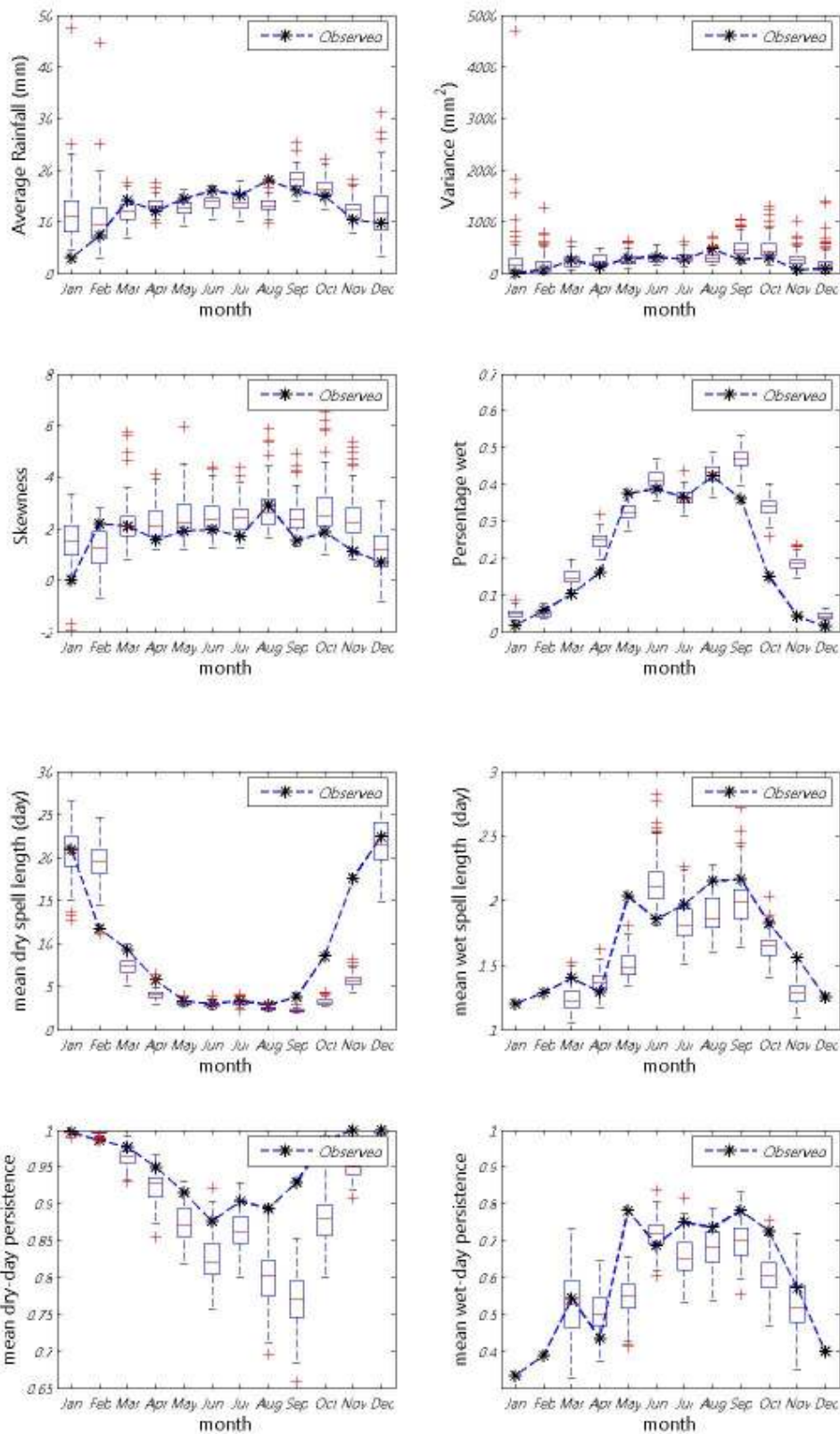
ภาพที่ ข.12 ค่าเฉลี่ย ความแปรปรวน สัมประสิทธิ์ความเบ้ เปอร์เซ็นต์ที่ฝนตก ช่วงเวลาที่ฝนหยุดและตก และจำนวนครั้งสัมผัสที่ฝนหยุดและตก ของข้อมูลฝนรายวันอดีตกับข้อมูลสังเคราะห์สำหรับสถานี 11022 (ปี ค.ศ.1991-2001)
