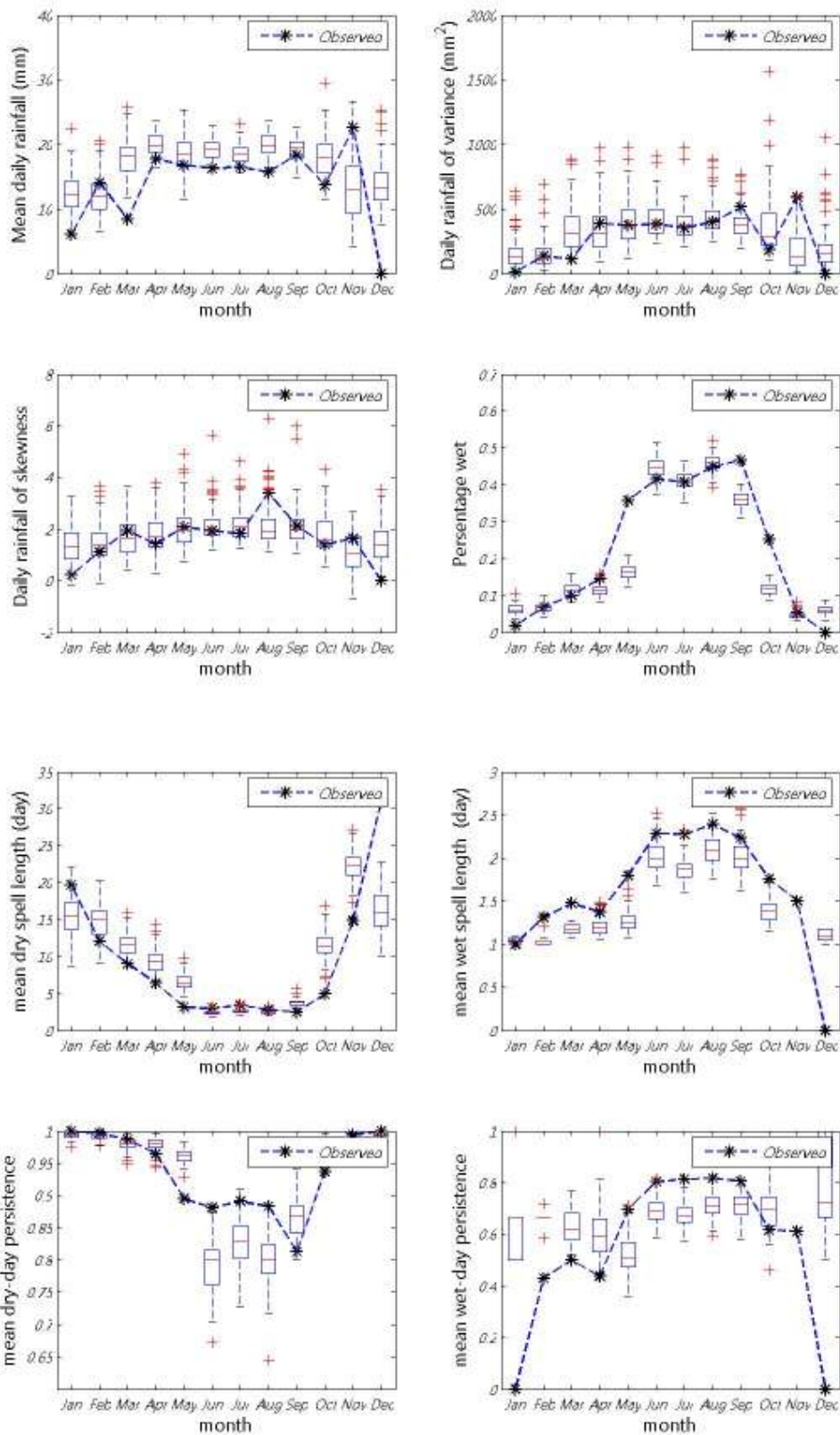
ภาพที่ ข.70 ค่าเฉลี่ย ความแปรปรวน สัมประสิทธิ์ความเบ้ เปอร์เซ็นต์ที่ฝนตก ช่วงเวลาที่ฝนหยุดและตก และจำนวนครั้งสัมผัสที่ฝนหยุดและตก ของข้อมูลฝนรายวันอดีตกับข้อมูลสังเคราะห์สำหรับสถานี 432004 (ปี ค.ศ.1991-2001)
