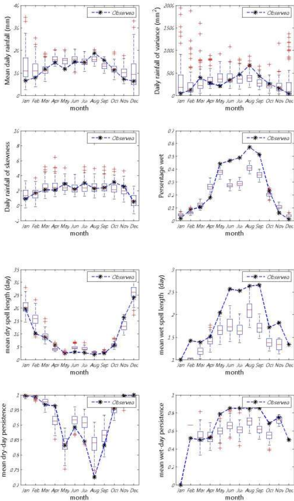
ภาพที่ ข.36 ค่าเฉลี่ย ความแปรปรวน สัมประสิทธิ์ความเบ้ เปอร์เซ็นต์ที่ฝนตก ช่วงเวลาที่ฝนหยุดและตก และจำนวนครั้งสัมผัสที่ฝนหยุดและตก ของข้อมูลฝนรายวันอดีตกับข้อมูลสังเคราะห์สำหรับสถานี 49301 (ปี ค.ศ.1991-2001)
