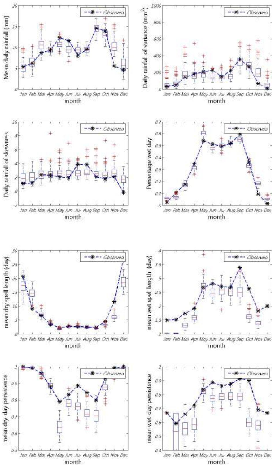
ภาพที่ ข.25 ค่าเฉลี่ย ความแปรปรวน สัมประสิทธิ์ความเบ้ เปอร์เซ็นต์ที่ฝนตก ช่วงเวลาที่ฝนหยุดและตก และจำนวนครั้งสัมผัสที่ฝนหยุดและตก ของข้อมูลฝนรายวันอดีตกับข้อมูลสังเคราะห์สำหรับสถานี 18073 (ปี ค.ศ. 1976-1990)
