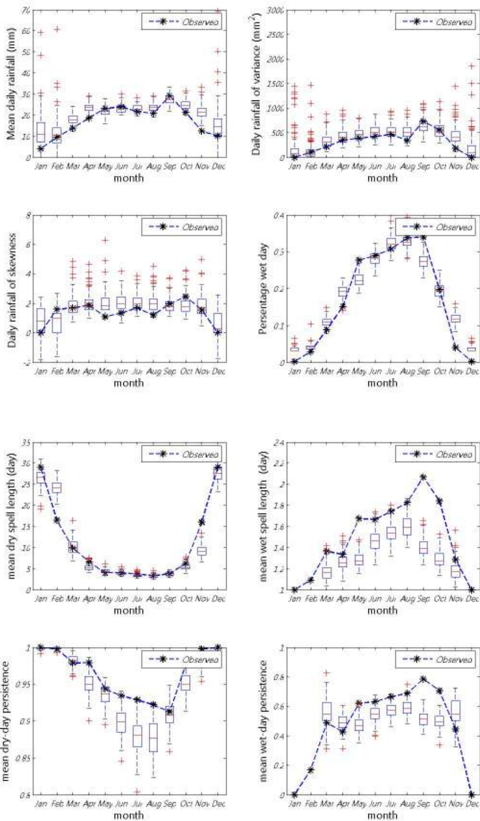
ภาพที่ ข.73 ค่าเฉลี่ย ความแปรปรวน สัมประสิทธิ์ความเบ้ เปอร์เซนต์ที่ฝนตก ช่วงเวลาที่ฝนหยุดและตก และจำนวนครั้งสัมผัสที่ฝนหยุดและตก ของข้อมูลฝนรายวันอดีตกับข้อมูลสังเคราะห์สำหรับสถานี 432006 (ปี ค.ศ. 1976-1990)
