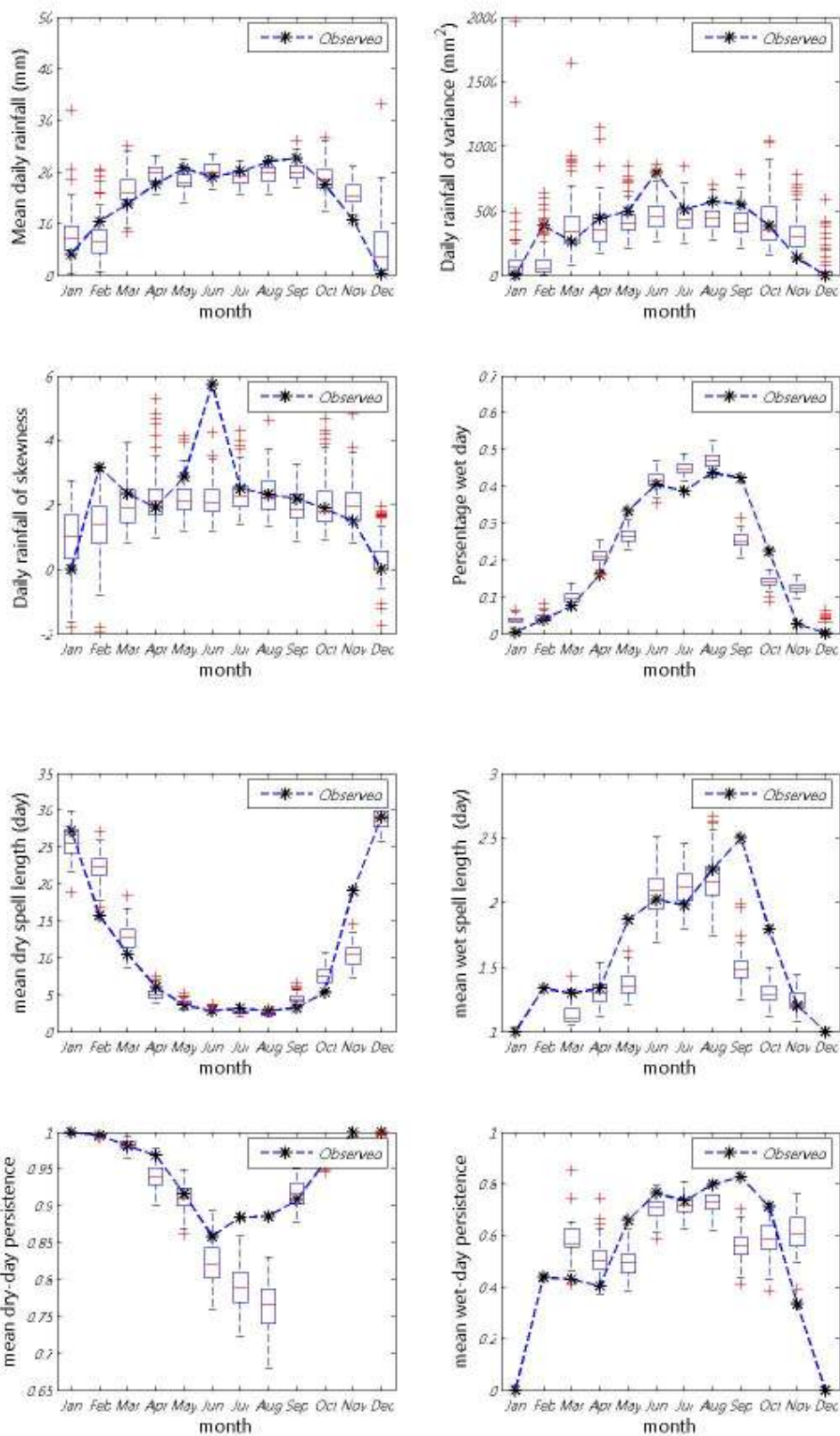
ภาพที่ ข.51 ค่าเฉลี่ย ความแปรปรวน สัมประสิทธิ์ความเบ้ เปอร์เซนต์ที่ฝนตก ช่วงเวลาที่ฝนหยุดและตก และจำนวนครั้งสัมผัสที่ฝนหยุดและตก ของข้อมูลฝนรายวันอดีตกับข้อมูลสังเคราะห์ สำหรับสถานี 406002 (ปี ค.ศ. 1976-1990)
