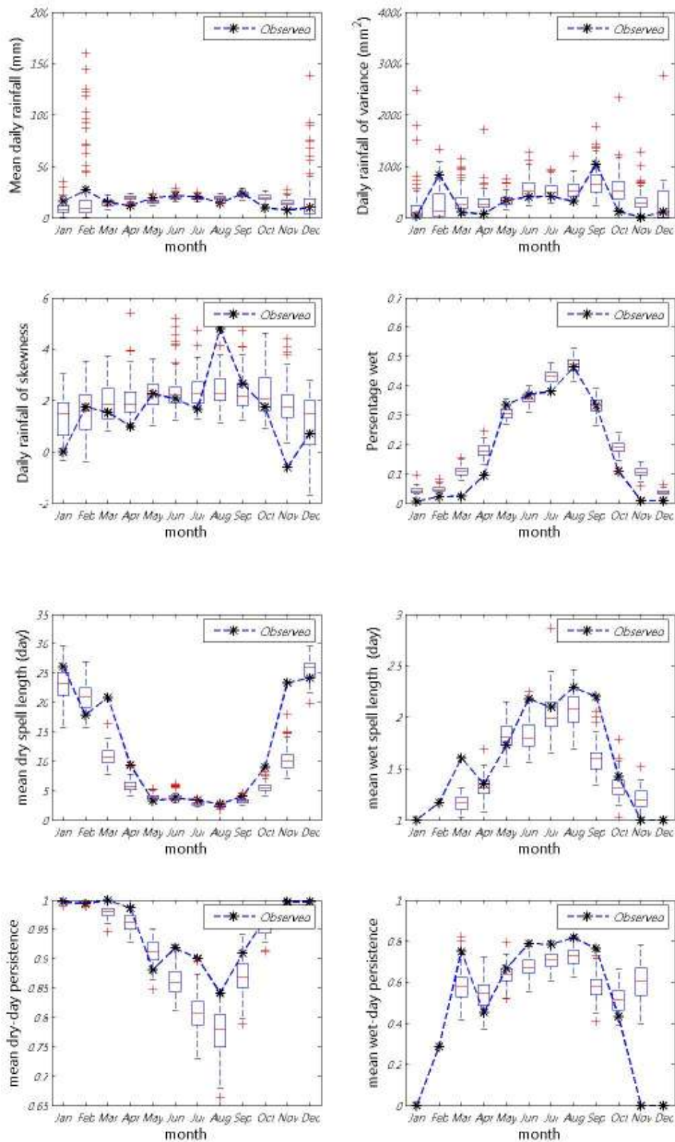
ภาพที่ ข.18 ค่าเฉลี่ย ความแปรปรวน สัมประสิทธิ์ความเบ้ เปอร์เซนต์ที่ฝนตก ช่วงเวลาที่ฝนหยุดและตก และจำนวนครั้งสัมผัสที่ฝนหยุดและตก ของข้อมูลฝนรายวันอดีตกับข้อมูลสังเคราะห์สำหรับสถานี 11210 (ปี ค.ศ.1991-2001)
