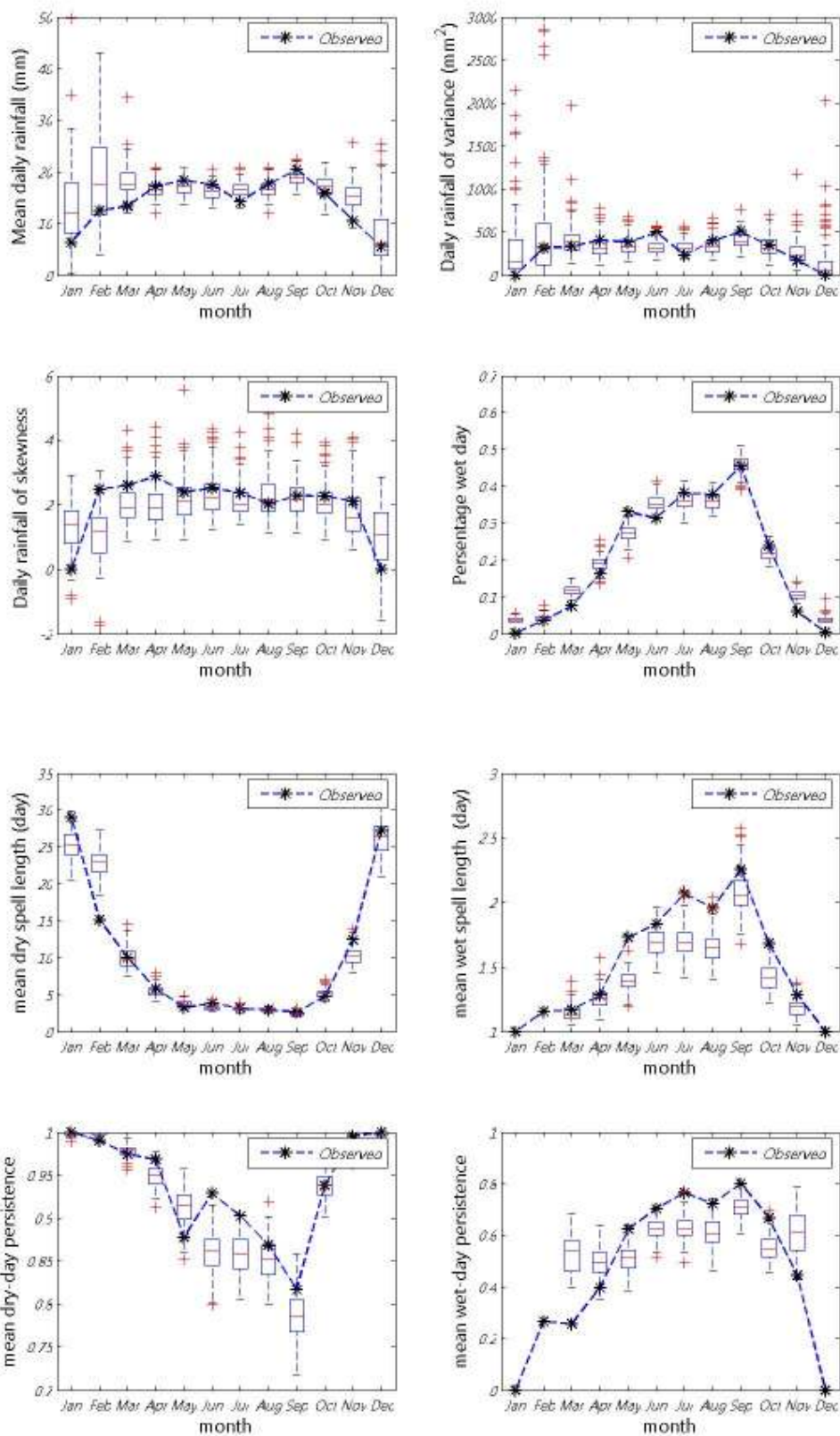
ภาพที่ ข.75 ค่าเฉลี่ย ความแปรปรวน สัมประสิทธิ์ความเบ้ เปอร์เซ็นต์ที่ฝนตก ช่วงเวลาที่ฝนหยุดและตก และจำนวนครั้งสัมผัสที่ฝนหยุดและตก ของข้อมูลฝนรายวันอดีตกับข้อมูลสังเคราะห์สำหรับสถานี 436004 (ปี ค.ศ. 1976-1990)
