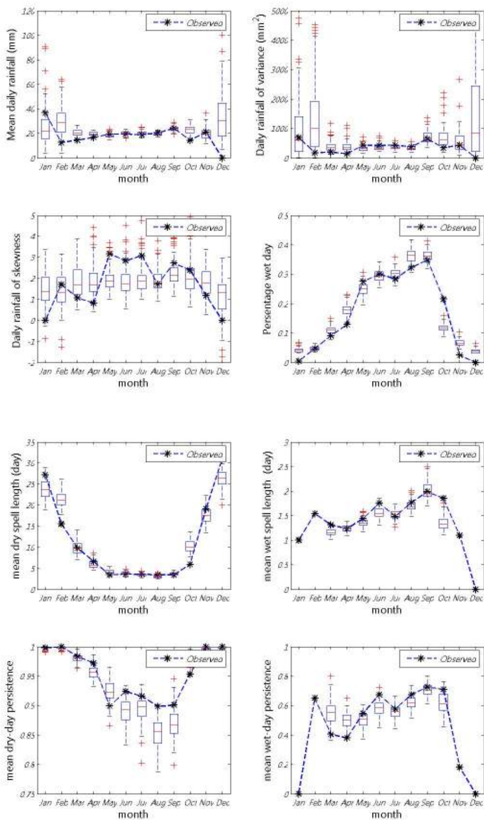
ภาพที่ ข.29 ค่าเฉลี่ย ความแปรปรวน สัมประสิทธิ์ความเบ้ เปอร์เซนต์ที่ฝนตก ช่วงเวลาที่ฝนหยุดและตก และจำนวนครั้งสัมผัสที่ฝนหยุดและตก ของข้อมูลฝนรายวันอดีตกับข้อมูลสังเคราะห์ สำหรับสถานี 21190 (ปี ค.ศ. 1976-1990)
