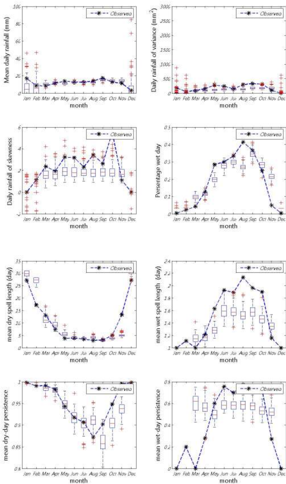
ภาพที่ ข.71 ค่าเฉลี่ย ความแปรปรวน สัมประสิทธิ์ความเบ้ เปอร์เซนต์ที่ฝนตก ช่วงเวลาที่ฝนหยุดและตก และจำนวนครั้งสัมผัสที่ฝนหยุดและตก ของข้อมูลฝนรายวันอดีตกับข้อมูลสังเคราะห์สำหรับสถานี 432005 (ปี ค.ศ. 1976-1990)
