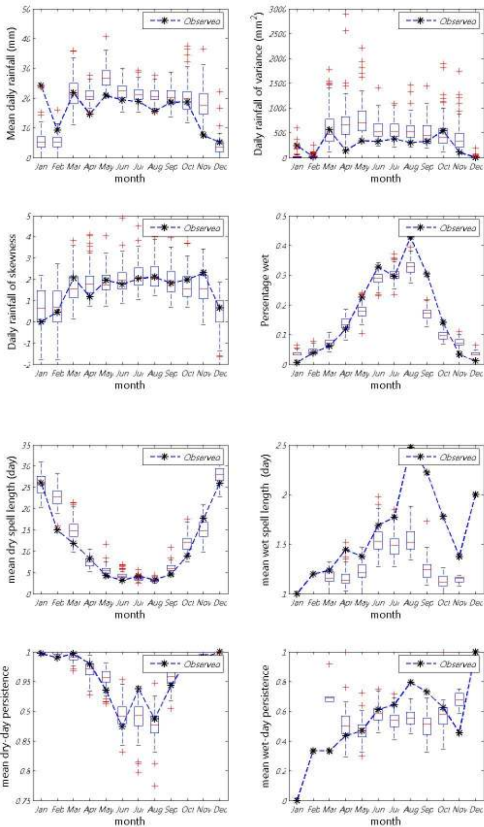
ภาพที่ ข.38 ค่าเฉลี่ย ความแปรปรวน สัมประสิทธิ์ความเบ้ เปอร์เซนต์ที่ฝนตก ช่วงเวลาที่ฝนหยุดและตก และจำนวนครั้งสัมผัสที่ฝนหยุดและตก ของข้อมูลฝนรายวันอดีตกับข้อมูลสังเคราะห์สำหรับสถานี 68150 (ปี ค.ศ.1991-2001)
