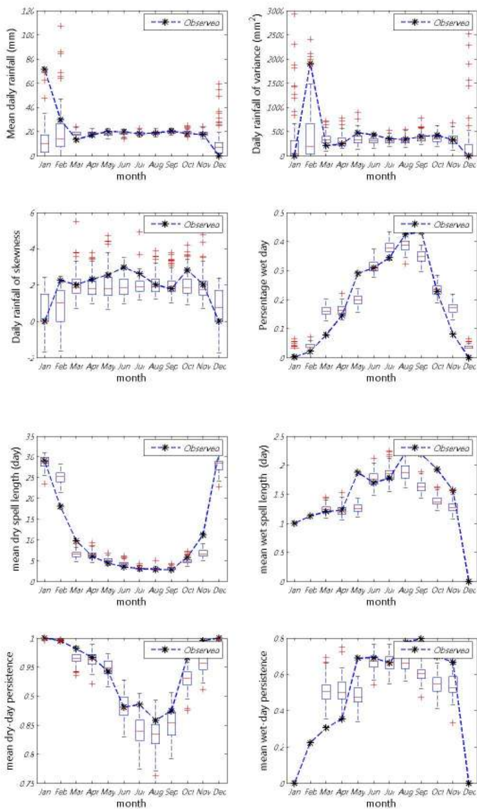
ภาพที่ ข.79 ค่าเฉลี่ย ความแปรปรวน สัมประสิทธิ์ความเบ้ เปอร์เซนต์ที่ฝนตก ช่วงเวลาที่ฝนหยุดและตก และจำนวนครั้งสัมผัสที่ฝนหยุดและตก ของข้อมูลฝนรายวันอดีตกับข้อมูลสังเคราะห์ สำหรับสถานี 436006 (ปี ค.ศ. 1976-1990)
