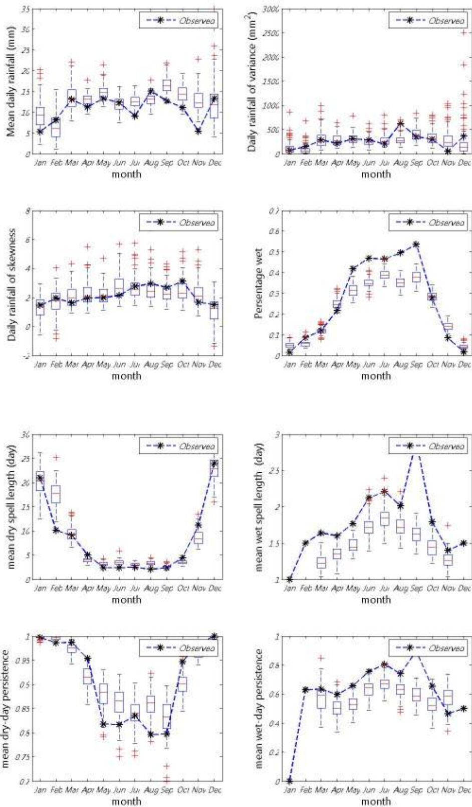
ภาพที่ ข.24 ค่าเฉลี่ย ความแปรปรวน สัมประสิทธิ์ความเบ้ เปอร์เซนต์ที่ฝนตก ช่วงเวลาที่ฝนหยุดและตก และจำนวนครั้งสัมผัสที่ฝนหยุดและตก ของข้อมูลฝนรายวันอดีตกับข้อมูลสังเคราะห์สำหรับสถานี 14112 (ปี ค.ศ.1991-2001)
