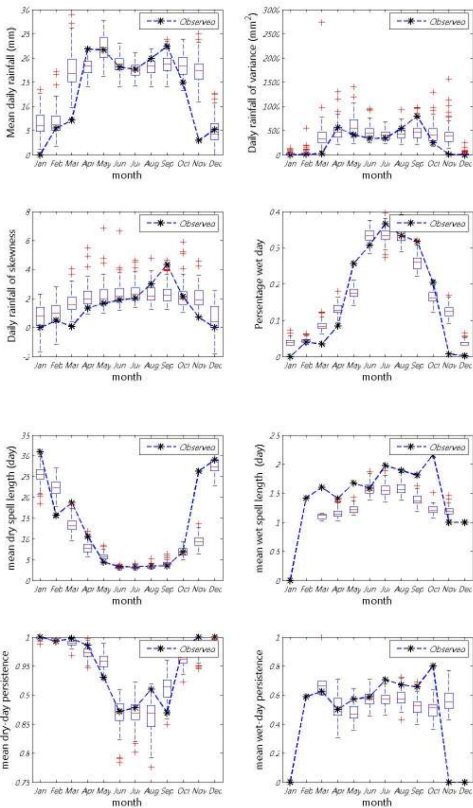
ภาพที่ ข.37 ค่าเฉลี่ย ความแปรปรวน สัมประสิทธิ์ความเบ้ เปอร์เซ็นต์ที่ฝนตก ช่วงเวลาที่ฝนหยุดและตก และจำนวนครั้งสัมผัสที่ฝนหยุดและตก ของข้อมูลฝนรายวันอดีตกับข้อมูลสังเคราะห์ สำหรับสถานี 68150 (ปี ค.ศ. 1976-1990)
