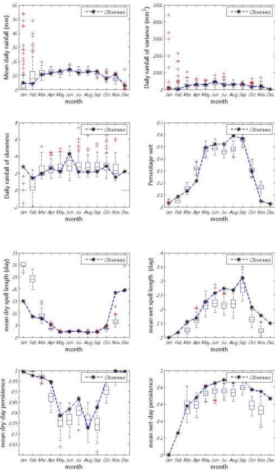
ภาพที่ ข.32 ค่าเฉลี่ย ความแปรปรวน สัมประสิทธิ์ความเบ้ เปอร์เซนต์ที่ฝนตก ช่วงเวลาที่ฝนหยุดและตก และจำนวนครั้งสัมผัสที่ฝนหยุดและตก ของข้อมูลฝนรายวันอดีตกับข้อมูลสังเคราะห์สำหรับสถานี 49013 (ปี ค.ศ.1991-2001)
