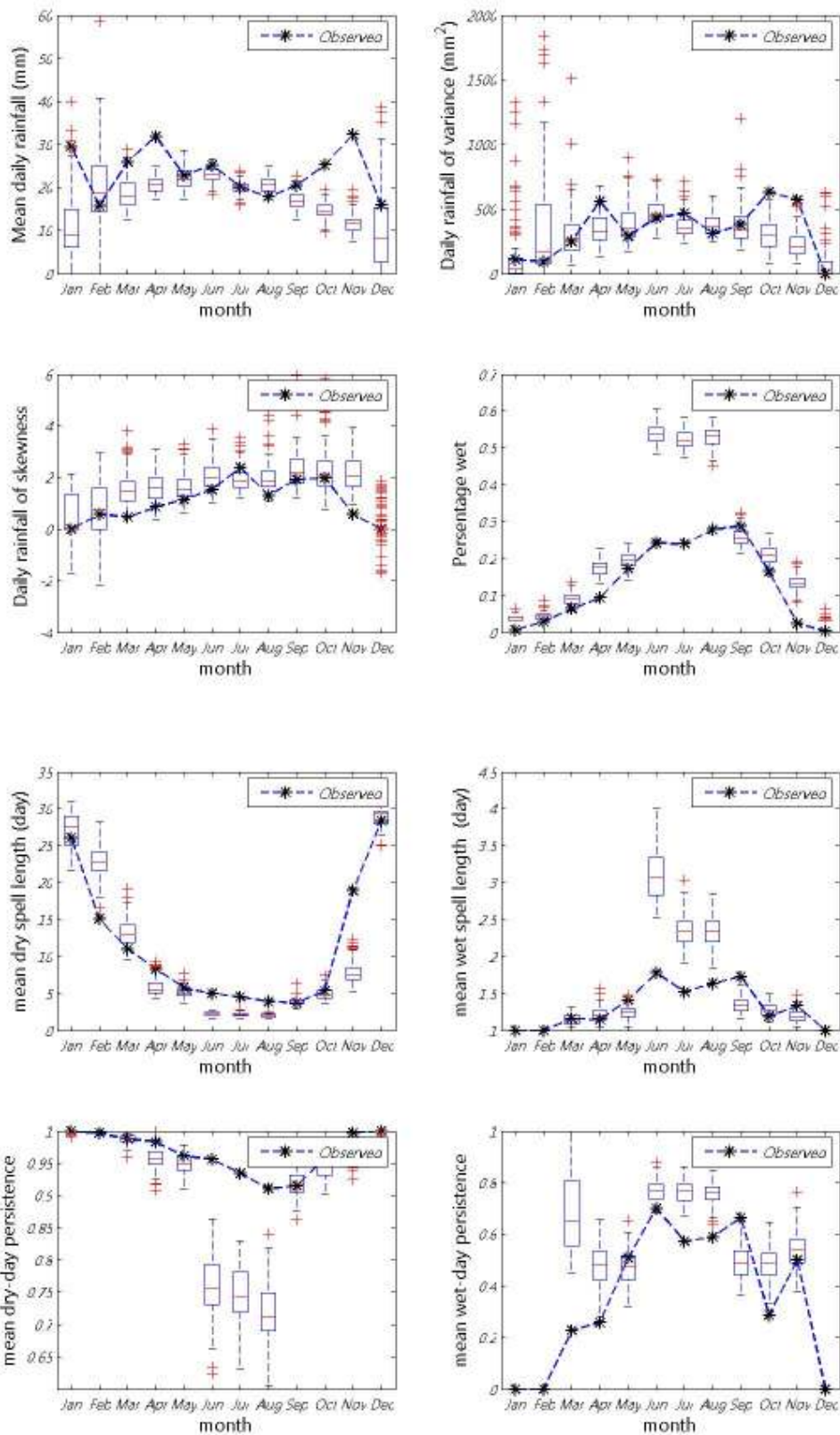
ภาพที่ ข.82 ค่าเฉลี่ย ความแปรปรวน สัมประสิทธิ์ความเบ้ เปอร์เซ็นต์ที่ฝนตก ช่วงเวลาที่ฝนหยุดและตก และจำนวนครั้งสัมผัสที่ฝนหยุดและตก ของข้อมูลฝนรายวันอดีตกับข้อมูลสังเคราะห์สำหรับสถานี 436007 (ปี ค.ศ.1991-2001)
