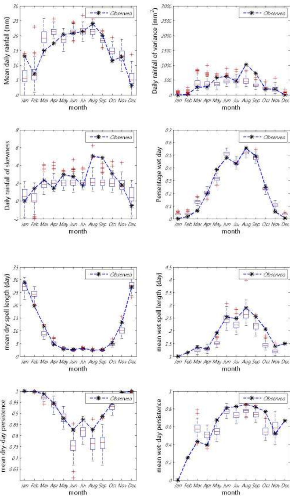
ภาพที่ ข.59 ค่าเฉลี่ย ความแปรปรวน สัมประสิทธิ์ความเบ้ เปอร์เซ็นต์ที่ฝนตก ช่วงเวลาที่ฝนหยุดและตก และจำนวนครั้งสัมผัสที่ฝนหยุดและตก ของข้อมูลฝนรายวันอดีตกับข้อมูลสังเคราะห์สำหรับสถานี 407006 (ปี ค.ศ. 1976-1990)
