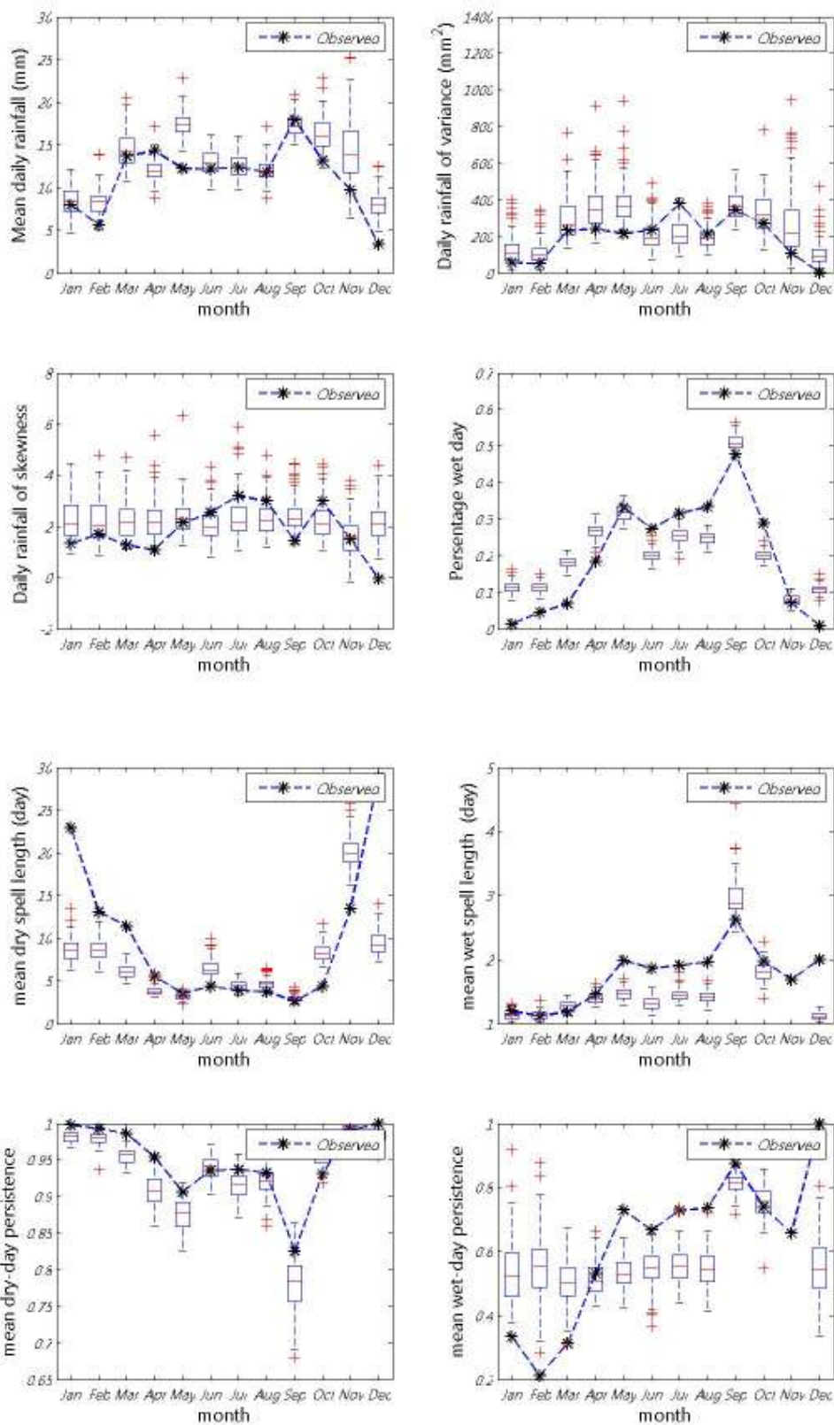
ภาพที่ ข.3 ค่าเฉลี่ย ความแปรปรวน สัมประสิทธิ์ความเบ้ เปอร์เซนต์ที่ฝนตก ช่วงเวลาที่ฝนหยุดและตก และจำนวนครั้งสัมพัทธ์ที่ฝนหยุดและตก ของข้อมูลฝนรายวันอดีตกับข้อมูลสังเคราะห์สำหรับสถานี 05023 (ปี ค.ศ. 1976-1990)
