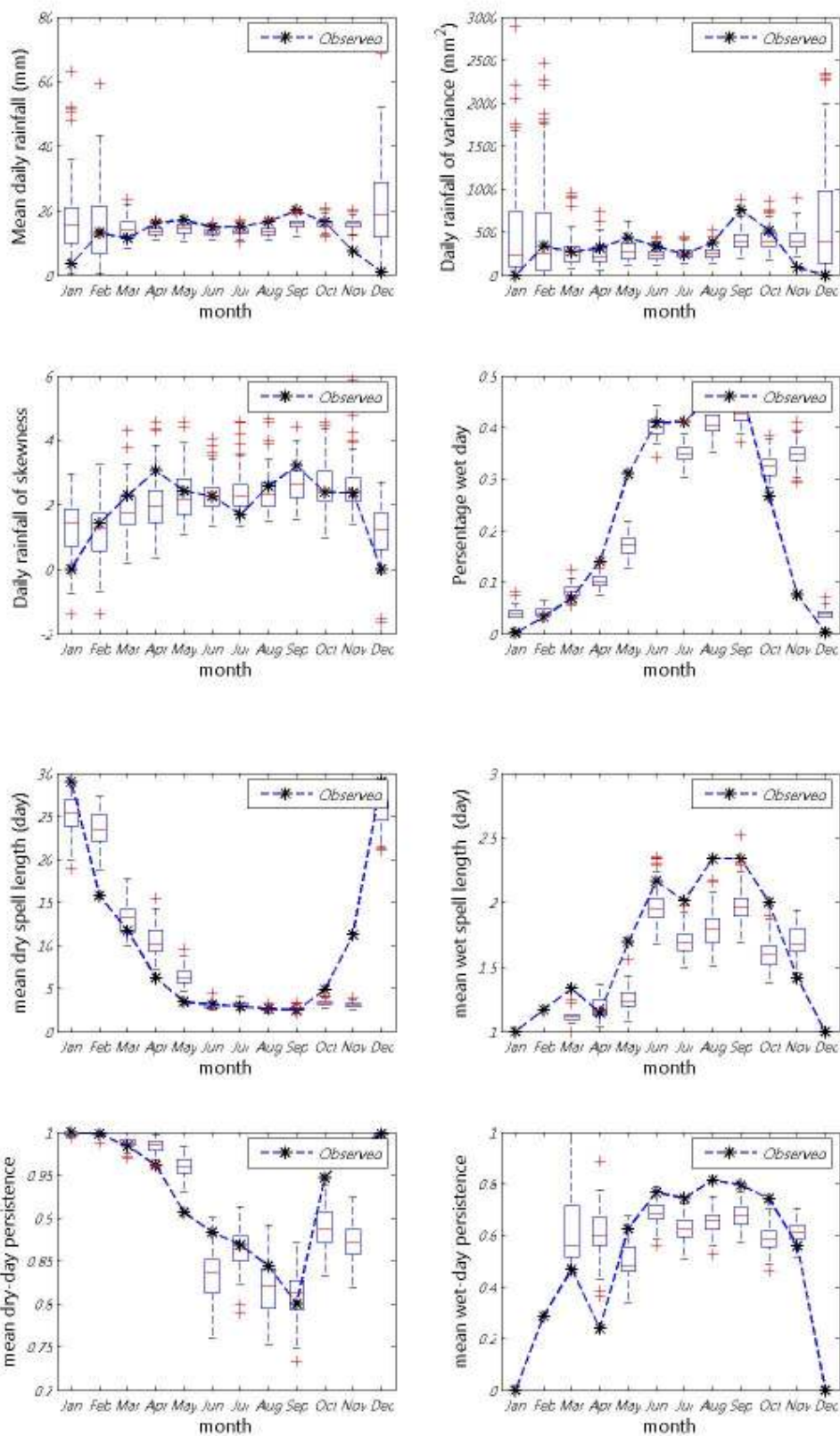
ภาพที่ ข.67 ค่าเฉลี่ย ความแปรปรวน สัมประสิทธิ์ความเบ้ เปอร์เซ็นต์ที่ฝนตก ช่วงเวลาที่ฝนหยุดและตก และจำนวนครั้งสัมผัสที่ฝนหยุดและตก ของข้อมูลฝนรายวันอดีตกับข้อมูลสังเคราะห์สำหรับสถานี 432001 (ปี ค.ศ. 1976-1990)
