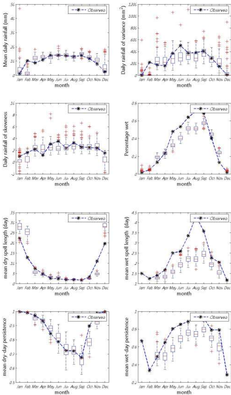
ภาพที่ ข.58 ค่าเฉลี่ย ความแปรปรวน สัมประสิทธิ์ความเบ้ เปอร์เซ็นต์ที่ฝนตก ช่วงเวลาที่ฝนหยุดและตก และจำนวนครั้งสัมผัสที่ฝนหยุดและตก ของข้อมูลฝนรายวันอดีตกับข้อมูลสังเคราะห์สำหรับสถานี 407002 (ปี ค.ศ.1991-2001)
