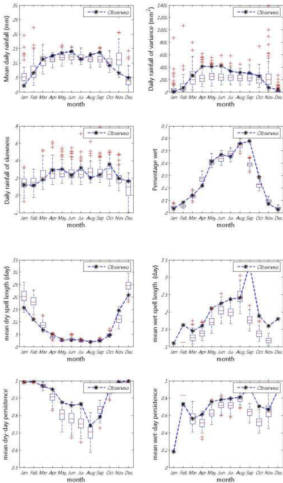
ภาพที่ ข.28 ค่าเฉลี่ย ความแปรปรวน สัมประสิทธิ์ความเบ้ เปอร์เซนต์ที่ฝนตก ช่วงเวลาที่ฝนหยุดและตก และจำนวนครั้งสัมผัสที่ฝนหยุดและตก ของข้อมูลฝนรายวันอดีตกับข้อมูลสังเคราะห์สำหรับสถานี 21043 (ปี ค.ศ.1991-2001)
