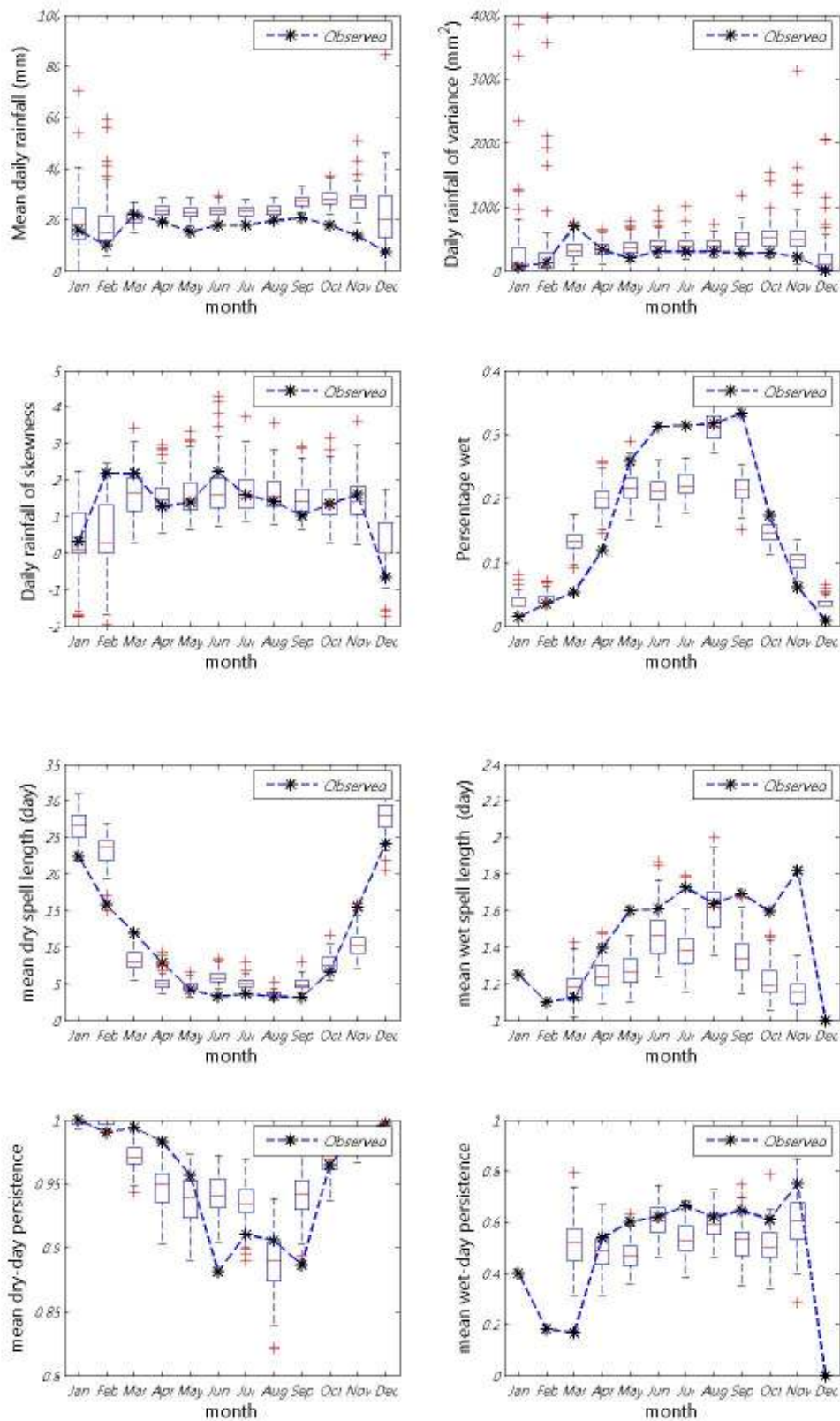
ภาพที่ ข.78 ค่าเฉลี่ย ความแปรปรวน สัมประสิทธิ์ความเบ้ เปอร์เซ็นต์ที่ฝนตก ช่วงเวลาที่ฝนหยุดและตก และจำนวนครั้งสัมผัสที่ฝนหยุดและตก ของข้อมูลฝนรายวันอดีตกับข้อมูลสังเคราะห์สำหรับสถานี 436005 (ปี ค.ศ.1991-2001)
