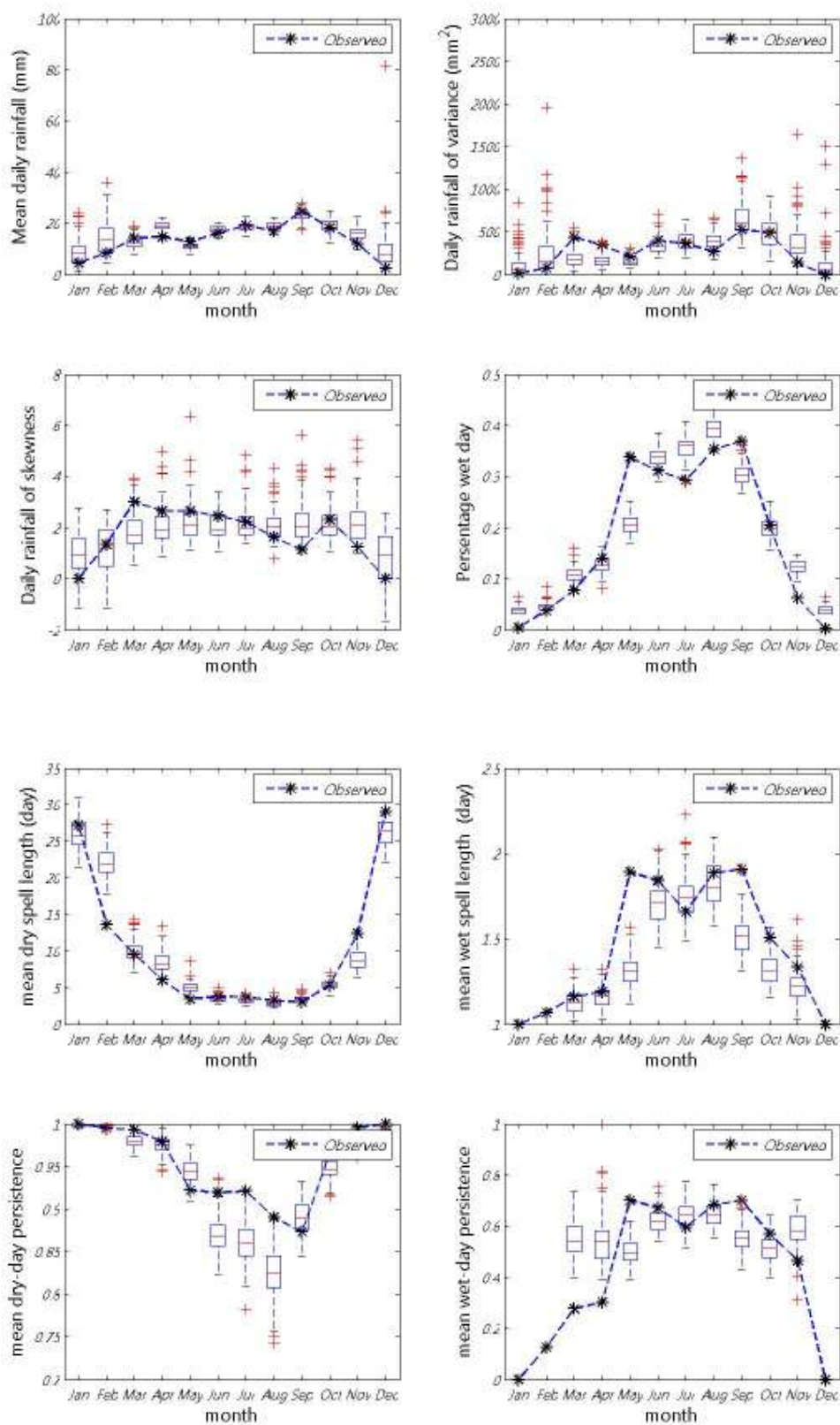
ภาพที่ ข.83 ค่าเฉลี่ย ความแปรปรวน สัมประสิทธิ์ความเบ้ เปอร์เซนต์ที่ฝนตก ช่วงเวลาที่ฝนหยุดและตก และจำนวนครั้งสัมผัสที่ฝนหยุดและตก ของข้อมูลฝนรายวันอดีตกับข้อมูลสังเคราะห์สำหรับสถานี 436013 (ปี ค.ศ. 1976-1990)
