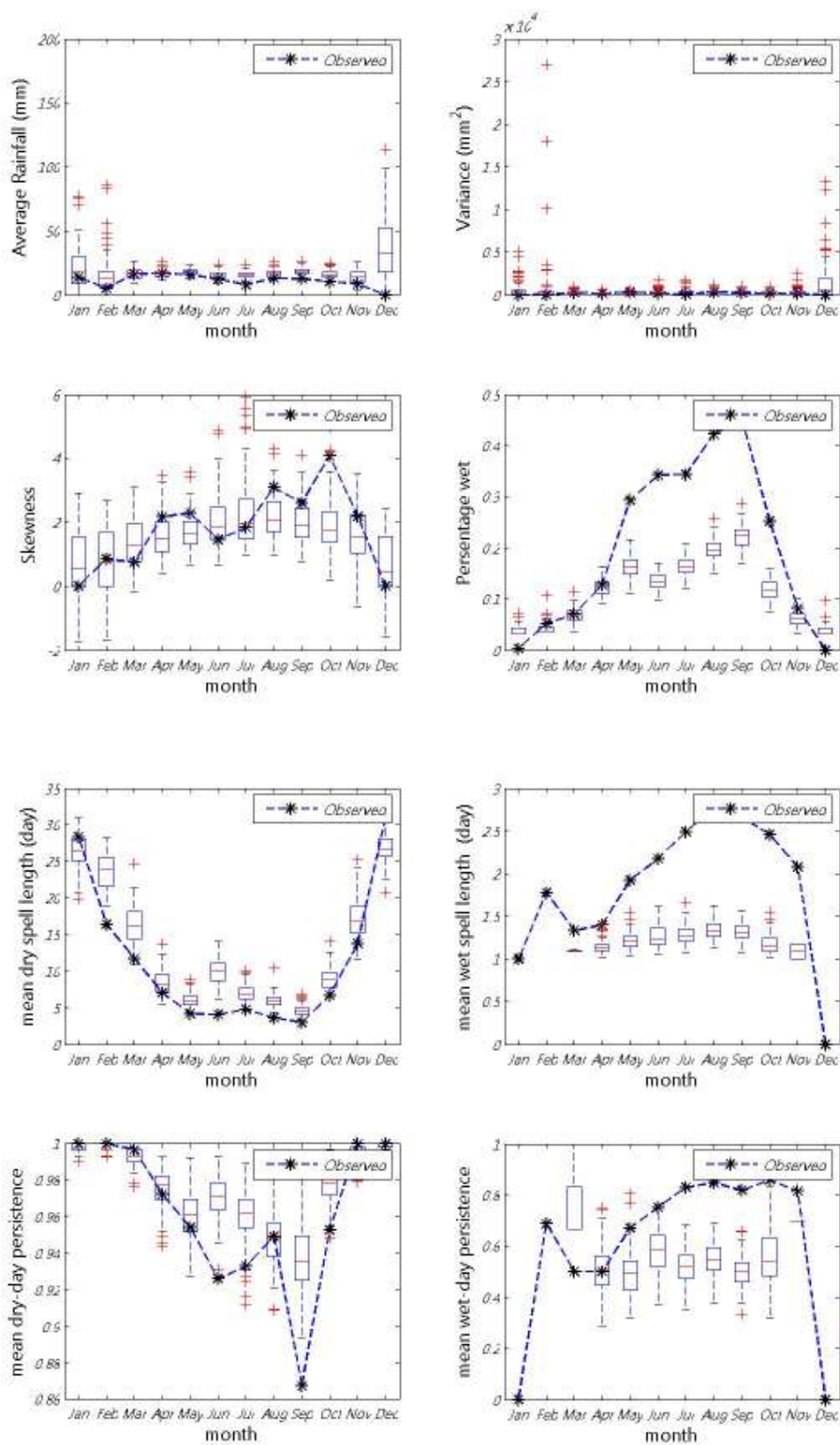
ภาพที่ ข.8 ค่าเฉลี่ย ความแปรปรวน สัมประสิทธิ์ความเบ้ เปอร์เซนต์ที่ฝนตก ช่วงเวลาที่ฝนหยุดและตก และจำนวนครั้งสัมผัสที่ฝนหยุดและตก ของข้อมูลฝนรายวันอดีตกับข้อมูลสังเคราะห์ สำหรับสถานี 05092 (ปี ค.ศ.1991-2001)
