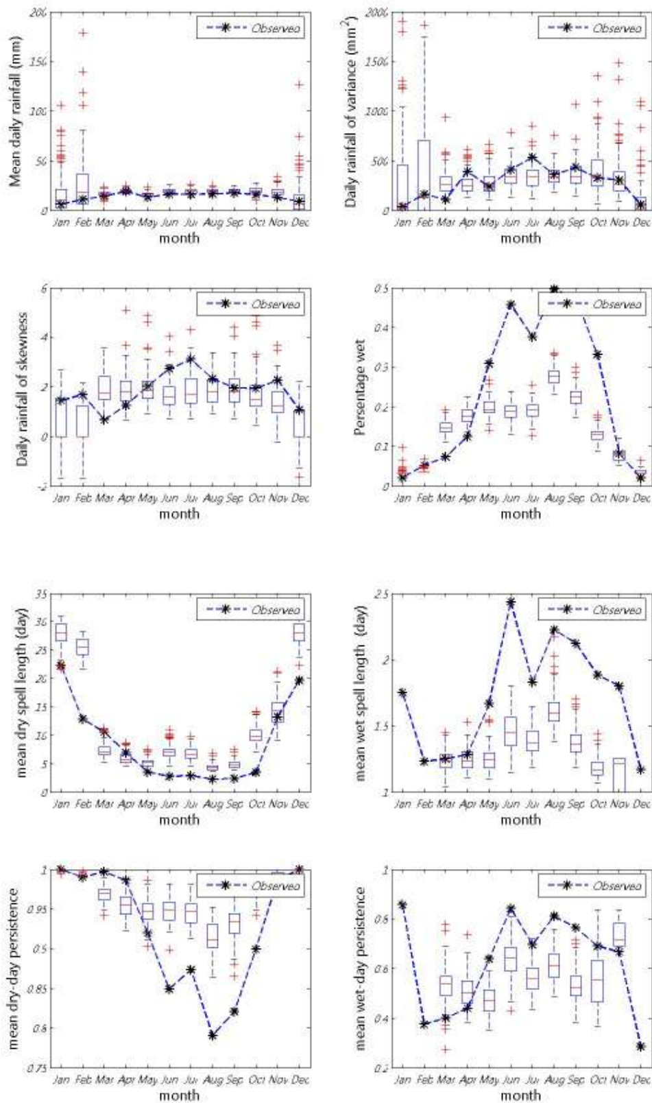
ภาพที่ ข.80 ค่าเฉลี่ย ความแปรปรวน สัมประสิทธิ์ความเบ้ เปอร์เซนต์ที่ฝนตก ช่วงเวลาที่ฝนหยุดและตก และจำนวนครั้งสัมผัสที่ฝนหยุดและตก ของข้อมูลฝนรายวันอดีตกับข้อมูลสังเคราะห์สำหรับสถานี 436006 (ปี ค.ศ.1991-2001)
