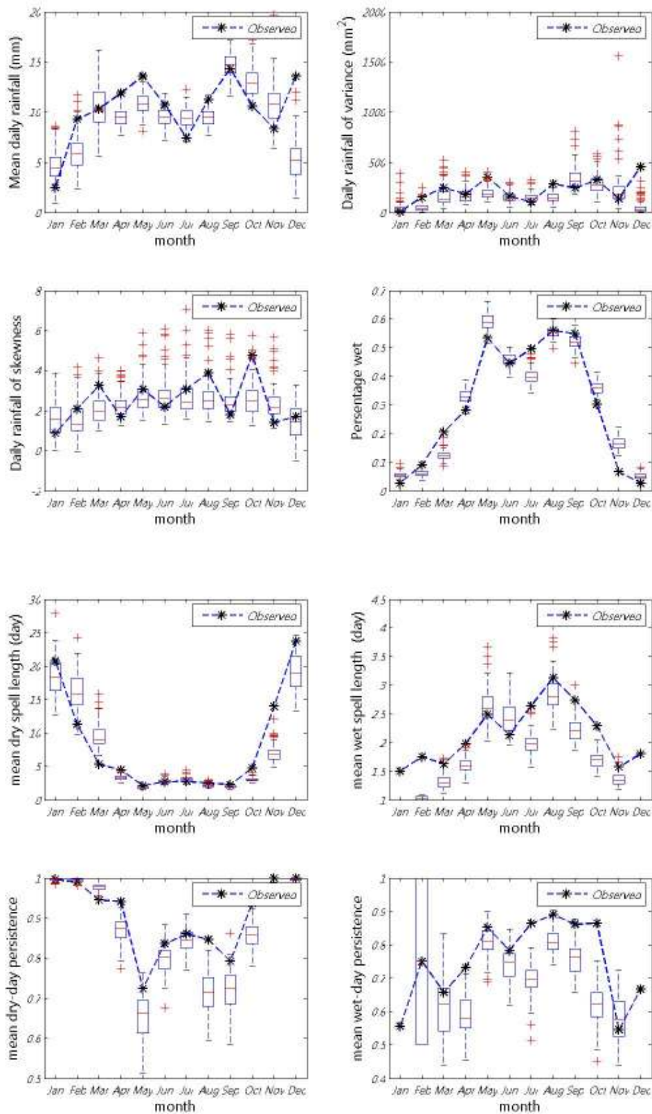
ภาพที่ ข.26 ค่าเฉลี่ย ความแปรปรวน สัมประสิทธิ์ความเบ้ เปอร์เซนต์ที่ฝนตก ช่วงเวลาที่ฝนหยุดและตก และจำนวนครั้งสัมผัสที่ฝนหยุดและตก ของข้อมูลฝนรายวันอดีตกับข้อมูลสังเคราะห์สำหรับสถานี 18073 (ปี ค.ศ.1991-2001)
