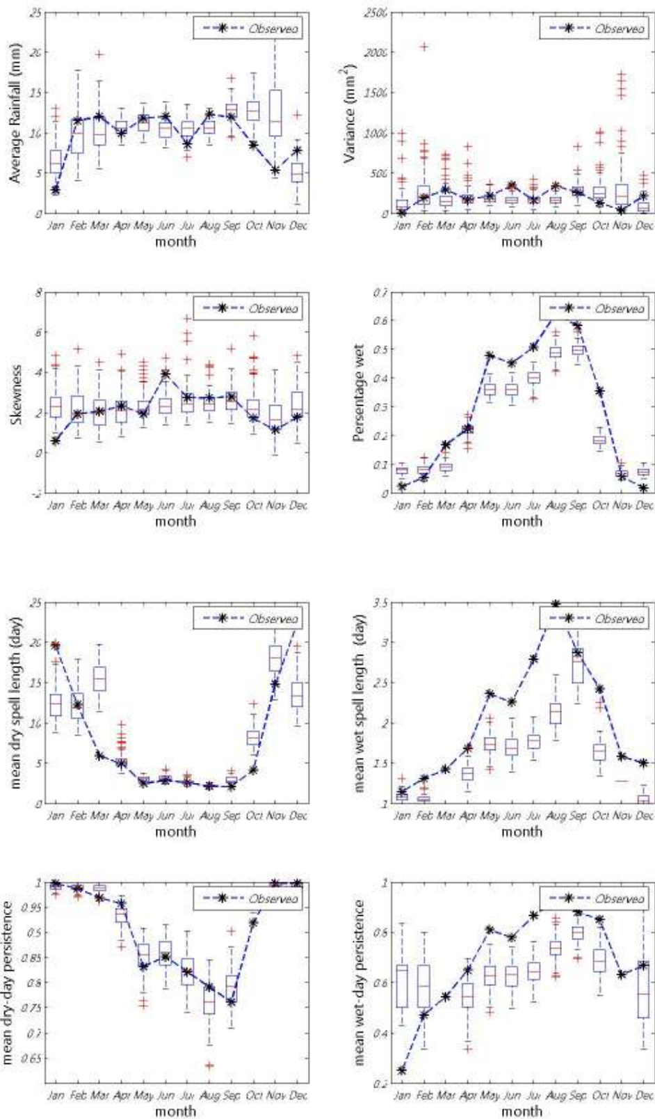
ภาพที่ ข.10 ค่าเฉลี่ย ความแปรปรวน สัมประสิทธิ์ความเบ้ เปอร์เซ็นต์ที่ฝนตก ช่วงเวลาที่ฝนหยุดและตก และจำนวนครั้งสัมผัสที่ฝนหยุดและตก ของข้อมูลฝนรายวันอดีตกับข้อมูลสังเคราะห์สำหรับสถานี 05171 (ปี ค.ศ.1991-2001)
