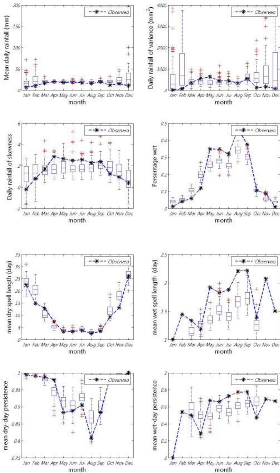
ภาพที่ ข.30 ค่าเฉลี่ย ความแปรปรวน สัมประสิทธิ์ความเบ้ เปอร์เซนต์ที่ฝนตก ช่วงเวลาที่ฝนหยุดและตก และจำนวนครั้งสัมพัทธ์ที่ฝนหยุดและตก ของข้อมูลฝนรายวันอดีตกับข้อมูลสังเคราะห์สำหรับสถานี 21190 (ปี ค.ศ.1991-2001)
