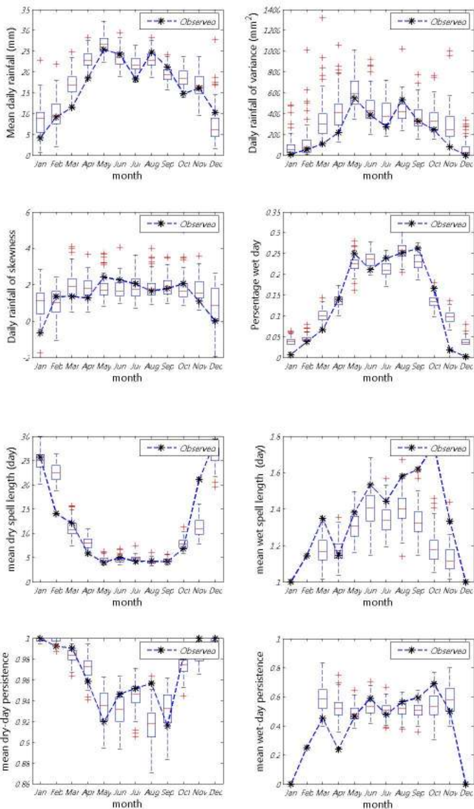
ภาพที่ ข.15 ค่าเฉลี่ย ความแปรปรวน สัมประสิทธิ์ความเบ้ เปอร์เซนต์ที่ฝนตก ช่วงเวลาที่ฝนหยุดและตก และจำนวนครั้งสัมผัสที่ฝนหยุดและตก ของข้อมูลฝนรายวันอดีตกับข้อมูลสังเคราะห์สำหรับสถานี 11202 (ปี ค.ศ. 1976-1990)
