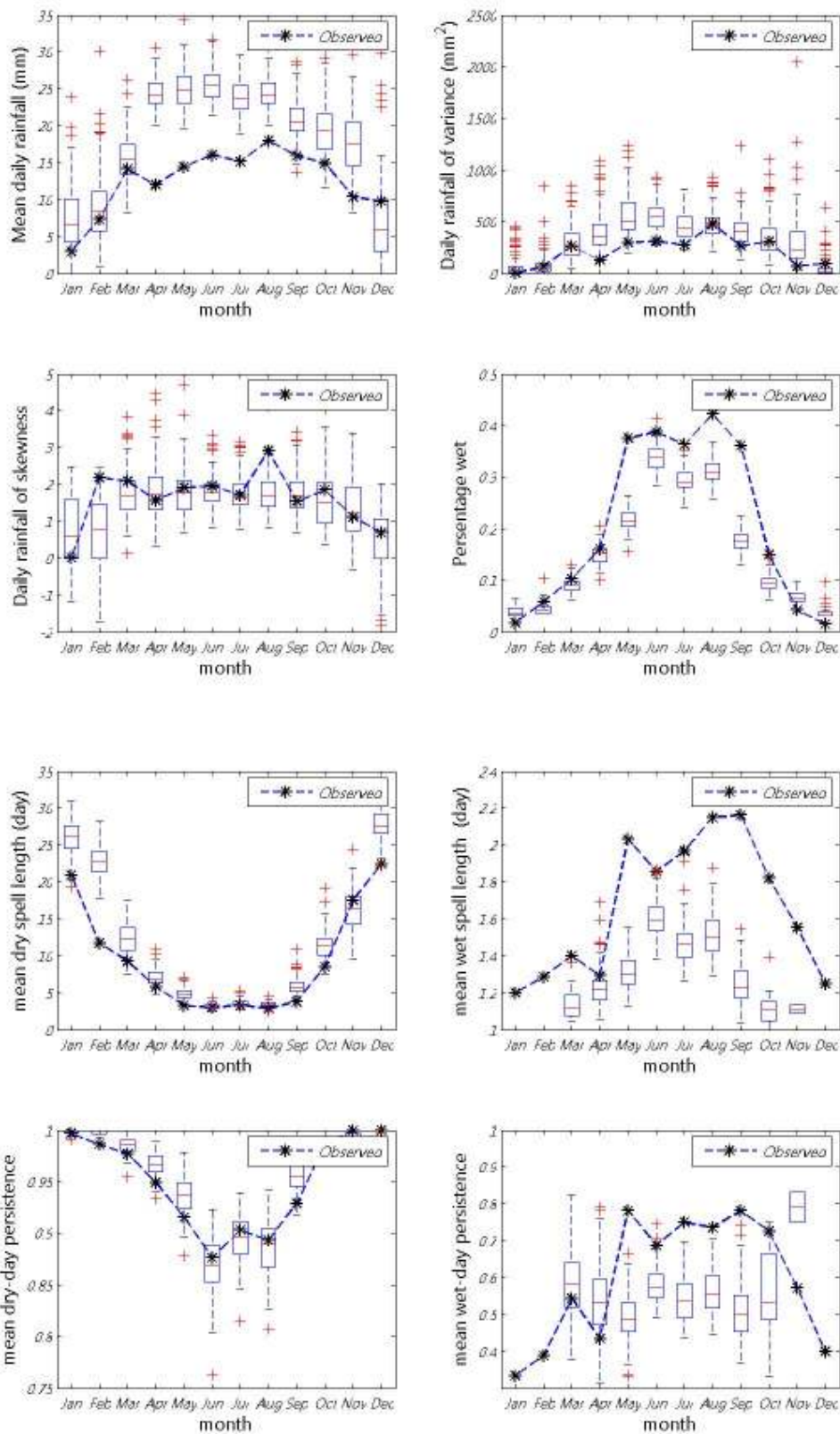
ภาพที่ ข.16 ค่าเฉลี่ย ความแปรปรวน สัมประสิทธิ์ความเบ้ เปอร์เซนต์ที่ฝนตก ช่วงเวลาที่ฝนหยุดและตก และจำนวนครั้งสัมพัทธ์ที่ฝนหยุดและตก ของข้อมูลฝนรายวันอดีตกับข้อมูลสังเคราะห์สำหรับสถานี 11202 (ปี ค.ศ.1991-2001)
