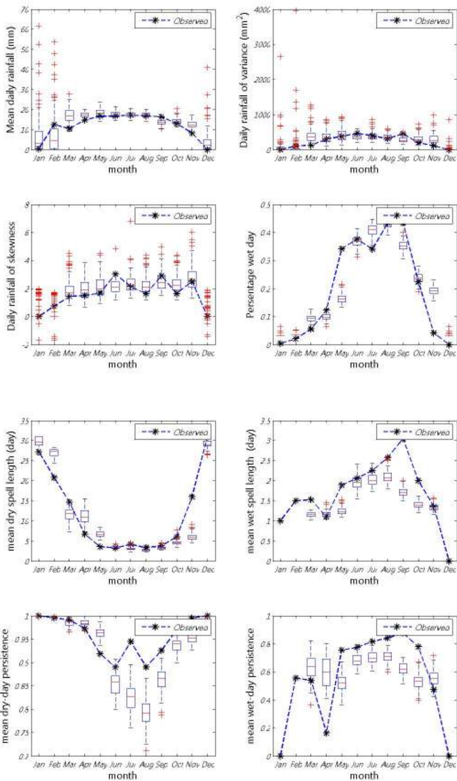
ภาพที่ ข.49 ค่าเฉลี่ย ความแปรปรวน สัมประสิทธิ์ความเบ้ เปอร์เซนต์ที่ฝนตก ช่วงเวลาที่ฝนหยุดและตก และจำนวนครั้งสัมพัทธ์ที่ฝนหยุดและตก ของข้อมูลฝนรายวันอดีตกับข้อมูลสังเคราะห์ สำหรับสถานี 405008 (ปี ค.ศ. 1976-1990)
