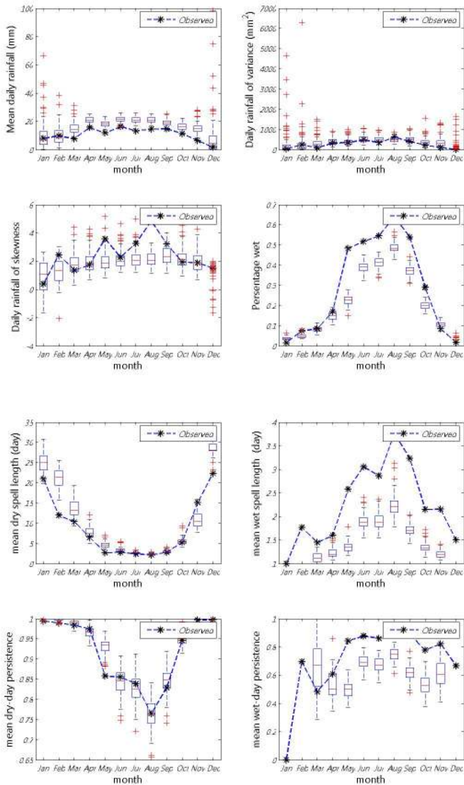
ภาพที่ ข.40 ค่าเฉลี่ย ความแปรปรวน สัมประสิทธิ์ความเบ้ เปอร์เซนต์ที่ฝนตก ช่วงเวลาที่ฝนหยุดและตก และจำนวนครั้งสัมผัสที่ฝนหยุดและตก ของข้อมูลฝนรายวันอดีตกับข้อมูลสังเคราะห์สำหรับสถานี 72022 (ปี ค.ศ.1991-2001)
