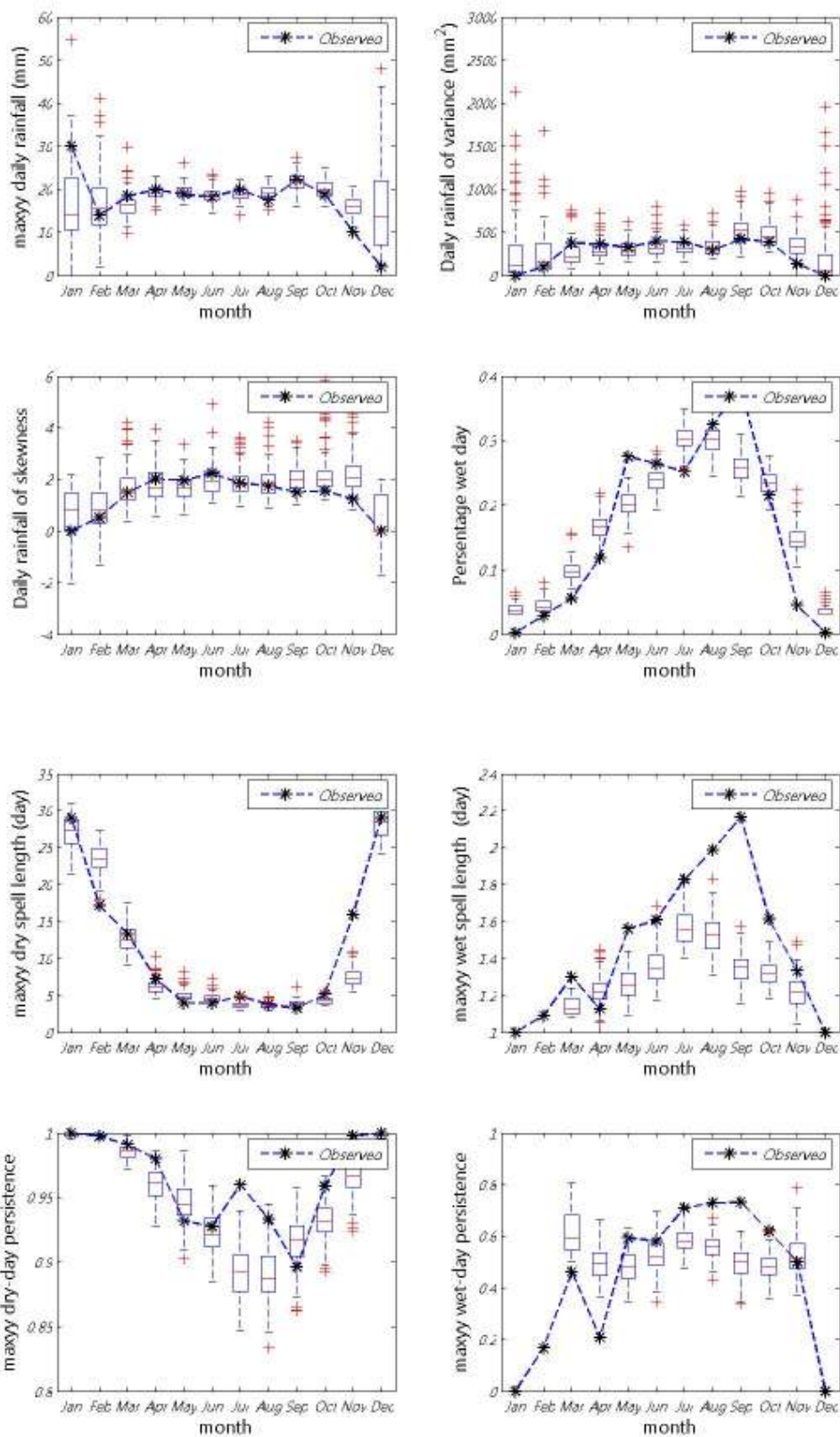
ภาพที่ ข.81 ค่าเฉลี่ย ความแปรปรวน สัมประสิทธิ์ความเบ้ เปอร์เซนต์ที่ฝนตก ช่วงเวลาที่ฝนหยุดและตก และจำนวนครั้งสัมผัสที่ฝนหยุดและตก ของข้อมูลฝนรายวันอดีตกับข้อมูลสังเคราะห์ สำหรับสถานี 436007 (ปี ค.ศ. 1976-1990)
