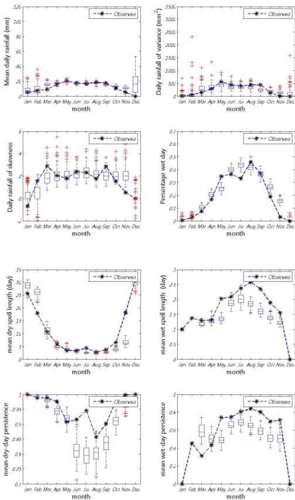
ภาพที่ ข.45 ค่าเฉลี่ย ความแปรปรวน สัมประสิทธิ์ความเบ้ เปอร์เซ็นต์ที่ฝนตก ช่วงเวลาที่ฝนหยุดและตก และจำนวนครั้งสัมผัสที่ฝนหยุดและตก ของข้อมูลฝนรายวันอดีตกับข้อมูลสังเคราะห์ สำหรับสถานี 404003 (ปี ค.ศ. 1976-1990)
