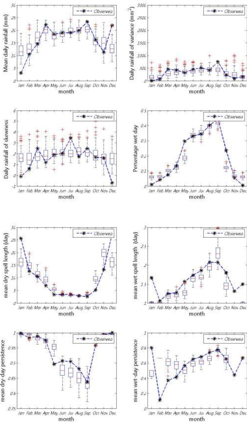
ภาพที่ ข. 69 ค่าเฉลี่ย ความแปรปรวน สัมประสิทธิ์ความเบ้ เปอร์เซนต์ที่ฝนตก ช่วงเวลาที่ฝนหยุดและตก และจำนวนครั้งสัมผัสที่ฝนหยุดและตก ของข้อมูลฝนรายวันอดีตกับข้อมูลสังเคราะห์สำหรับสถานี 432004 (ปี ค.ศ. 1976-1990)
