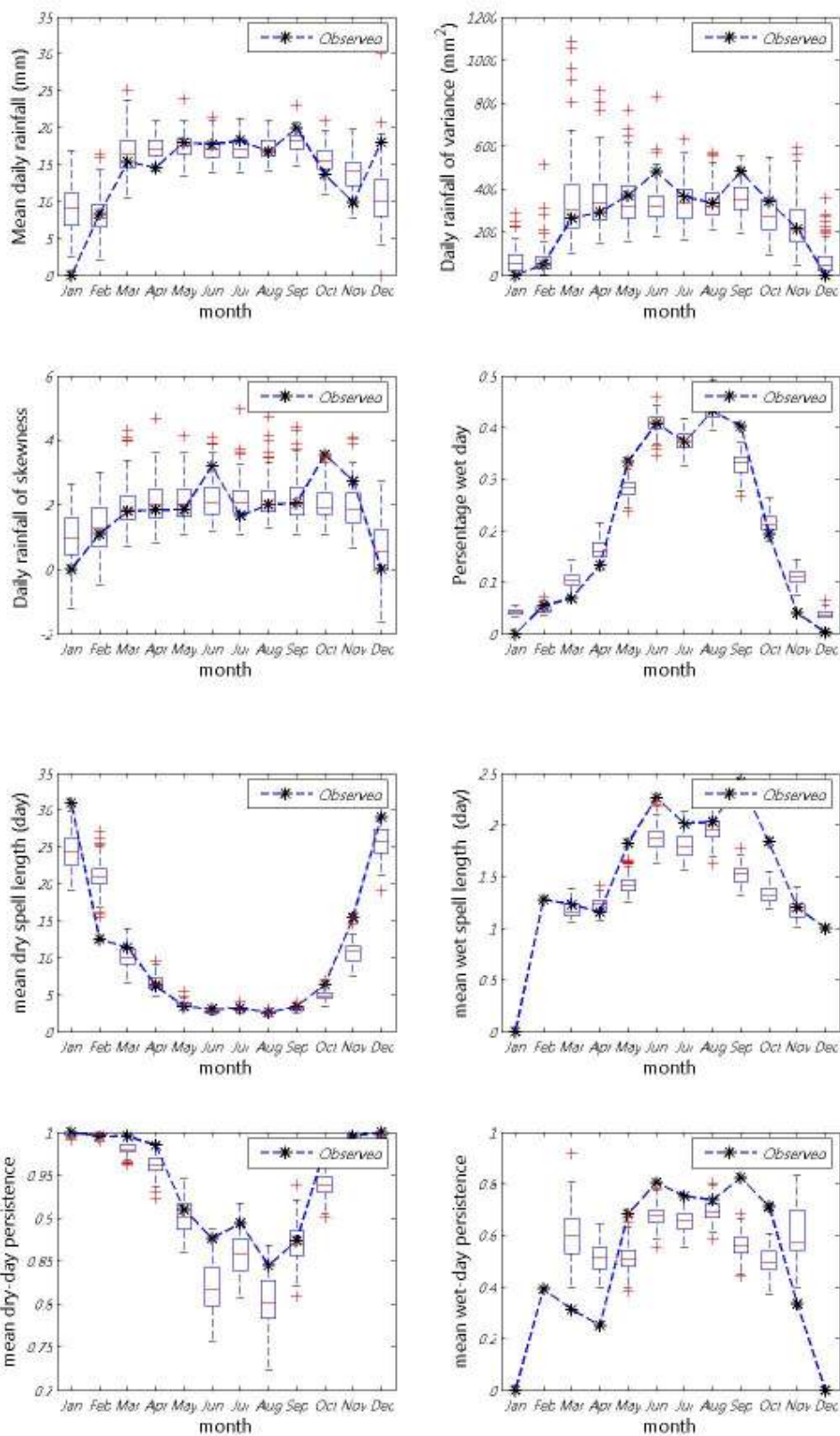
ภาพที่ ข.13 ค่าเฉลี่ย ความแปรปรวน สัมประสิทธิ์ความเบ้ เปอร์เซนต์ที่ฝนตก ช่วงเวลาที่ฝนหยุดและตก และจำนวนครั้งสัมผัสที่ฝนหยุดและตก ของข้อมูลฝนรายวันอดีตกับข้อมูลสังเคราะห์สำหรับสถานี 11170 (ปี ค.ศ. 1976-1990)
