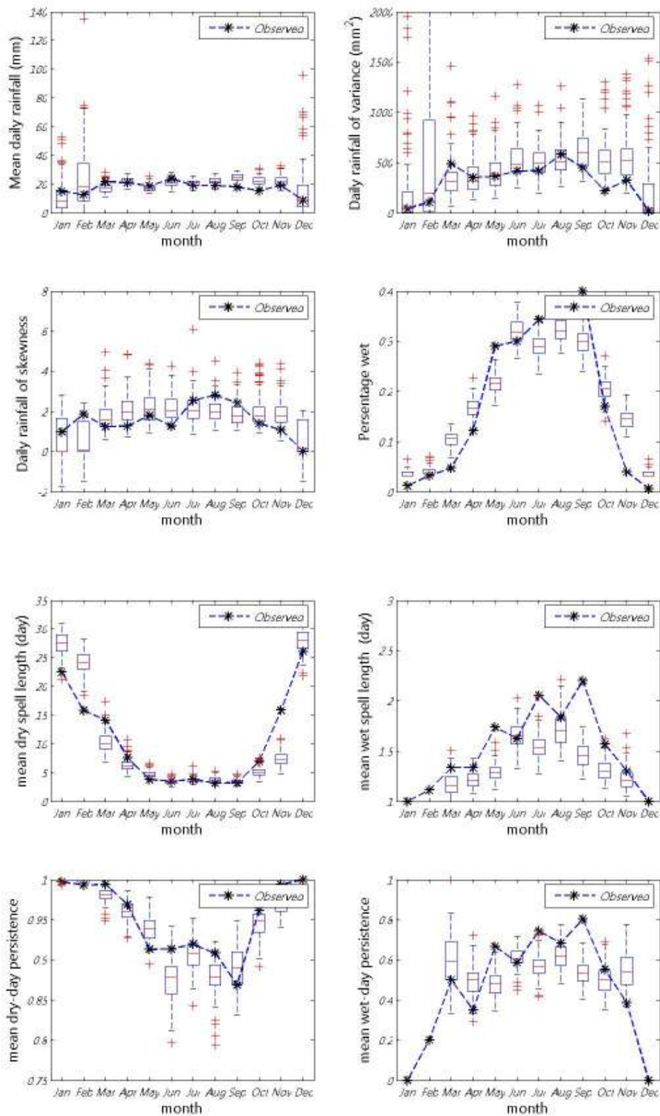
ภาพที่ ข.48 ค่าเฉลี่ย ความแปรปรวน สัมประสิทธิ์ความเบ้ เปอร์เซนต์ที่ฝนตก ช่วงเวลาที่ฝนหยุดและตก และจำนวนครั้งสัมผัสที่ฝนหยุดและตก ของข้อมูลฝนรายวันอดีตกับข้อมูลสังเคราะห์สำหรับสถานี 405002 (ปี ค.ศ.1991-2001)
