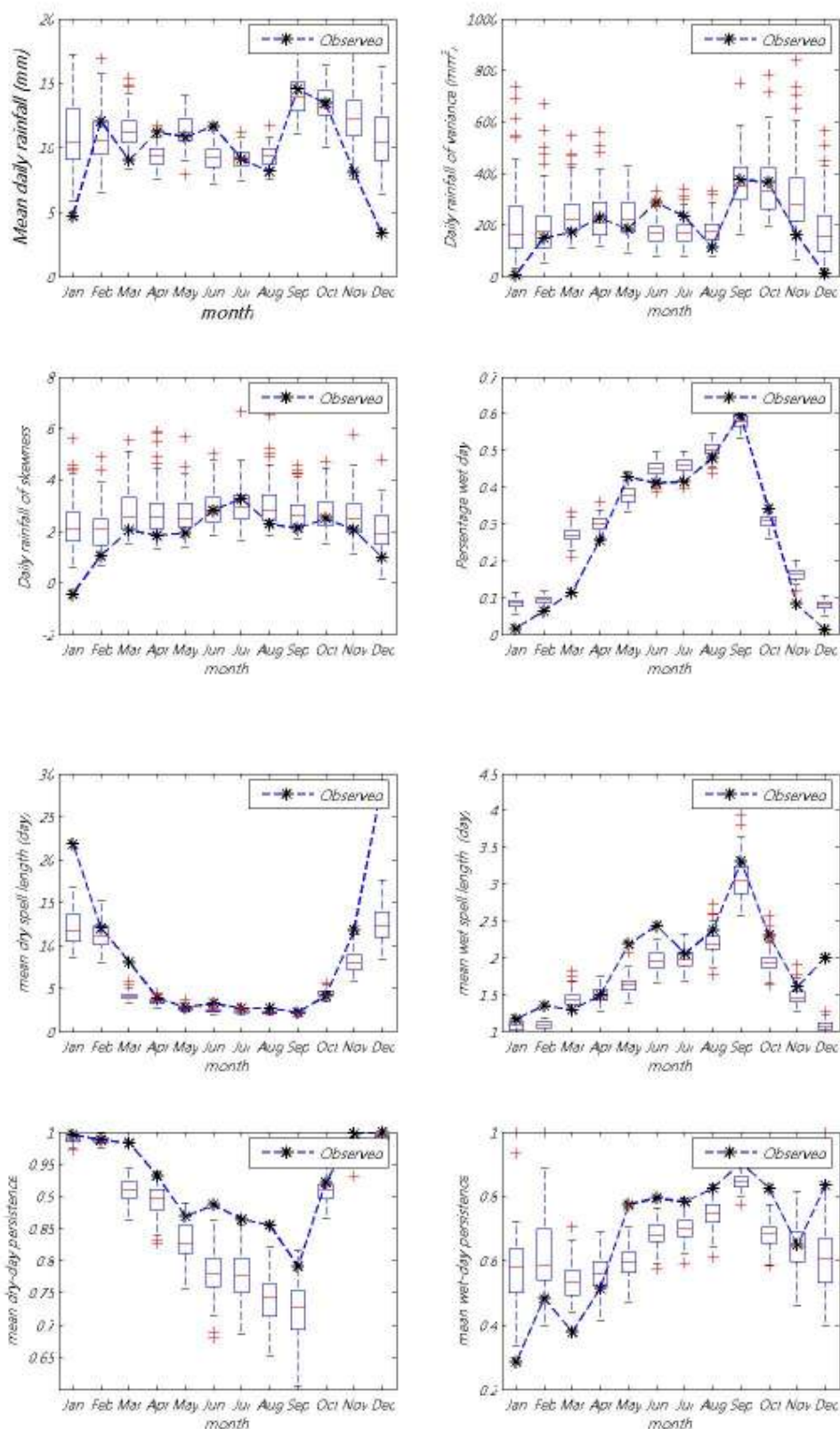
ภาพที่ ข.1 ค่าเฉลี่ย ความแปรปรวน สัมประสิทธิ์ความเบ้ เปอร์เซ็นต์ที่ฝนตก ช่วงเวลาที่ฝนหยุดและตก และจำนวนครั้งสัมผัสที่ฝนหยุดและตก ของข้อมูลฝนรายวันอดีตกับข้อมูลสังเคราะห์สำหรับสถานี 05013 (ปี ค.ศ. 1976-1990)
