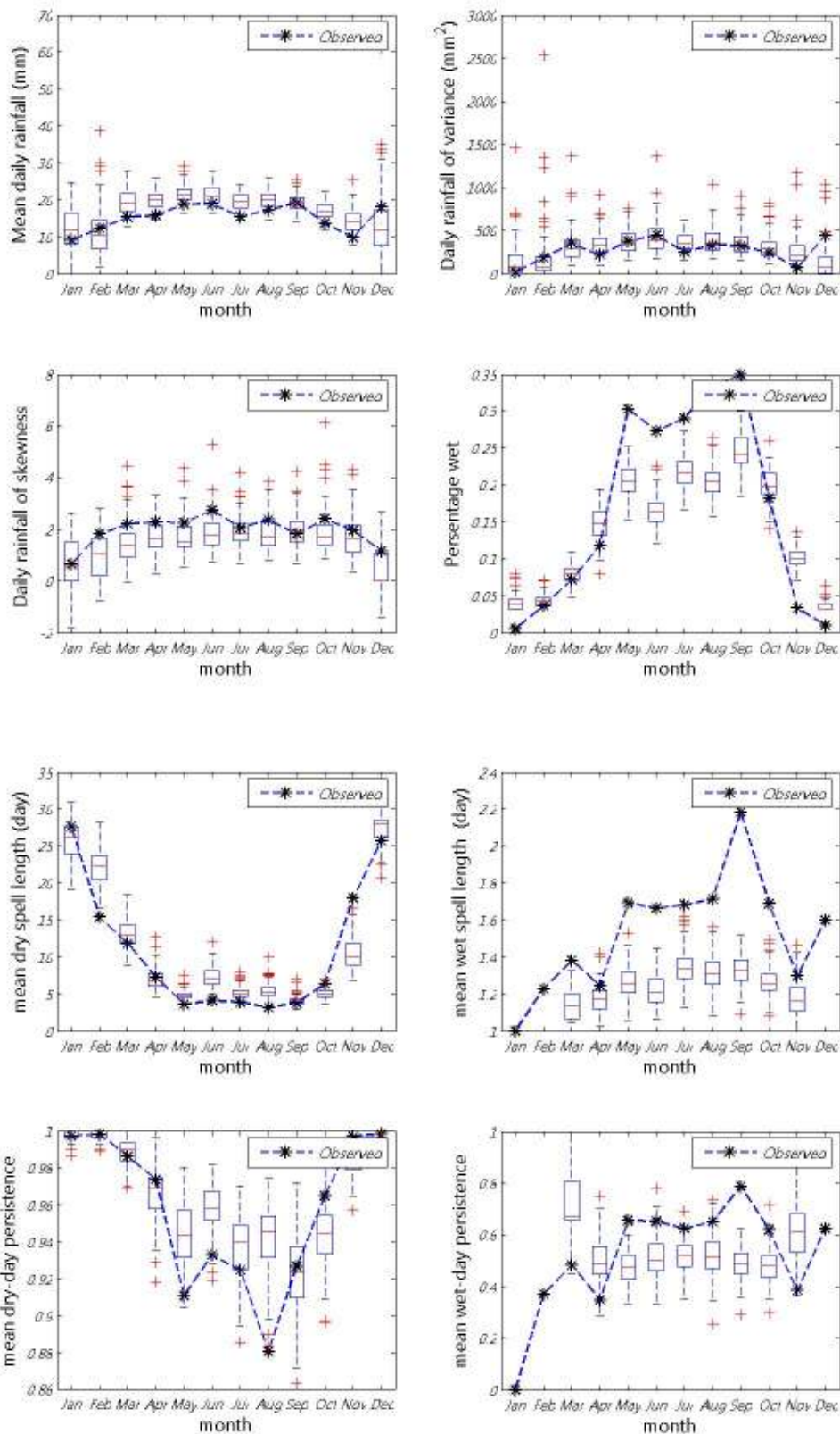
ภาพที่ ข.22 ค่าเฉลี่ย ความแปรปรวน สัมประสิทธิ์ความเบ้ เปอร์เซ็นต์ที่ฝนตก ช่วงเวลาที่ฝนหยุดและตก และจำนวนครั้งสัมผัสที่ฝนหยุดและตก ของข้อมูลฝนรายวันอดีตกับข้อมูลสังเคราะห์สำหรับสถานี 14062 (ปี ค.ศ.1991-2001)
