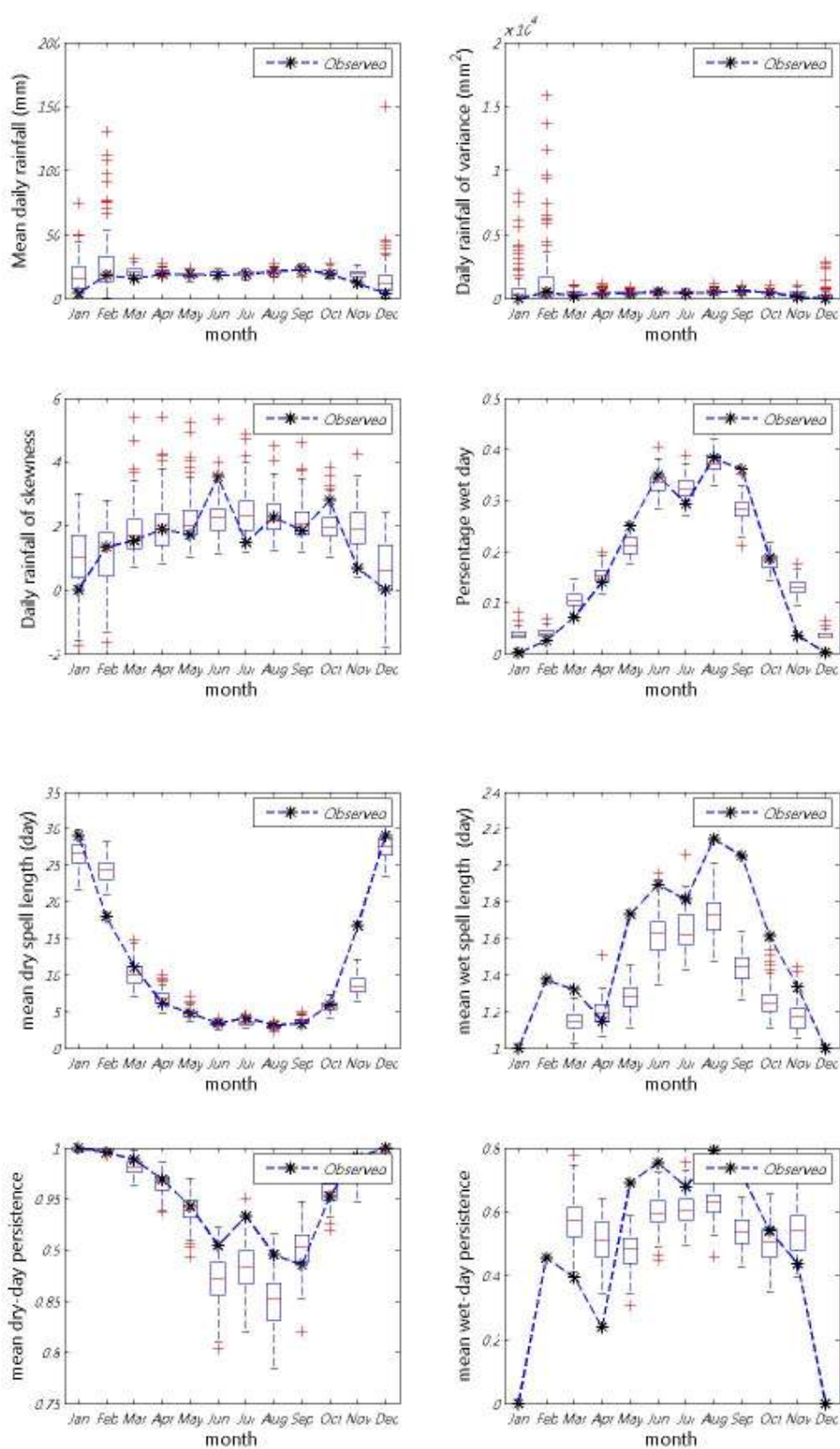
ภาพที่ ข.47 ค่าเฉลี่ย ความแปรปรวน สัมประสิทธิ์ความเบ้ เปอร์เซนต์ที่ฝนตก ช่วงเวลาที่ฝนหยุดและตก และจำนวนครั้งสัมผัสที่ฝนหยุดและตก ของข้อมูลฝนรายวันอดีตกับข้อมูลสังเคราะห์สำหรับสถานี 405002 (ปี ค.ศ. 1976-1990)
