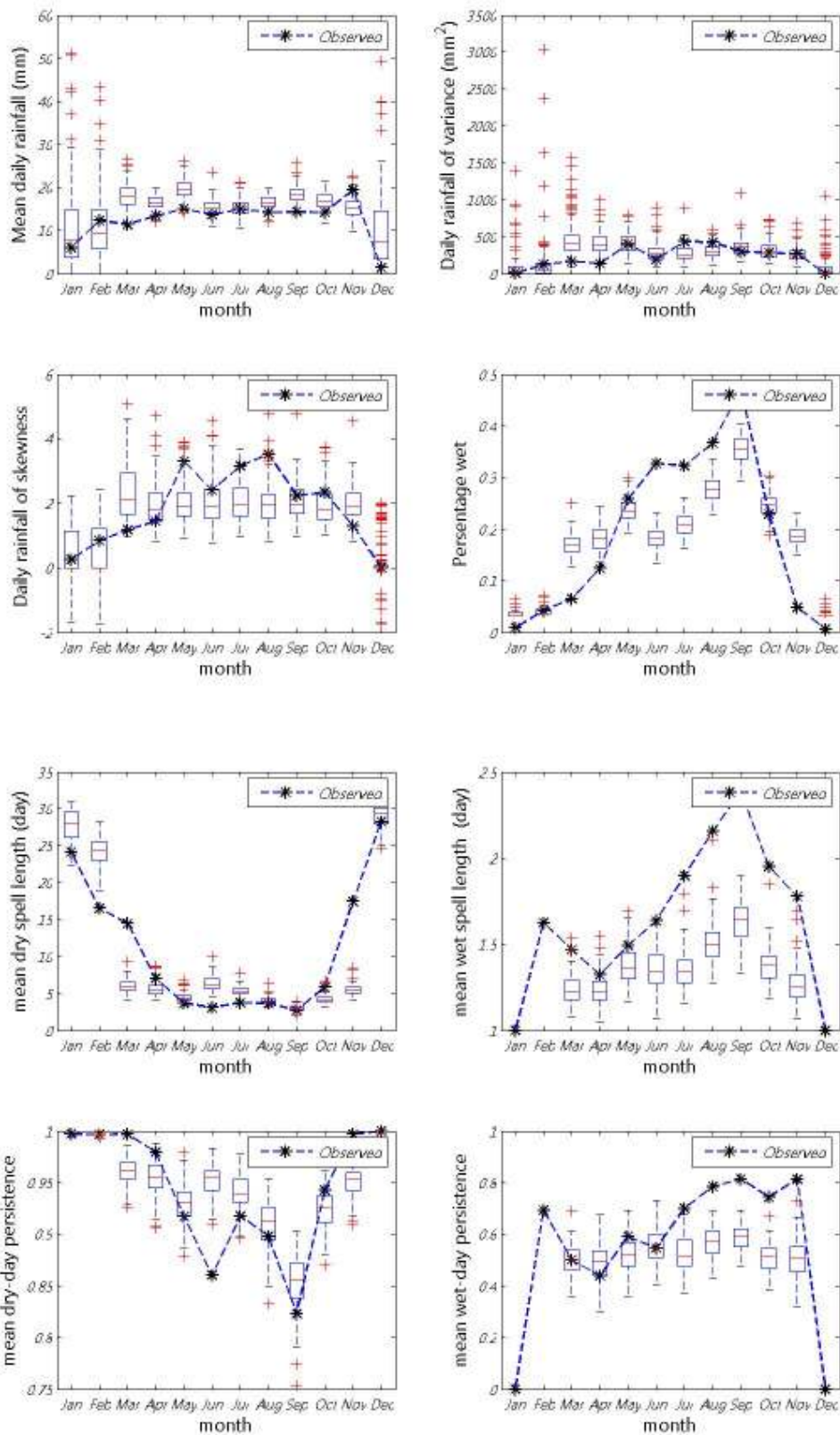
ภาพที่ ข.76 ค่าเฉลี่ย ความแปรปรวน สัมประสิทธิ์ความเบ้ เปอร์เซนต์ที่ฝนตก ช่วงเวลาที่ฝนหยุดและตก และจำนวนครั้งสัมผัสที่ฝนหยุดและตก ของข้อมูลฝนรายวันอดีตกับข้อมูลสังเคราะห์สำหรับสถานี 436004 (ปี ค.ศ.1991-2001)
