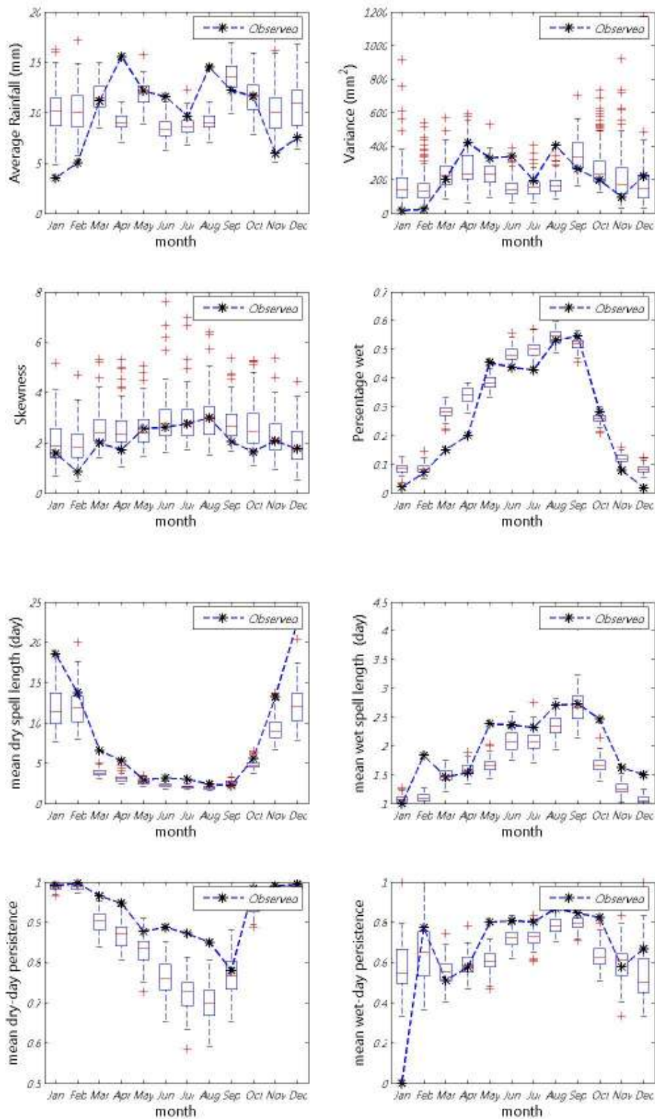
ภาพที่ ข.2 ค่าเฉลี่ย ความแปรปรวน สัมประสิทธิ์ความเบ้ เปอร์เซนต์ที่ฝนตก ช่วงเวลาที่ฝนหยุดและตก และจำนวนครั้งสัมผัสที่ฝนหยุดและตก ของข้อมูลฝนรายวันอดีตกับข้อมูลสังเคราะห์ สำหรับสถานี 05013 (ปี ค.ศ.1991-2001)
