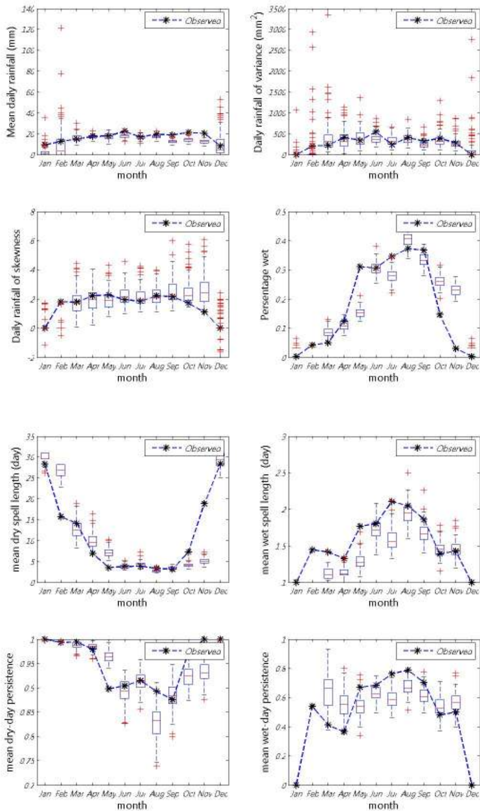
ภาพที่ ข.50 ค่าเฉลี่ย ความแปรปรวน สัมประสิทธิ์ความเบ้ เปอร์เซ็นต์ที่ฝนตก ช่วงเวลาที่ฝนหยุดและตก และจำนวนครั้งสัมผัสที่ฝนหยุดและตก ของข้อมูลฝนรายวันอดีตกับข้อมูลสังเคราะห์สำหรับสถานี 405008 (ปี ค.ศ.1991-2001)
