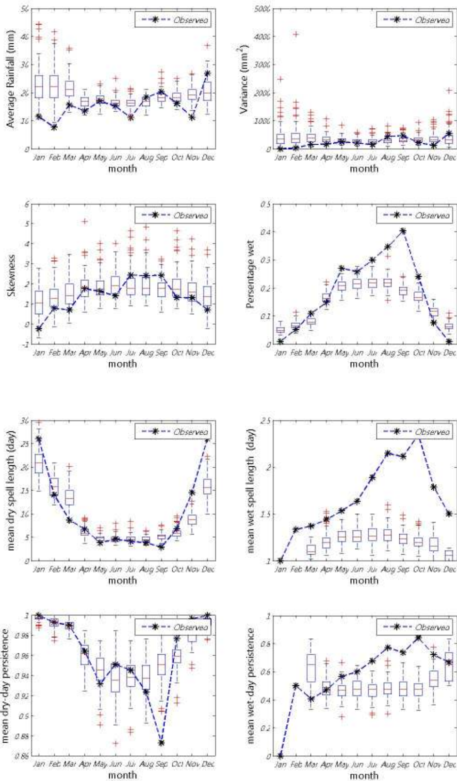
ภาพที่ ข.6 ค่าเฉลี่ย ความแปรปรวน สัมประสิทธิ์ความเบ้ เปอร์เซนต์ที่ฝนตก ช่วงเวลาที่ฝนหยุดและตก และจำนวนครั้งสัมผัสที่ฝนหยุดและตก ของข้อมูลฝนรายวันอดีตกับข้อมูลสังเคราะห์ สำหรับสถานี 05032 (ปี ค.ศ.1991-2001)
