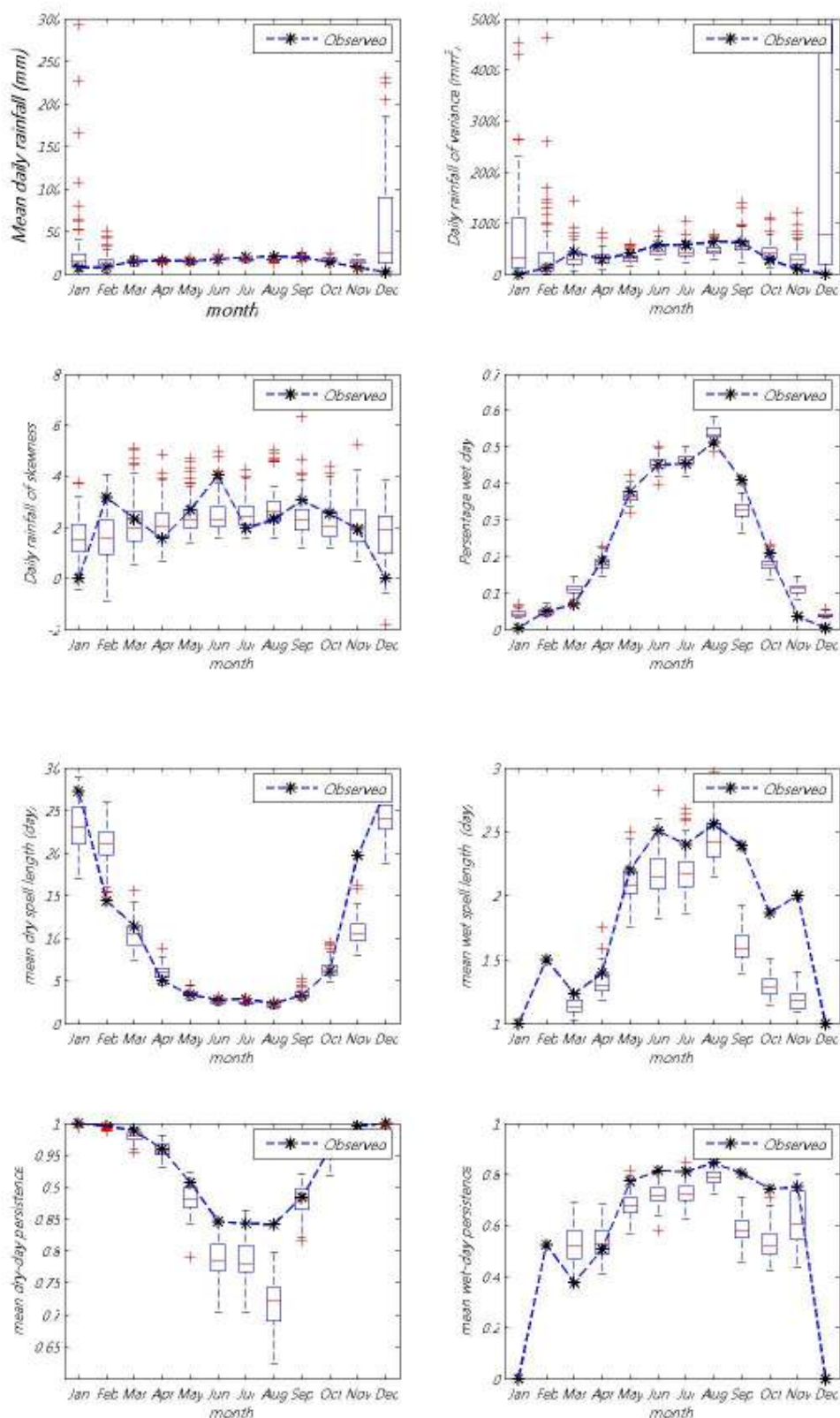
ภาพที่ ข.17 ค่าเฉลี่ย ความแปรปรวน สัมประสิทธิ์ความเบ้ เปอร์เซนต์ที่ฝนตก ช่วงเวลาที่ฝนหยุด และตก และจำนวนครั้งสัมผัสที่ฝนหยุดและตก ของข้อมูลฝนรายวันอดีตกับข้อมูลสังเคราะห์ สำหรับสถานี 11210 (ปี ค.ศ. 1976-1990)
