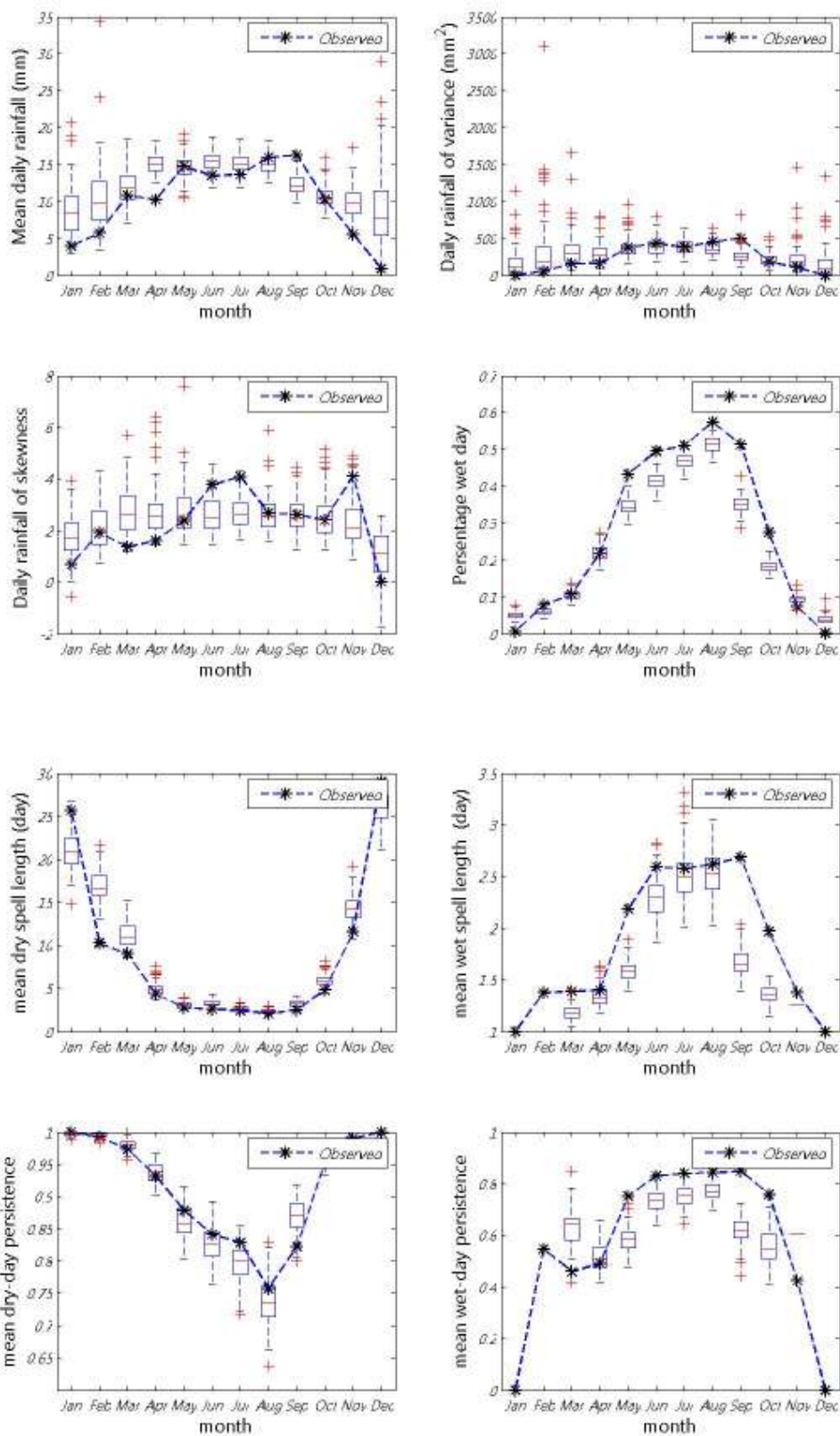
ภาพที่ ข.35 ค่าเฉลี่ย ความแปรปรวน สัมประสิทธิ์ความเบ้ เปอร์เซนต์ที่ฝนตก ช่วงเวลาที่ฝนหยุดและตก และจำนวนครั้งสัมผัสที่ฝนหยุดและตก ของข้อมูลฝนรายวันอดีตกับข้อมูลสังเคราะห์สำหรับสถานี 49301 (ปี ค.ศ. 1976-1990)
