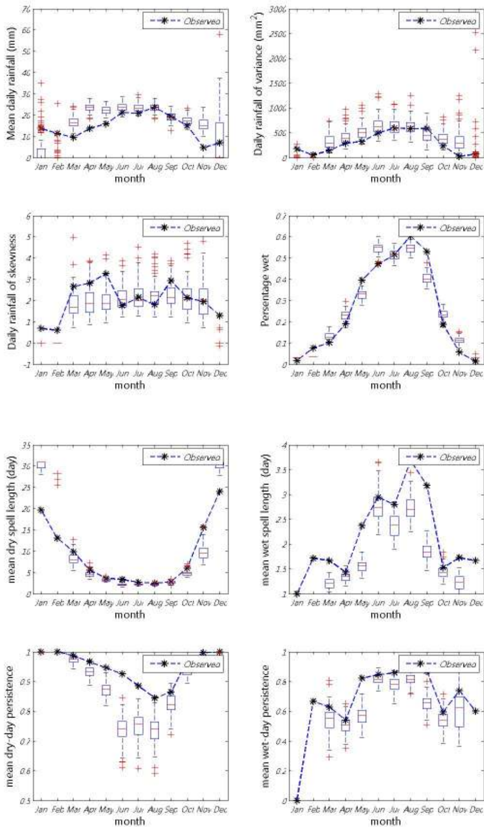
ภาพที่ ข.54 ค่าเฉลี่ย ความแปรปรวน สัมประสิทธิ์ความเบ้ เปอร์เซนต์ที่ฝนตก ช่วงเวลาที่ฝนหยุดและตก และจำนวนครั้งสัมผัสที่ฝนหยุดและตก ของข้อมูลฝนรายวันอดีตกับข้อมูลสังเคราะห์สำหรับสถานี 406004 (ปี ค.ศ.1991-2001)
