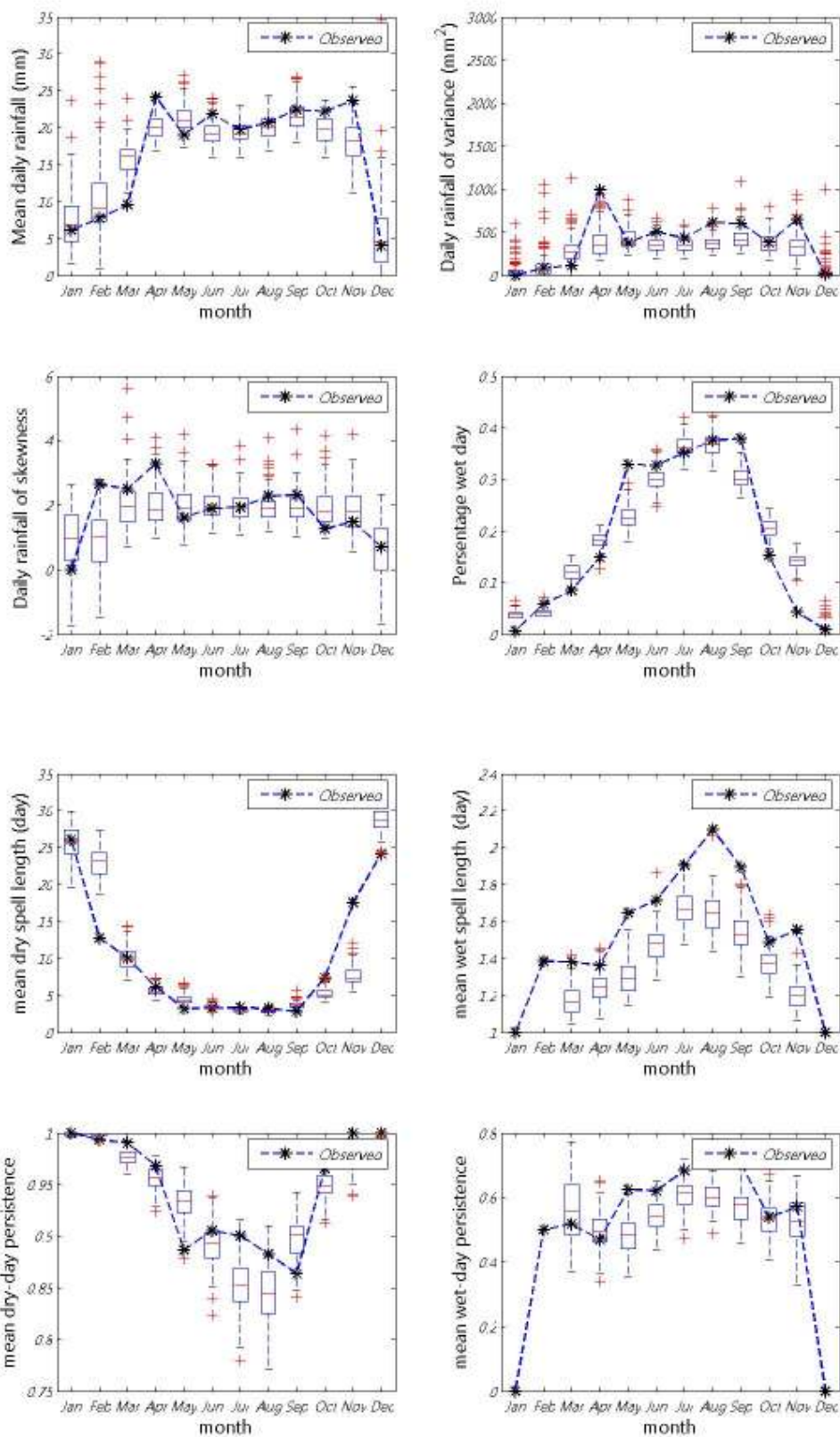
ภาพที่ ข.65 ค่าเฉลี่ย ความแปรปรวน สัมประสิทธิ์ความเบ้ เปอร์เซ็นต์ที่ฝนตก ช่วงเวลาที่ฝนหยุดและตก และจำนวนครั้งสัมผัสที่ฝนหยุดและตก ของข้อมูลฝนรายวันอดีตกับข้อมูลสังเคราะห์สำหรับสถานี 409004 (ปี ค.ศ. 1976-1990)
