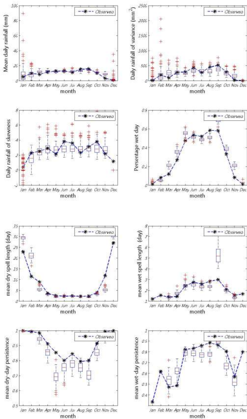
ภาพที่ ข.31 ค่าเฉลี่ย ความแปรปรวน สัมประสิทธิ์ความเบ้ เปอร์เซ็นต์ที่ฝนตก ช่วงเวลาที่ฝนหยุดและตก และจำนวนครั้งสัมผัสที่ฝนหยุดและตก ของข้อมูลฝนรายวันอดีตกับข้อมูลสังเคราะห์สำหรับสถานี 49013 (ปี ค.ศ. 1976-1990)
