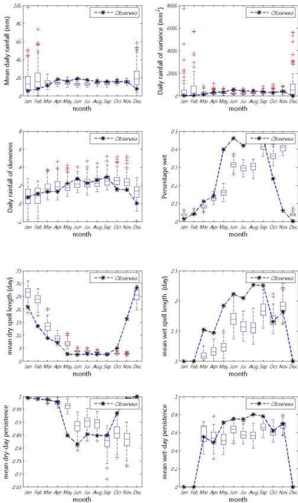
ภาพที่ ข.68 ค่าเฉลี่ย ความแปรปรวน สัมประสิทธิ์ความเบ้ เปอร์เซนต์ที่ฝนตก ช่วงเวลาที่ฝนหยุดและตก และจำนวนครั้งสัมผัสที่ฝนหยุดและตก ของข้อมูลฝนรายวันอดีตกับข้อมูลสังเคราะห์สำหรับสถานี 432001 (ปี ค.ศ.1991-2001)
