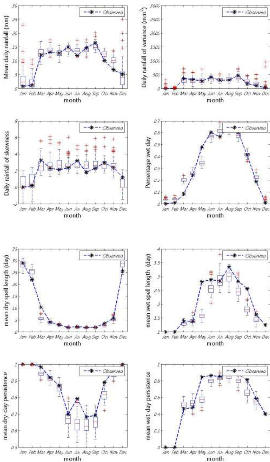
ภาพที่ ข.57 ค่าเฉลี่ย ความแปรปรวน สัมประสิทธิ์ความเบ้ เปอร์เซนต์ที่ฝนตก ช่วงเวลาที่ฝนหยุดและตก และจำนวนครั้งสัมผัสที่ฝนหยุดและตก ของข้อมูลฝนรายวันอดีตกับข้อมูลสังเคราะห์ สำหรับสถานี 407002 (ปี ค.ศ. 1976-1990)
