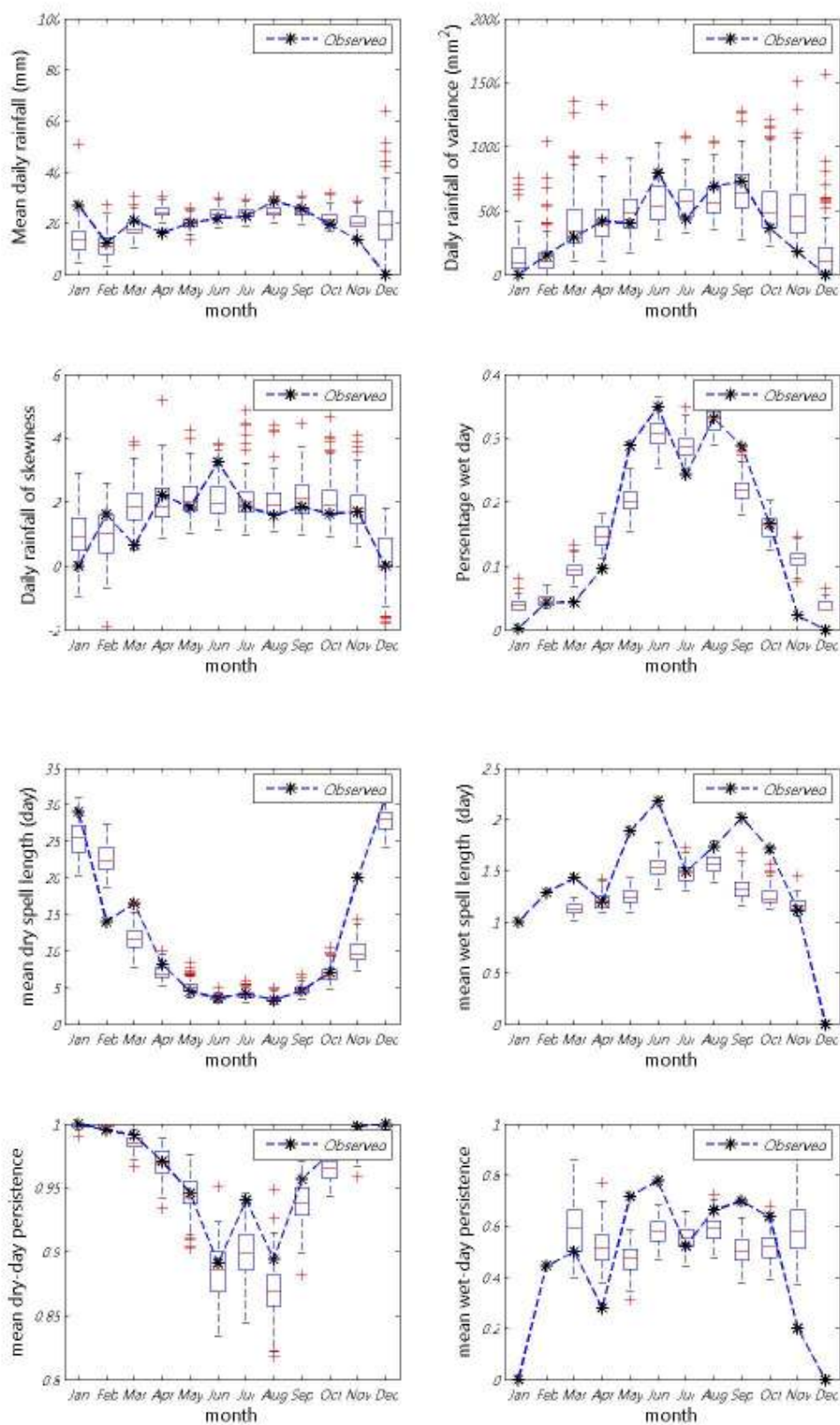
ภาพที่ ข.33 ค่าเฉลี่ย ความแปรปรวน สัมประสิทธิ์ความเบ้ เปอร์เซนต์ที่ฝนตก ช่วงเวลาที่ฝนหยุดและตก และจำนวนครั้งสัมผัสที่ฝนหยุดและตก ของข้อมูลฝนรายวันอดีตกับข้อมูลสังเคราะห์สำหรับสถานี 49062 (ปี ค.ศ. 1976-1990)
