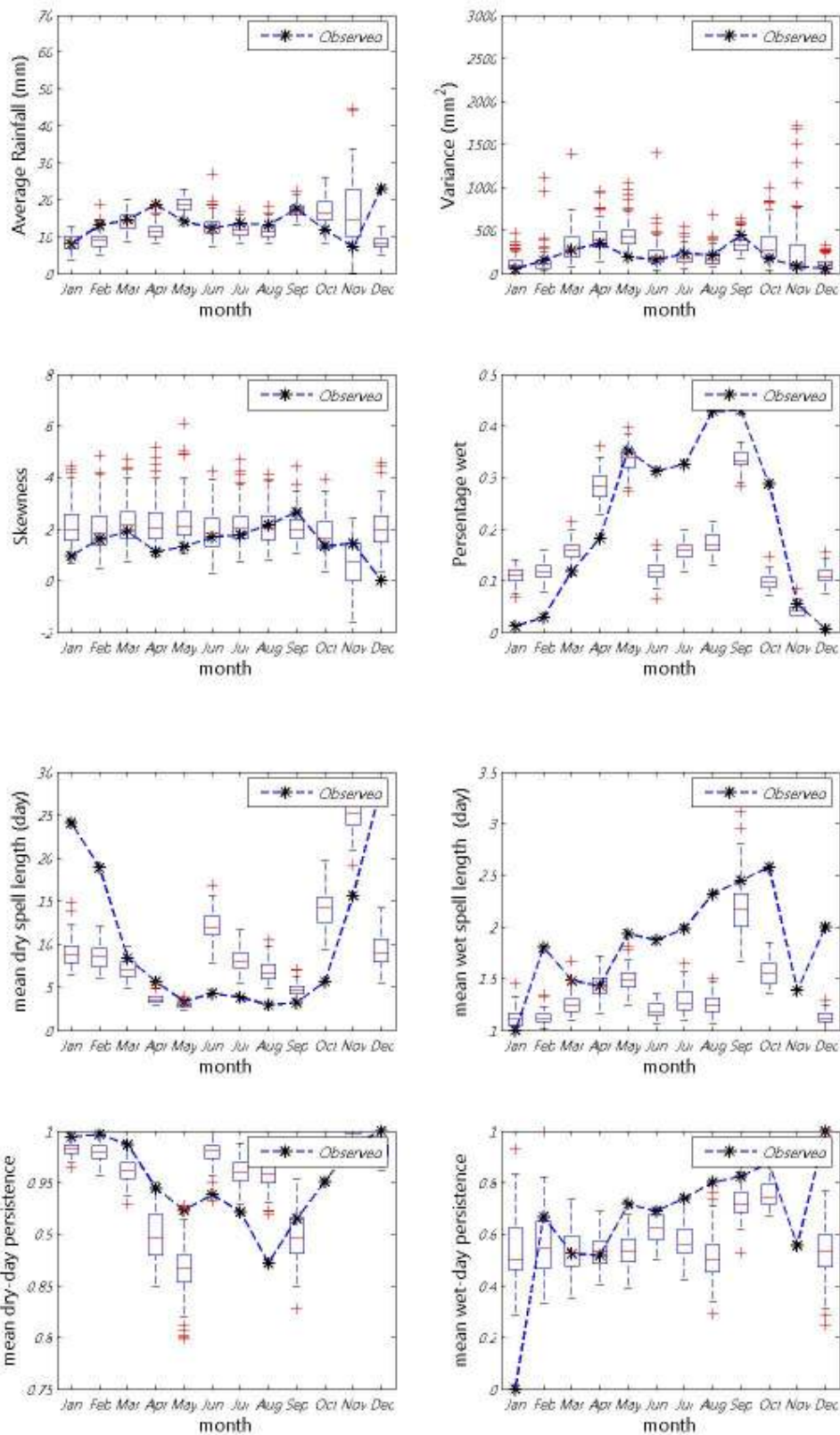
ภาพที่ ข.4 ค่าเฉลี่ย ความแปรปรวน สัมประสิทธิ์ความเบ้ เปอร์เซ็นต์ที่ฝนตก ช่วงเวลาที่ฝนหยุดและตก และจำนวนครั้งสัมผัสที่ฝนหยุดและตก ของข้อมูลฝนรายวันอดีตกับข้อมูลสังเคราะห์ สำหรับสถานี 05023 (ปี ค.ศ.1991-2001)
