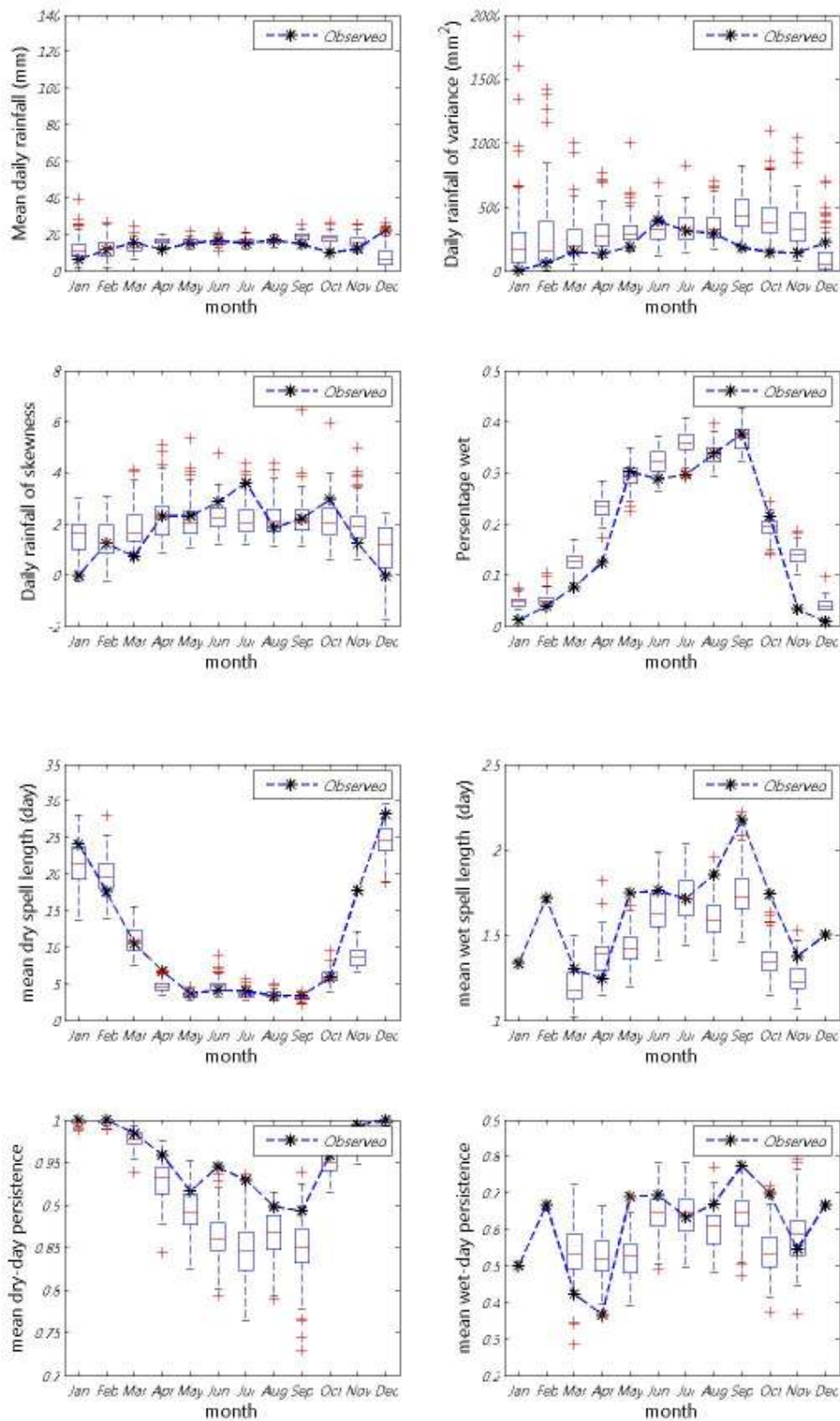
ภาพที่ ข.44 ค่าเฉลี่ย ความแปรปรวน สัมประสิทธิ์ความเบ้ เปอร์เซนต์ที่ฝนตก ช่วงเวลาที่ฝนหยุดและตก และจำนวนครั้งสัมผัสที่ฝนหยุดและตก ของข้อมูลฝนรายวันอดีตกับข้อมูลสังเคราะห์สำหรับสถานี 75052 (ปี ค.ศ.1991-2001)
