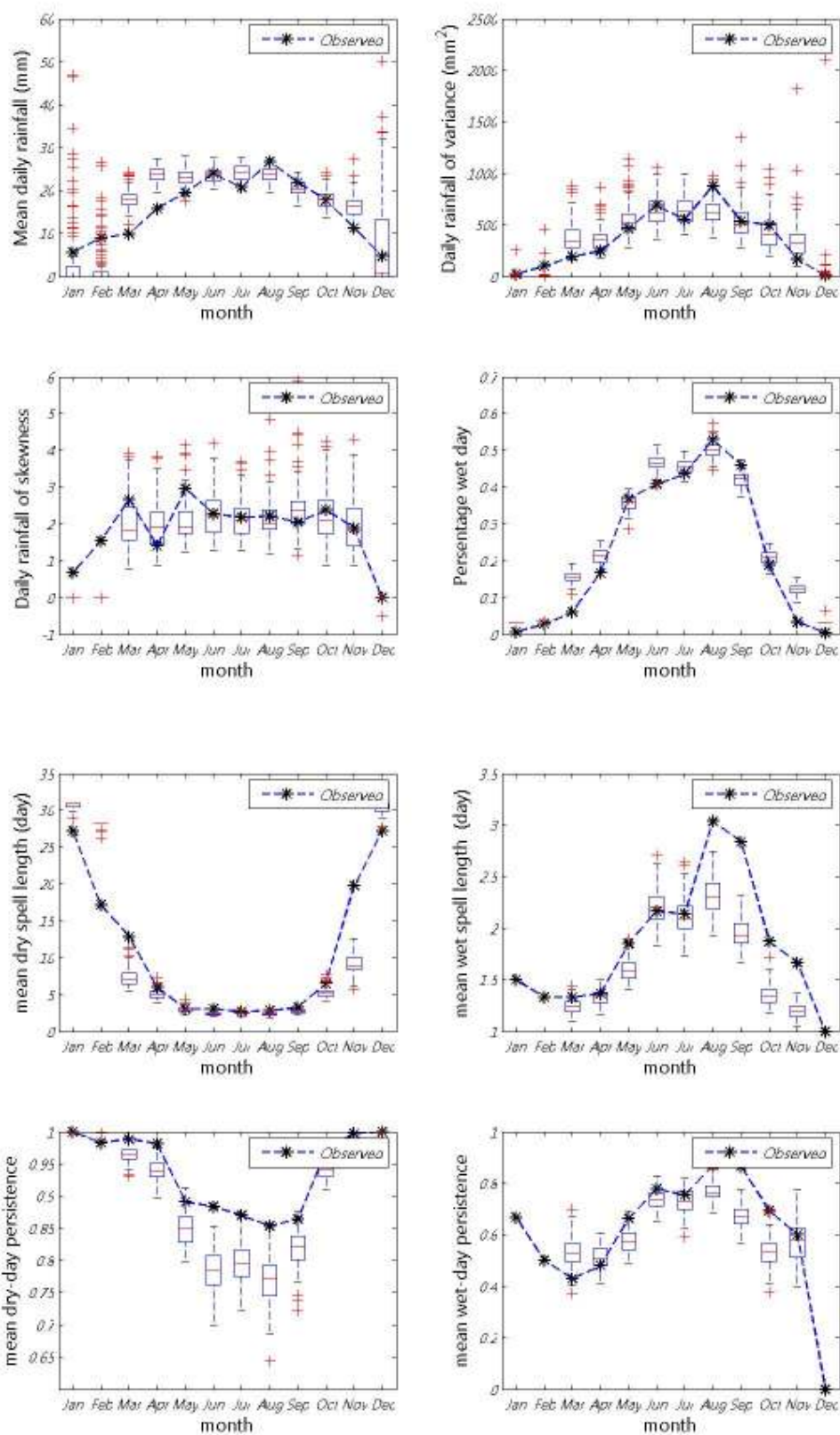
ภาพที่ ข.53 ค่าเฉลี่ย ความแปรปรวน สัมประสิทธิ์ความเบ้ เปอร์เซนต์ที่ฝนตก ช่วงเวลาที่ฝนหยุดและตก และจำนวนครั้งสัมผัสที่ฝนหยุดและตก ของข้อมูลฝนรายวันอดีตกับข้อมูลสังเคราะห์สำหรับสถานี 406004 (ปี ค.ศ. 1976-1990)
