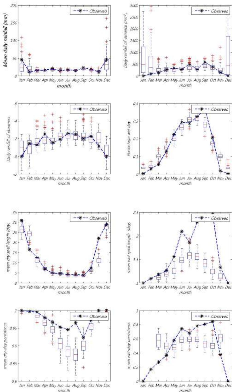
ภาพที่ ข.7 ค่าเฉลี่ย ความแปรปรวน สัมประสิทธิ์ความเบ้ เปอร์เซนต์ที่ฝนตก ช่วงเวลาที่ฝนหยุดและตก และจำนวนครั้งสัมผัสที่ฝนหยุดและตก ของข้อมูลฝนรายวันอดีตกับข้อมูลสังเคราะห์ สำหรับสถานี 05092 (ปี ค.ศ. 1976-1990)
