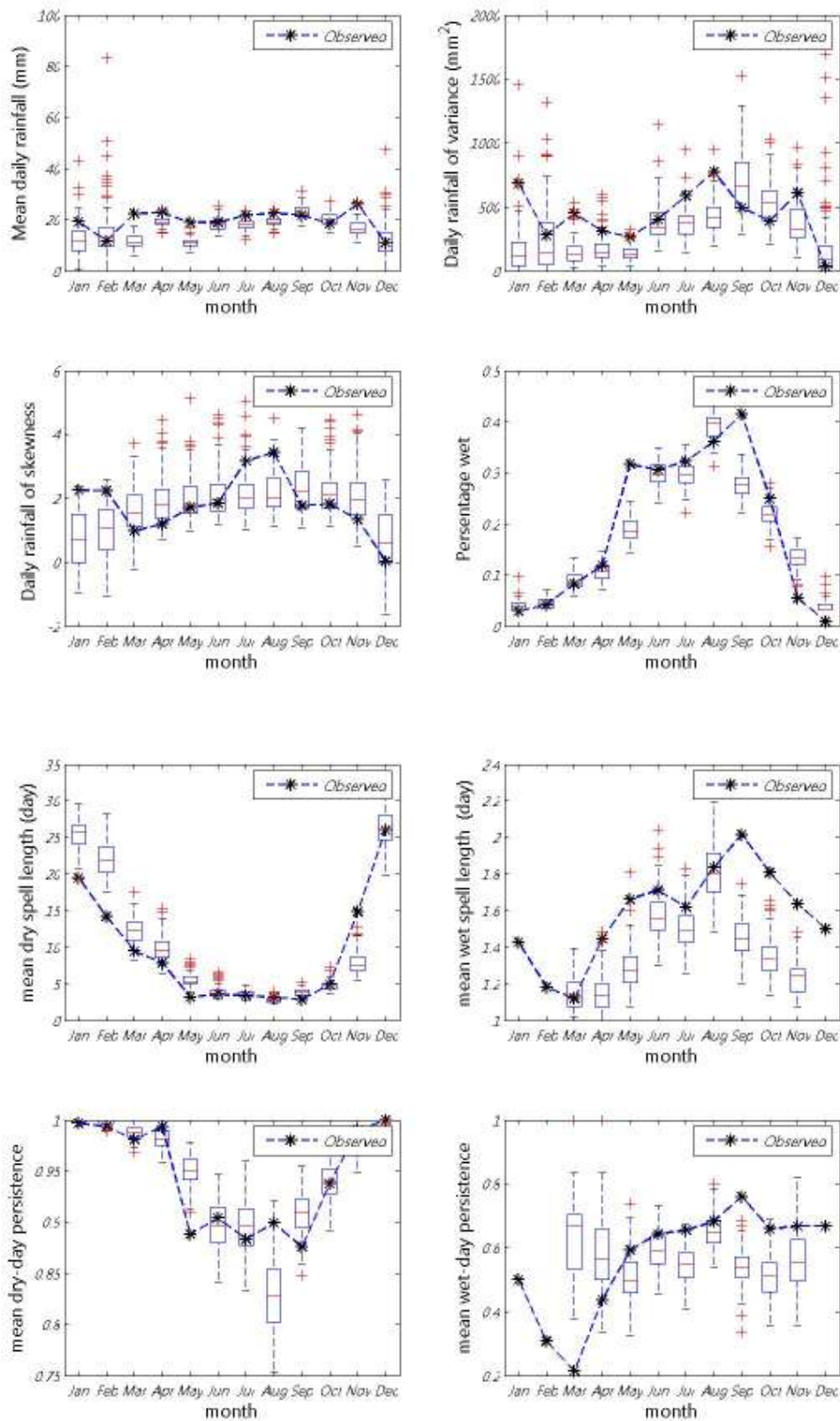
ภาพที่ ข.84 ค่าเฉลี่ย ความแปรปรวน สัมประสิทธิ์ความเบ้ เปอร์เซนต์ที่ฝนตก ช่วงเวลาที่ฝนหยุดและตก และจำนวนครั้งสัมผัสที่ฝนหยุดและตก ของข้อมูลฝนรายวันอดีตกับข้อมูลสังเคราะห์สำหรับสถานี 436013 (ปี ค.ศ.1991-2001)
