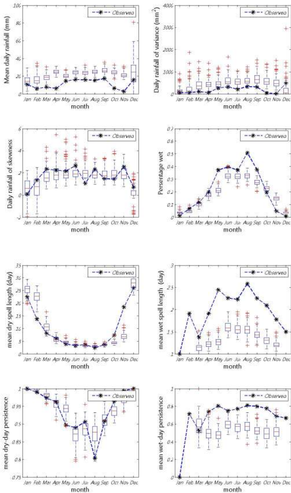
ภาพที่ ข.34 ค่าเฉลี่ย ความแปรปรวน สัมประสิทธิ์ความเบ้ เปอร์เซนต์ที่ฝนตก ช่วงเวลาที่ฝนหยุดและตก และจำนวนครั้งสัมผัสที่ฝนหยุดและตก ของข้อมูลฝนรายวันอดีตกับข้อมูลสังเคราะห์สำหรับสถานี 49062 (ปี ค.ศ.1991-2001)
