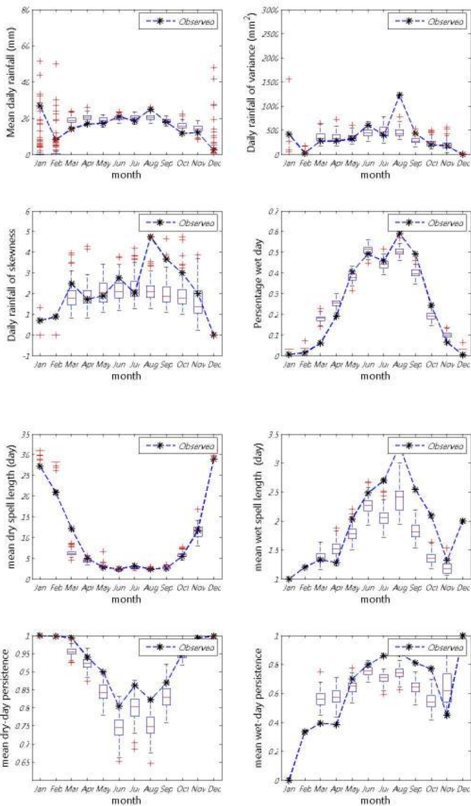
ภาพที่ ข.61 ค่าเฉลี่ย ความแปรปรวน สัมประสิทธิ์ความเบ้ เปอร์เซนต์ที่ฝนตก ช่วงเวลาที่ฝนหยุดและตก และจำนวนครั้งสัมผัสที่ฝนหยุดและตก ของข้อมูลฝนรายวันอดีตกับข้อมูลสังเคราะห์สำหรับสถานี 407009 (ปี ค.ศ. 1976-1990)
