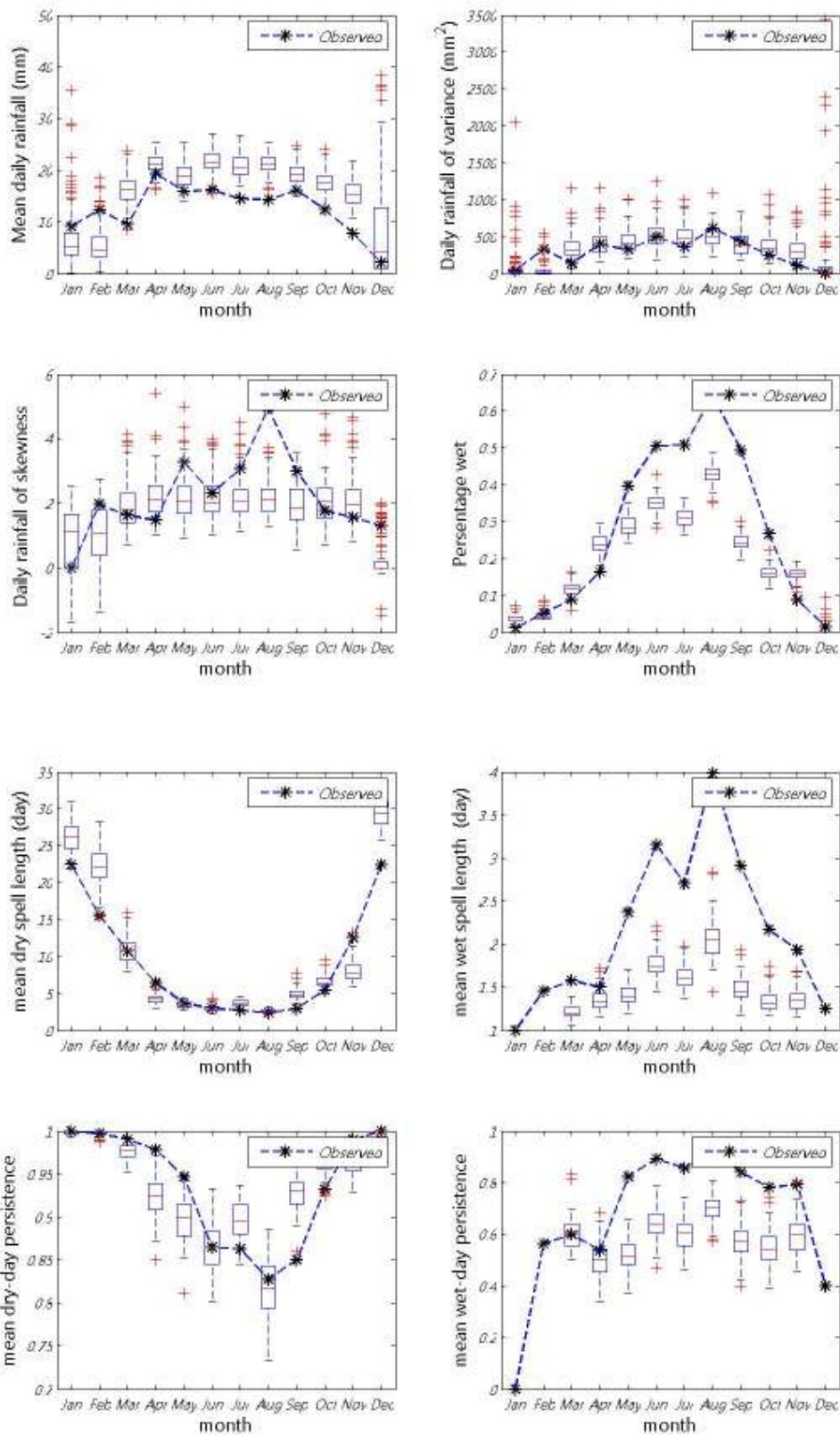
ภาพที่ ข.52 ค่าเฉลี่ย ความแปรปรวน สัมประสิทธิ์ความเบ้ เปอร์เซนต์ที่ฝนตก ช่วงเวลาที่ฝนหยุดและตก และจำนวนครั้งสัมผัสที่ฝนหยุดและตก ของข้อมูลฝนรายวันอดีตกับข้อมูลสังเคราะห์สำหรับสถานี 406002 (ปี ค.ศ.1991-2001)
