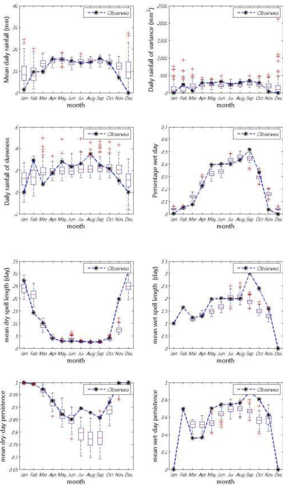
ภาพที่ ข.19 ค่าเฉลี่ย ความแปรปรวน สัมประสิทธิ์ความเบ้ เปอร์เซนต์ที่ฝนตก ช่วงเวลาที่ฝนหยุดและตก และจำนวนครั้งสัมผัสที่ฝนหยุดและตก ของข้อมูลฝนรายวันอดีตกับข้อมูลสังเคราะห์สำหรับสถานี 14052 (ปี ค.ศ. 1976-1990)
