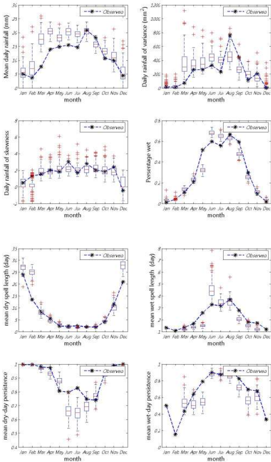
ภาพที่ ข.60 ค่าเฉลี่ย ความแปรปรวน สัมประสิทธิ์ความเบ้ เปอร์เซนต์ที่ฝนตก ช่วงเวลาที่ฝนหยุดและตก และจำนวนครั้งสัมผัสที่ฝนหยุดและตก ของข้อมูลฝนรายวันอดีตกับข้อมูลสังเคราะห์สำหรับสถานี 407006 (ปี ค.ศ.1991-2001)
