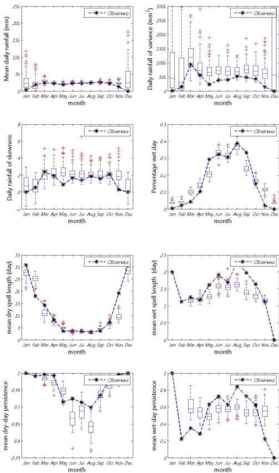
ภาพที่ ข.55 ค่าเฉลี่ย ความแปรปรวน สัมประสิทธิ์ความเบ้ เปอร์เซนต์ที่ฝนตก ช่วงเวลาที่ฝนหยุดและตก และจำนวนครั้งสัมผัสที่ฝนหยุดและตก ของข้อมูลฝนรายวันอดีตกับข้อมูลสังเคราะห์สำหรับสถานี 406005 (ปี ค.ศ. 1976-1990)
