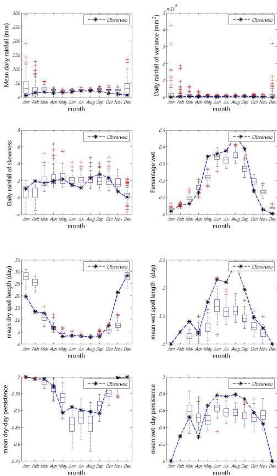
ภาพที่ ข.56 ค่าเฉลี่ย ความแปรปรวน สัมประสิทธิ์ความเบ้ เปอร์เซนต์ที่ฝนตก ช่วงเวลาที่ฝนหยุดและตก และจำนวนครั้งสัมพัทธ์ที่ฝนหยุดและตก ของข้อมูลฝนรายวันอดีตกับข้อมูลสังเคราะห์สำหรับสถานี 406005 (ปี ค.ศ.1991-2001)
