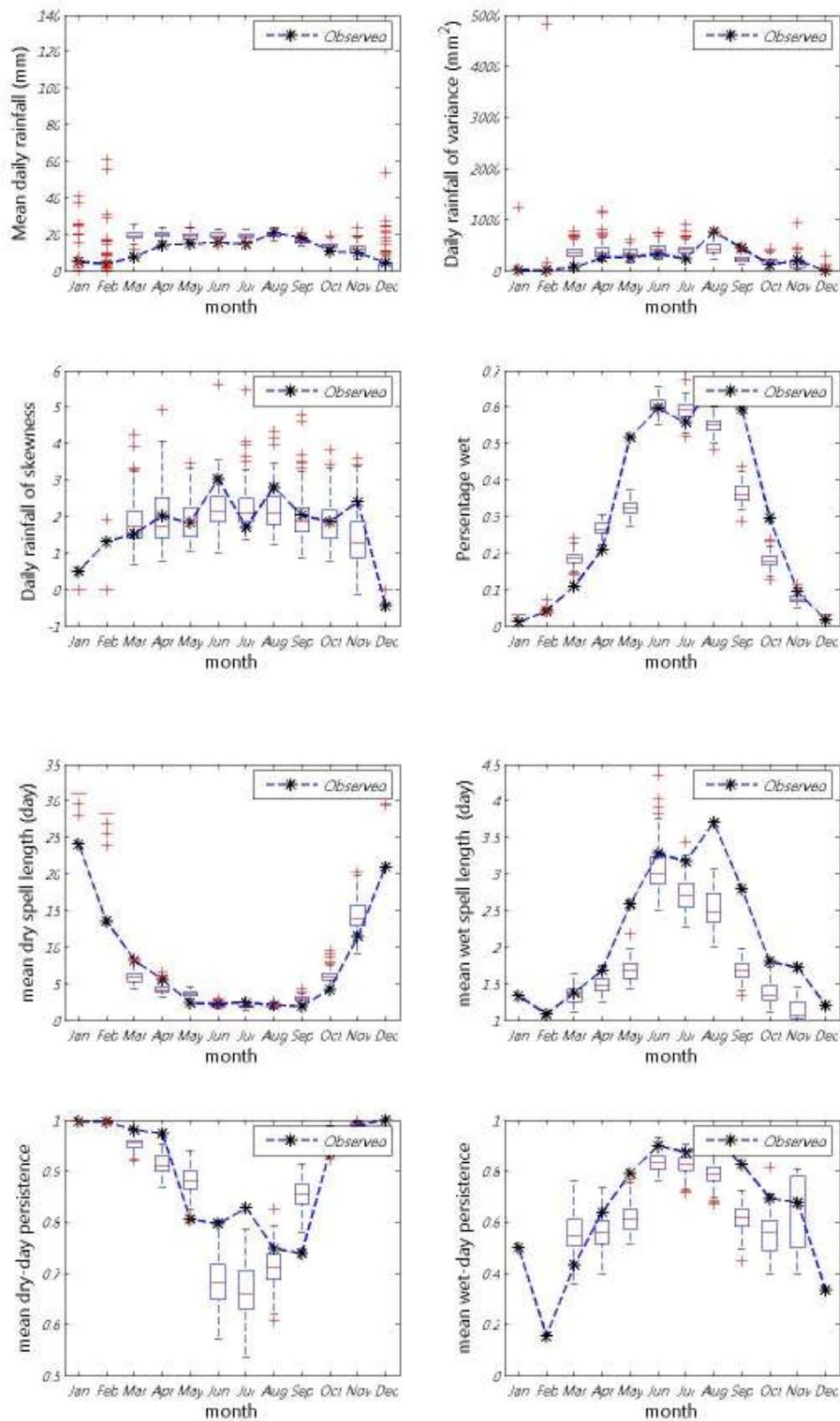
ภาพที่ ข.62 ค่าเฉลี่ย ความแปรปรวน สัมประสิทธิ์ความเบ้ เปอร์เซนต์ที่ฝนตก ช่วงเวลาที่ฝนหยุดและตก และจำนวนครั้งสัมผัสที่ฝนหยุดและตก ของข้อมูลฝนรายวันอดีตกับข้อมูลสังเคราะห์ สำหรับสถานี 407009 (ปี ค.ศ.1991-2001)
