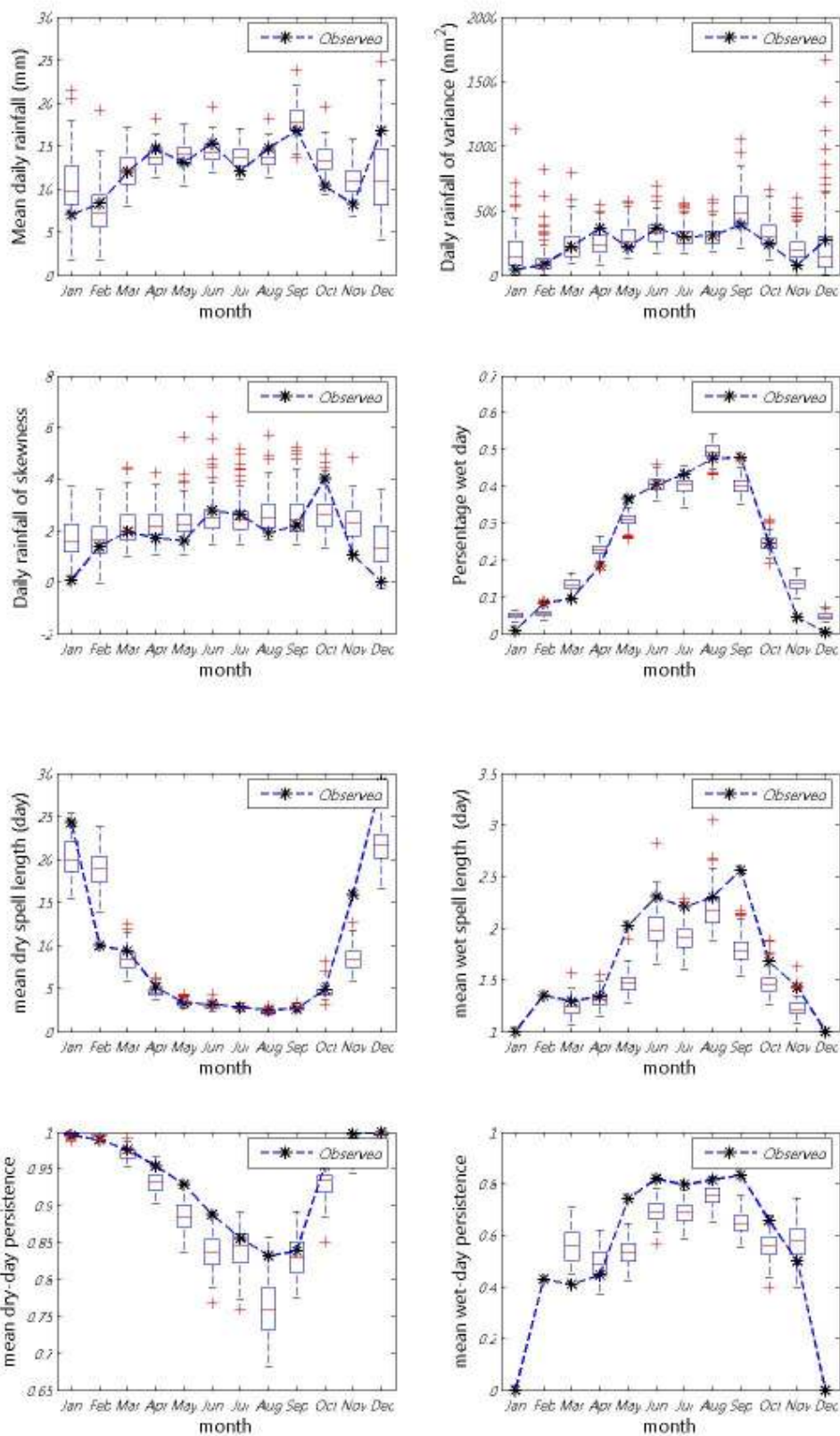
ภาพที่ ข.11 ค่าเฉลี่ย ความแปรปรวน สัมประสิทธิ์ความเบ้ เปอร์เซนต์ที่ฝนตก ช่วงเวลาที่ฝนหยุดและตก และจำนวนครั้งสัมผัสที่ฝนหยุดและตก ของข้อมูลฝนรายวันอดีตกับข้อมูลสังเคราะห์สำหรับสถานี 11022 (ปี ค.ศ. 1976-1990)
