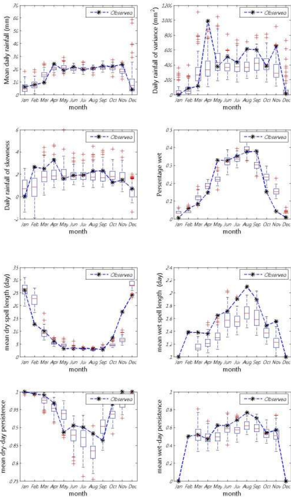
ภาพที่ ข.66 ค่าเฉลี่ย ความแปรปรวน สัมประสิทธิ์ความเบ้ เปอร์เซนต์ที่ฝนตก ช่วงเวลาที่ฝนหยุดและตก และจำนวนครั้งสัมผัสที่ฝนหยุดและตก ของข้อมูลฝนรายวันอดีตกับข้อมูลสังเคราะห์สำหรับสถานี 409004 (ปี ค.ศ.1991-2001)
