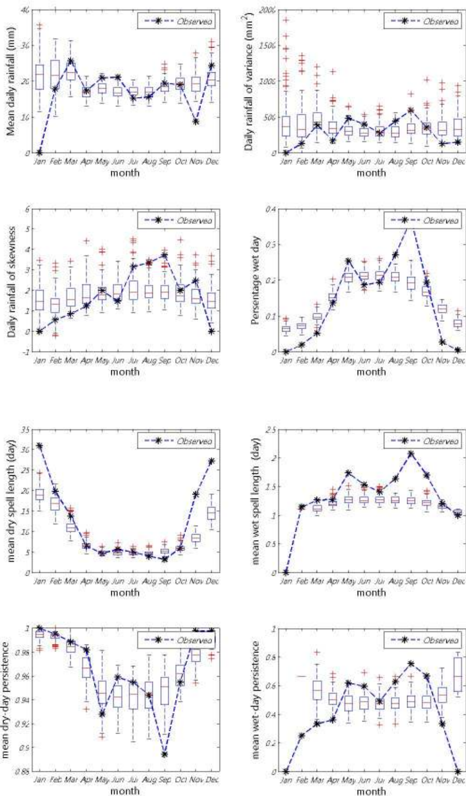
ภาพที่ ข.5 ค่าเฉลี่ย ความแปรปรวน สัมประสิทธิ์ความเบ้ เปอร์เซนต์ที่ฝนตก ช่วงเวลาที่ฝนหยุดและตก และจำนวนครั้งสัมผัสที่ฝนหยุดและตก ของข้อมูลฝนรายวันอดีตกับข้อมูลสังเคราะห์สำหรับสถานี 05032 (ปี ค.ศ. 1976-1990)
