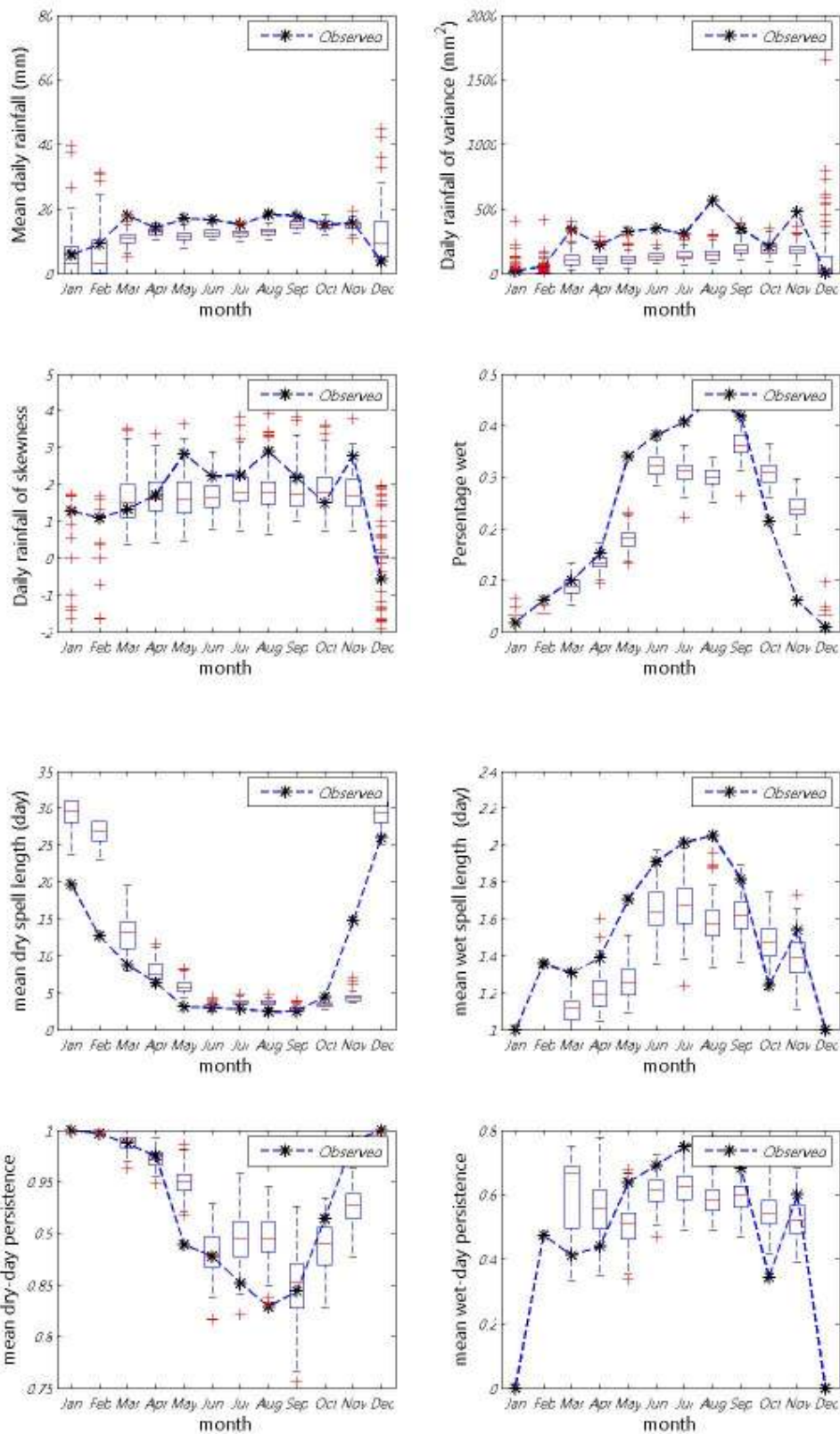
ภาพที่ ข.72 ค่าเฉลี่ย ความแปรปรวน สัมประสิทธิ์ความเบ้ เปอร์เซ็นต์ที่ฝนตก ช่วงเวลาที่ฝนหยุดและตก และจำนวนครั้งสัมพัทธ์ที่ฝนหยุดและตก ของข้อมูลฝนรายวันอดีตกับข้อมูลสังเคราะห์สำหรับสถานี 432005 (ปี ค.ศ.1991-2001)
