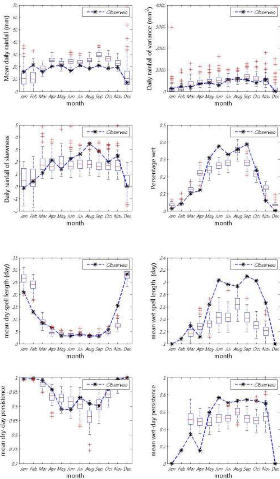
ภาพที่ ข.74 ค่าเฉลี่ย ความแปรปรวน สัมประสิทธิ์ความเบ้ เปอร์เซนต์ที่ฝนตก ช่วงเวลาที่ฝนหยุดและตก และจำนวนครั้งสัมผัสที่ฝนหยุดและตก ของข้อมูลฝนรายวันอดีตกับข้อมูลสังเคราะห์สำหรับสถานี 432006 (ปี ค.ศ.1991-2001)
