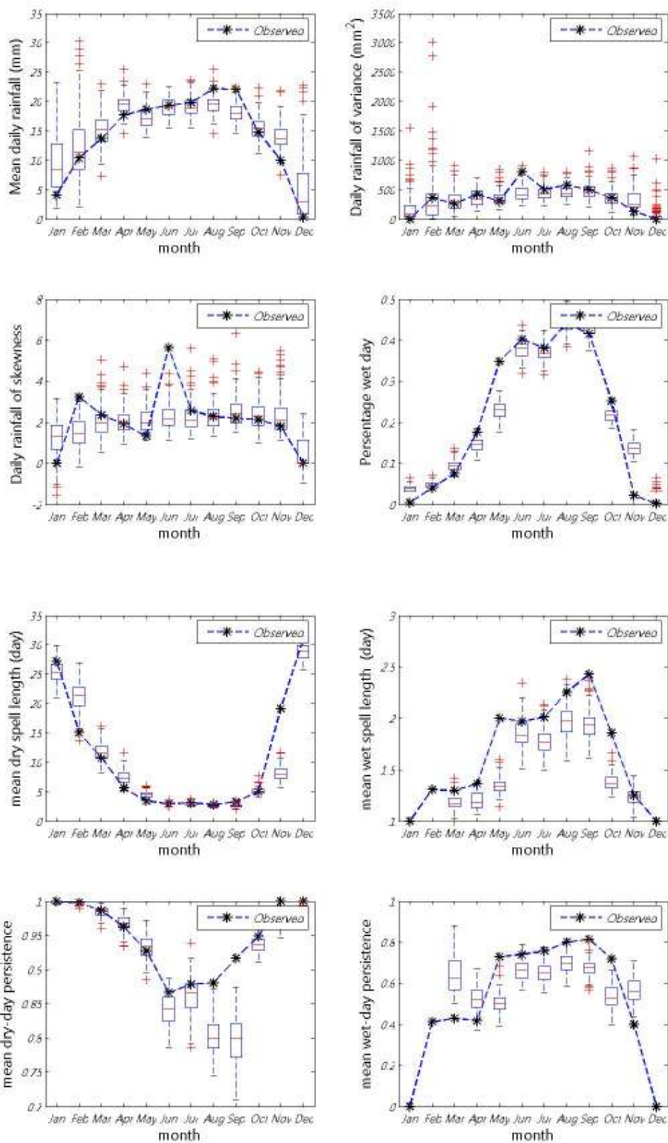
ภาพที่ ข.39 ค่าเฉลี่ย ความแปรปรวน สัมประสิทธิ์ความเบ้ เปอร์เซนต์ที่ฝนตก ช่วงเวลาที่ฝนหยุดและตก และจำนวนครั้งสัมผัสที่ฝนหยุดและตก ของข้อมูลฝนรายวันอดีตกับข้อมูลสังเคราะห์สำหรับสถานี 72022 (ปี ค.ศ. 1976-1990)
