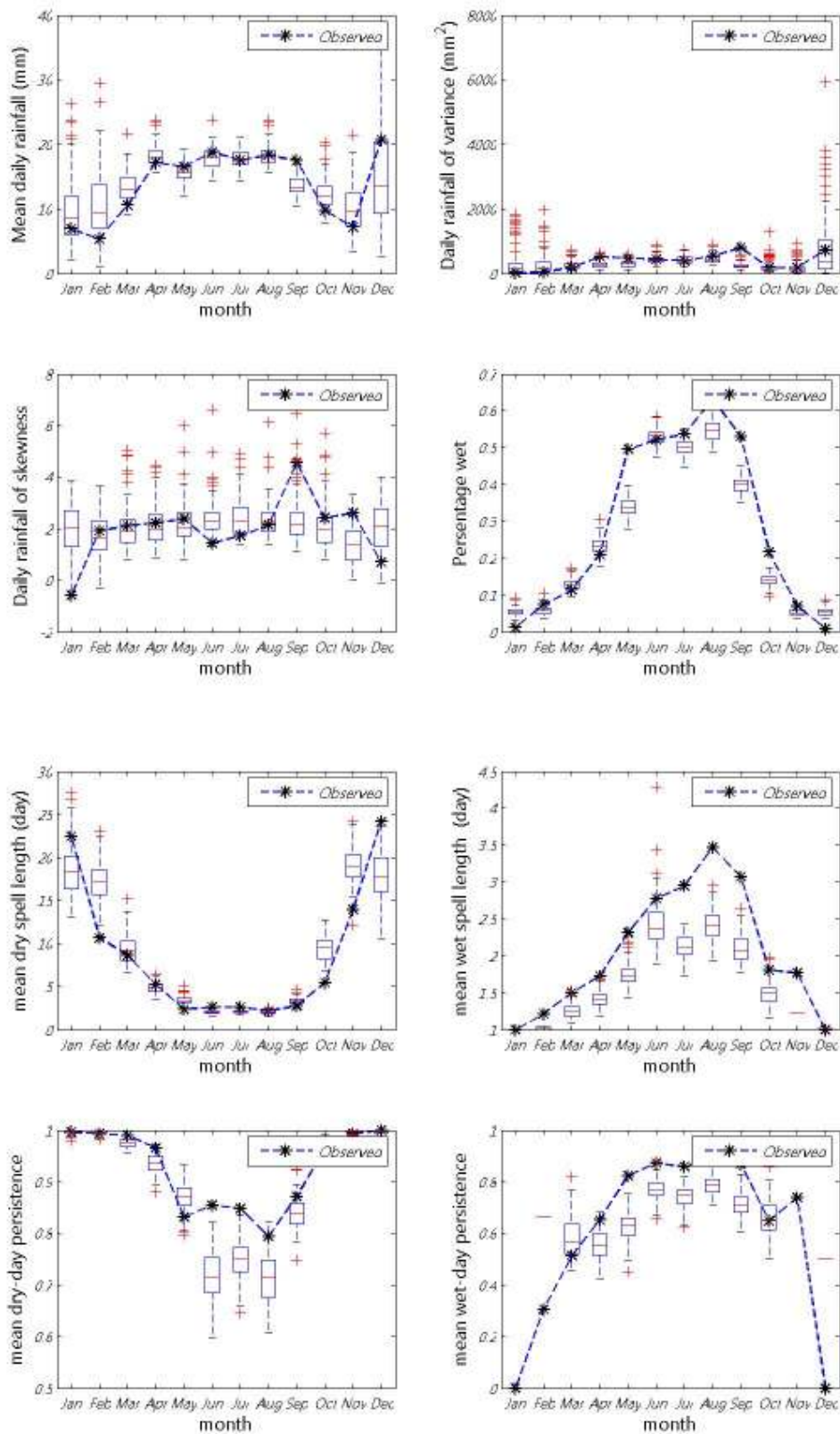
ภาพที่ ข.64 ค่าเฉลี่ย ความแปรปรวน สัมประสิทธิ์ความเบ้ เปอร์เซนต์ที่ฝนตก ช่วงเวลาที่ฝนหยุดและตก และจำนวนครั้งสัมพัทธ์ที่ฝนหยุดและตก ของข้อมูลฝนรายวันอดีตกับข้อมูลสังเคราะห์สำหรับสถานี 407015 (ปี ค.ศ.1991-2001)
