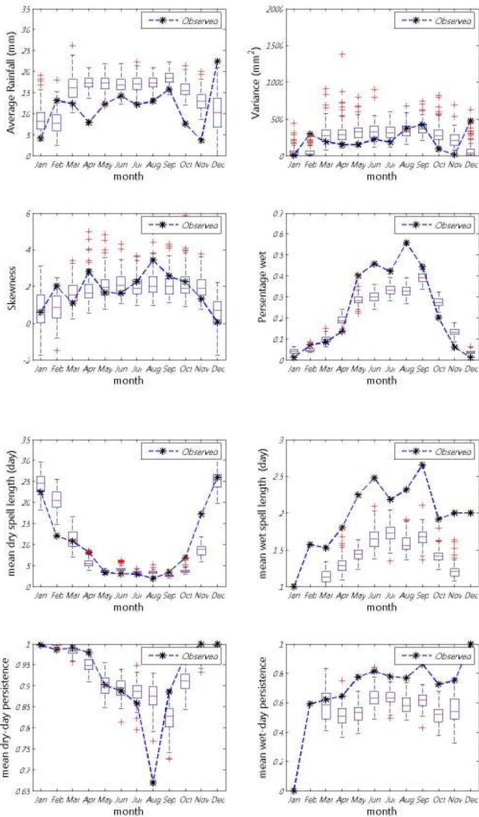
ภาพที่ ข.14 ค่าเฉลี่ย ความแปรปรวน สัมประสิทธิ์ความเบ้ เปอร์เซนต์ที่ฝนตก ช่วงเวลาที่ฝนหยุดและตก และจำนวนครั้งสัมผัสที่ฝนหยุดและตก ของข้อมูลฝนรายวันอดีตกับข้อมูลสังเคราะห์สำหรับสถานี 11170 (ปี ค.ศ.1991-2001)
