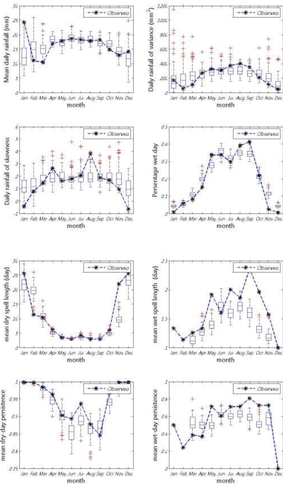
ภาพที่ ข.41 ค่าเฉลี่ย ความแปรปรวน สัมประสิทธิ์ความเบ้ เปอร์เซนต์ที่ฝนตก ช่วงเวลาที่ฝนหยุดและตก และจำนวนครั้งสัมผัสที่ฝนหยุดและตก ของข้อมูลฝนรายวันอดีตกับข้อมูลสังเคราะห์สำหรับสถานี 75032 (ปี ค.ศ. 1976-1990)
