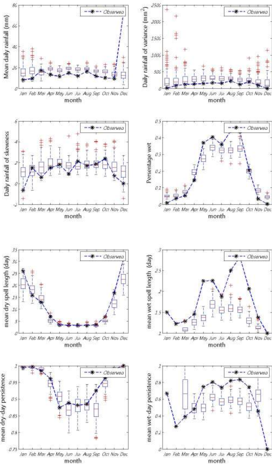
ภาพที่ ข.42 ค่าเฉลี่ย ความแปรปรวน สัมประสิทธิ์ความเบ้ เปอร์เซ็นต์ที่ฝนตก ช่วงเวลาที่ฝนหยุดและตก และจำนวนครั้งสัมผัสที่ฝนหยุดและตก ของข้อมูลฝนรายวันอดีตกับข้อมูลสังเคราะห์สำหรับสถานี 75032 (ปี ค.ศ.1991-2001)
