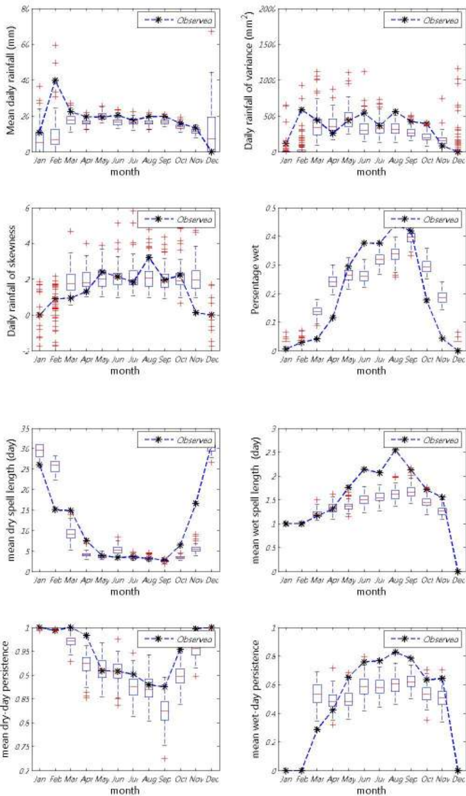
ภาพที่ ข.46 ค่าเฉลี่ย ความแปรปรวน สัมประสิทธิ์ความเบ้ เปอร์เซนต์ที่ฝนตก ช่วงเวลาที่ฝนหยุดและตก และจำนวนครั้งสัมผัสที่ฝนหยุดและตก ของข้อมูลฝนรายวันอดีตกับข้อมูลสังเคราะห์สำหรับสถานี 404003 (ปี ค.ศ.1991-2001)
