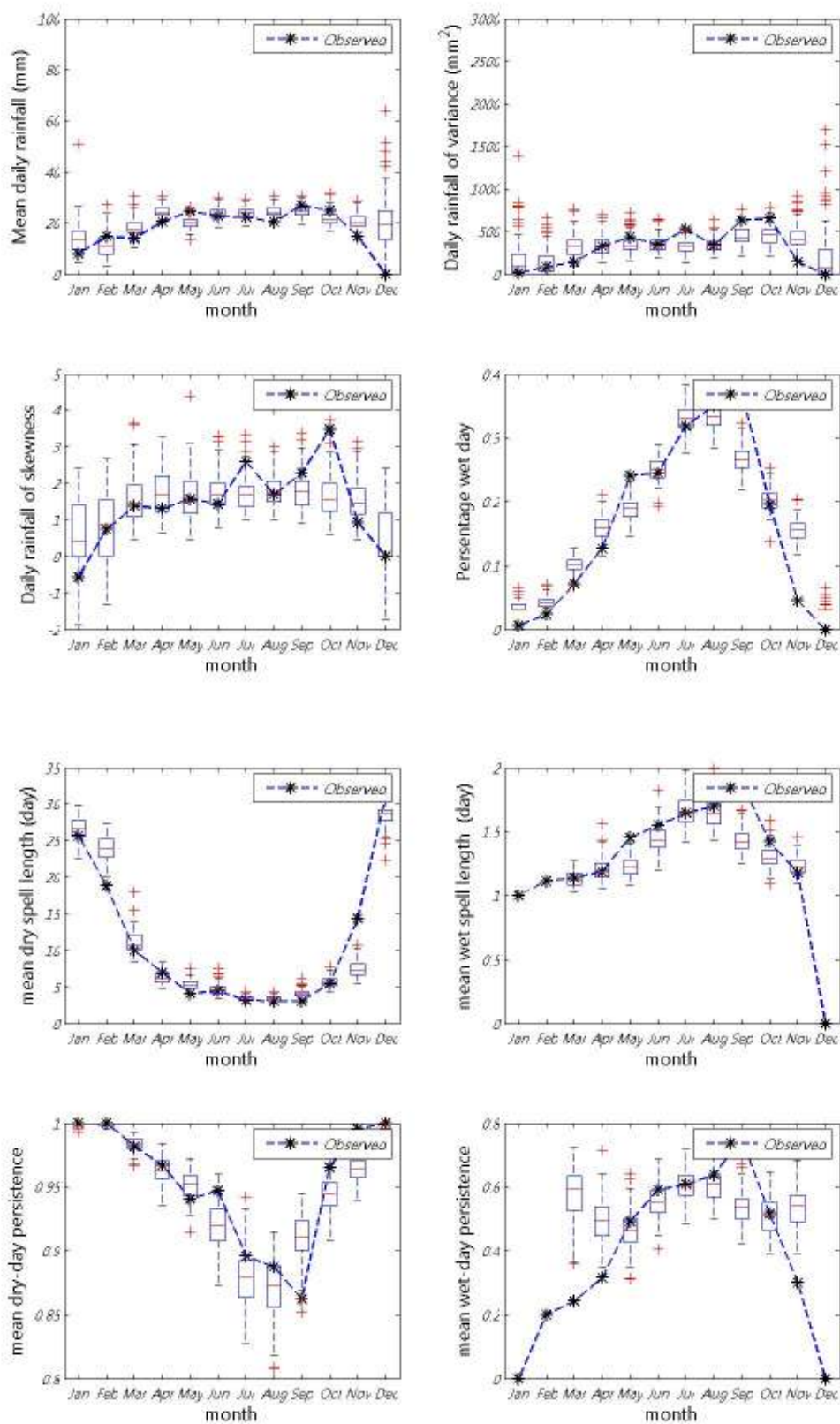
ภาพที่ ข.77 ค่าเฉลี่ย ความแปรปรวน สัมประสิทธิ์ความเบ้ เปอร์เซนต์ที่ฝนตก ช่วงเวลาที่ฝนหยุดและตก และจำนวนครั้งสัมผัสที่ฝนหยุดและตก ของข้อมูลฝนรายวันอดีตกับข้อมูลสังเคราะห์สำหรับสถานี 436005 (ปี ค.ศ. 1976-1990)
