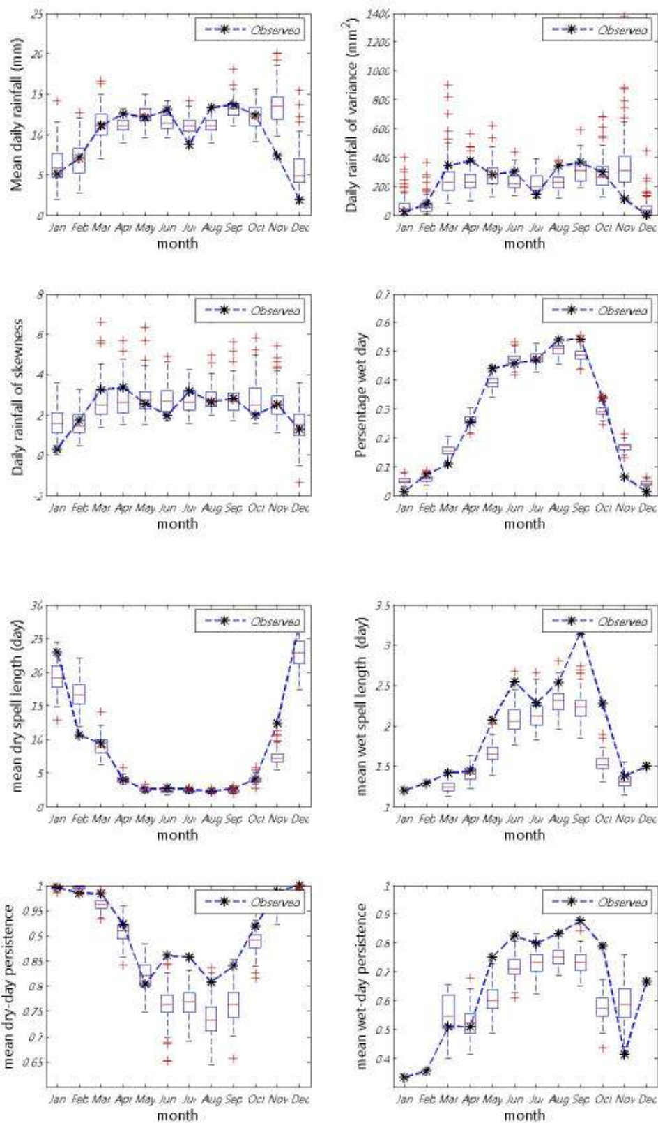
ภาพที่ ข.27 ค่าเฉลี่ย ความแปรปรวน สัมประสิทธิ์ความเบ้ เปอร์เซ็นต์ที่ฝนตก ช่วงเวลาที่ฝนหยุดและตก และจำนวนครั้งสัมผัสที่ฝนหยุดและตก ของข้อมูลฝนรายวันอดีตกับข้อมูลสังเคราะห์สำหรับสถานี 21043 (ปี ค.ศ. 1976-1990)
