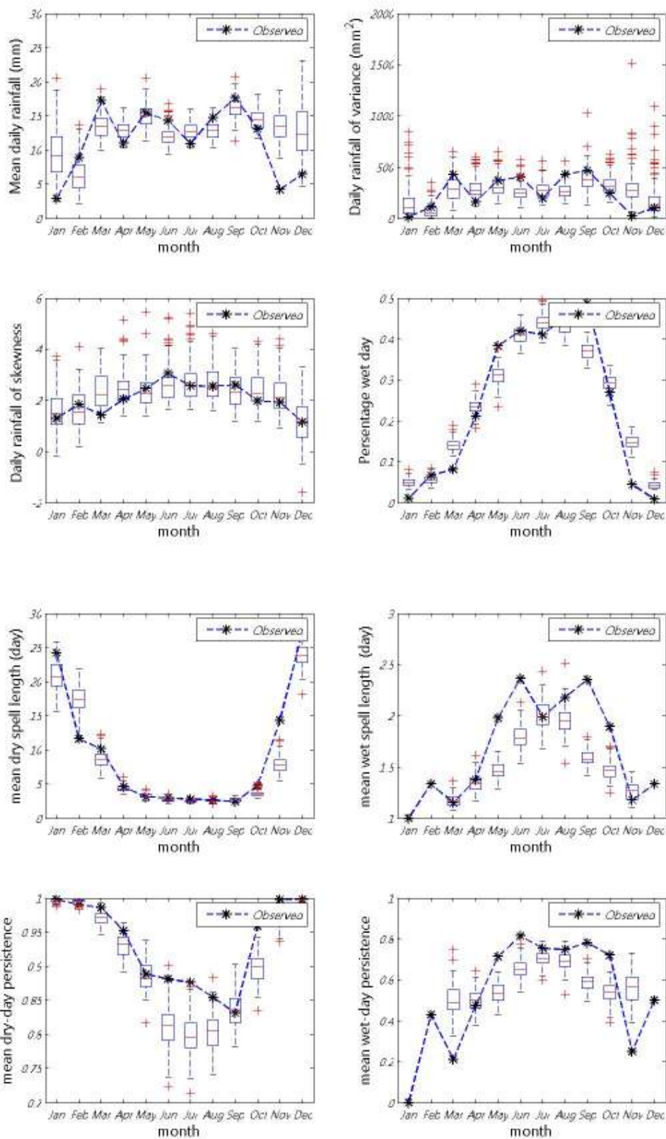
ภาพที่ ข.23 ค่าเฉลี่ย ความแปรปรวน สัมประสิทธิ์ความเบ้ เปอร์เซนต์ที่ฝนตก ช่วงเวลาที่ฝนหยุดและตก และจำนวนครั้งสัมผัสที่ฝนหยุดและตก ของข้อมูลฝนรายวันอดีตกับข้อมูลสังเคราะห์สำหรับสถานี 14112 (ปี ค.ศ. 1976-1990)
