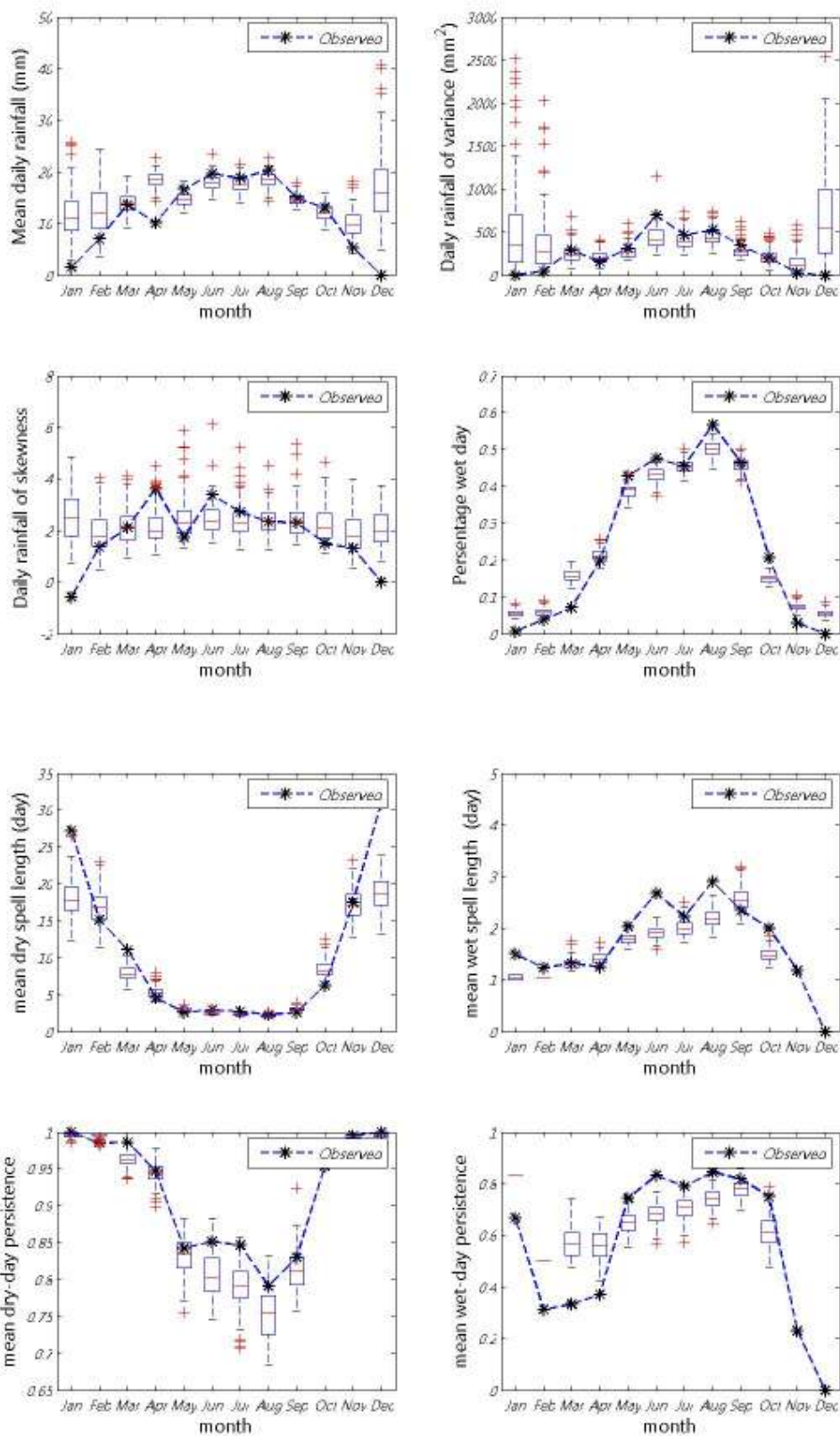
ภาพที่ ข.63 ค่าเฉลี่ย ความแปรปรวน สัมประสิทธิ์ความเบ้ เปอร์เซนต์ที่ฝนตก ช่วงเวลาที่ฝนหยุดและตก และจำนวนครั้งสัมผัสที่ฝนหยุดและตก ของข้อมูลฝนรายวันอดีตกับข้อมูลสังเคราะห์สำหรับสถานี 407015 (ปี ค.ศ. 1976-1990)
