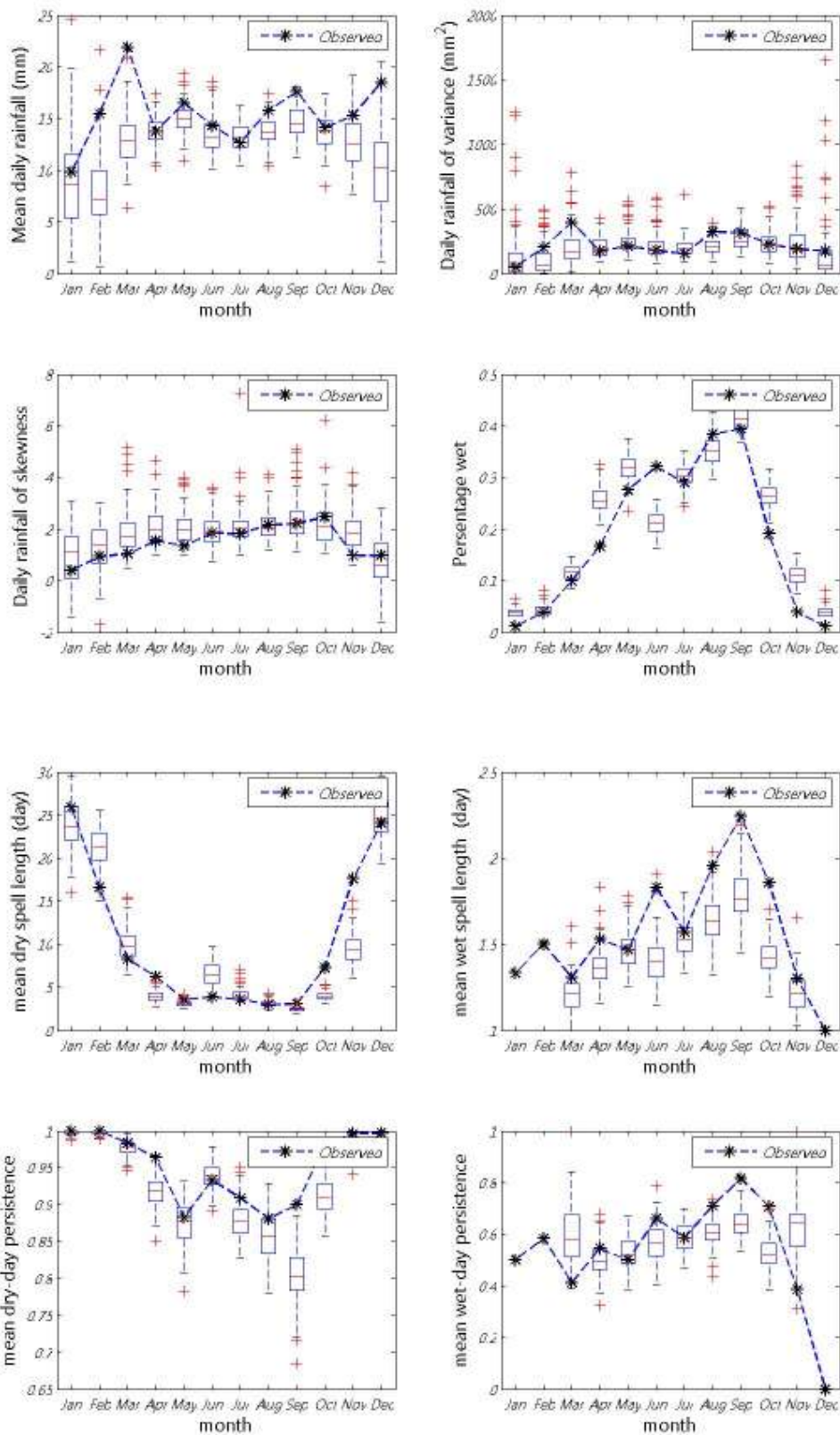
ภาพที่ ข.20 ค่าเฉลี่ย ความแปรปรวน สัมประสิทธิ์ความเบ้ เปอร์เซ็นต์ที่ฝนตก ช่วงเวลาที่ฝนหยุดและตก และจำนวนครั้งสัมผัสที่ฝนหยุดและตก ของข้อมูลฝนรายวันอดีตกับข้อมูลสังเคราะห์สำหรับสถานี 14052 (ปี ค.ศ.1991-2001)
