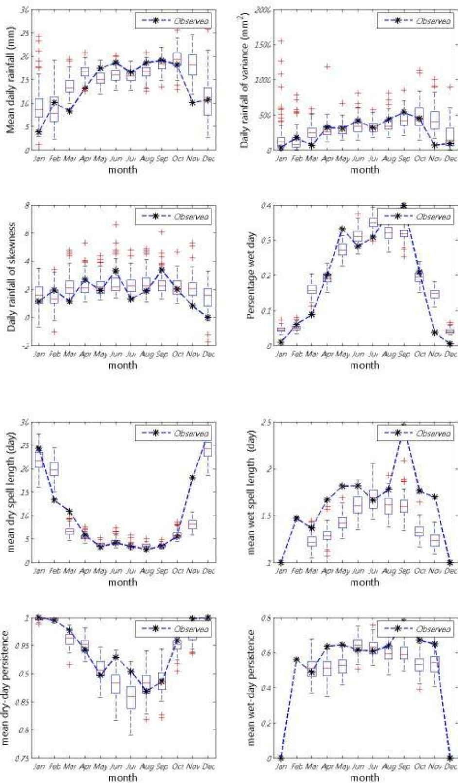
ภาพที่ ข.43 ค่าเฉลี่ย ความแปรปรวน สัมประสิทธิ์ความเบ้ เปอร์เซ็นต์ที่ฝนตก ช่วงเวลาที่ฝนหยุดและตก และจำนวนครั้งสัมผัสที่ฝนหยุดและตก ของข้อมูลฝนรายวันอดีตกับข้อมูลสังเคราะห์สำหรับสถานี 75052 (ปี ค.ศ. 1976-1990)
