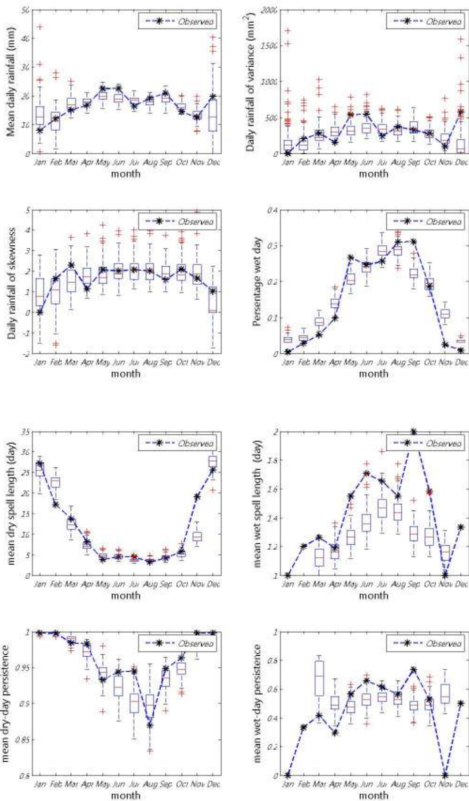
ภาพที่ ข.21 ค่าเฉลี่ย ความแปรปรวน สัมประสิทธิ์ความเบ้ เปอร์เซนต์ที่ฝนตก ช่วงเวลาที่ฝนหยุดและตก และจำนวนครั้งสัมผัสที่ฝนหยุดและตก ของข้อมูลฝนรายวันอดีตกับข้อมูลสังเคราะห์สำหรับสถานี 14062 (ปี ค.ศ. 1976-1990)
