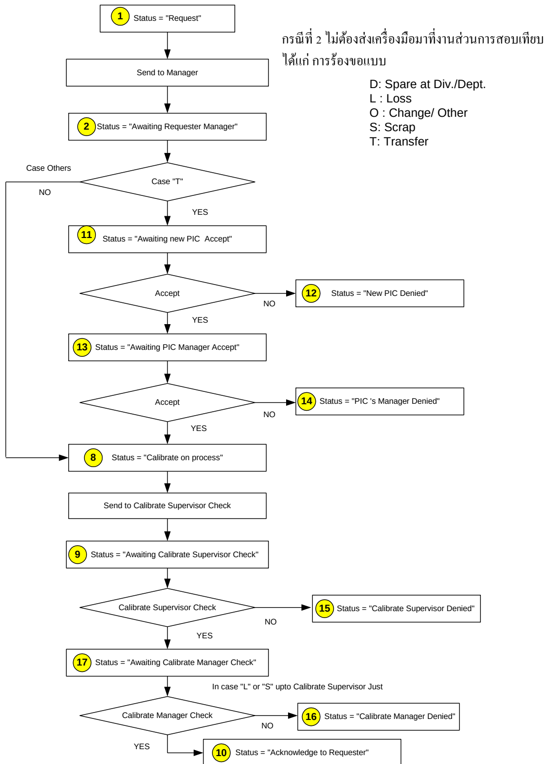
รูป 4.2 แสดงกระแสนงานของระบบใหม่กรณีไม่ต้องส่งเครื่องมือ
