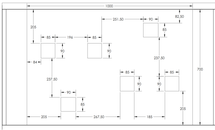
(ก) แสดงการออกแบบการวางแผงนิตรอน
