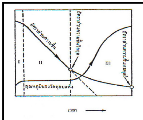
รูปที่ 2.9 เส้นลักษณะเฉพาะของการอบแห้ง
