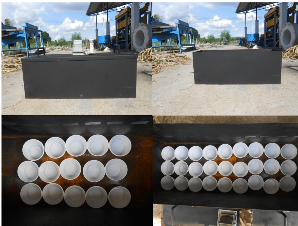
รูปที่ 4.4 การทดลองหาระยะการกระจายตัวของคลิ่นจากแมกนีตรอน 1 ตัว
