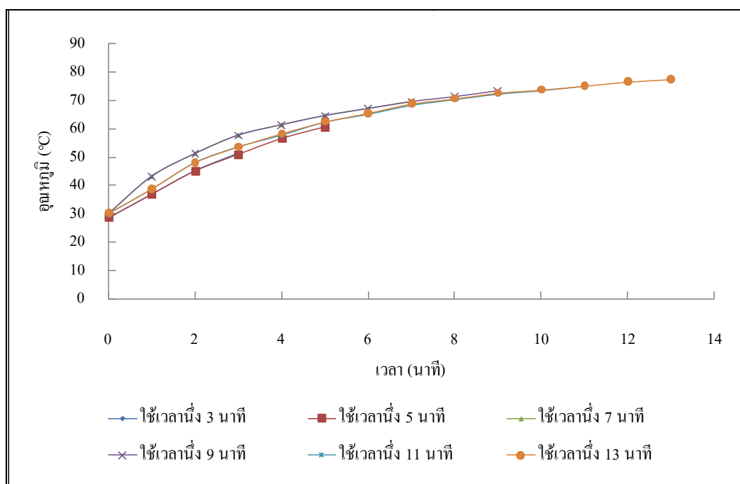
รูปที่ 4.49 การนึ่งปาล์มน้ำมันด้วยเตาอบไมโครเวฟแบบครัวเรือน
