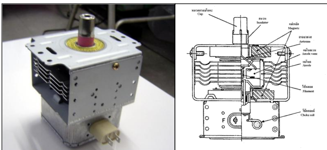
รูปที่ 2.1 แมกนีตรอน
