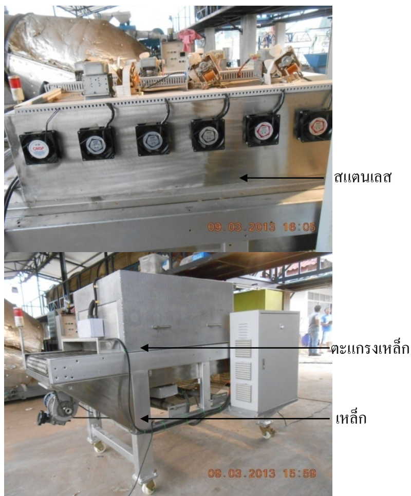
รูปที่ 4.15 ชนิดและวัสดุที่ใช้สร้างห้องอบไมโครเวฟร่วมกับลมร้อน
