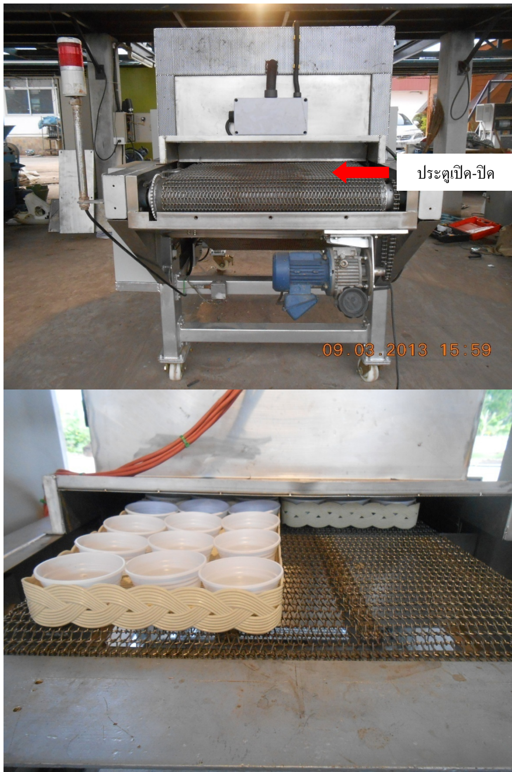
รูปที่ 4.12 แสดงลักษณะทางเข้า-ออก วัสดุดิบ
