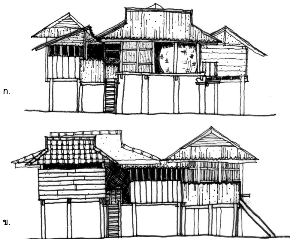
ภาพที่ 4.14 รูปด้านของเรือนไทดำ หลังที่ 5
