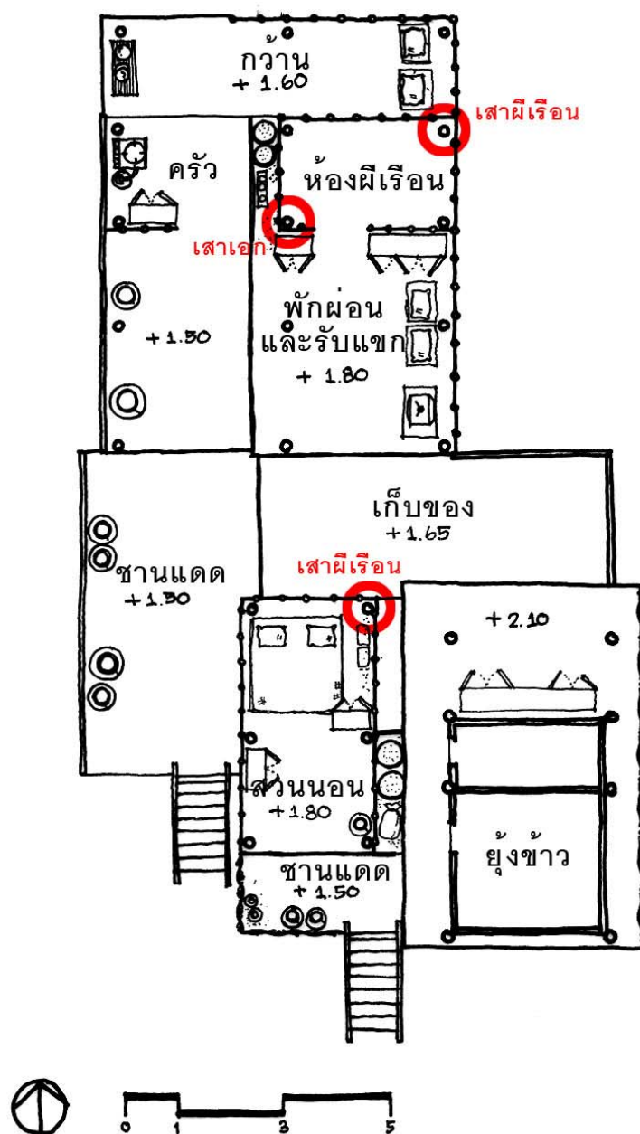
ภาพที่ 4.4 ผังพื้นเรือนไทดำ หลังที่ 2
