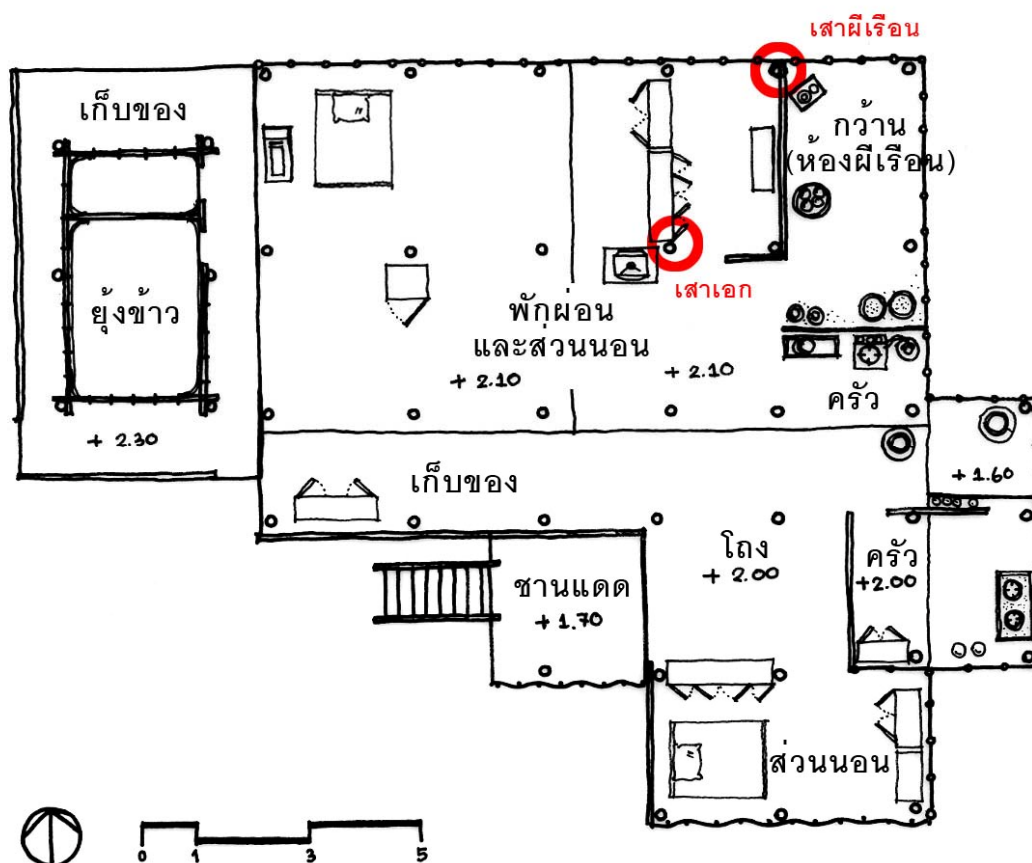
ผังพื้นเรือนไทดำ หลังที่ 3
