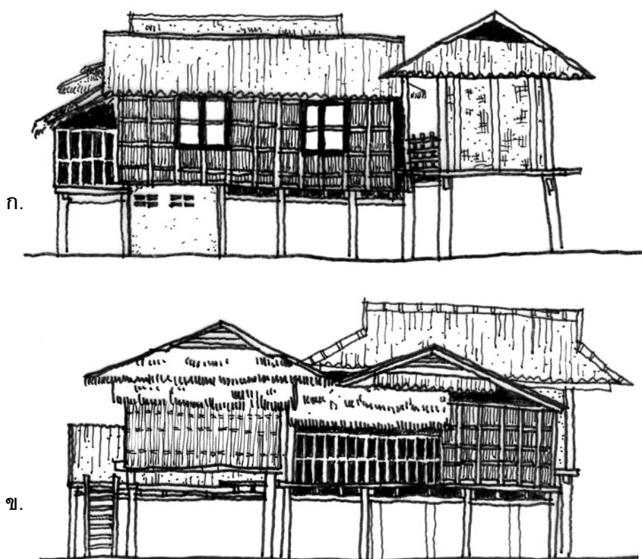
รูปด้านของเรือนไทดำ หลังที่ 4
