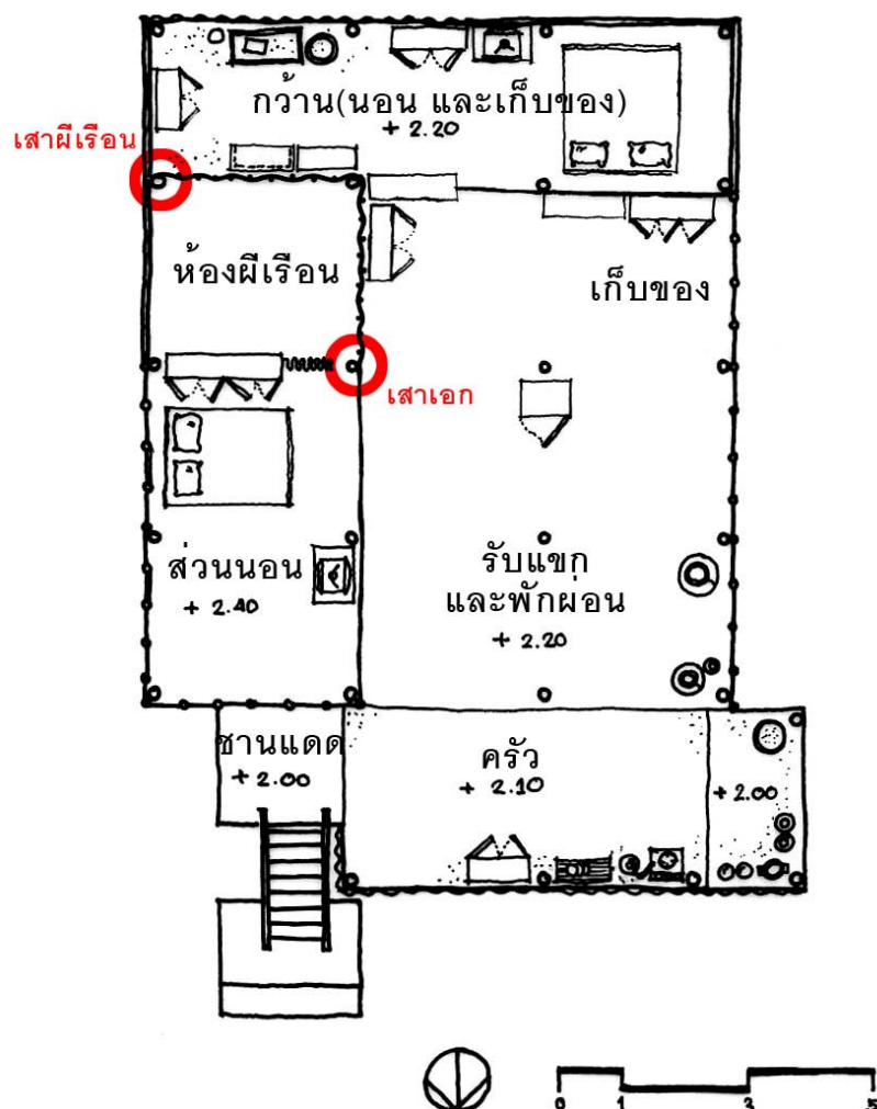
ภาพที่ 4.16 ผังพื้นเรือนไทดำ หลังที่ 6
