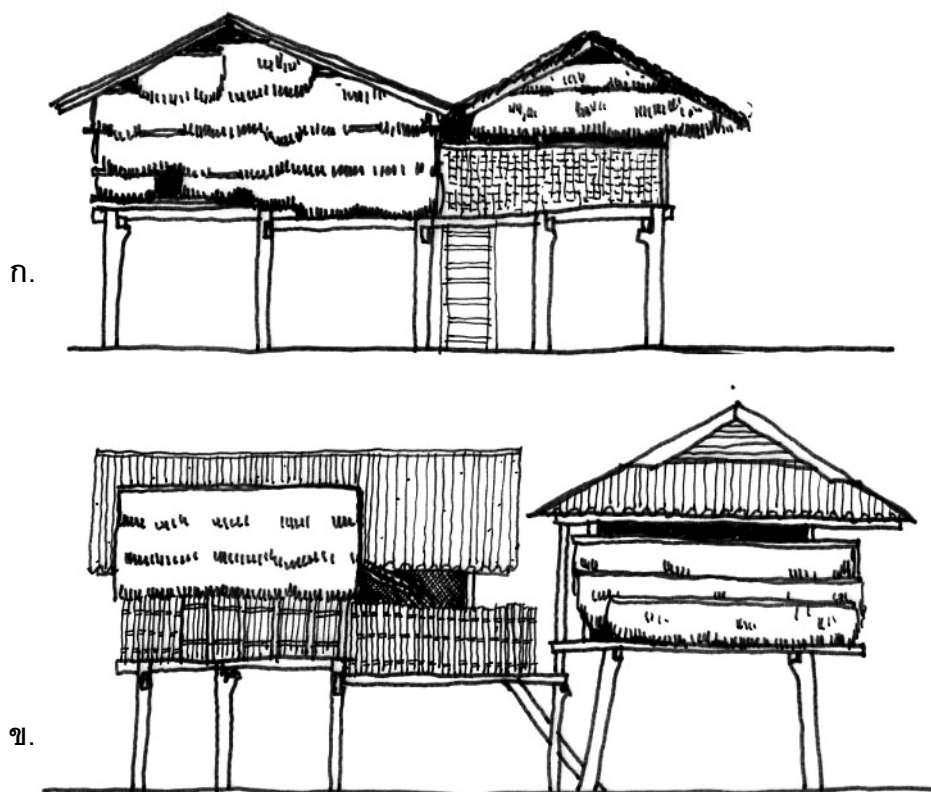
ภาพที่ 4.20 รูปด้านของเรือนไทดำ หลังที่ 7
