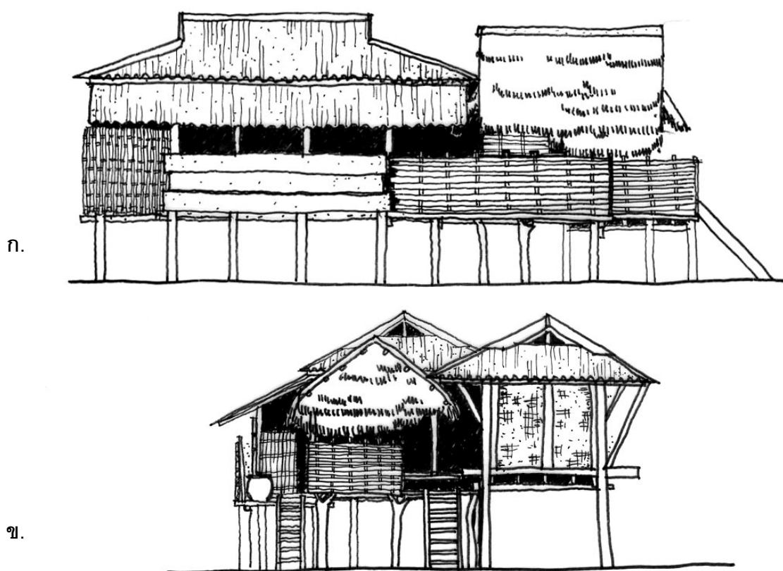
รูปด้านของเรือนไทดำ หลังที่ 2
