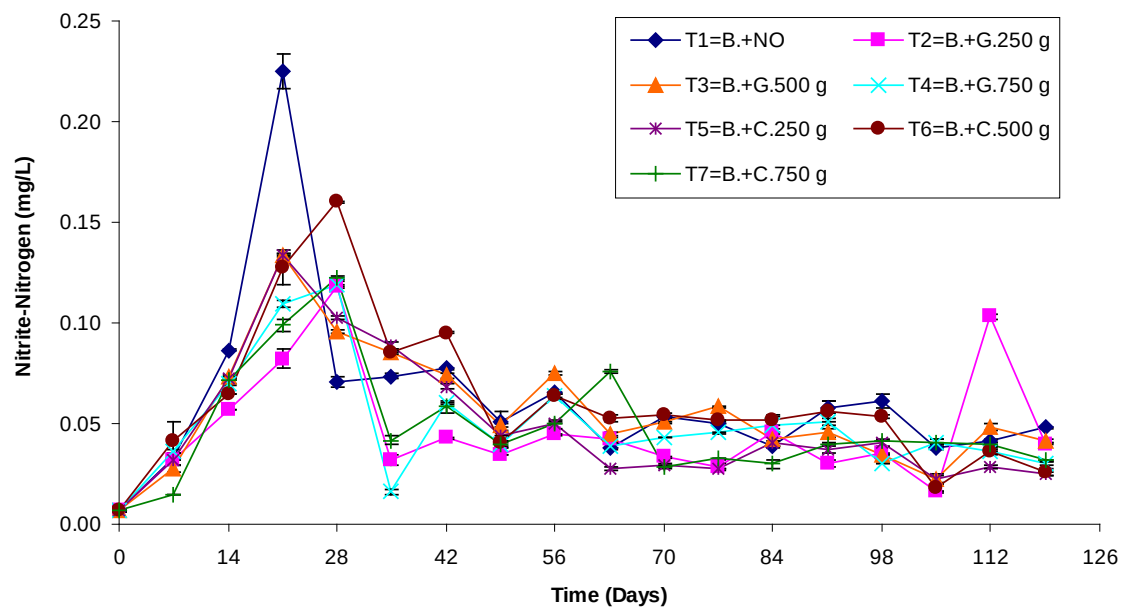
ภาพที่ 22 ปริมาณไนไตรท์-ไนโตรเจนเฉลี่ยในแต่ละชุดการทดลอง ตลอดระยะเวลา 4 เดือน
