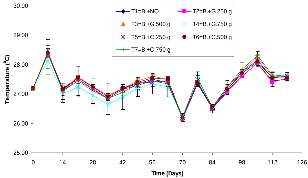
ภาพที่ 14 ค่าอุณหภูมิน้ำทะเลเฉลี่ย ณ เวลา 8.00 น. ในแต่ละชุดการทดลอง ตลอดระยะเวลา 4 เดือน
