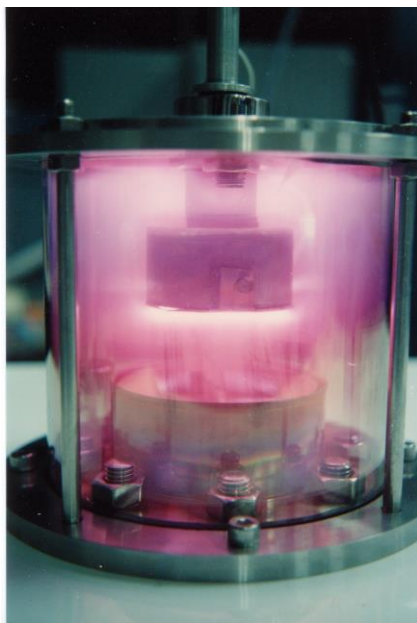
ภาพที่ 2-3 ระบบการเคลือบในสุญญากาศด้วยวิธีสปัตเตอริง
