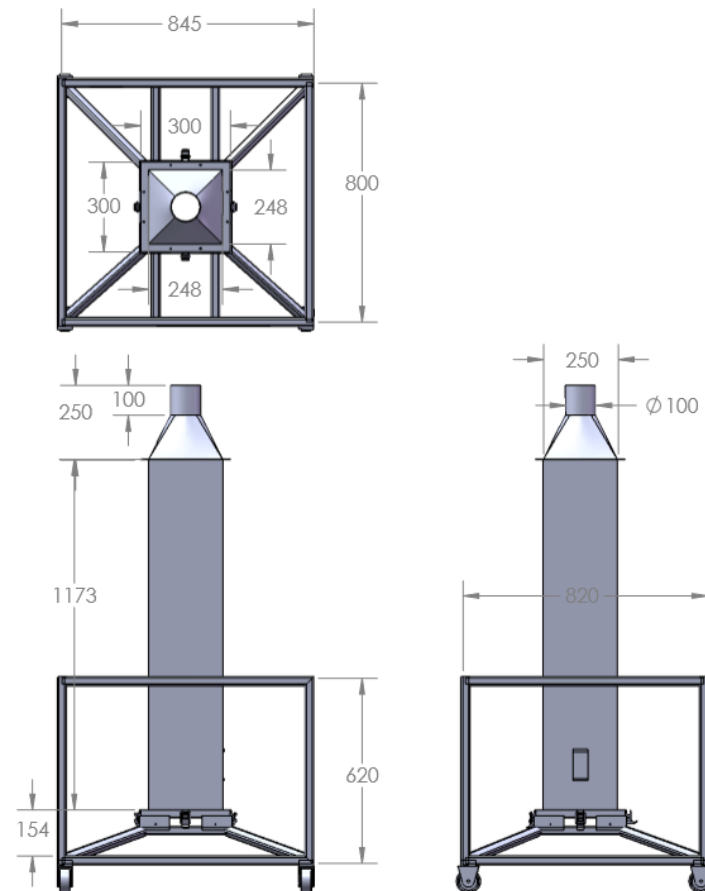
รูปที่ ก-2 เครื่องกำเนิดควัน
