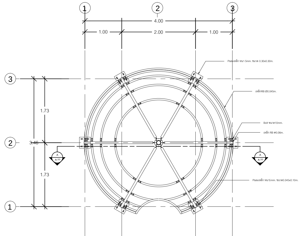
แปลนโครงสร้าง มาตราส่วน 1:50
