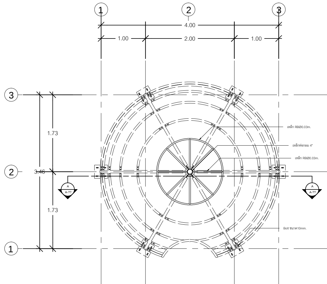
แปลนโครงสร้างหลังคา มาตราส่วน 1:50
