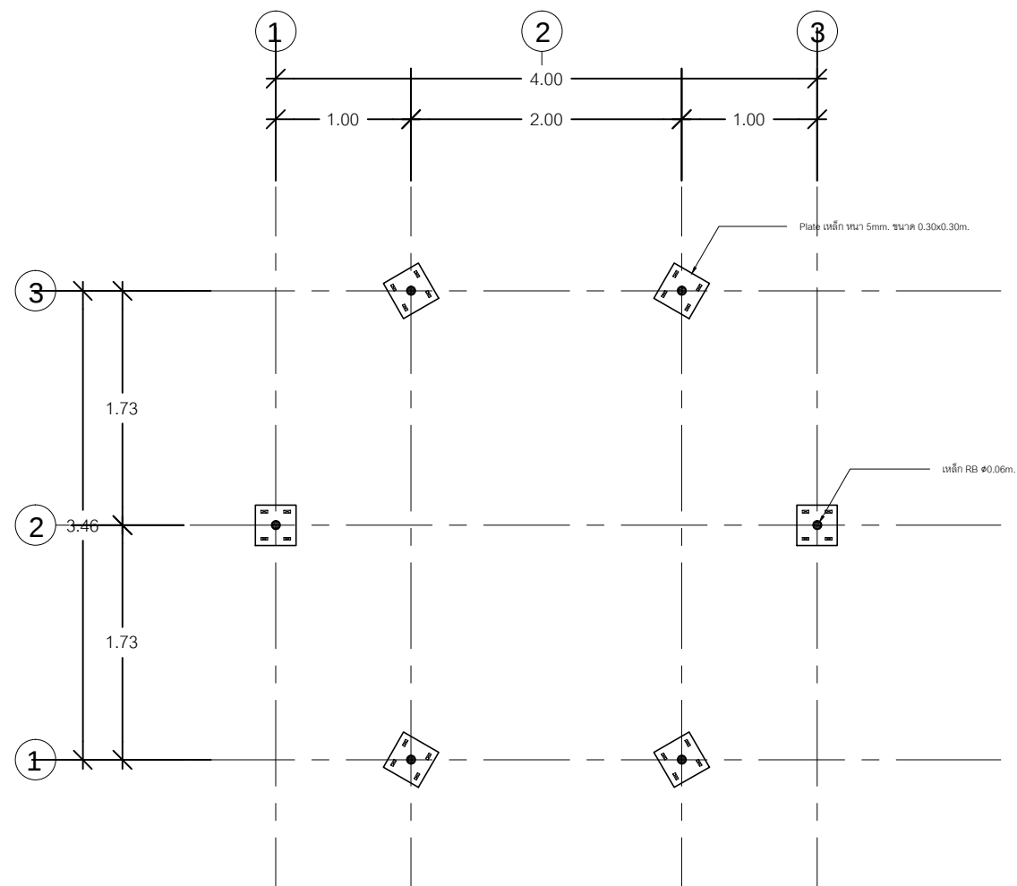
แปลนฐานโครงสร้าง มาตราส่วน 1:50
