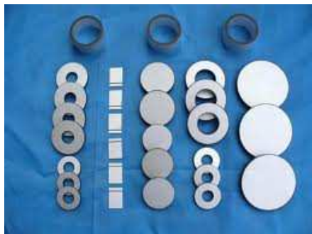
รูปที่ 1 แผ่นเพลตเซรามิกที่นำมาทำอัลตราโซนิคทรานสดิวเซอร์
