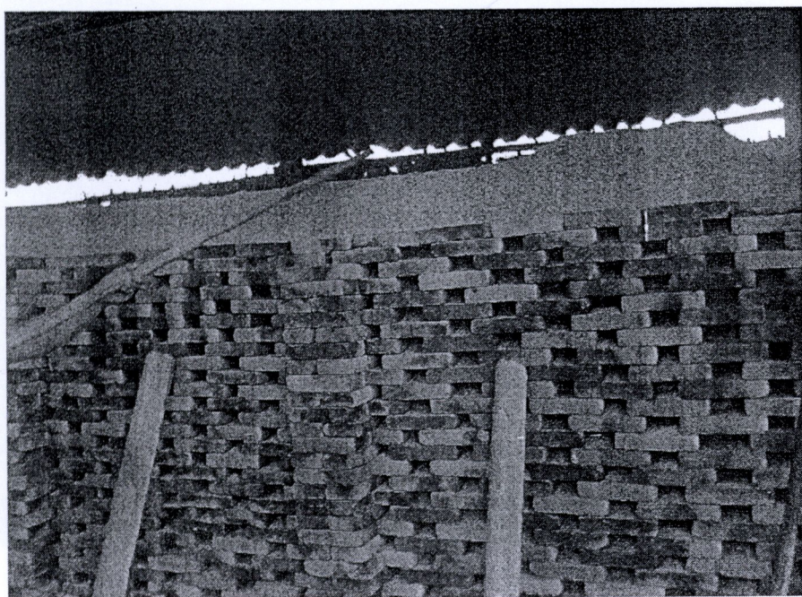
ภาพที่ 5 เตาเผาอิฐแบบเปิด โดยใช้เกลบเป็นเชื้อเพลิง
