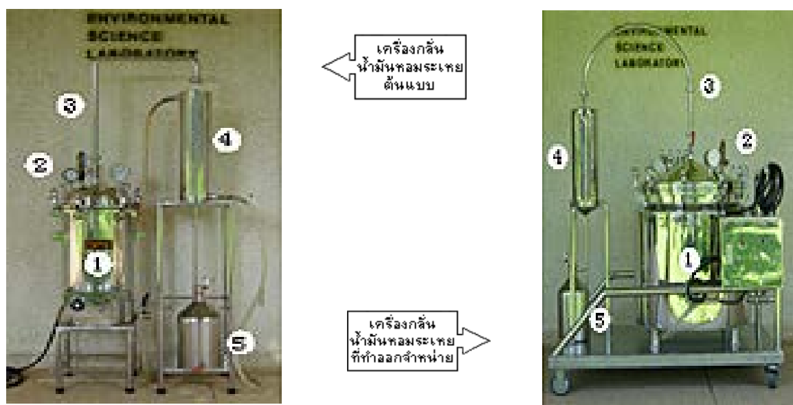
ภาพที่ 3 เครื่องกลั่นน้ำมันหอมระเหย
