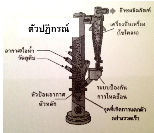
รูปที่ 2.11 เครื่องปฏิกรณ์แบบฟลูอิโดซ์แบบไหลเวียน (ปรับปรุงจาก http://www.jfe-rd.co.jp )
