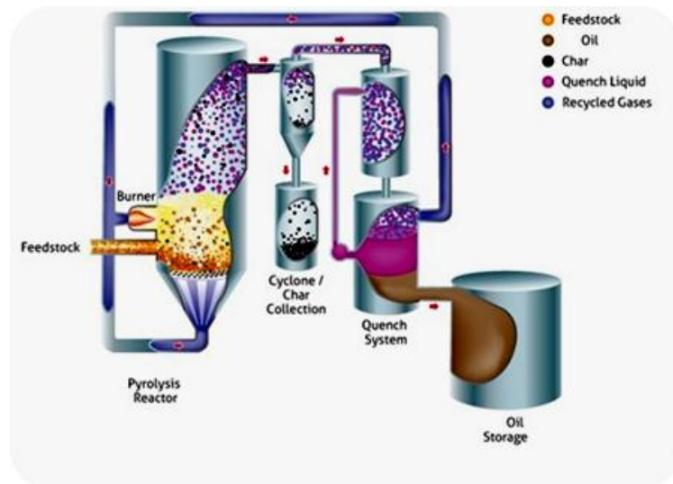
รูปที่ 2.5 กระบวนการไพโรไลซิส (ดัดแปลงจาก
