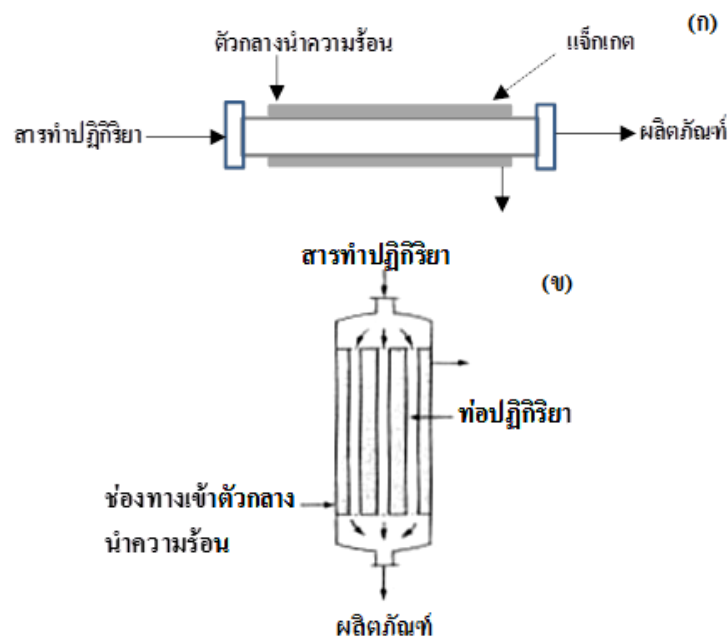
รูปที่ 2.9 เครื่องปฏิกรณ์แบบท่อไหล (ดัดแปลงจาก Bilgesü et al. , 2006)
