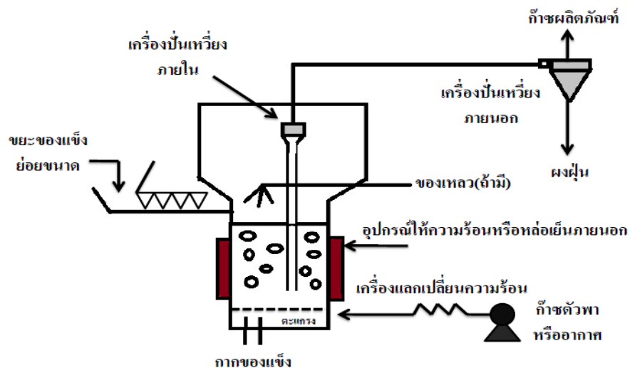
รูปที่ 2.10 เครื่องปฏิกรณ์แบบฟลูอิดไคซ์แบบพองก๊าซ (Yang, 1995)
