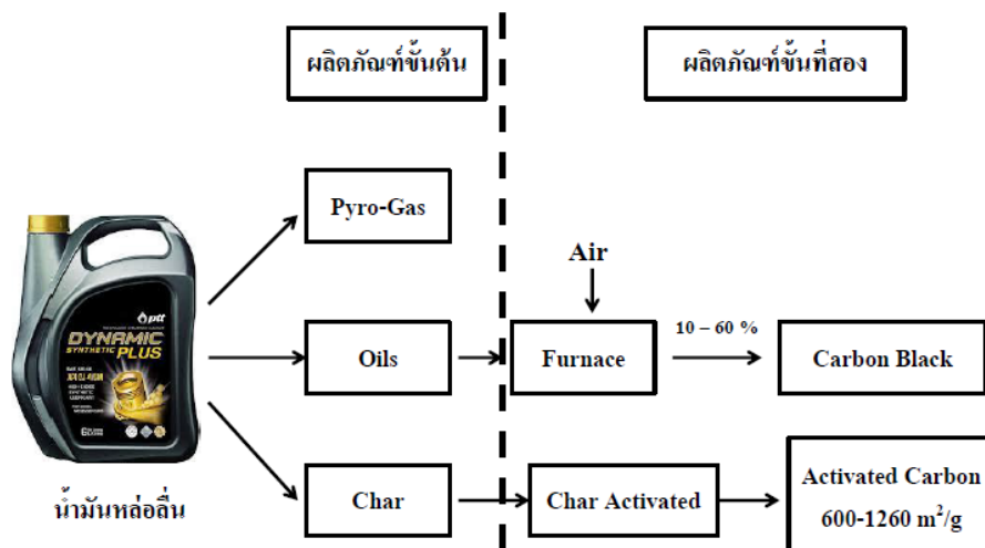
รูปที่ 2.6 ผลิตภัณฑ์ต่างๆที่เกิดจากการเปลี่ยนน้ำมันหล่อลื่นเป็นน้ำมันโดยกระบวนการไพโรไลซิส (ดัดแปลงจาก
