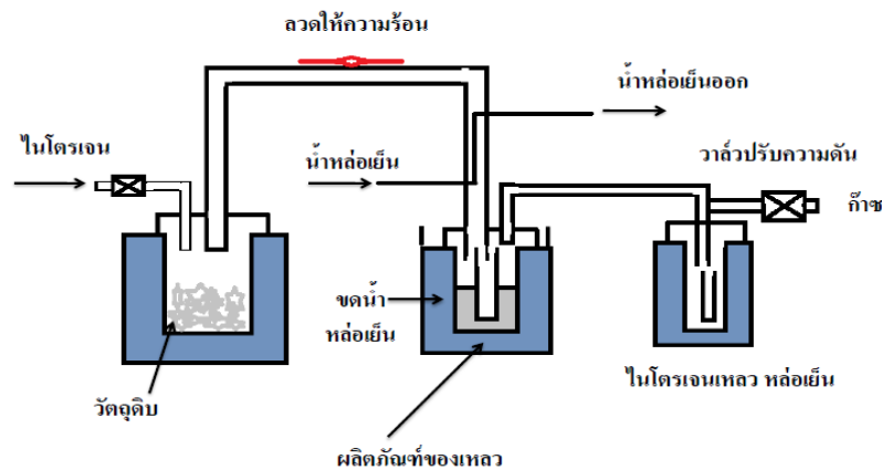
รูปที่ 2.7 เครื่องปฏิกรณ์แบบเบดคงที่แสดงในระบบแบบกึ่งต่อเนื่อง
