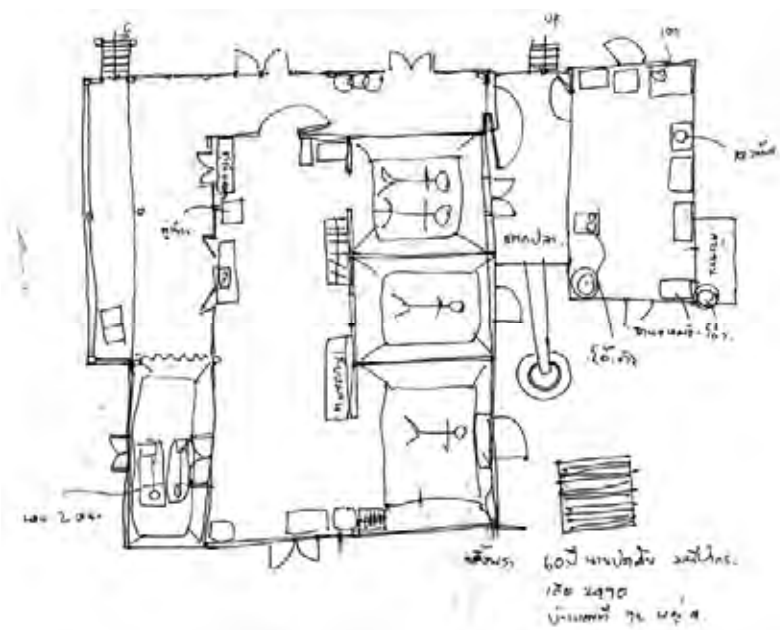
แผนผังที่ 15 ผังแสดงพื้นที่ใช้สอยชั้นบน
