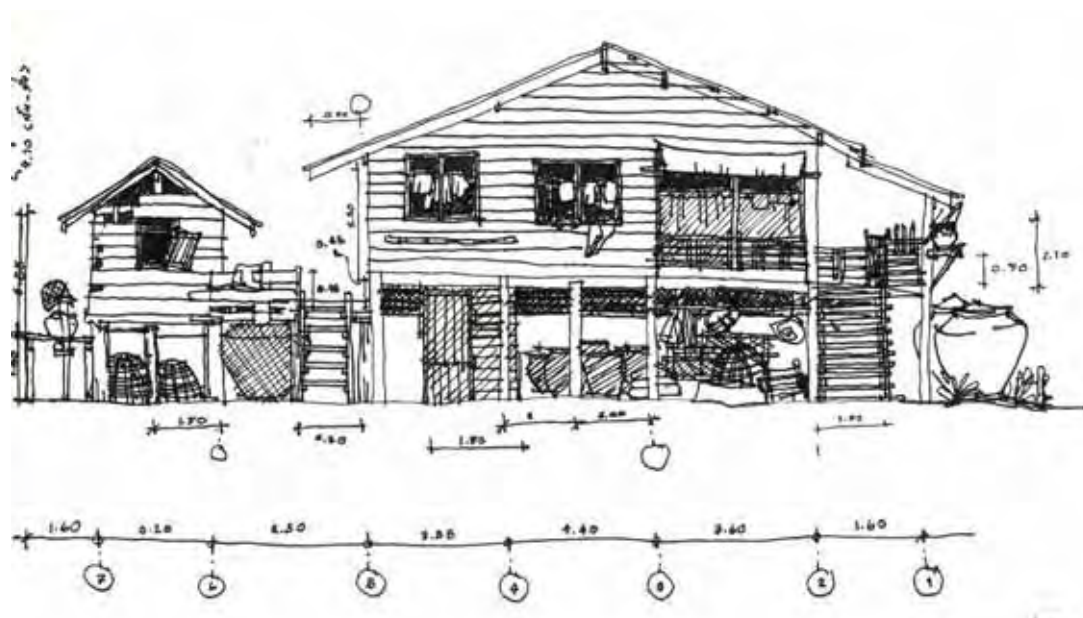
ลายเส้นที่ 6 รูปด้านทิศเหนือ
