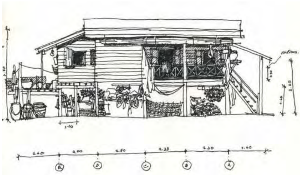
ลายเส้น 7 รูปด้านทิศตะวันตก
