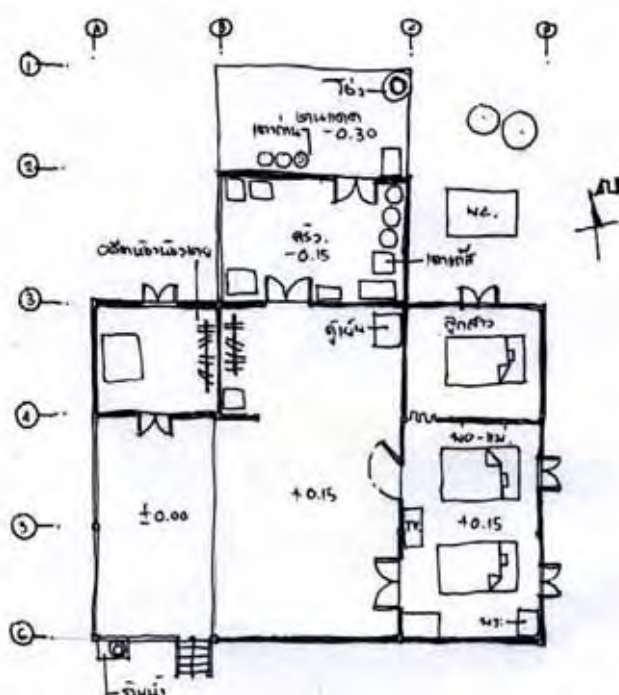
แผนผังที่ 17 ผังแสดงพื้นที่ใช้สอยชั้นบน
