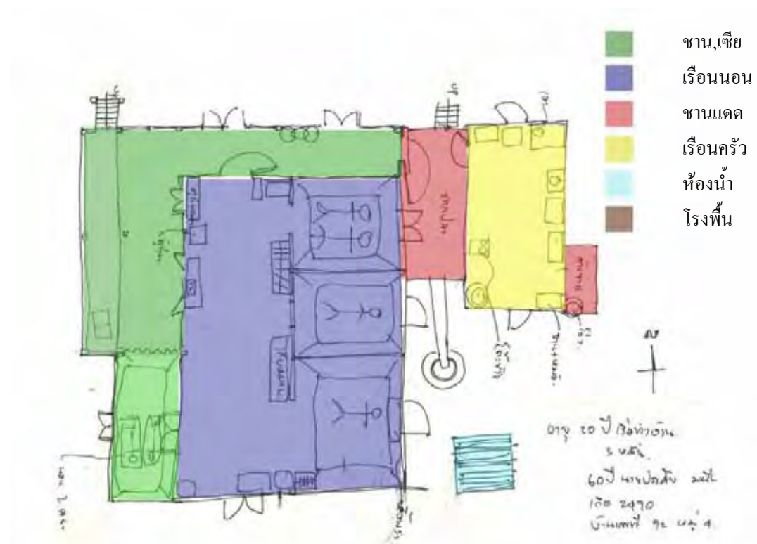
แผนผังที่ 31 แสดงพื้นที่ใช้สอยเรือนเลขที่ 92 บ้านท่าบ่อ
