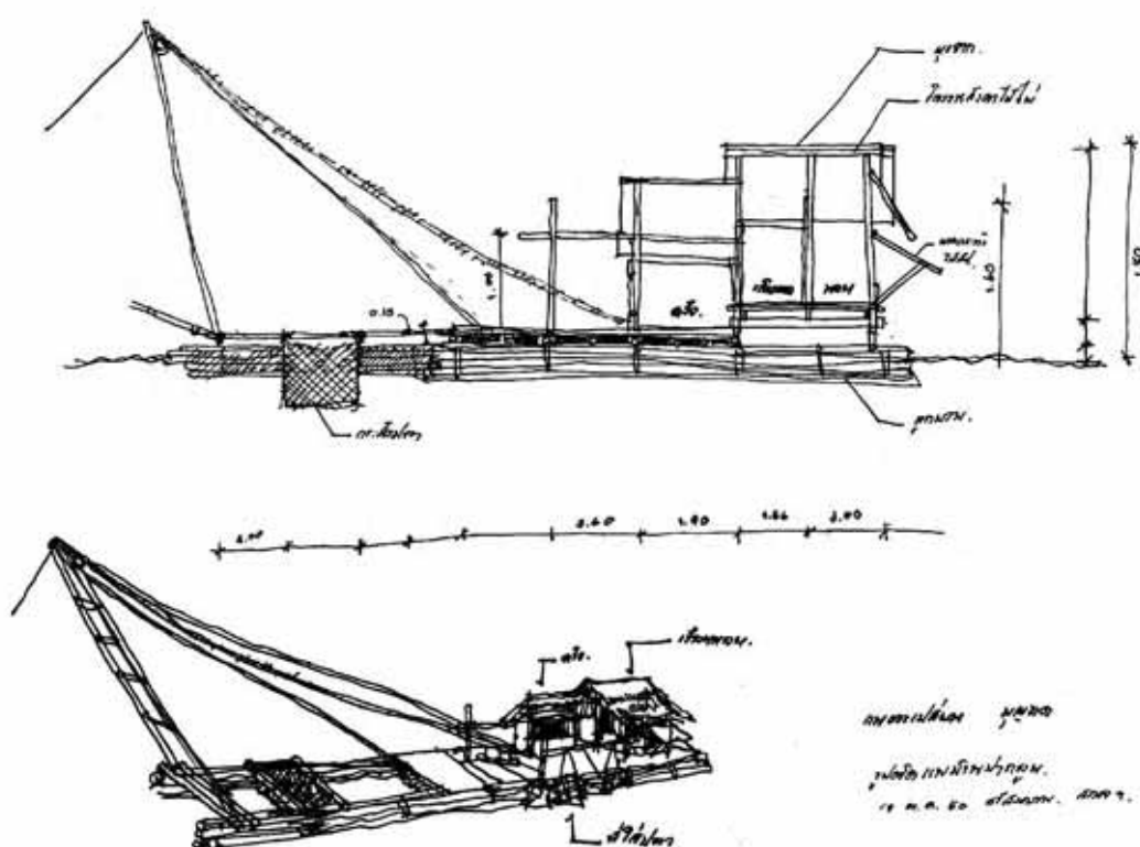
ลายเส้น 10 รูปตัดแสดงองค์ประกอบแพกระดุ้ง
