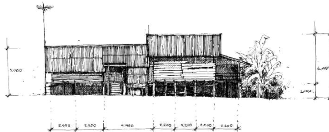
ลักษณะรูปด้าน หลังเรือน ด้านทิศเหนือ
