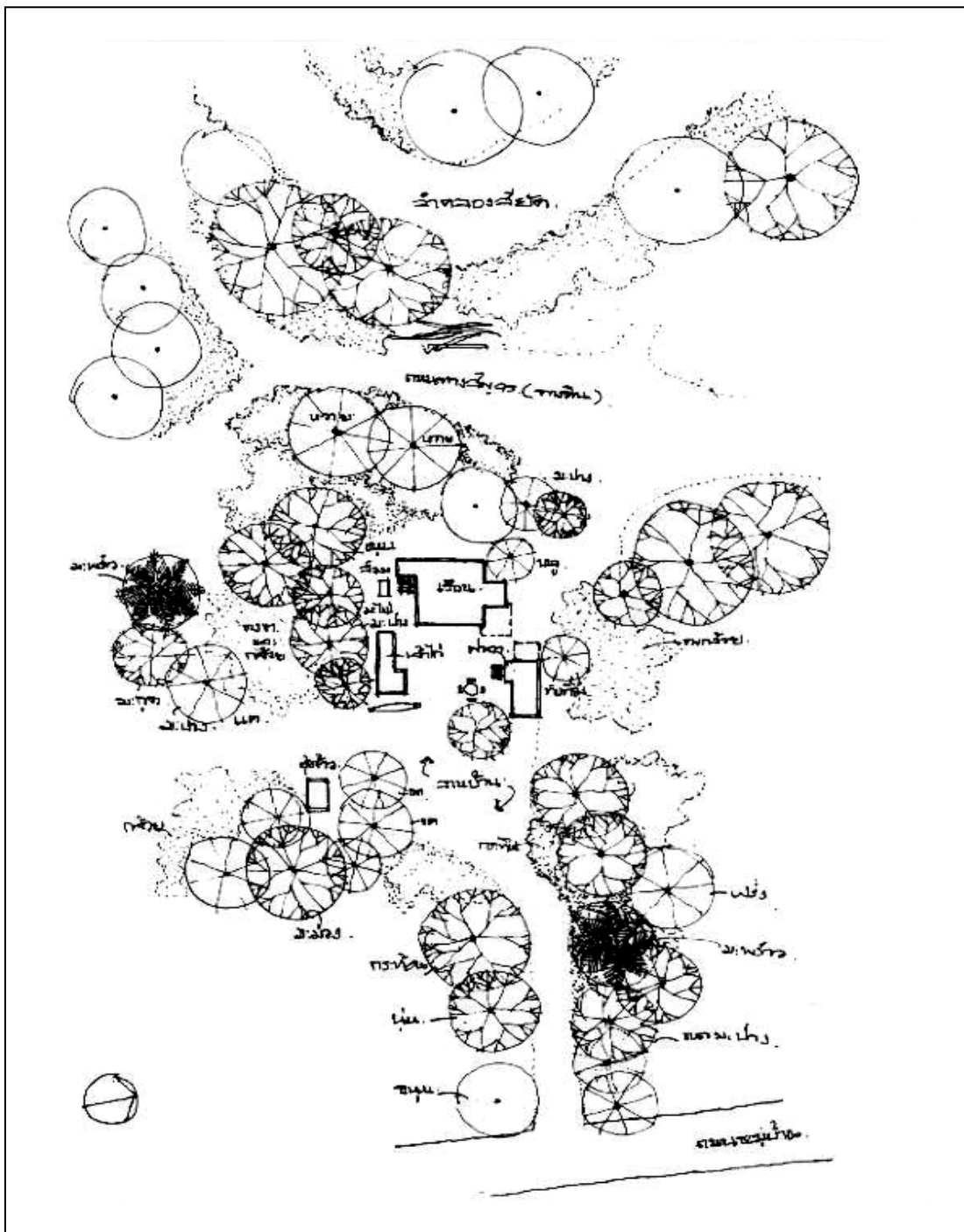
ลายเส้นที่ 19 แสดงการจัดวางผังบริเวณของเรือนคุณยายแดง นพเถา (จากการลงสำรวจภาคสนามในพื้นที่บ้านบางมะเฟือง อำเภอสนามชัยเขต จังหวัด ฉะเชิงเทรา, ตุลาคม 2550)
