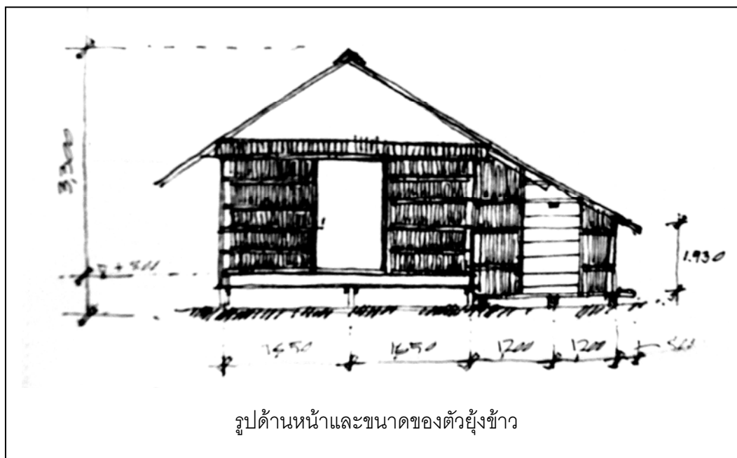
ลายเส้นที่ 22 แสดงรูปด้านและขนาดของซุงข้าว
