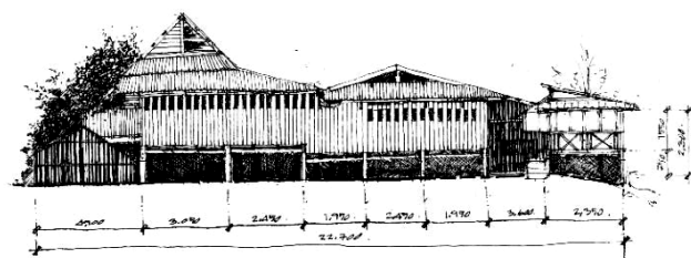
ลักษณะรูปด้าน หน้าเรือน ด้านทิศตะวันออก
