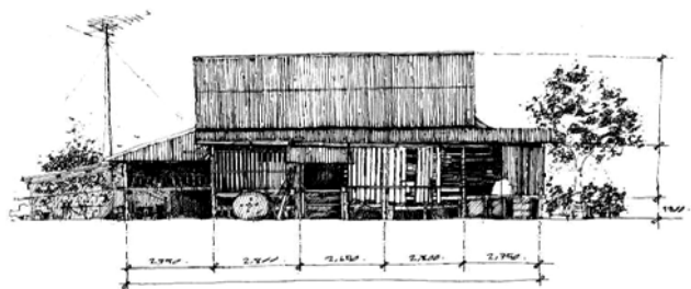
ลักษณะรูปด้าน หน้าเรือน ด้านทิศเหนือ
