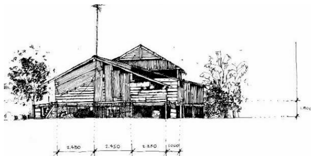
ลักษณะรูปด้าน ข้างเรือน ด้านทิศตะวันออก
