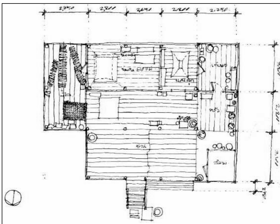
ลายเส้นที่ 51 แสดงลักษณะการจัดวางพื้นที่ใช้สอยภายในเรือน คุณพิศมหมาย สีสุพา (จากการลงสำรวจภาคสนามในพื้นที่บ้านบางมะเฟือง อำเภอสนมชัยเขต จังหวัด ฉะเชิงเทรา, กันยายน 2551)
