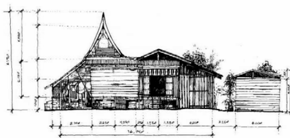
ลักษณะรูปด้าน หน้าเรือน ด้านทิศตะวันออก
