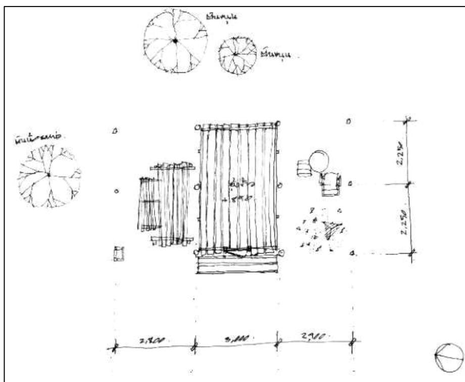
ลายเส้นที่ 34 แสดงลักษณะการจัดวางผังบริเวณของเรือนคุณลุงแฉล้ม แก้ววิจิตร
