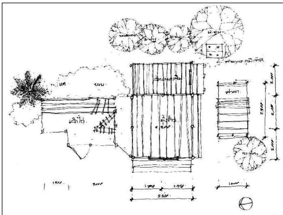
ลายเส้นที่ 28 แสดงผังยั้งข้าว (เล้าข้าว) ตัวยั้งหันหน้าไปทางทิศตะวันตก
