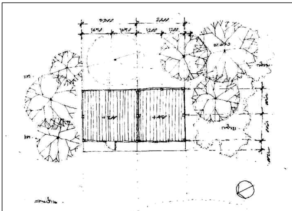
ลายเส้นที่ 20 แสดงการจัดวางผังยังข้าวซึ่งตัวยังหันหน้าไปทางทิศวันตกเฉียงเหนือ (จากการลงสำรวจภาคสนามในพื้นที่บ้านบางมะเฟือง อำเภอสนมชัยเขต จังหวัด ฉะเชิงเทรา, กันยายน 2550)
