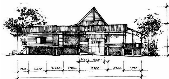
ลักษณะรูปด้าน ข้างเรือน ด้านทิศตะวันตก
