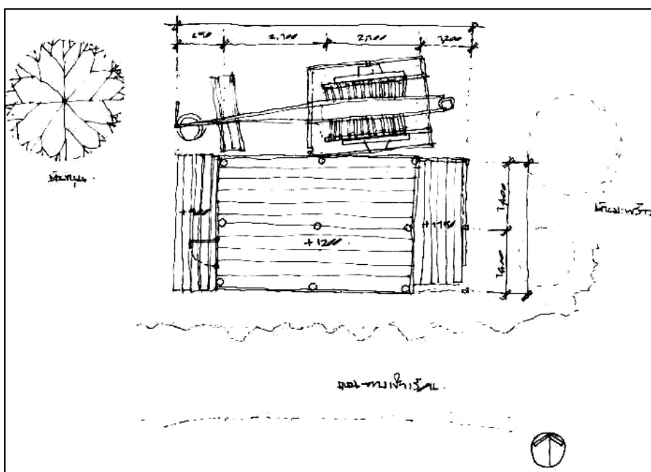
ลายเส้นที่ 55 แสดงลักษณะการจัดวางผังยังข้าวเรือน คุณลุงเรื่อง สุริยา
