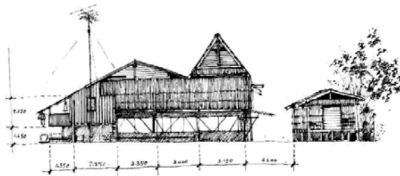
ลักษณะรูปด้าน ข้างเรือน ด้านทิศตะวันออก
