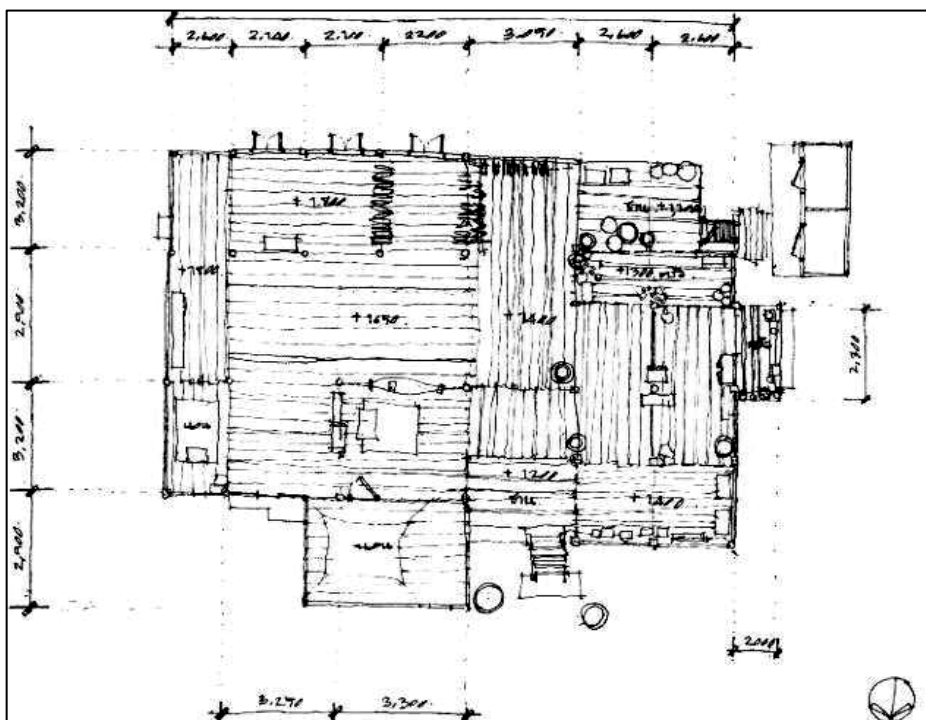
ลายเส้นที่ 36 แสดงลักษณะการจัดวางพื้นที่ใช้สอยของผังเรือนคุณลุงแชร่ม แก้ววิจิตร (จากการลงสำรวจภาคสนามในพื้นที่บ้านบางมะเฟือง อำเภอสนมชัยเขต จังหวัดฉะเชิงเทรา, กรกฎาคม 2551)
