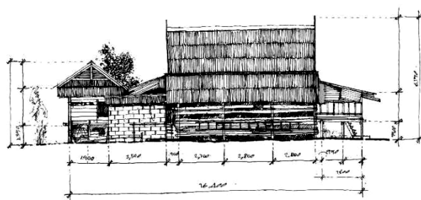
ลักษณะรูปด้าน ข้างเรือน ด้านทิศใต้
