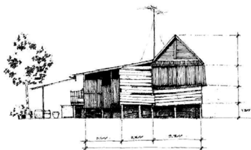
ลักษณะรูปด้าน ข้างเรือน ด้านทิศตะวันออก
