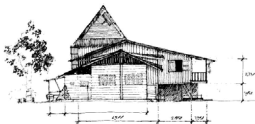
ลักษณะรูปด้าน ข้างเรือน ด้านทิศตะวันตก
