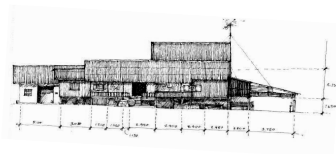
ลักษณะรูปด้าน หน้าเรือน ด้านทิศใต้
