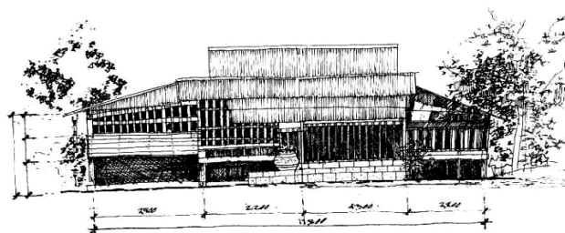
ลักษณะรูปด้าน ข้างเรือน ด้านทิศเหนือ
