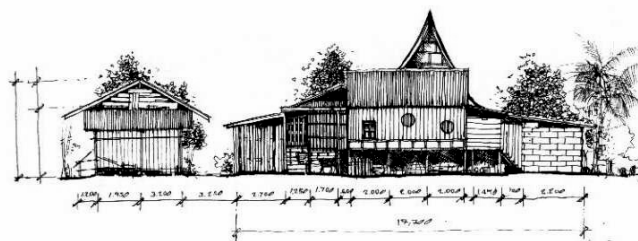
ลักษณะรูปด้าน หลังเรือน ด้านทิศตะวันตก
