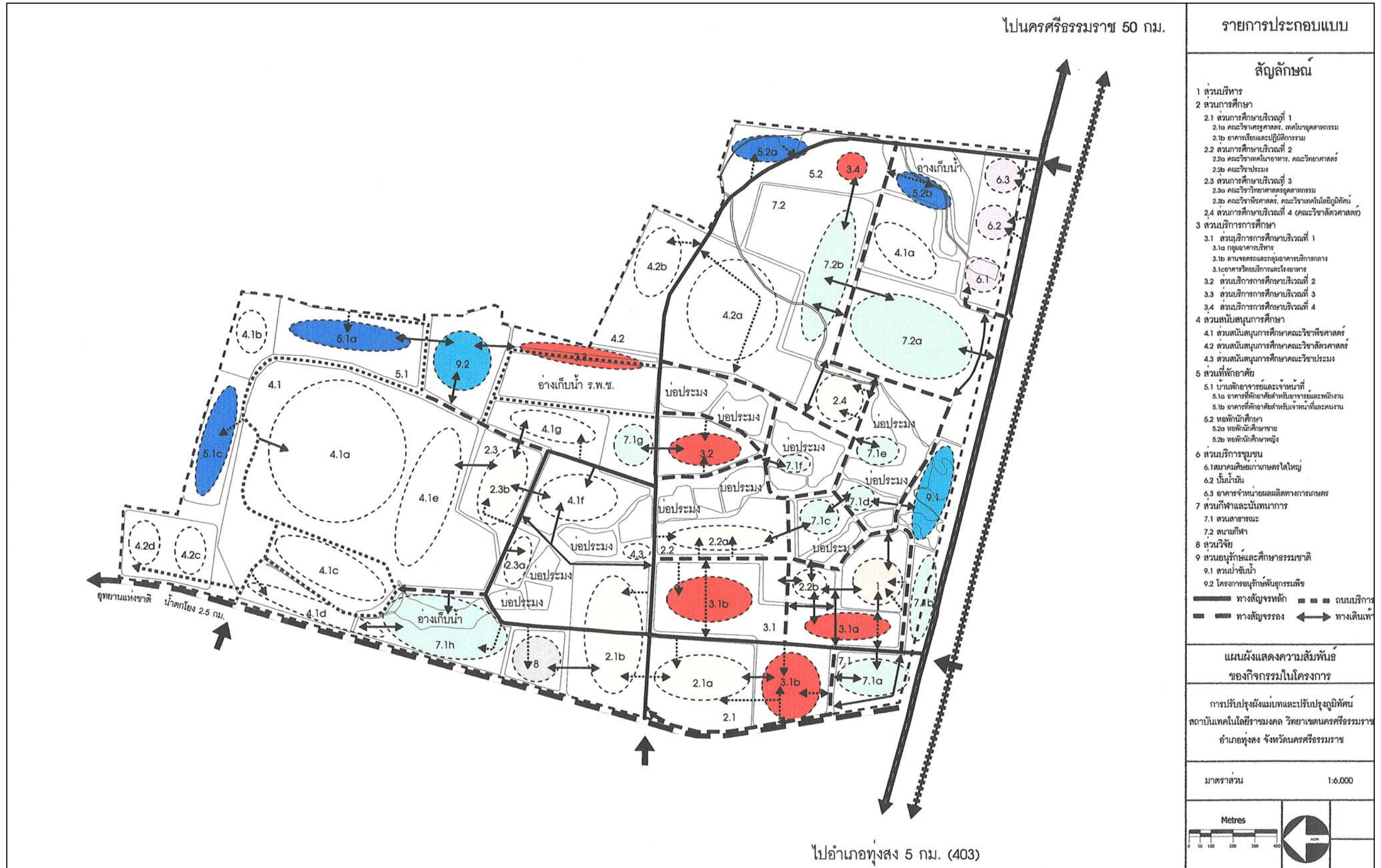
ภาพที่ 99 ผังแสดงความสัมพันธ์ในรูปแบบแผนภาพวงกลม (Balloon diagram)
