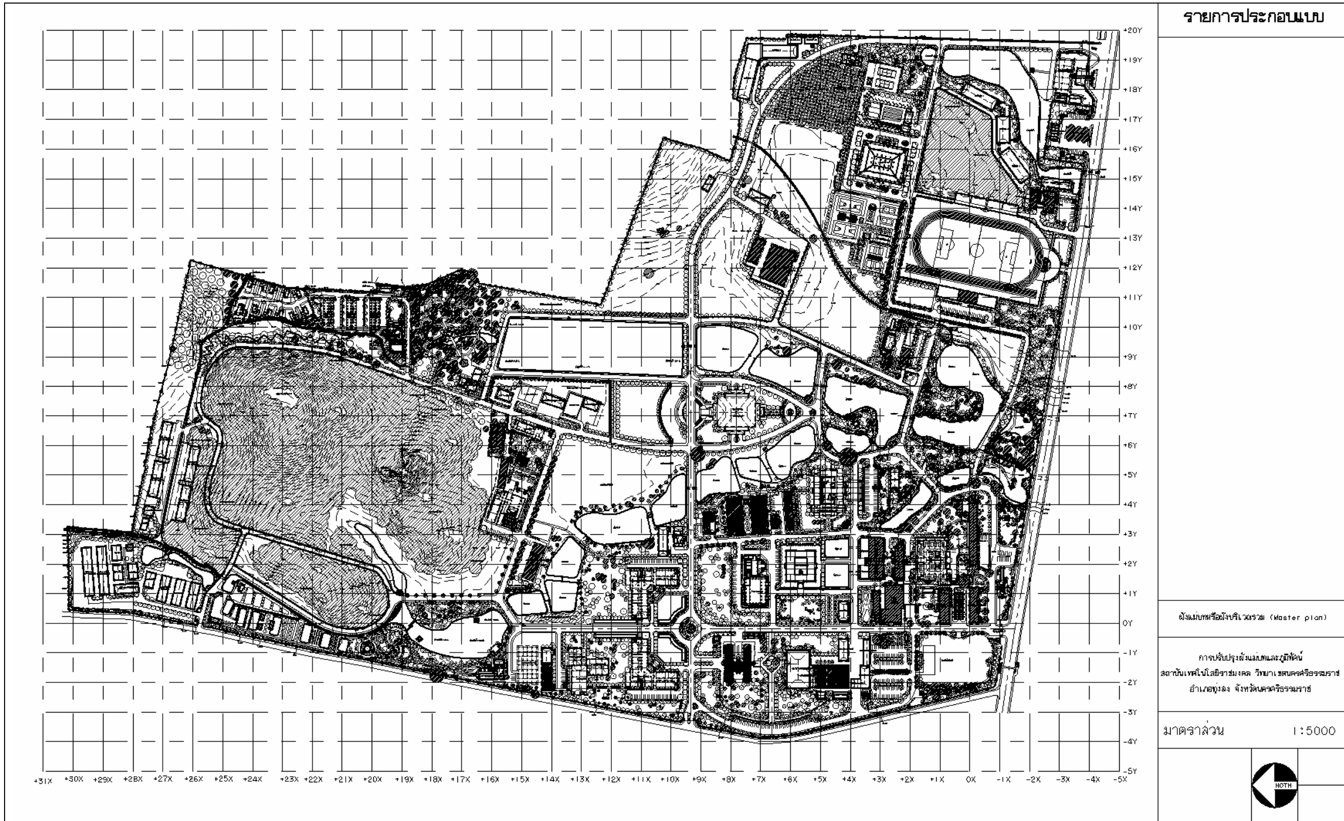
ภาพที่ 104 ผังแสดงผังแม่บทหรือผังบริเวณรวม (Master plan)
