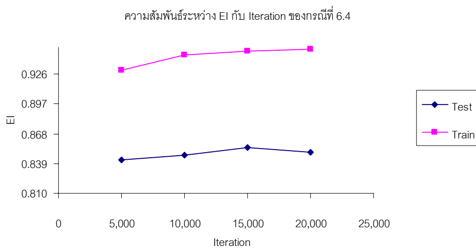
ภาพที่ 66 การเปรียบเทียบค่าประสิทธิภาพของโครงข่ายประสาทเทียมเมื่อทำการเปลี่ยนจำนวนรอบที่ใช้ในกระบวนการเรียนรู้ (ลำนํ้ายม)
