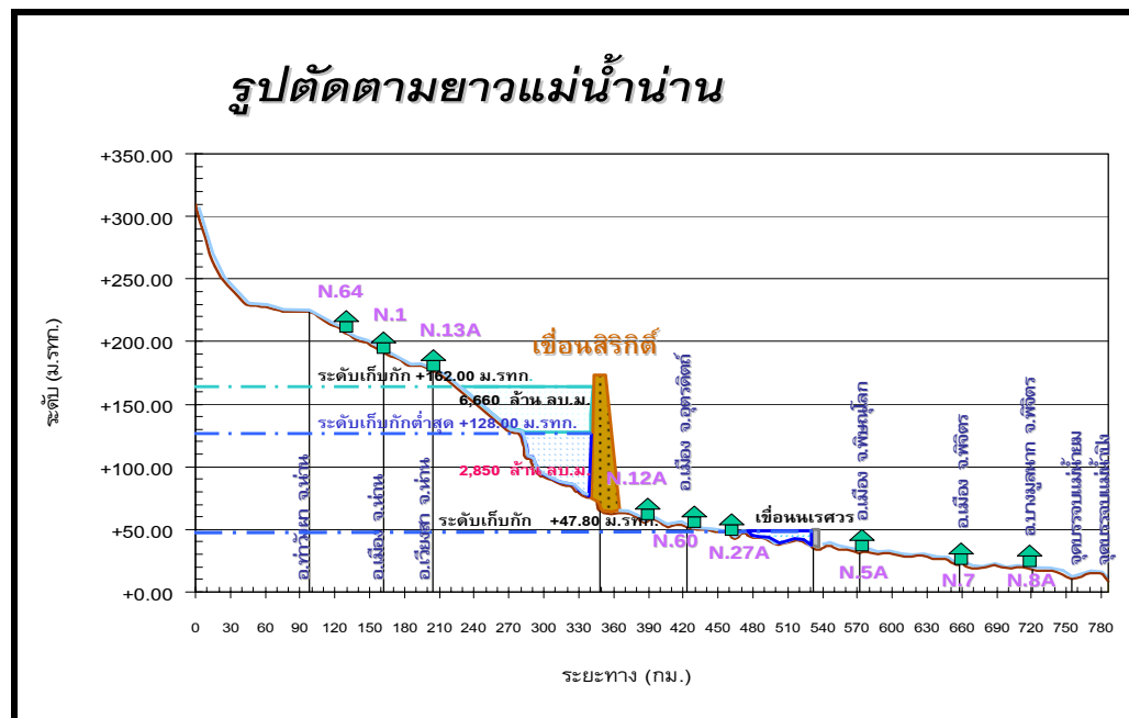
ภาพที่ 25 รูปตัดตามยาวแม่น้ำน่าน
