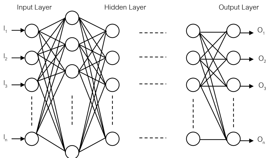
ภาพที่ 16 โครงสร้างของโครงข่ายประสาทเทียมแบบ Backpropagation
