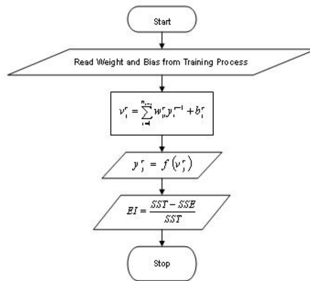
ภาพที่ 39 ขั้นตอนกระบวนการทดสอบของโปรแกรม KUnet (Training Procedure in KUnet Program)
