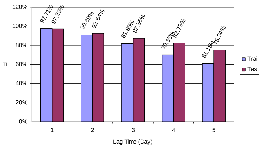
ภาพที่ 67 ประสิทธิภาพของโครงข่ายประสาทเทียม ณ วันพยากรณ์ (Lag Time) ต่างๆ (ล้านน้ำยม)
