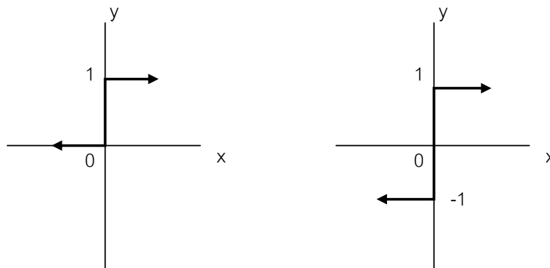
ภาพที่ 5 Threshold Logic Function
