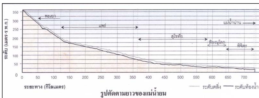
ภาพที่ 19 แสดงรูปตัดตามยาวของแม่น้ำยม
