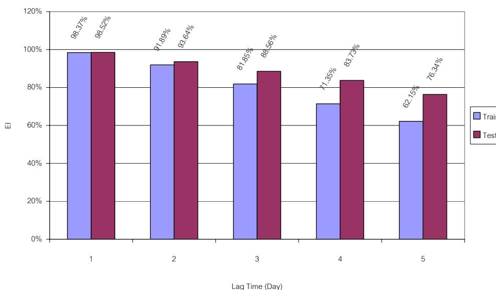
ภาพที่ 80 ประสิทธิภาพของโครงข่ายประสาทเทียม ณ วันพยากรณ์ (Lag Time) ต่างๆ (ลำน้ำน่าน)
