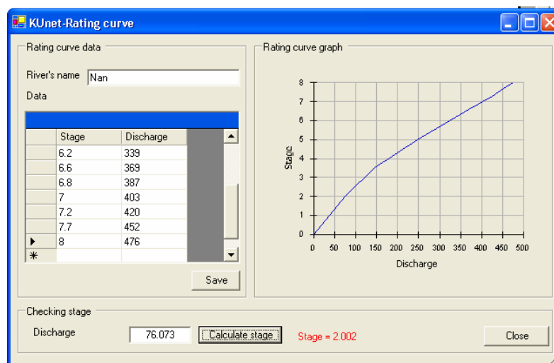
ภาพที่ 52 หน้าจอที่ใช้ในการแปลงอัตราการไหลให้เป็นระดับน้ำ
