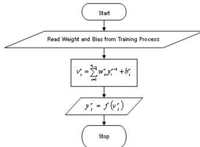
ภาพที่ 40 ขั้นตอนกระบวนการพยากรณ์ของโปรแกรม KUnet (Training Procedure in KUnet Program)
