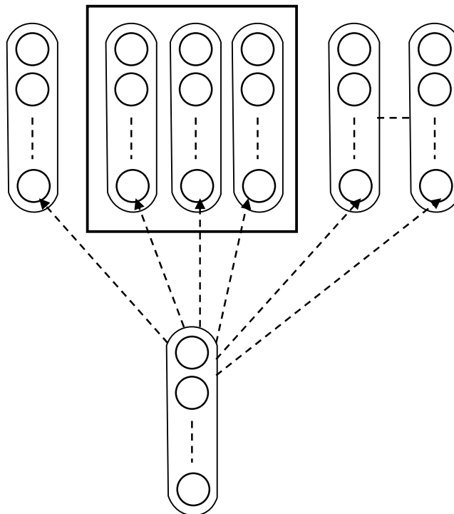
ภาพที่ 12 Single Layer, Topologically Ordered Networks
