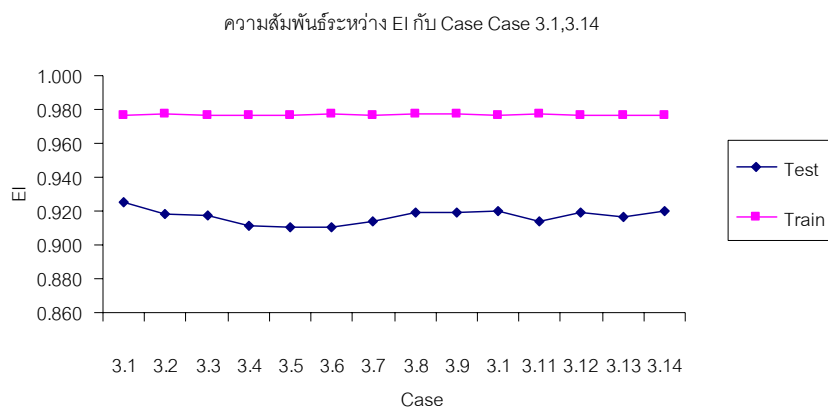
ภาพที่ 69 การเปรียบเทียบค่าประสิทธิภาพของโครงข่ายประสาทเทียม เมื่อทำการเปลี่ยนจำนวนหน่วยในชั้นแฝง (ลำนำนาน)
