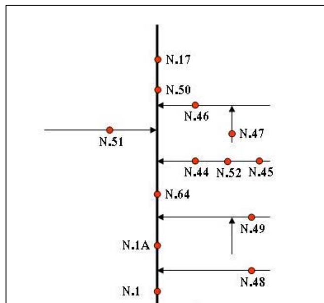
ภาพที่ 30 แผนผังสถานีวัดน้ำท่า ลำน้ำน่าน
