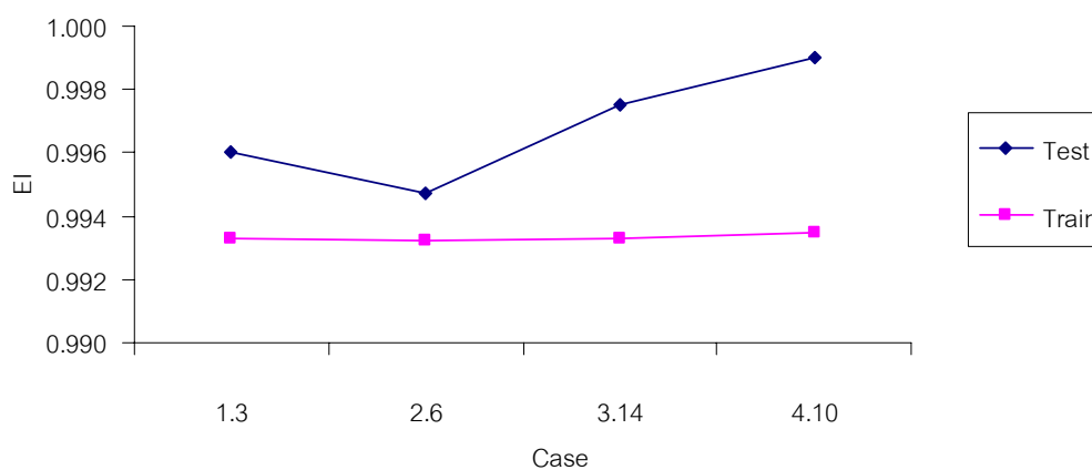
ภาพที่ 70 การเปรียบเทียบโครงข่ายประสาทเทียมที่ให้ค่าประสิทธิภาพสูงที่สุดของกรณีศึกษา ก (ถ่านน้ำมัน)
