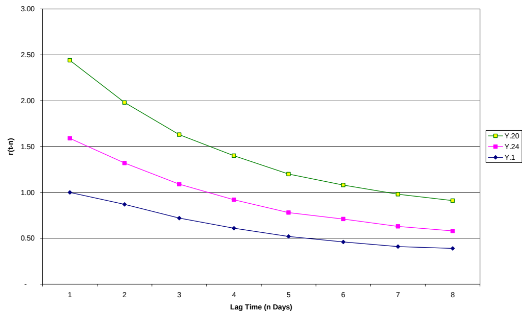
ภาพที่ 35 กราฟแสดงค่าสัมประสิทธิ์สหสัมพันธ์ของสถานีวัดน้ำในพื้นที่ลุ่มน้ำยมที่มีอิทธิพลต่อสถานี Y.1 ในวันย้อนหลัง (Lag Time) ต่างๆ
