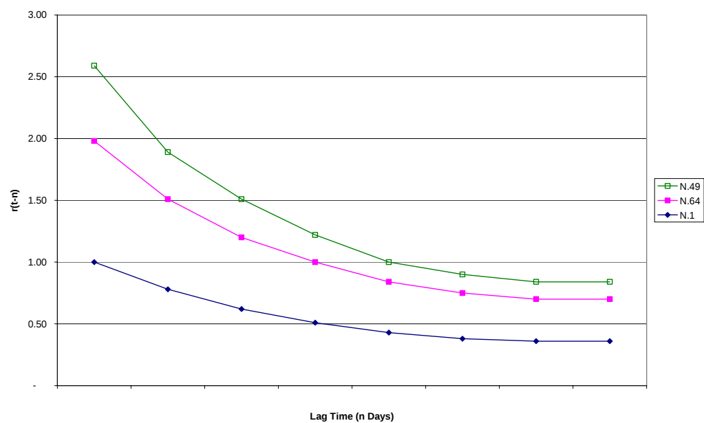
ภาพที่ 36 กราฟแสดงค่าสัมประสิทธิ์สหสัมพันธ์ของสถานีวัดน้ำในพื้นที่ลุ่มน้ำน่านที่มีอิทธิพลต่อสถานี N.1 ในวันย้อนหลัง (Lag Time) ต่างๆ
