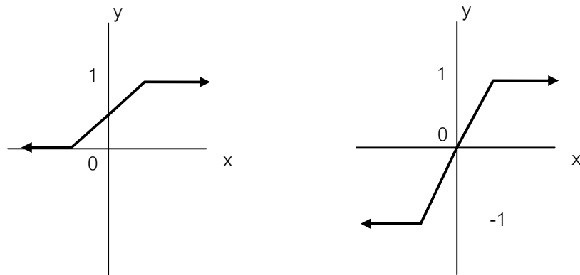
ภาพที่ 6 Hard Limit Function
