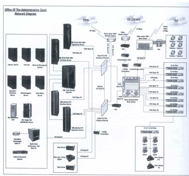
แผนภาพที่ ๓ ผังคอมพิวเตอร์และเครือข่ายภายในส่วนกลาง
