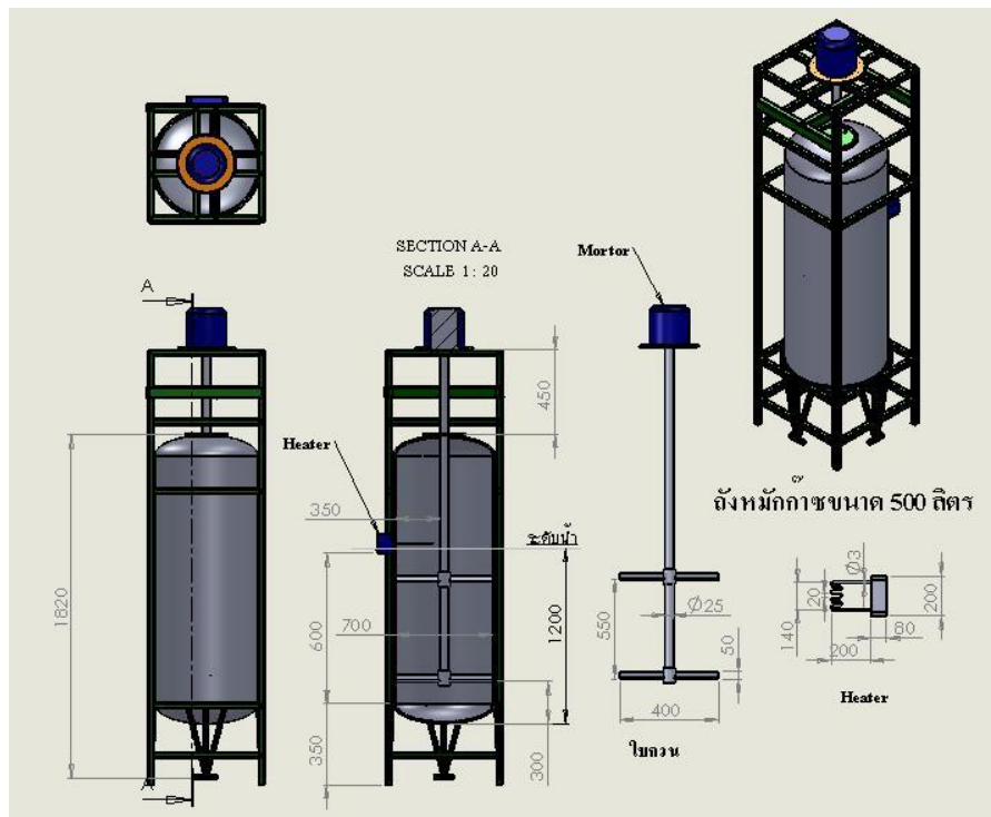
รูปที่ ก. 1 – 5 แบบที่ใช้ดำเนินการสร้าง
