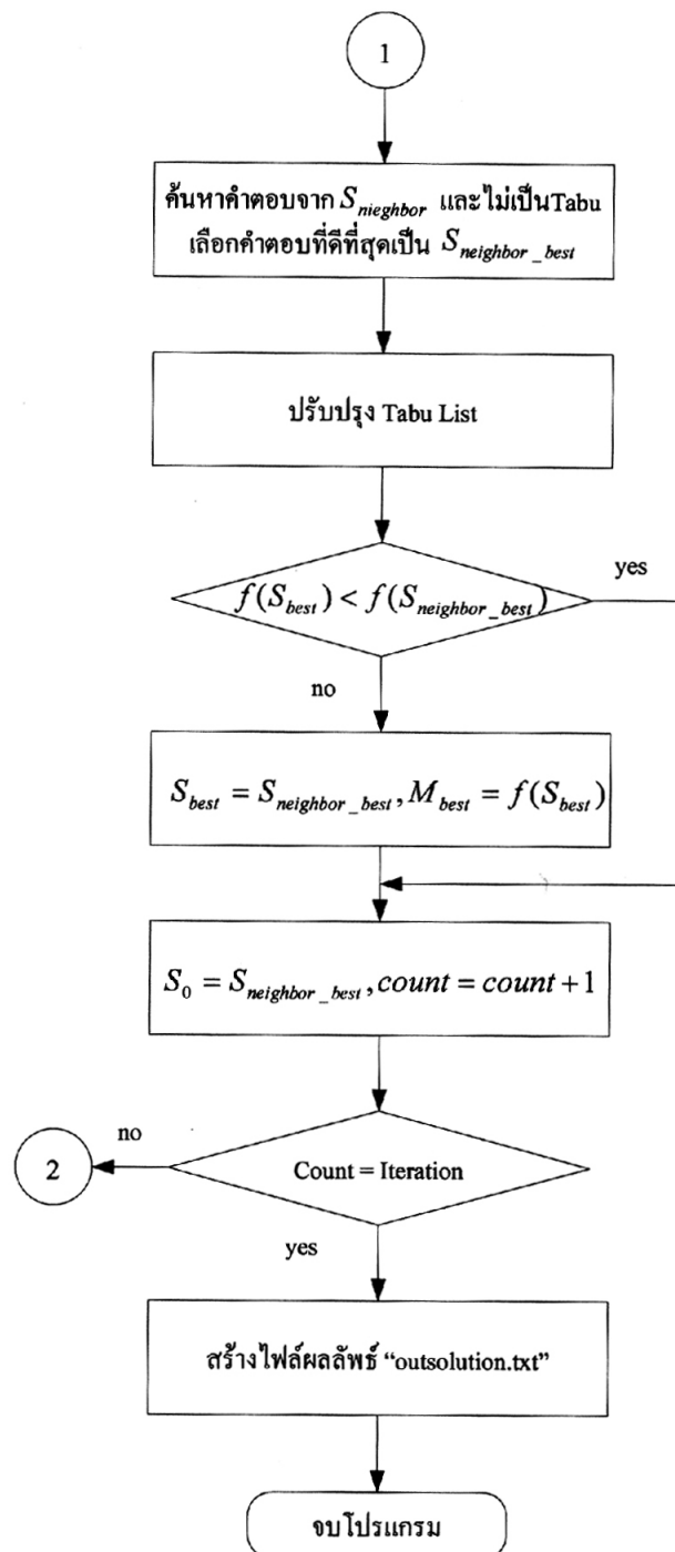
ภาพที่ 5 ขั้นตอนการทำงานของโปรแกรมจัดการการผลิตแบบไฟล์ชื่อป โดยใช้วิธีการหาคำตอบแบบทามู
