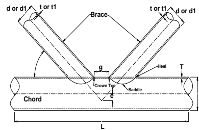
b) Circular K-joint
