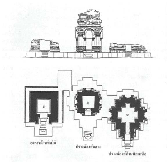
แผนผังที่ 1 ผังอาคารปราสาทเขาน้อย
