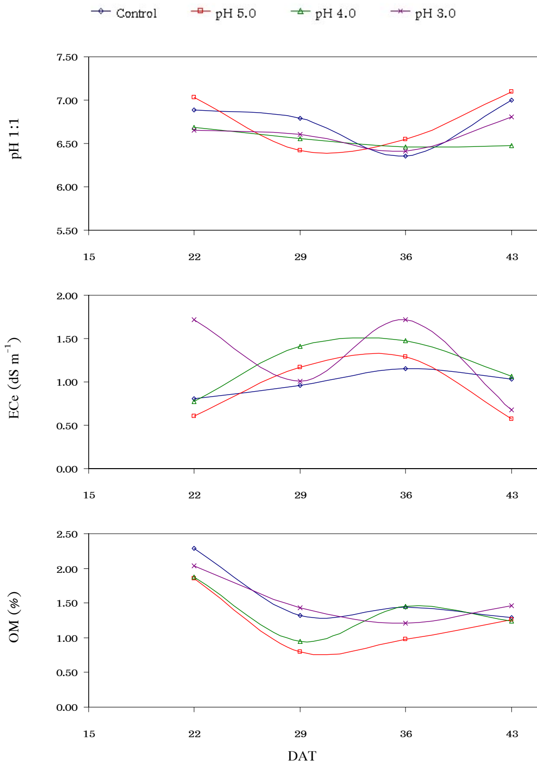
ภาพที่ 12 การเปลี่ยนแปลง pH 1:1, ECe และ OM ของชุดดินบางกอกที่ระดับความลึก 0-20 cm ภายหลังจากได้รับฝนจำลองที่เกิดจากอนุโมลซัลเฟตที่เวลาต่างๆ
