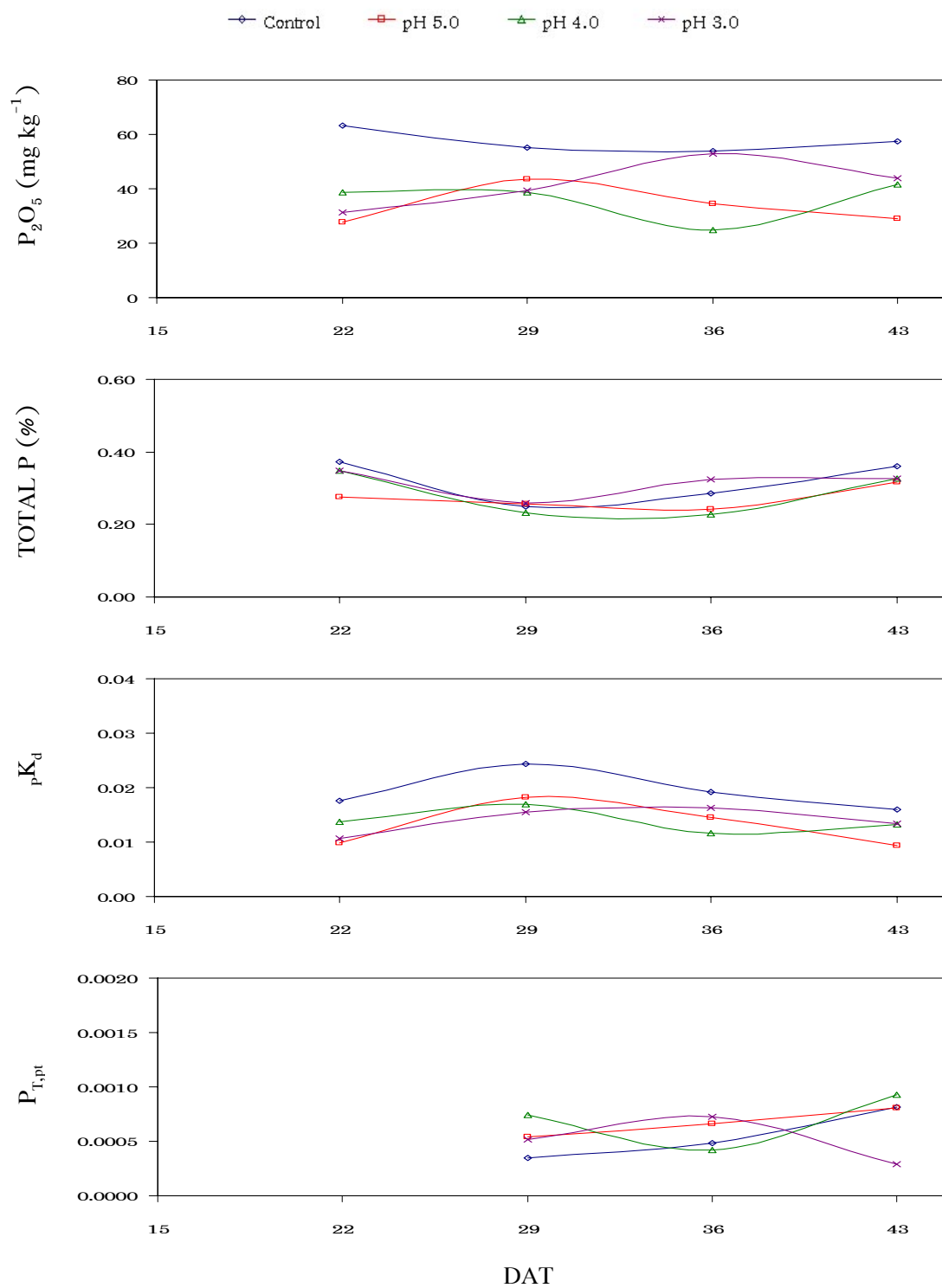
ภาพที่ 14 การเปลี่ยนแปลง P_2O_5 , Total P, pK_d และ P_{\Gamma,pt} ของชุดดินบางกอกที่ระดับความลึก 0-20 cm ภายหลังจากได้รับฝนจำลองที่เกิดจากอนุโมลซัลเฟตที่เวลาต่างๆ
