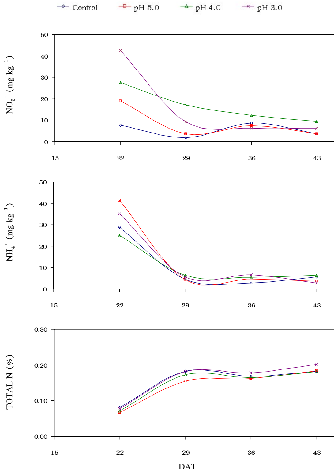
ภาพที่ 13 การเปลี่ยนแปลง \text{NO}_3^- , \text{NH}_4^+ , Total N, N_{K_d} และ N_{T,pt} ของชุดดินบางกอกที่ระดับความลึก 0-20 cm ภายหลังจากได้รับฝนจำลองที่เกิดจากอนุโมลซัลเฟตที่เวลาต่างๆ
