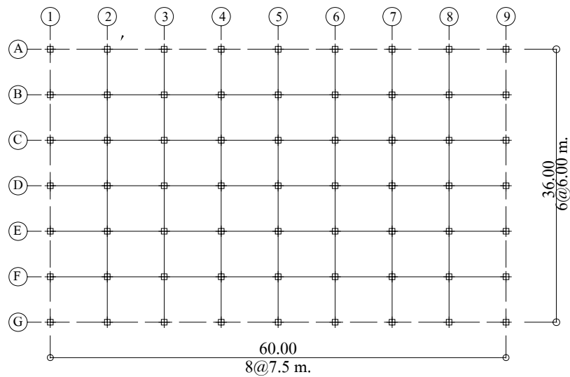
รูปที่ 6.1 แผนผังอาคาร 3 ชั้น
