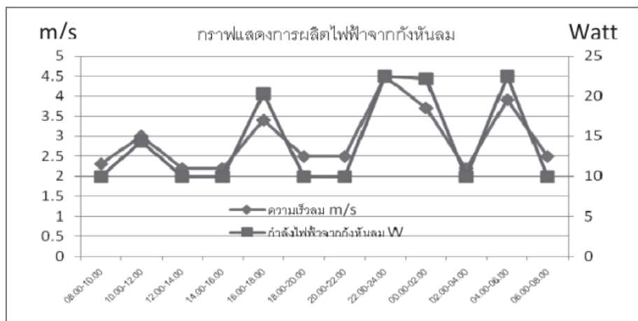
ภาพที่ 5 กำลังไฟฟ้าที่ผลิตได้จากกังหันลมแกนนอน 3 ใบพัดขนาดเส้นผ่านศูนย์กลาง 2.4 m
