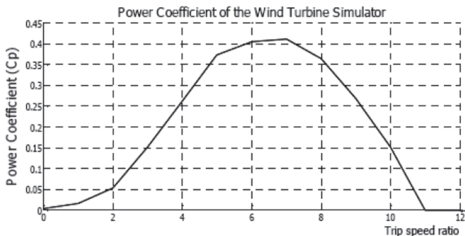
ภาพที่ 3 ประสิทธิภาพของกังหันลมที่ค่าอัตราส่วนความเร็วปลายใบ ต่างๆ (สว้าง ขาดิทอง และ วิรัชย์ โรยรินรินทร์, 2554)
