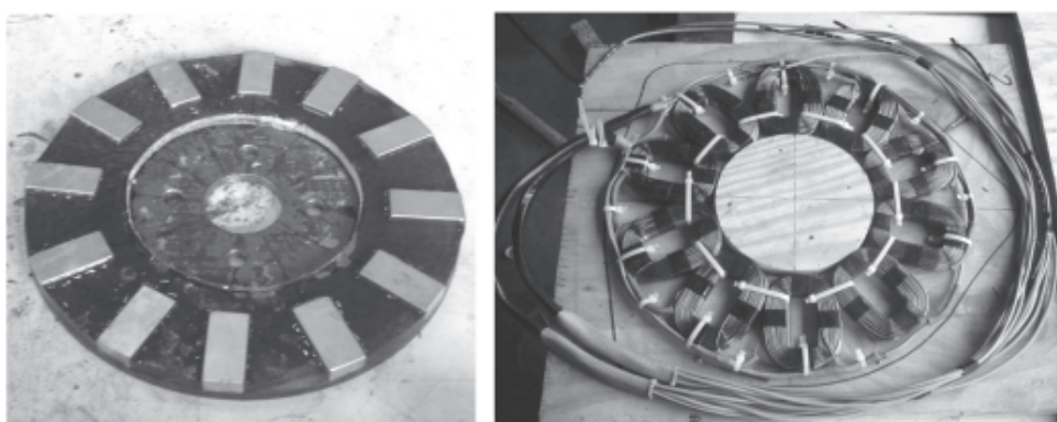
ภาพที่ 4 เครื่องกำเนิดไฟฟ้าที่สร้างจากแม่เหล็ก 12 แท่งและขดลวดที่พันขึ้นเอง
