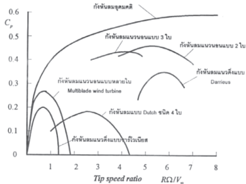
ประสิทธิภาพของกังหันลม
