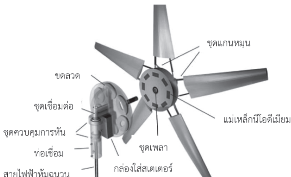
ภาพที่ 2 ชุดใบพัดและแกนหมุนใบพัดกับชุดเครื่องกำเนิดไฟฟ้า
