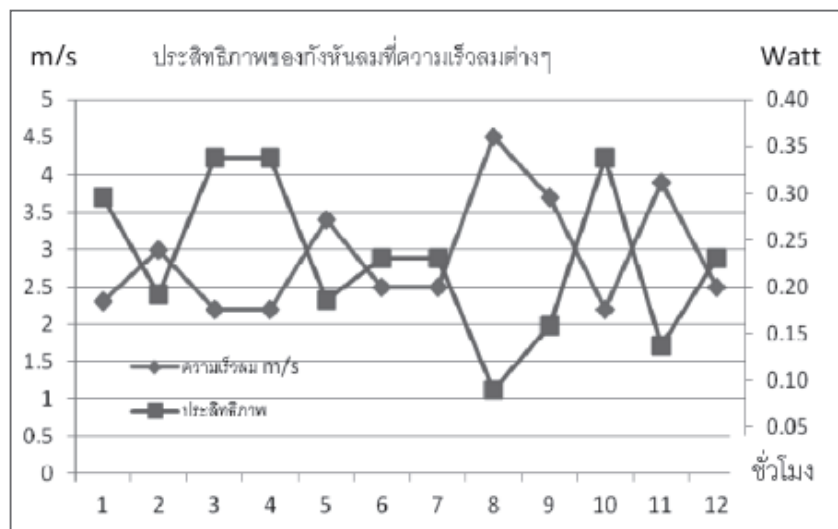
ภาพที่ 6 แสดงความเปลี่ยนแปลงของค่าประสิทธิภาพของกังหันลมที่ความเร็วลมต่างๆ
