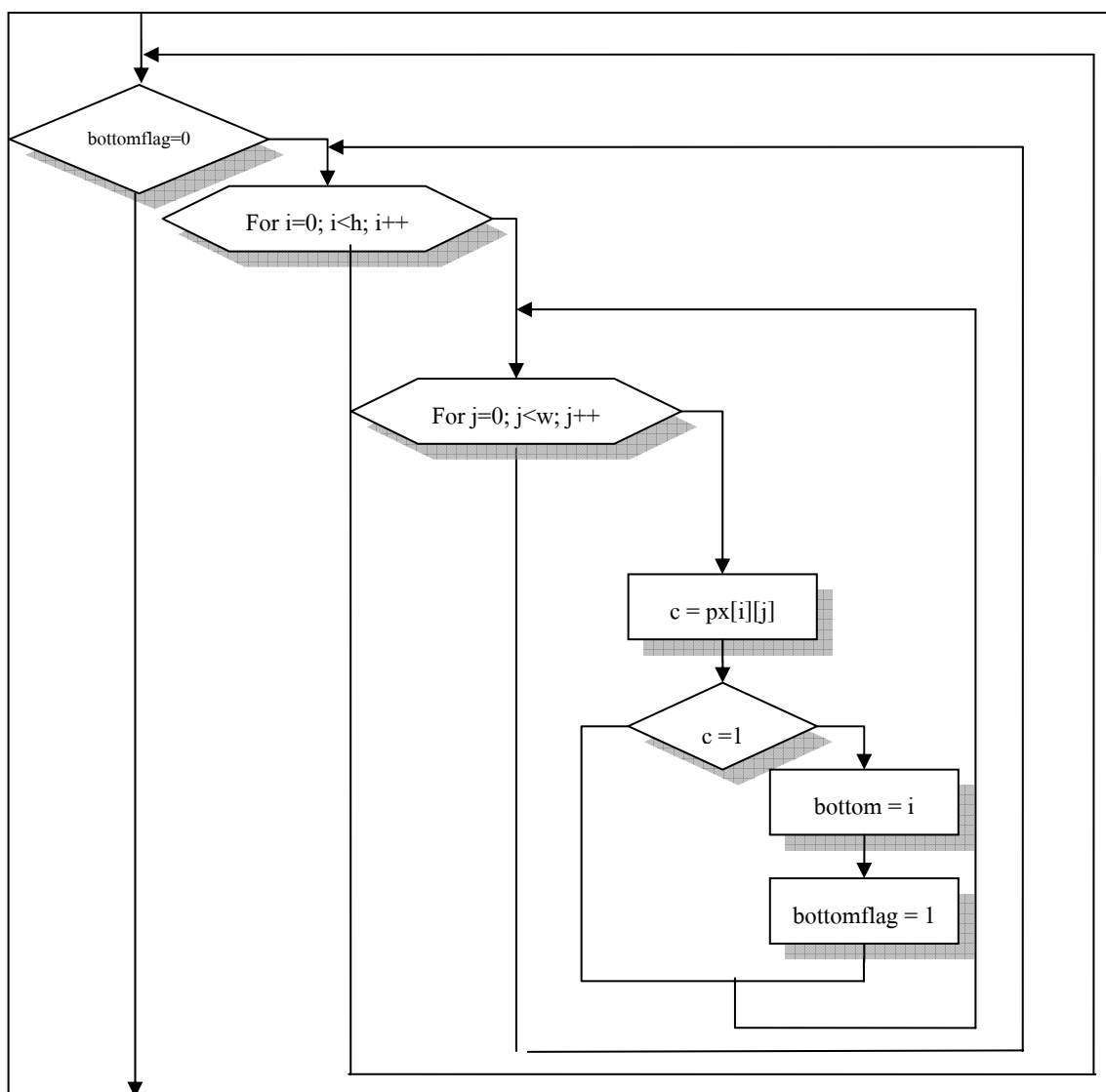
รูปที่ 12 แสดงขั้นตอนการหาค่าขอบเขตล่างของตัวอักษร
