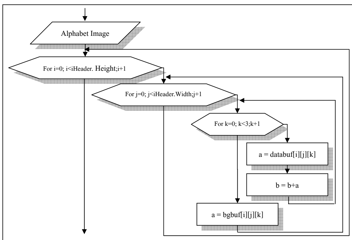
รูปที่ 8 ขั้นตอนการอ่านค่าสีในแต่ละพิกเซลเพื่อทำการรวมค่าสี
