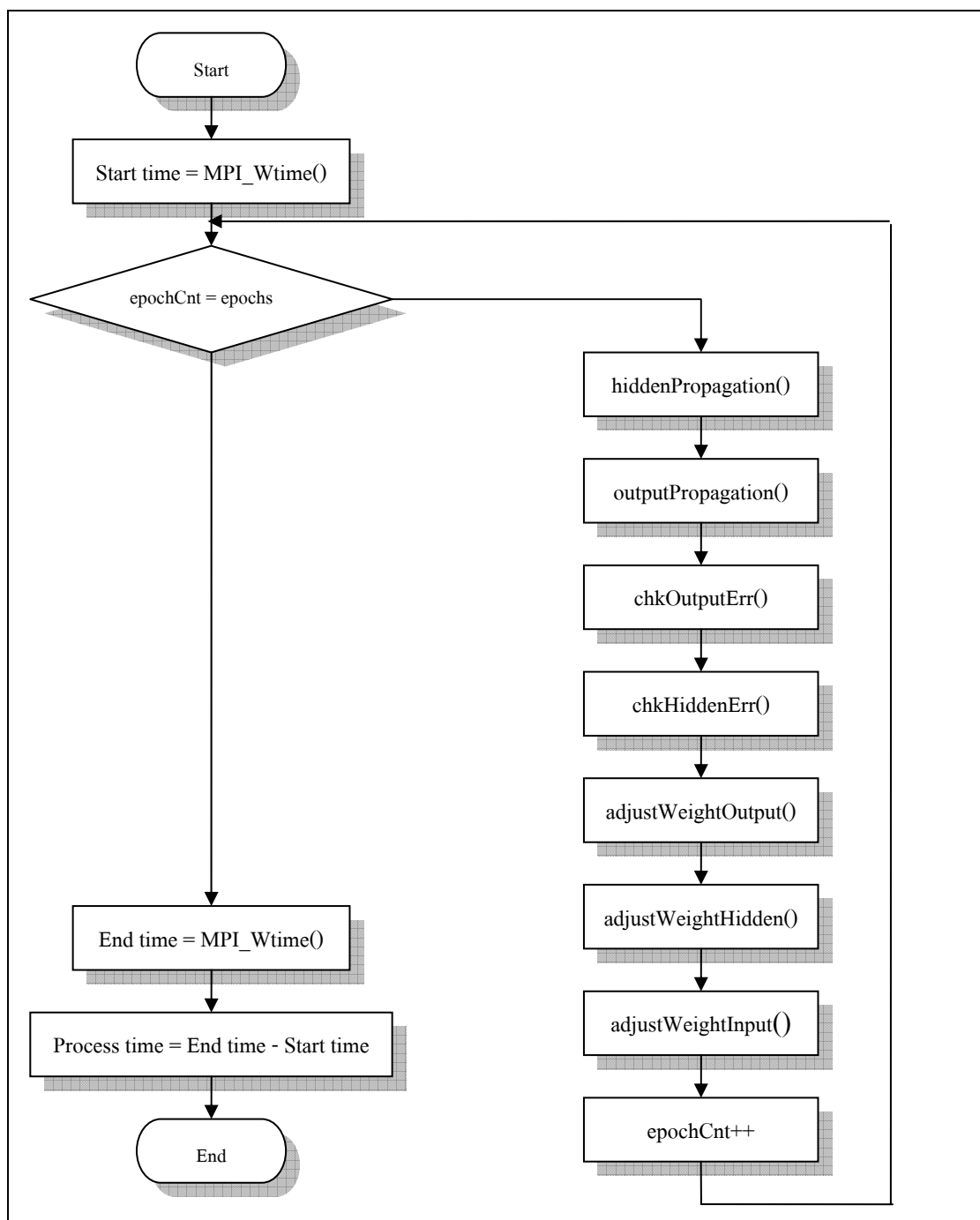
รูปที่ 19 ขั้นตอนการทำงานของโปรแกรมประยุกต์การเรียนรู้จำแบบปกติ
