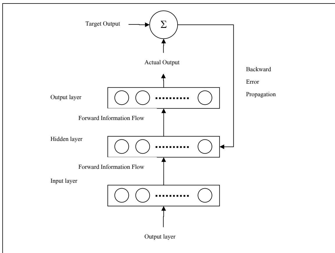
รูปที่ 3 แสดงรูปแบบ Backpropagation Neural Network
