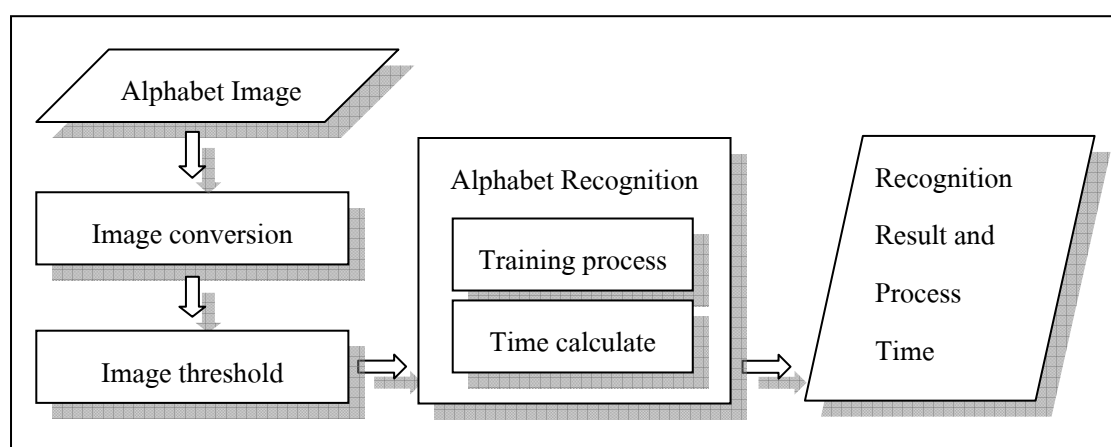
รูปที่ 6 ขั้นตอนการทำงานของโปรแกรมประยุกต์การรู้จำแบบปกติ
