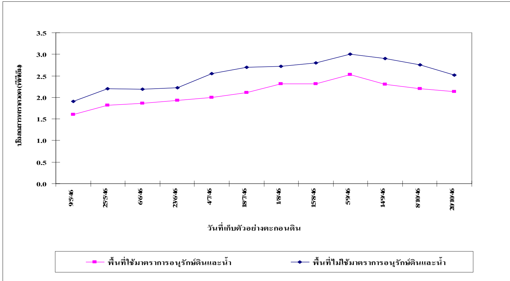
ภาพที่ 20 ปริมาณสารฟรอกตตัวอย่างตะกอนดินจากอาคารวัดน้ำพื้นที่มีการใช้และไม่ใช้มาตรการอนุรักษ์ดินและน้ำ
