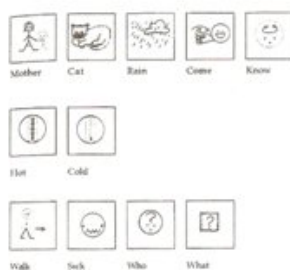
Picsyms
