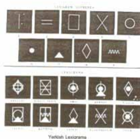
Yerkes Lexigrams
