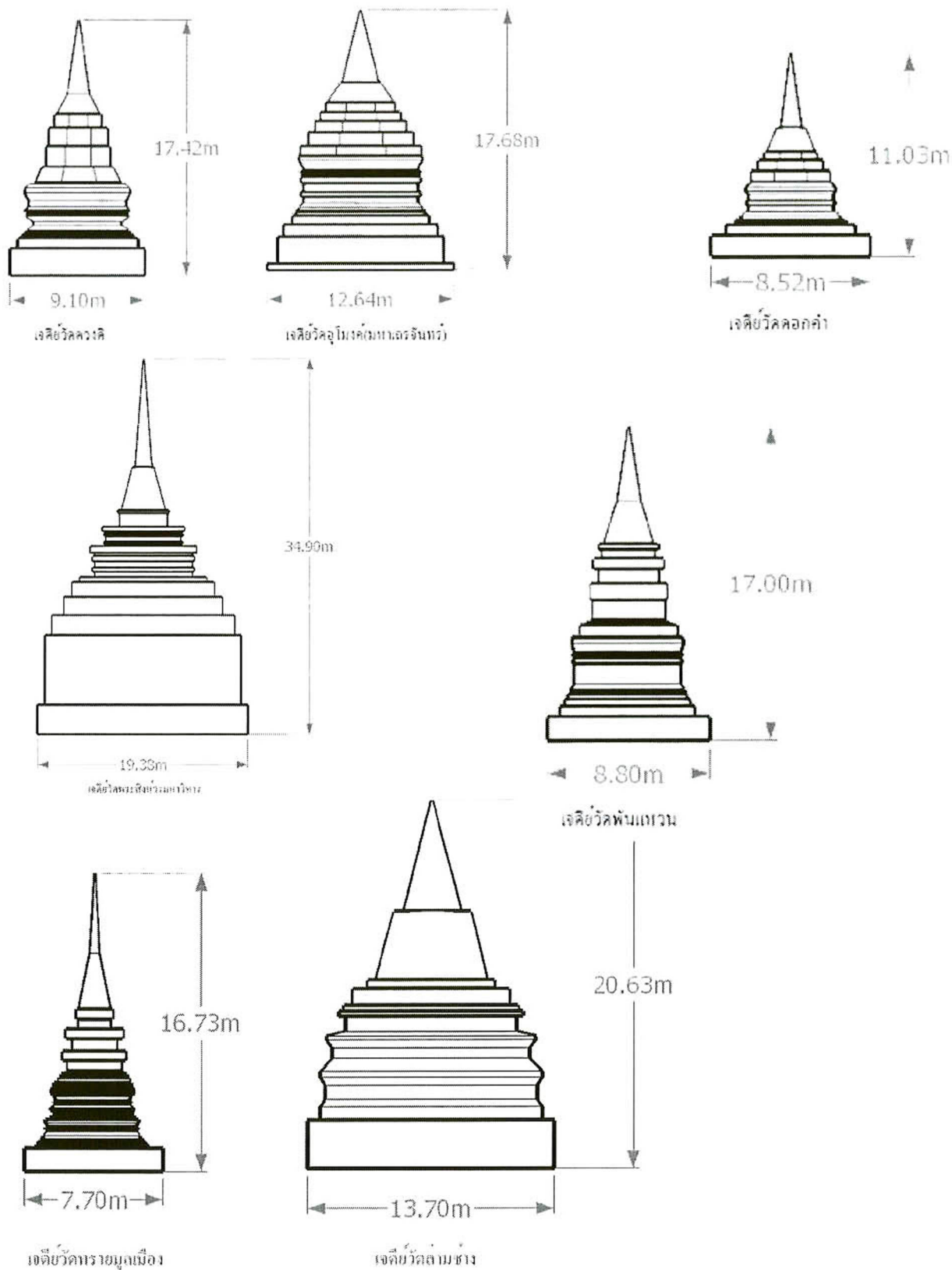
รูปที่ ๔.๒ ลักษณะทางกายภาพของเจดีย์ทรงระฆังแบบพื้นเมือง (ไม่ตามสเกล)
