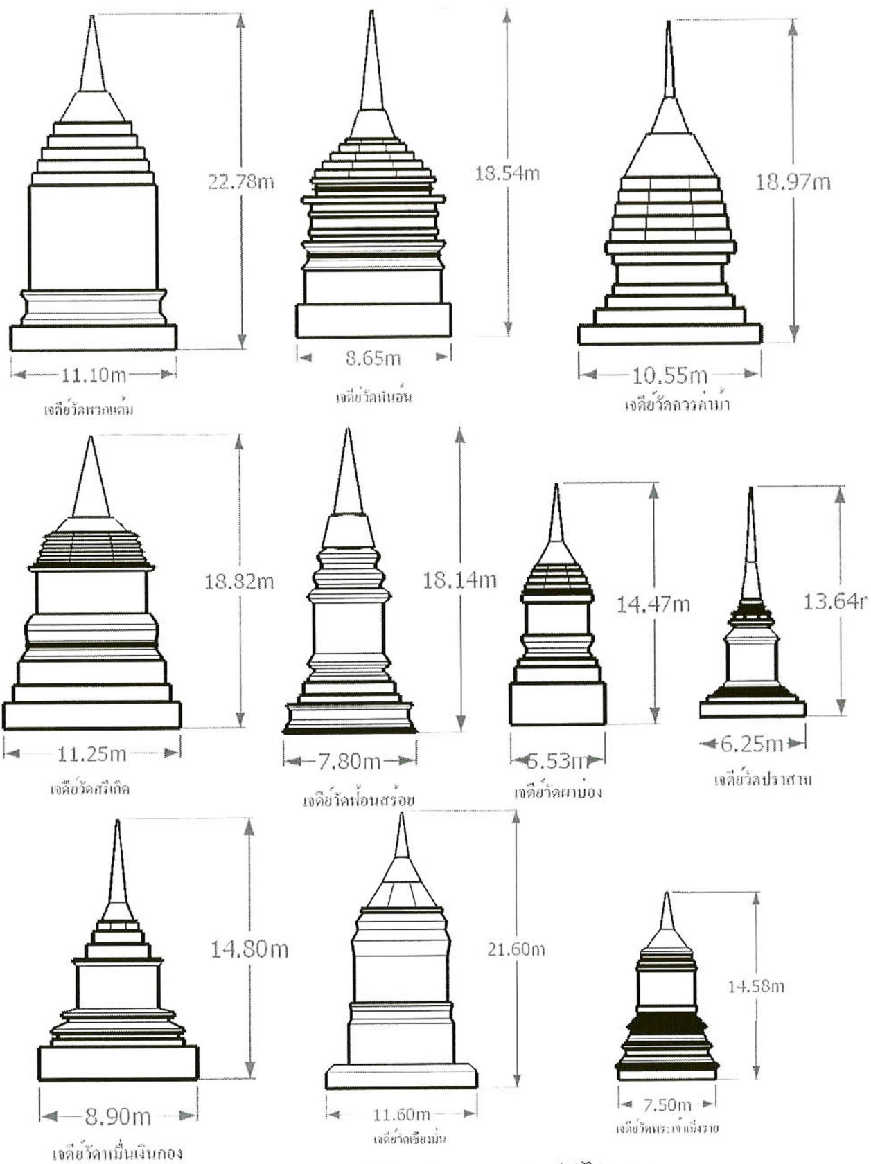
รูปที่ ๔.๕ ลักษณะทางกายภาพของเจดีย์ทรงปราสาทยอดเจดีย์(ไม่ตามสเกล)
