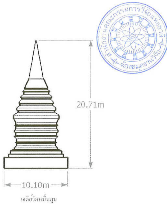
รูปที่ ๔.๘ ลักษณะทางกายภาพของเจดีย์ทรงอื่นๆ(เจดีย์เพ็ญมูม) (ไม่ตามสเกล)
