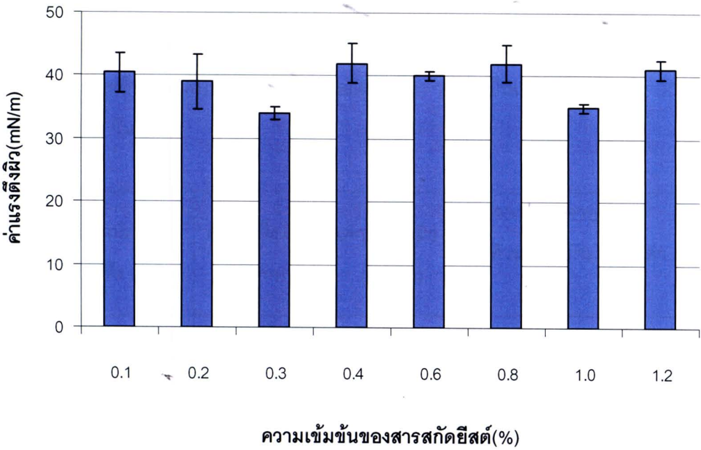
รูปที่ 4.3 แสดงค่าแรงตึงผิวของน้ำเลี้ยงเชื้อจาก Pichia anomala PY1 ที่แปรผันความเข้มข้นของสารสกัดยีสต์ในอาหารเลี้ยงเชื้อที่ใช้ไขมันถั่วเหลืองร่วมกับน้ำตาลกลูโคสในอัตราส่วน 2:1 เป็นแหล่งคาร์บอนที่ 30 องศาเซลเซียส เป็นเวลา 7 วัน
