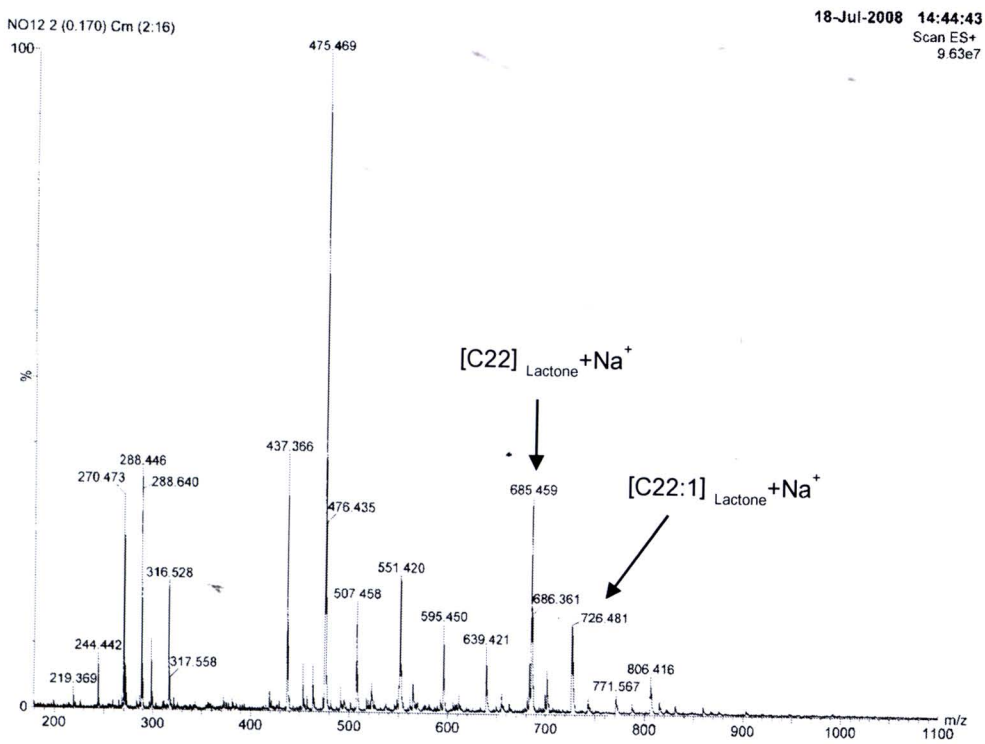
รูปที่ 4.23 โคโรมาโตแกรมของ LC-MS ของตัวอย่างสาร E
