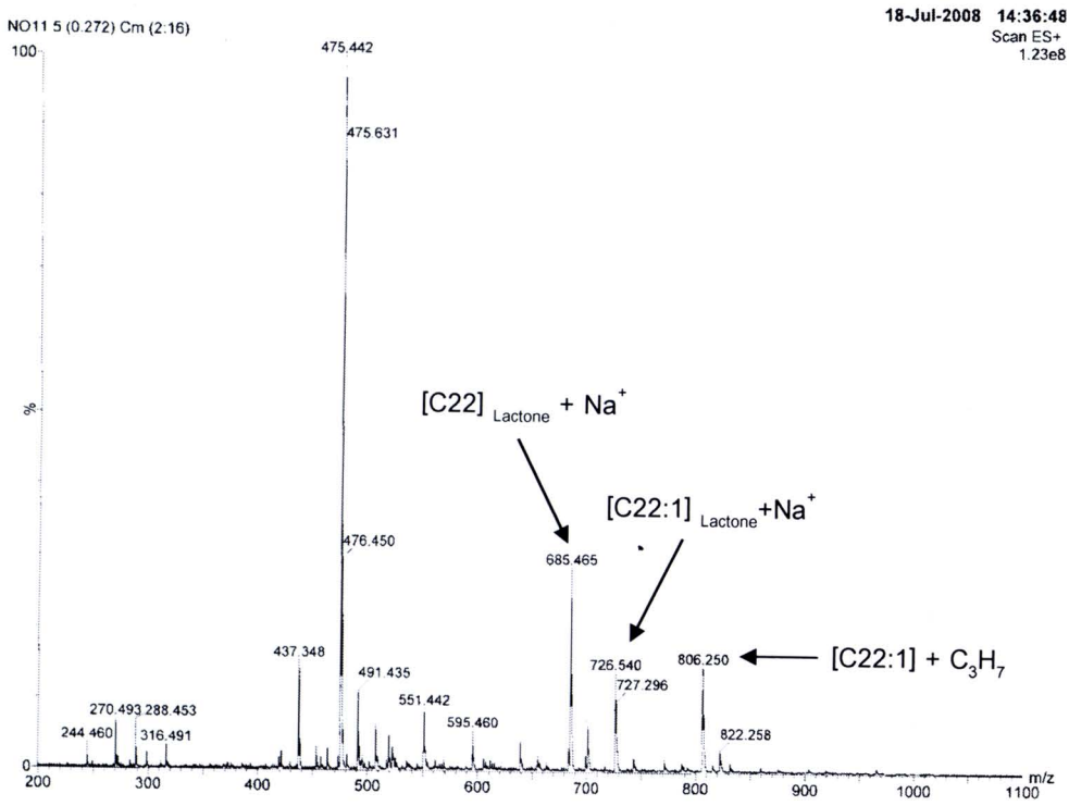
รูปที่ 4.22 โคโรมาโตแกรมของ LC-MS ของตัวอย่างสาร D
