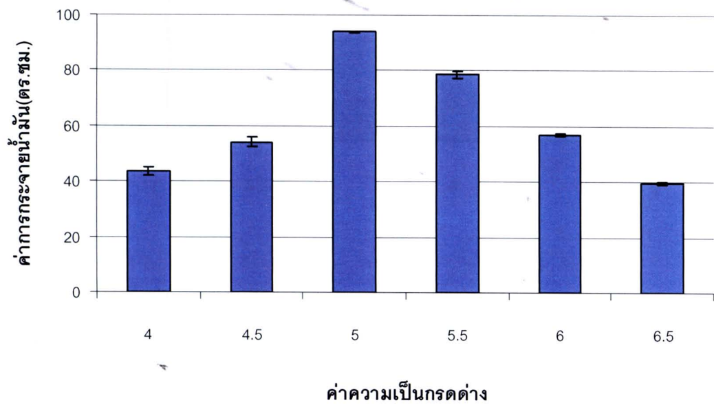
รูปที่ 4.6 แสดงค่าการกระจายน้ำมันของน้ำเลี้ยงเชื้อจาก Pichia anomala สายพันธุ์ PY1 ทำการแปรผันค่าความเป็นกรดต่างเริ่มต้นของอาหารเลี้ยงเชื้อที่ใช้น้ำมันถั่วเหลืองร่วมกับน้ำตาลกลูโคสในอัตราส่วน 2:1 เป็นแหล่งคาร์บอน เท่ากับ 4.0, 4.5, 5.0, 5.5, 6.0 และ 6.5
