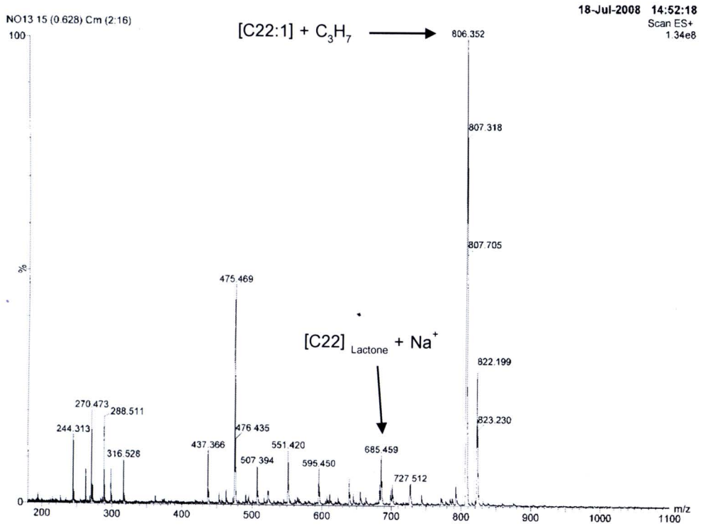
รูปที่ 4.24 โครมาโตแกรมของ LC-MS ของตัวอย่างสาร F
