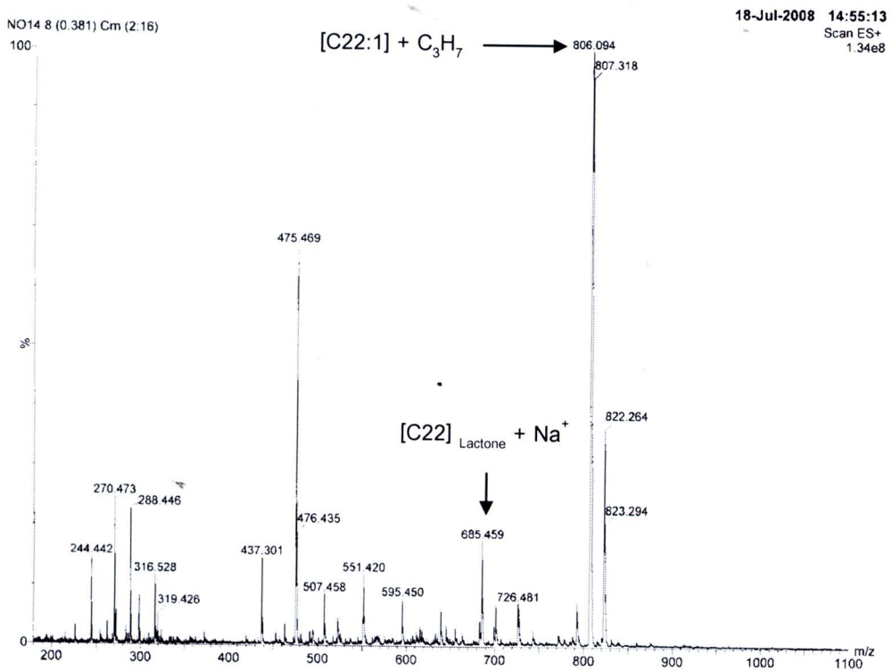
รูปที่ 4.25 โครมาโตแกรมของ LC-MS ของตัวอย่างสาร G
