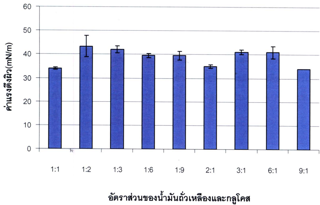
รูปที่ 4.1 แสดงค่าแรงตึงผิวของน้ำเลี้ยงเชื้อจาก Pichia anomala PY1 ที่ใช้น้ำมันถั่วเหลืองร่วมกับน้ำตาลกลูโคสในอัตราส่วนต่างๆ กันเป็นแหล่งคาร์บอนที่ 30 องศาเซลเซียส เป็นเวลา 7 วัน
