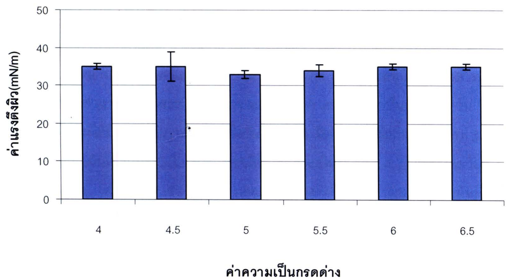
รูปที่ 4.5 แสดงค่าแรงดึงผิวของน้ำเลี้ยงเชื้อจาก Pichia anomala สายพันธุ์ PY1 ทำการแปรผันค่าความเป็นกรดต่างเริ่มต้นของอาหารเลี้ยงเชื้อที่ใช้น้ำมันถั่วเหลืองร่วมกับน้ำตาลกลูโคสในอัตราส่วน 2:1 เป็นแหล่งคาร์บอน เท่ากับ 4.0, 4.5, 5.0, 5.5, 6.0 และ 6.5
