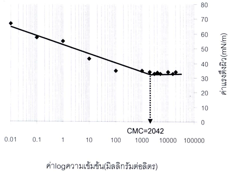
รูปที่ 4.14 แสดงการหาค่า CMC ซึ่งเขียนกราฟระหว่างค่าแรงตึงผิวและ log ของความเข้มข้นของ สารลดแรงตึงผิวสังเคราะห์ เคมีเทค 307
