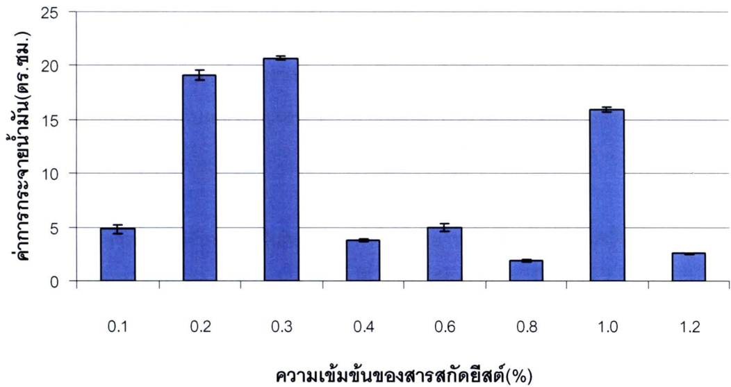
รูปที่ 4.4 แสดงค่าการกระจายน้ำมันของน้ำเลี้ยงเชื้อจาก Pichia anomala PY1 ที่แปรผันความเข้มข้นของสารสกัดยีสต์ในอาหารเลี้ยงเชื้อที่ใช้น้ำมันถั่วเหลืองร่วมกับน้ำตาลกลูโคสในอัตราส่วน 2:1 เป็นแหล่งคาร์บอนที่ 30 องศาเซลเซียส เป็นเวลา 7 วัน
