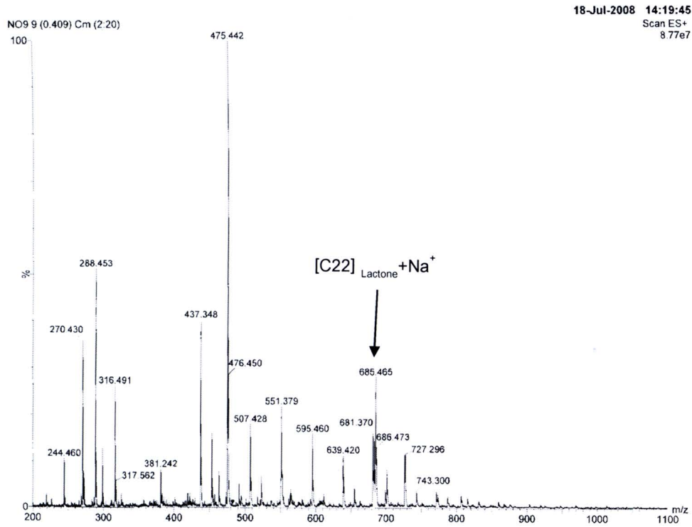
รูปที่ 4.20 โคโรมาโตแกรมของ LC-MS ของตัวอย่างสาร B
