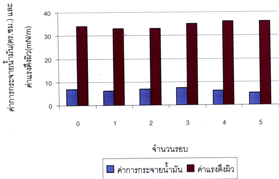
รูปที่ 4.12 กราฟแสดงจำนวนรอบทดสอบค่าการกระจายน้ำมันและค่าแรงตึงผิวของสารลดแรงตึงผิวชีวภาพที่ผลิตได้จาก Pichia anomala สายพันธุ์ PY 1 และผ่านการบ่มที่ 121 องศาเซลเซียส เป็นเวลา 15 นาที
