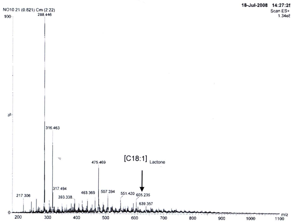
รูปที่ 4.21 โคโรมาโตแกรมของ LC-MS ของตัวอย่างสาร C
