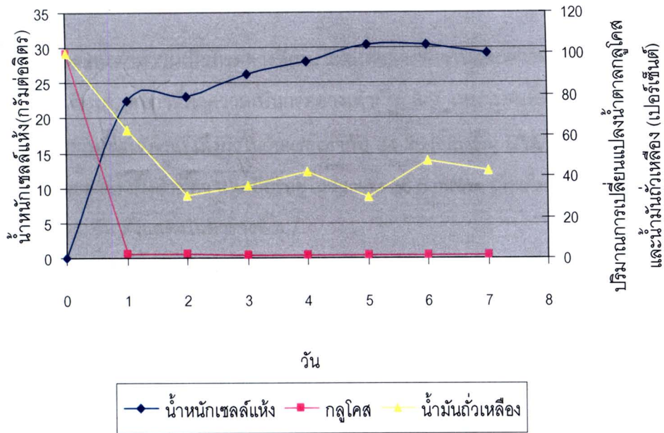
รูปที่ 4.9 กราฟแสดงความสัมพันธ์ระหว่างการเจริญของเชื้อยีสต์ Pichia anomala สายพันธุ์ PY1 และการเปลี่ยนแปลงปริมาณน้ำมันถั่วเหลืองและน้ำตาลกลูโคสที่ถูกใช้ไปในอาหารเลี้ยงเชื้อที่ประกอบด้วย น้ำมันถั่วเหลืองและน้ำตาลกลูโคสในอัตราส่วน 2:1 เป็นแหล่งคาร์บอน
