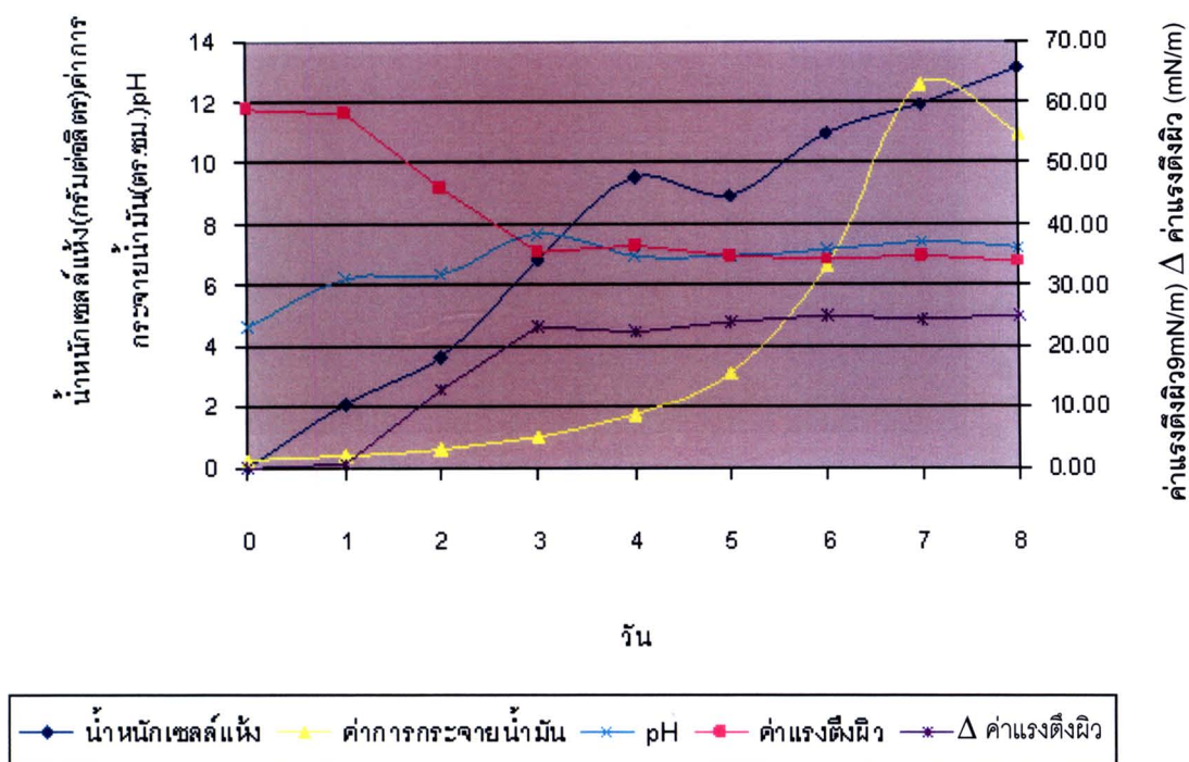
รูปที่ 4.8 กราฟแสดงความสัมพันธ์ระหว่างการเจริญของเชื้อยีสต์ Pichia anomala สายพันธุ์ PY1 และการผลิตสารลดแรงตึงผิวชีวภาพในอาหารเลี้ยงเชื้อที่ใช้น้ำมันถั่วเหลืองเป็นแหล่งคาร์บอนเพียงชนิดเดียว
