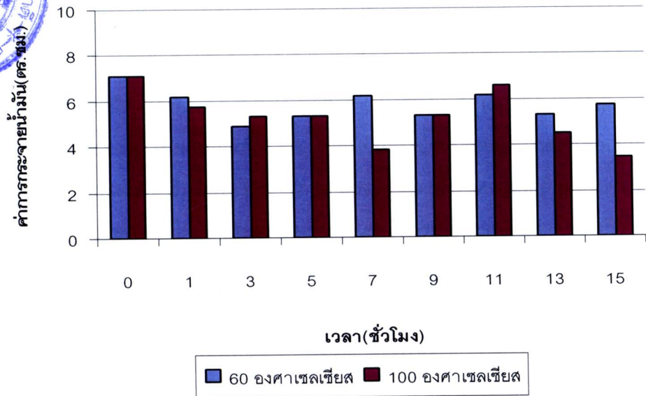
รูปที่ 4.11 กราฟแสดงค่าการกระจายน้ำมันของสารลดแรงตึงผิวชีวภาพที่ผลิตได้จาก Pichia anomala สายพันธุ์ PY 1 ที่อุณหภูมิ 60 และ 100 องศาเซลเซียส
