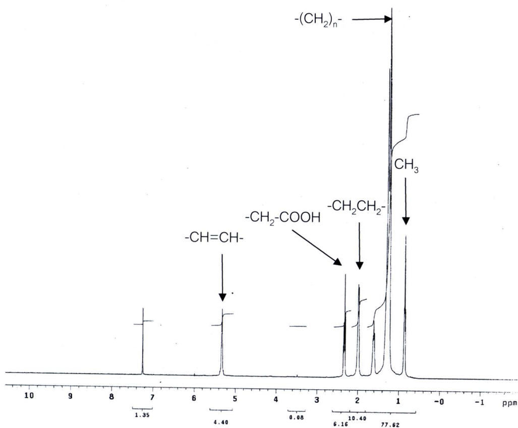
รูปที่ 4.26 ^1\text{H} -NMR spectrum ของตัวอย่าง G
