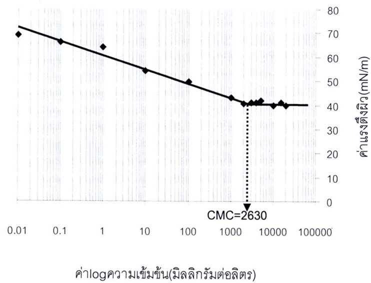
รูปที่ 4.16 แสดงการหาค่า CMC ซึ่งเขียนกราฟระหว่างค่าแรงตึงผิวและ log ของความเข้มข้นของสารลดแรงตึงผิวสังเคราะห์ไฮเดียมโดเดซิลซัลเฟต
