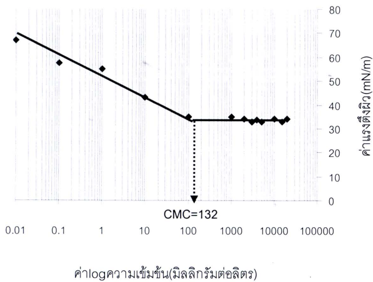
รูปที่ 4.13 แสดงการหาค่า CMC ซึ่งเขียนกราฟระหว่างค่าแรงตึงผิวและ log ของความเข้มข้นของสารลดแรงตึงผิวชีวภาพที่ผลิตได้จาก Pichia anomala สายพันธุ์ PY1
