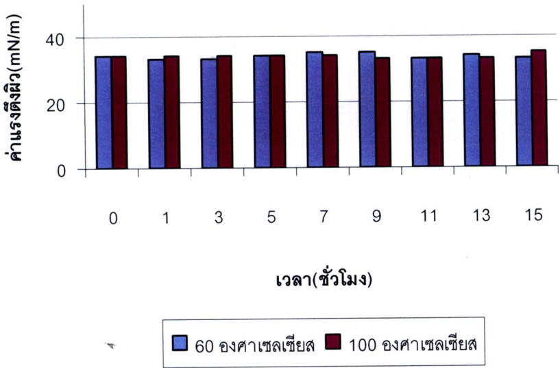
รูปที่ 4.10 กราฟแสดงค่าแรงตึงผิวของสารลดแรงตึงผิวชีวภาพที่ผลิตได้จาก Pichia anomala สายพันธุ์ PY 1 ที่อุณหภูมิ 60 และ 100 องศาเซลเซียส
