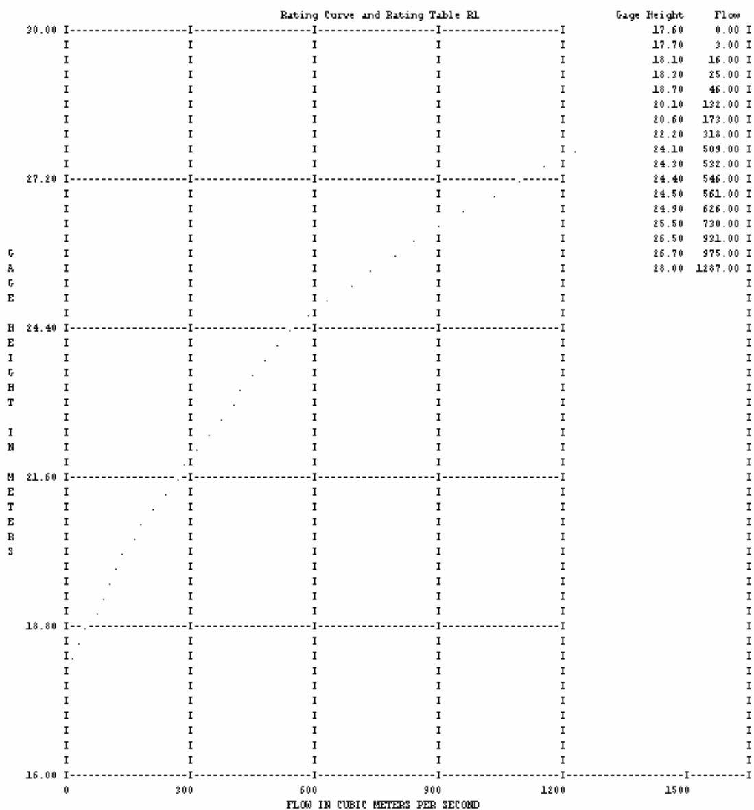
ภาพที่ 10 ตัวอย่างข้อมูลความสัมพันธ์ระหว่างระดับและปริมาณน้ำของสถานี N14A ที่มา: กรมชลประทาน (2547)
