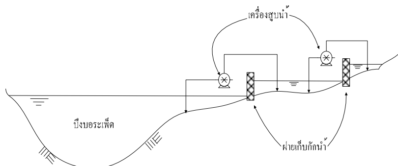
ภาพที่ 2 ลักษณะการสูบน้ำและการสร้างฝายทดน้ำของเกษตรกรในพื้นที่รอบบึงบอระเพ็ด ที่มา: นุชนารถและคณะ (2549)
