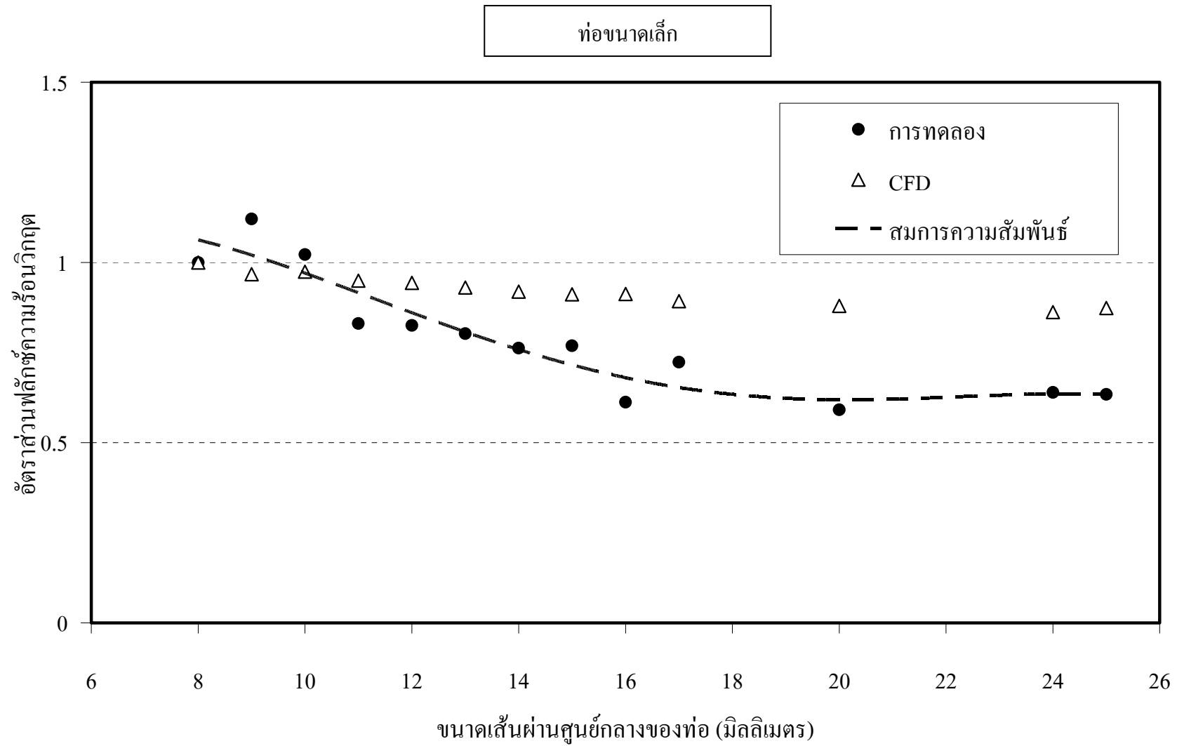
ภาพที่ 49 กราฟฟลักซ์ความร้อนวิกฤตสำหรับท่อ 8-25 มิลลิเมตร
