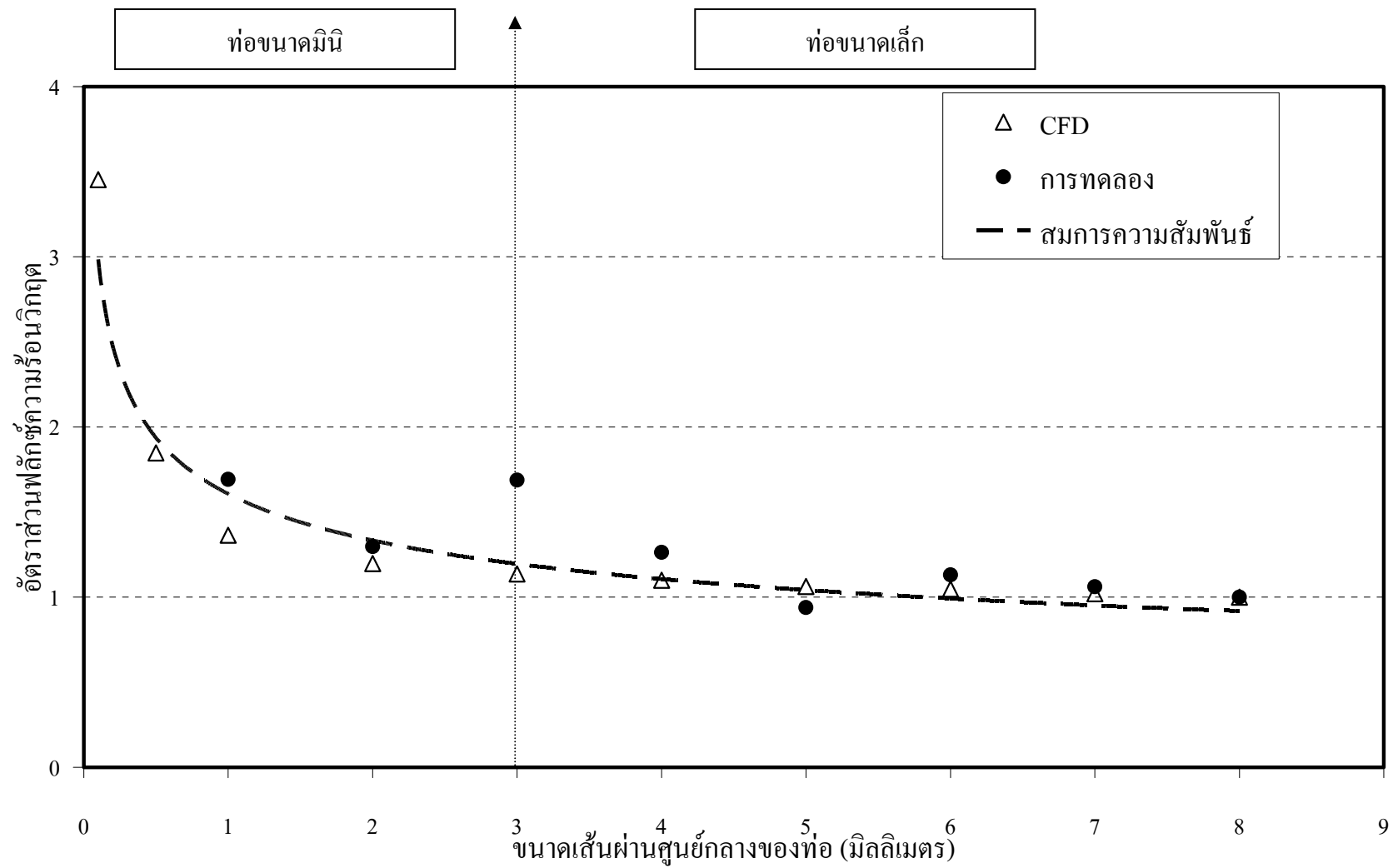
ภาพที่ 50 กราฟฟลักซ์ความร้อนวิกฤตสำหรับท่อ 0.1-8 มิลลิเมตร
