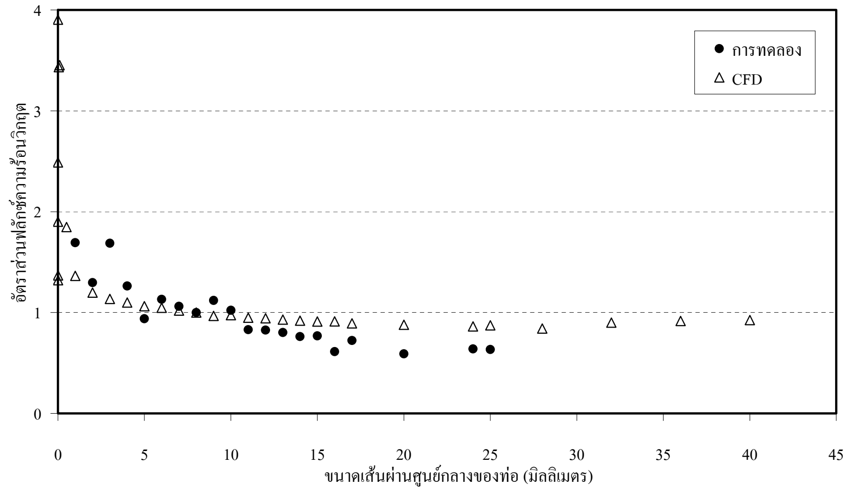
ภาพที่ 48 กราฟเปรียบเทียบฟลักซ์ความร้อนวิกฤตที่คำนวณได้กับการทดลอง
