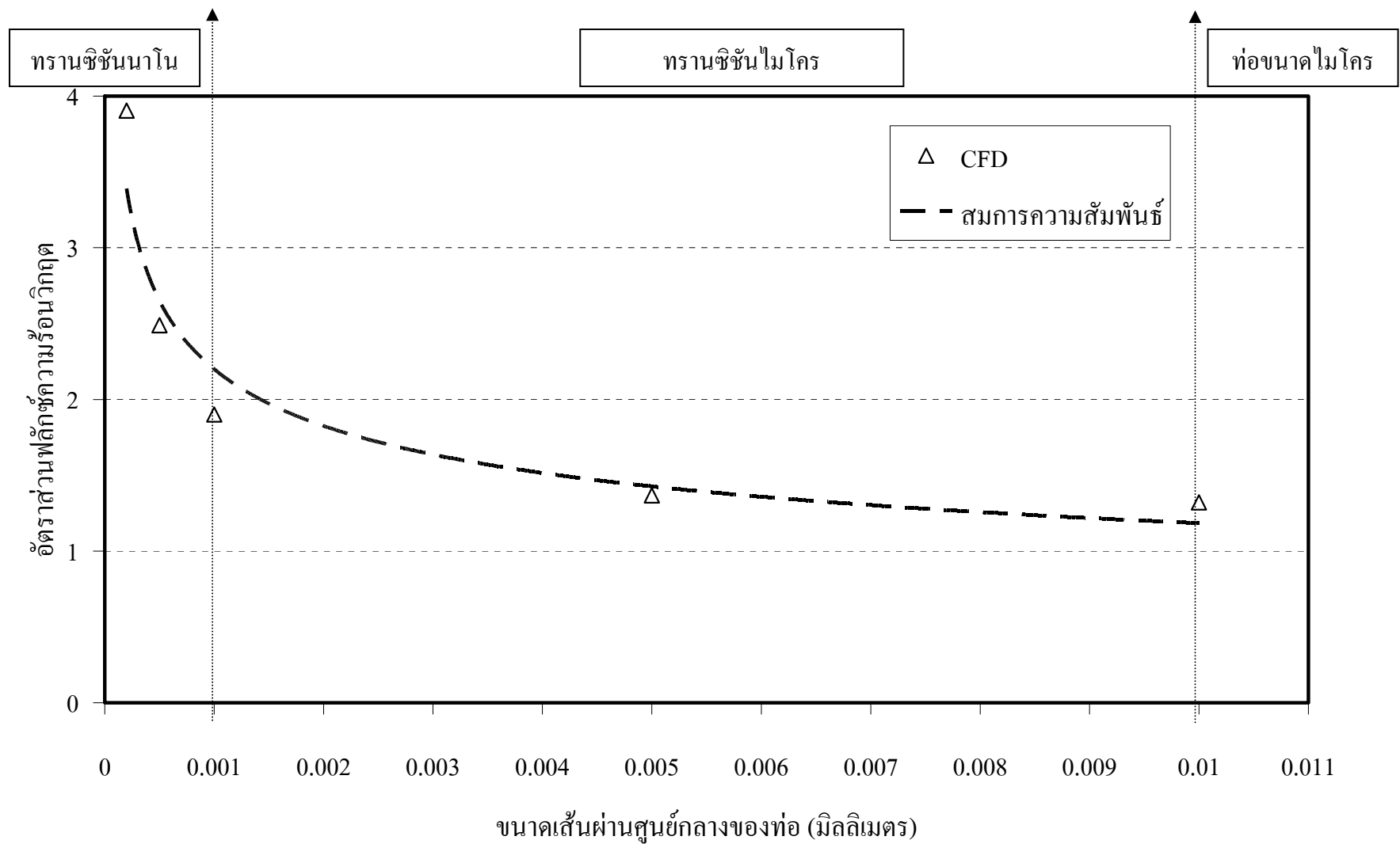
ภาพที่ 52 กราฟฟังก์ชันความร้อนวิกฤตสำหรับท่อ 0.0002-0.01 มิลลิเมตร
