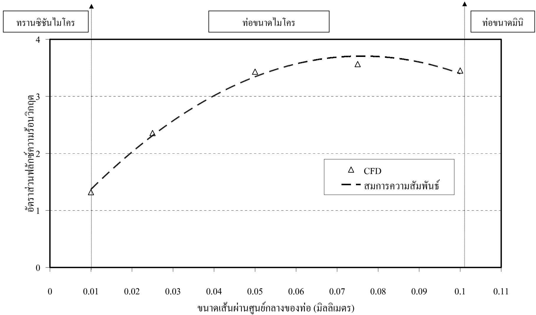
ภาพที่ 51 กราฟพื้นที่ผิวความร้อนวิกฤตสำหรับท่อ 0.01-0.1 มิลลิเมตร
