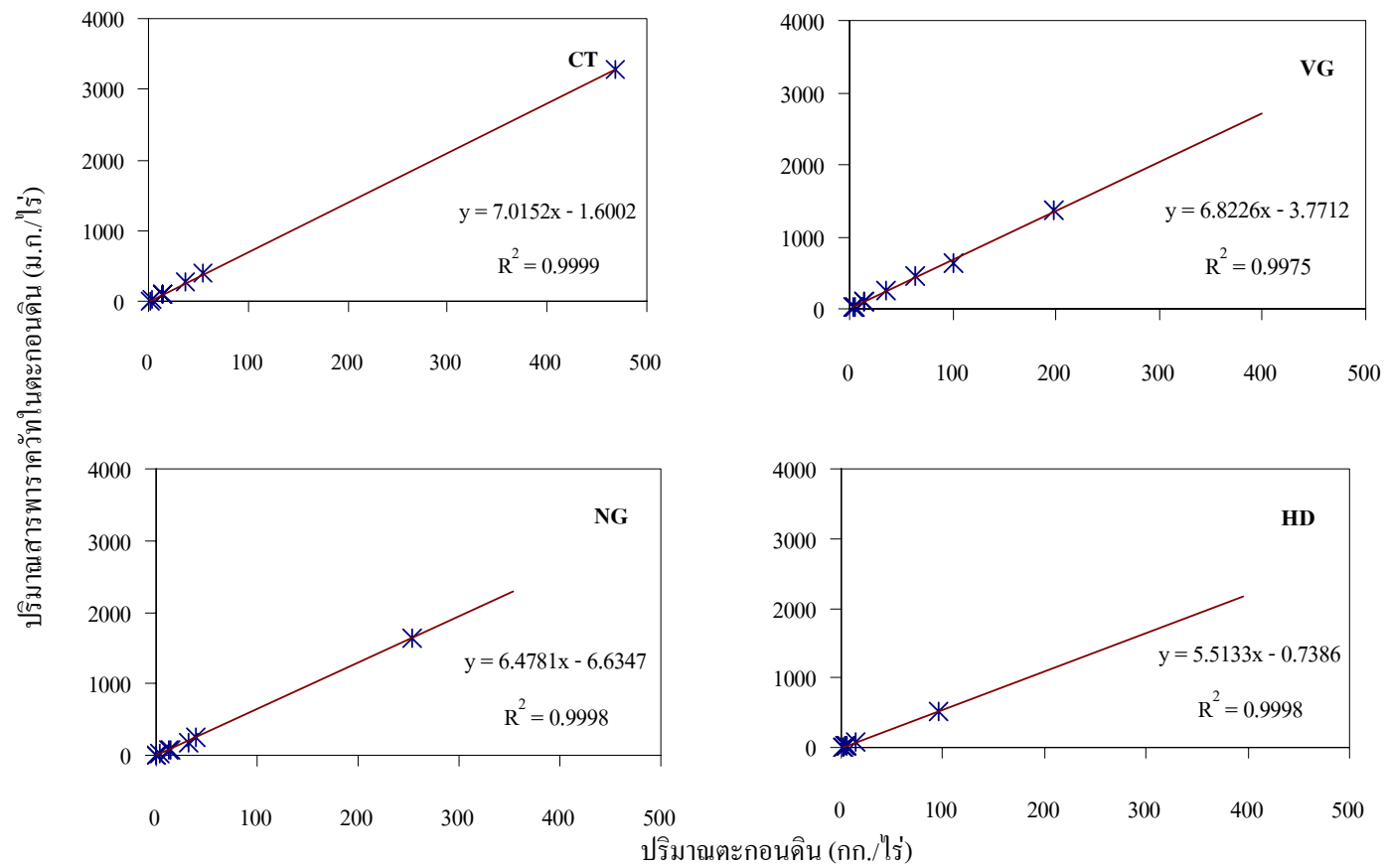
ภาพที่ 18 ความสัมพันธ์ของสารพาราควัทในตะกอนดินกับปริมาณตะกอนดินจากทั้ง 4 แปลงทดลอง ฤดูเพาะปลูกปี พ.ศ. 2546 (CT = แปลงที่ไม่มีมาตรการอนุรักษ์ดินและน้ำ VG = แปลงแถบหญ้าแฝกแถวเดี่ยว NG = แปลงแถบหญ้าธรรมชาติ และ HD = แปลงคูรับน้ำขอบเขา)
