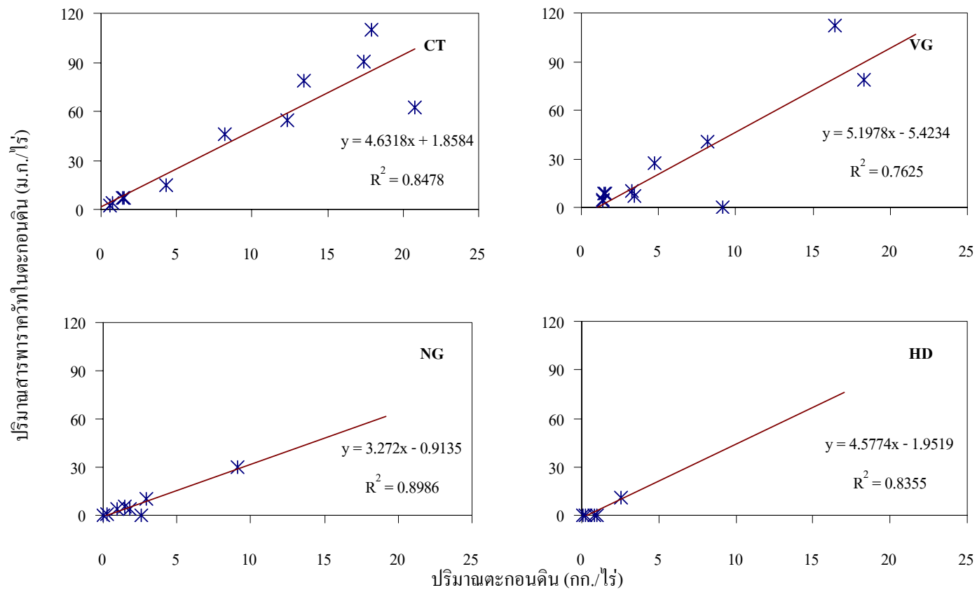
ภาพที่ 19 ความสัมพันธ์ของสารพาราควัทในตะกอนดินกับปริมาณตะกอนดินจากทั้ง 4 แปลงทดลอง ฤดูเพาะปลูกปี พ.ศ. 2547 (CT = แปลงที่ไม่มีมาตรการอนุรักษ์ดินและน้ำ VG = แปลงแถบหญ้าแฝกแถวเดี่ยว NG = แปลงแถบหญ้าธรรมชาติ และ HD = แปลงคูรับน้ำขอบเขา)
