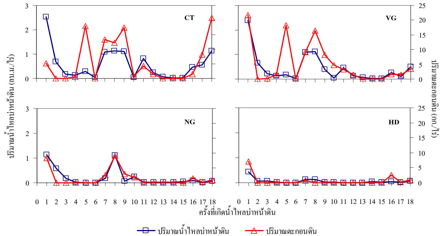
ภาพที่ 13 ปริมาณตะกอนดินและปริมาณน้ำไหลบ่าหน้าดินที่เกิดขึ้นในฤดูเพาะปลูกปี พ.ศ. 2547 (CT = แปลงที่ไม่มีมาตรการอนุรักษ์ดินและน้ำ VG = แปลงแถบหญ้าแฝกแถวเดี่ยว NG = แปลงแถบหญ้าธรรมชาติ และ HD = แปลงคูรับน้ำขอบเขา)
