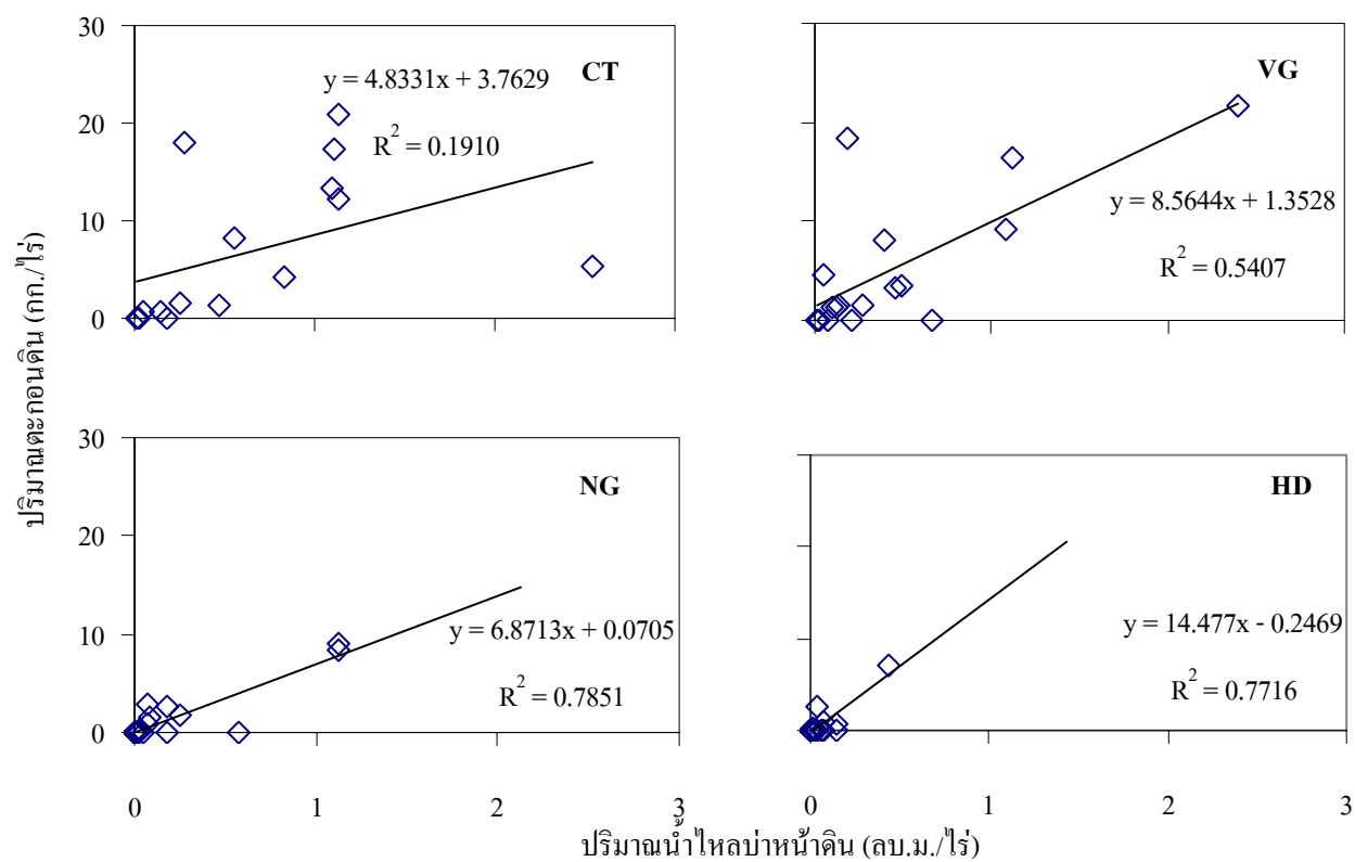
ภาพที่ 14 ความสัมพันธ์ระหว่างปริมาณตะกอนดินกับปริมาณน้ำไหลบ่าหน้าดิน ในฤดูเพาะปลูกปี พ.ศ. 2547 (CT = แปลงที่ไม่มีมาตรการอนุรักษ์ดินและน้ำ VG = แปลงแถบหญ้าแฝกแถวเดี่ยว NG = แปลงแถบหญ้าธรรมชาติ และ HD = แปลงคูรับน้ำขอบเขา)
