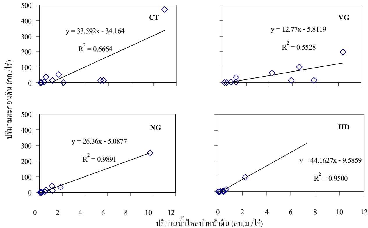
ภาพที่ 12 ความสัมพันธ์ระหว่างปริมาณตะกอนดินกับปริมาณน้ำไหลบ่าหน้าดิน ในฤดูเพาะปลูกปี พ.ศ. 2546 (CT = แปลงที่ไม่มีมาตรการอนุรักษ์ดินและน้ำ VG = แปลงแถบหญ้าแฝกแถวเดี่ยว NG = แปลงแถบหญ้าธรรมชาติ และ HD = แปลงคูรับน้ำขอบเขา)
