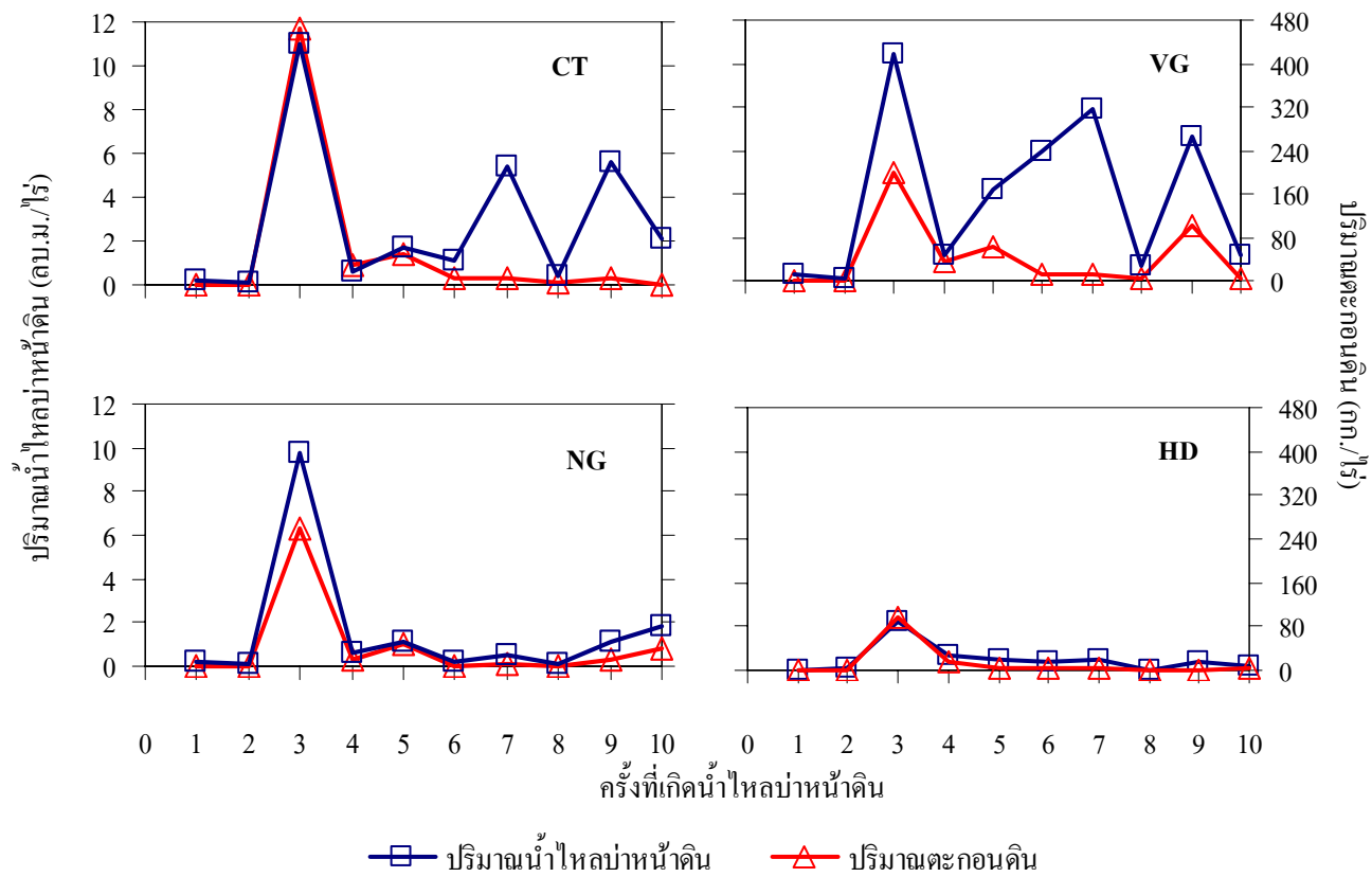
ภาพที่ 11 ปริมาณตะกอนดินและปริมาณน้ำไหลบ่าหน้าดินที่เกิดขึ้นในฤดูเพาะปลูกปี พ.ศ. 2546 (CT = แปลงที่ไม่มีมาตรการอนุรักษ์ดินและน้ำ VG = แปลงแถบหญ้าแฝกแถวเดี่ยว NG = แปลงแถบหญ้าธรรมชาติ และ HD = แปลงคูรับน้ำขอบเขา)
