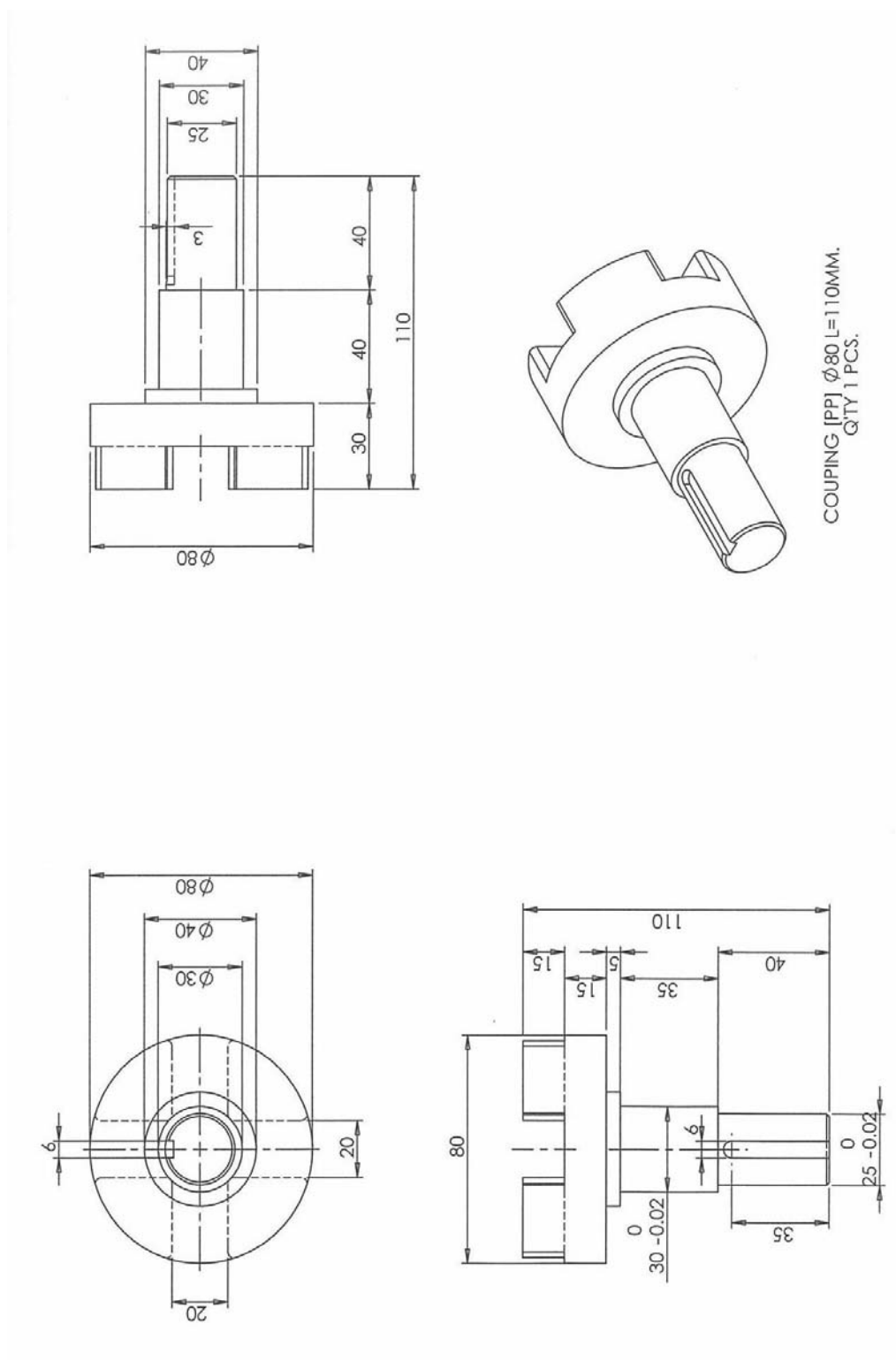
ภาพที่ ก.9 แบบวาดคัปปลิ่งขับถังหมุน
