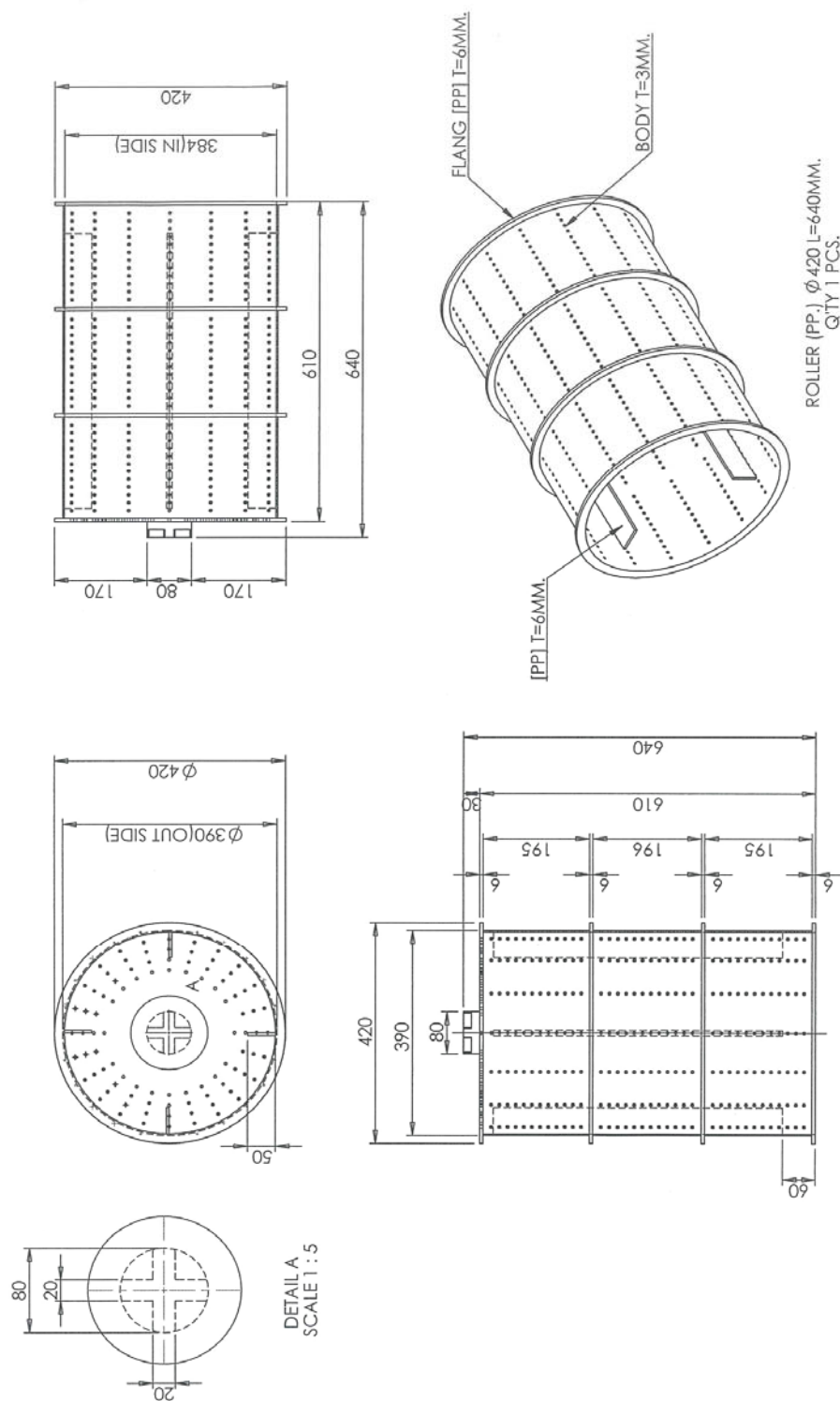
ภาพที่ ก.7 แบบวาดถึงหมุน
