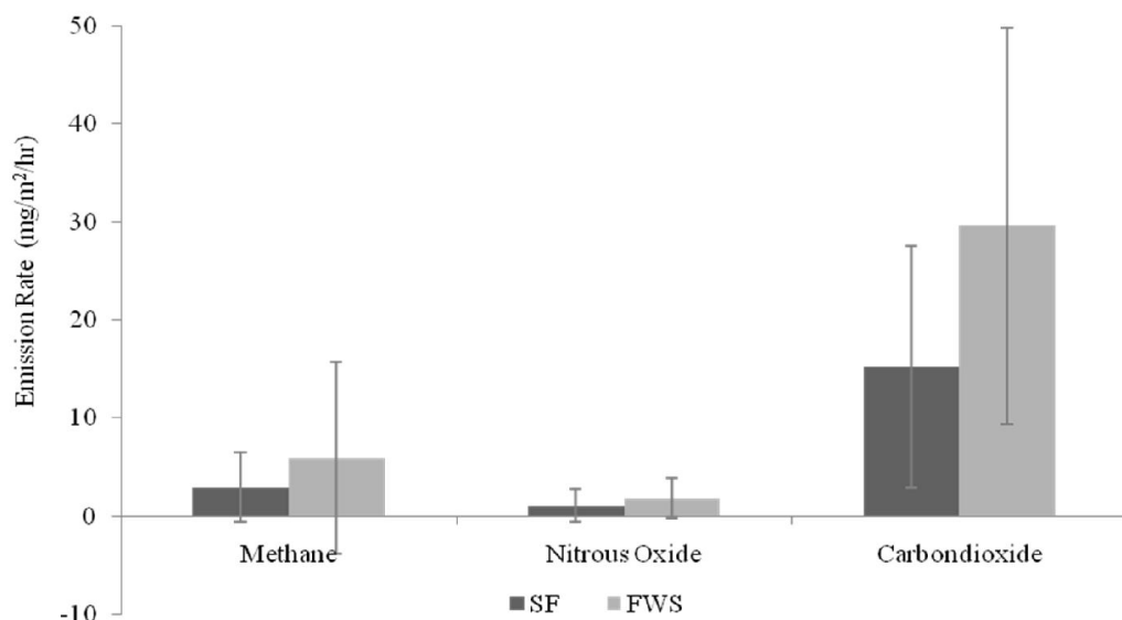
รูปที่ 4-23 เปรียบเทียบอัตราการปลดปล่อยก๊าซเรือนกระจกจากพื้นที่ชุ่มน้ำประดิษฐ์แบบไหลใต้ผิวดินกลางกับพื้นที่ชุ่มน้ำประดิษฐ์แบบไหลผ่านพื้นผิว
