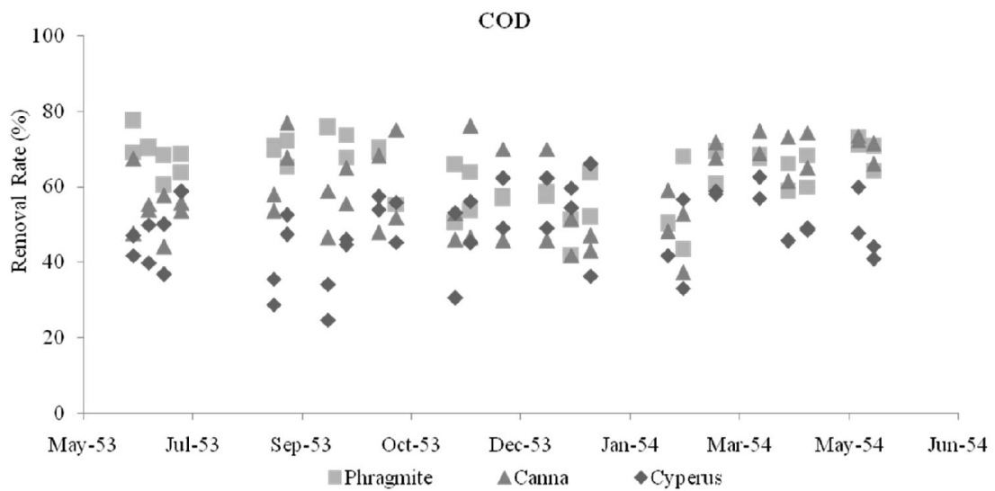
รูปที่ 4-12 ประสิทธิภาพการบำบัดซีโอดีของพืชชนิดต่าง ๆ ในพื้นที่ชุ่มน้ำประดิษฐ์แบบไหลผ่านพื้นผิว
