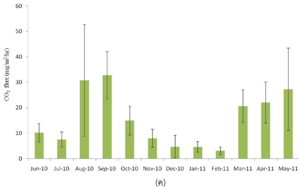
รูปที่ 4-17 อัตราการปลดปล่อยก๊าซเรือนกระจกจากพื้นที่ชุ่มน้ำประดิษฐ์แบบไหลใต้ผิวดินที่ปลูกด้วยพืชจำพวกกก (ก) ก๊าซมีเทน (ข) ก๊าซไนตรัสออกไซด์ (ค) ก๊าซคาร์บอนไดออกไซด์
