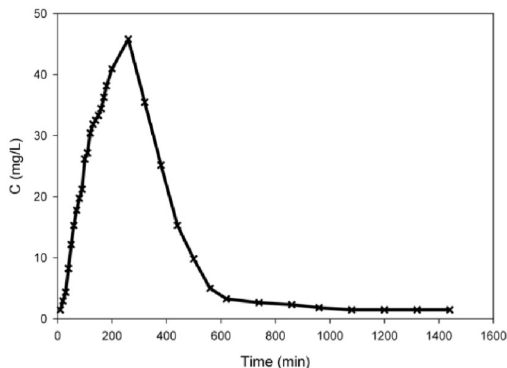
รูปที่ 4-1 ความสัมพันธ์ระหว่างความเข้มข้นของคลอไรด์ กับเวลาสำหรับบ่อดูดที่ปลูกกกในพื้นที่ชุ่มน้ำประดิษฐ์แบบไหลใต้ผิวดิน (SF)
