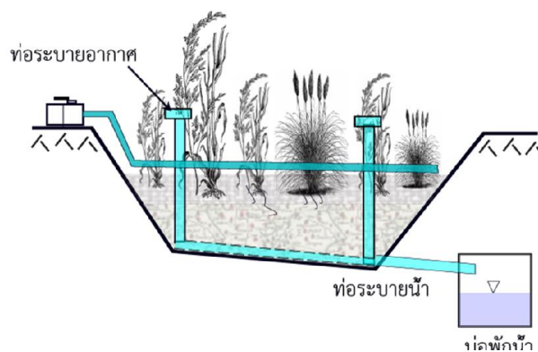
รูปที่ 2-8 พื้นที่ชุ่มน้ำประดิษฐ์ที่น้ำไหลได้ผิวชั้นกรองในแนวดิ่ง (Vertical Flow: VF)
