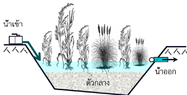
รูปที่ 2-6 พื้นที่ชุ่มน้ำประดิษฐ์ที่น้ำไหลท่วมผิวชั้นกรองอย่างอิสระ (Free Water Surface Systems: FWS)
