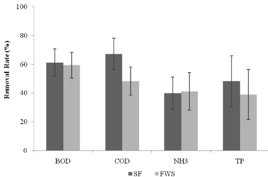
รูปที่ 4-10 เปรียบเทียบประสิทธิภาพการบำบัดมลพิษระหว่างพื้นที่ชุ่มน้ำประดิษฐ์แบบไหลใต้ผิวดิน (SF) และแบบไหลผ่านพื้นผิว (FWS)
