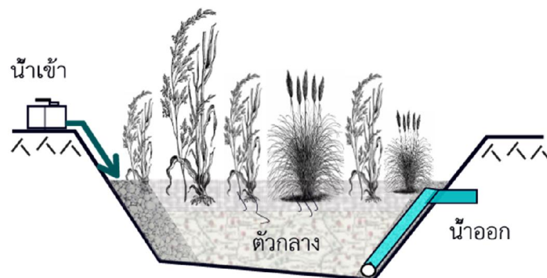
รูปที่ 2-7 พื้นที่ชุ่มน้ำประดิษฐ์ที่น้ำไหลใต้ผิวน้ำชั้นกรองในแนวนอน (Subsurface Flow Systems: SF)
