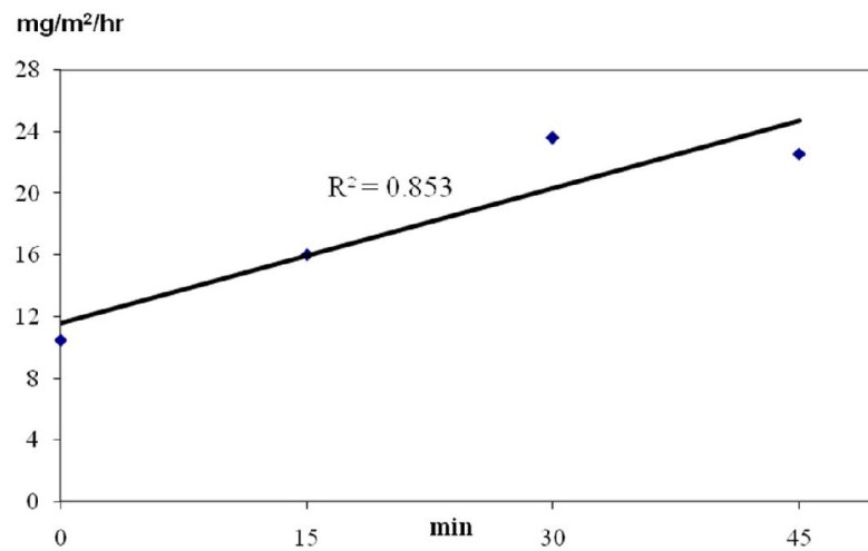
รูปที่ 3-10 ตัวอย่างความสัมพันธ์แบบ linear regression ระหว่างการเปลี่ยนแปลงความเข้มข้นของก๊าซที่สนใจกับเวลาที่เก็บตัวอย่าง
