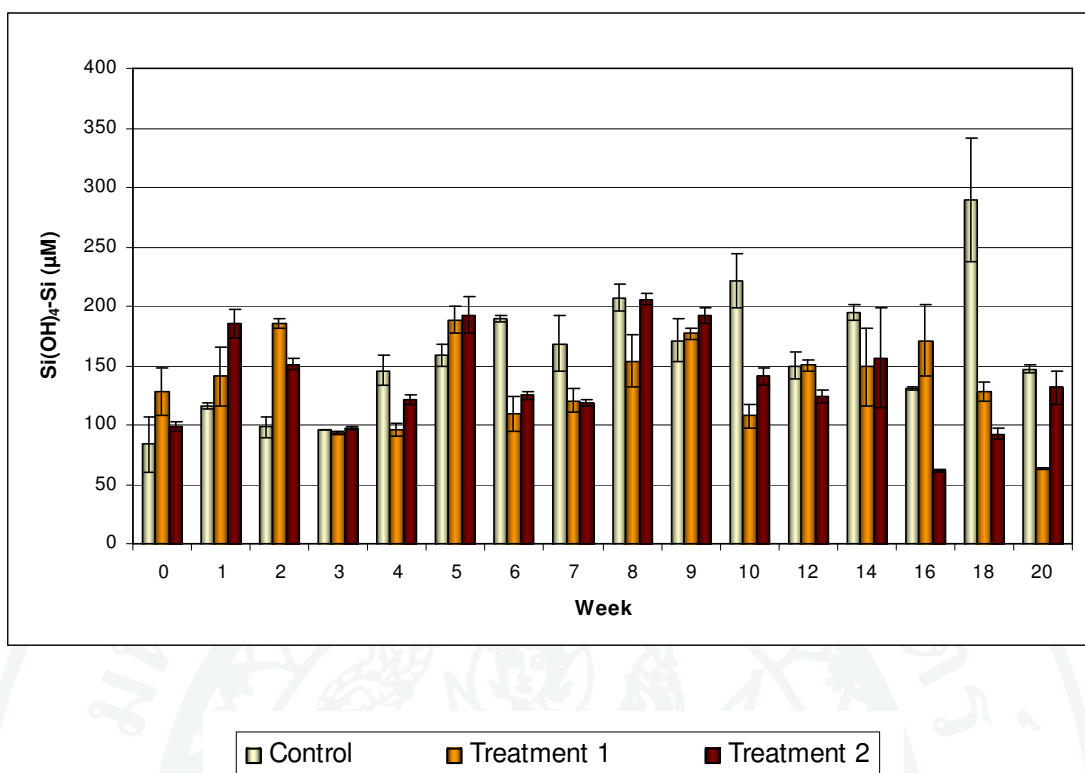
ภาพที่ 26 เปรียบเทียบการเปลี่ยนแปลงปริมาณซิลิเกต-ซิลิคอน (ไมโคร โมลาร์) ในน้ำระหว่างอนุภาคดินตะกอน เมื่อไม่มีการใส่ปุ๋ย (Control) ใส่ปุ๋ย 1.5 กรัม (Treatment 1) และ 3.0 กรัม (Treatment 2) ต่อกลไกกรัมดินตะกอน (ค่าเฉลี่ย±SD)
