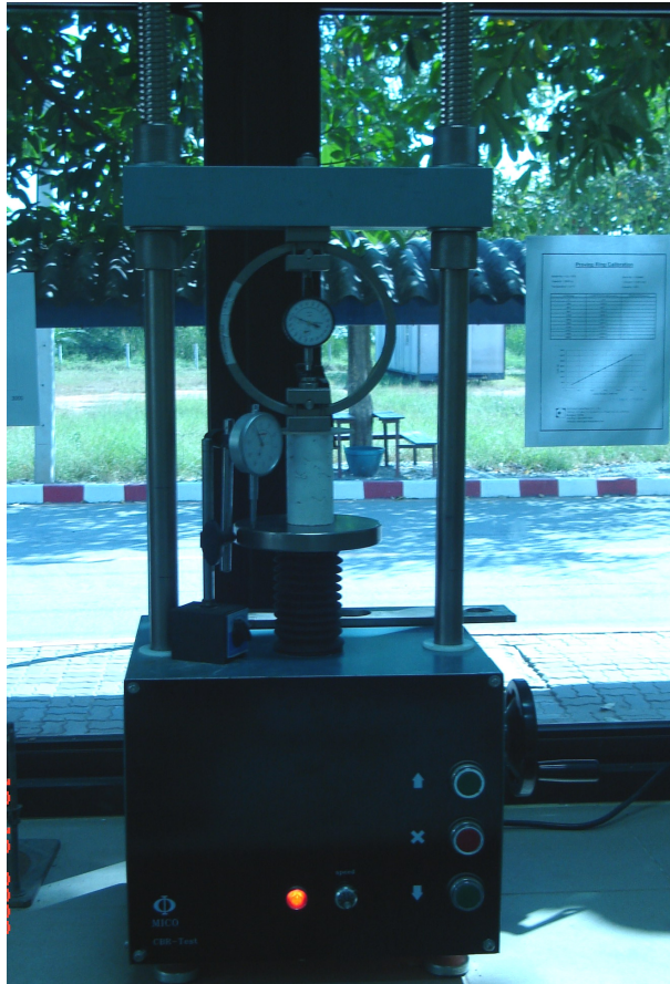
ภาพที่ ก.5 เครื่องมือทดสอบและการทดสอบ Unconfined Compression Test
