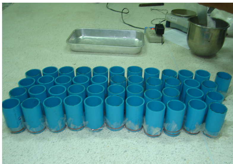
ภาพที่ ก.1 การเตรียมแบบหล่อท่อ PVC.ขนาดเส้นผ่านศูนย์กลาง 5 เซนติเมตร ความสูง 10 เซนติเมตร
