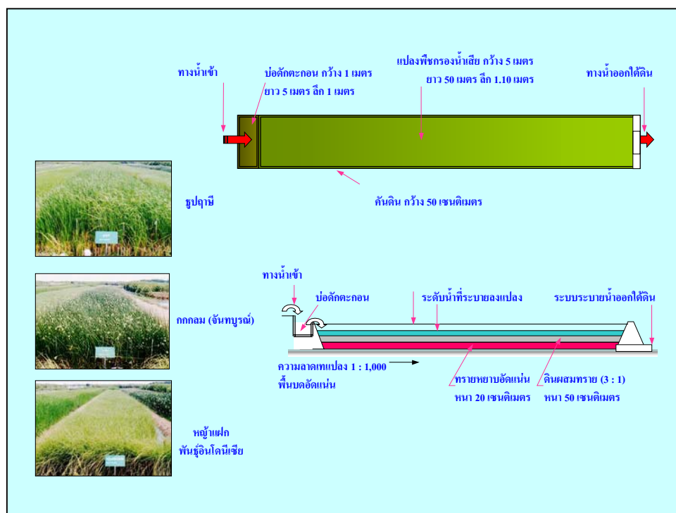
ภาพผนวกที่ 4 ญ ระบบพื้นที่ชุ่มน้ำเทียม
