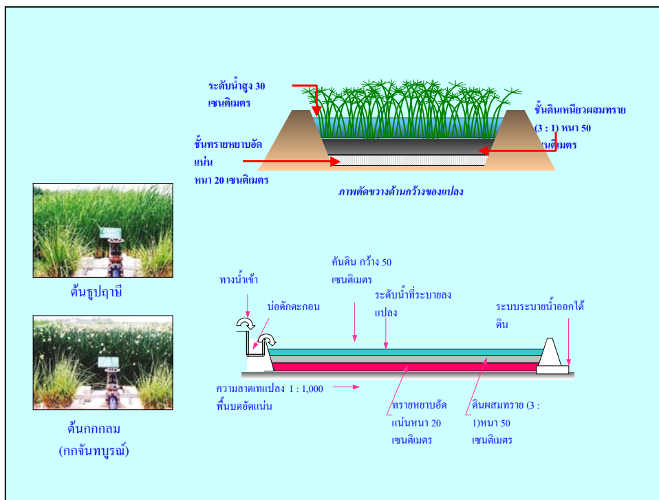
ภาพผนวกที่ 3 ญ ระบบบำบัดน้ำเสียด้วยพืชกรองน้ำเสีย
