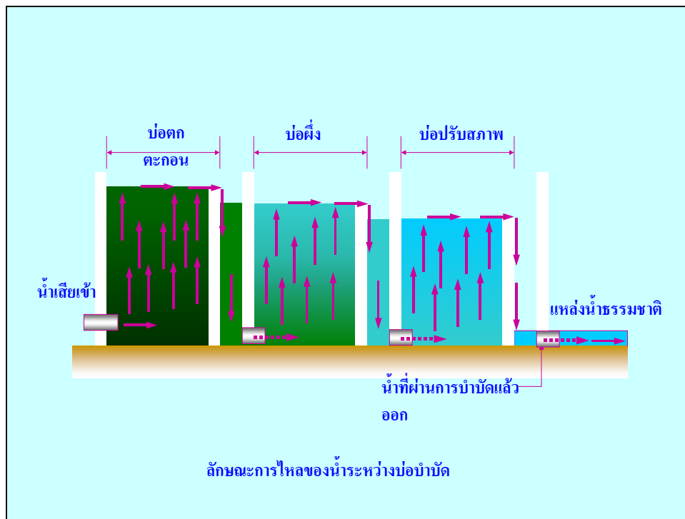
ภาพผนวกที่ 1 ญ ระบบบำบัดน้ำเสียแบบบ่อผึ่ง
