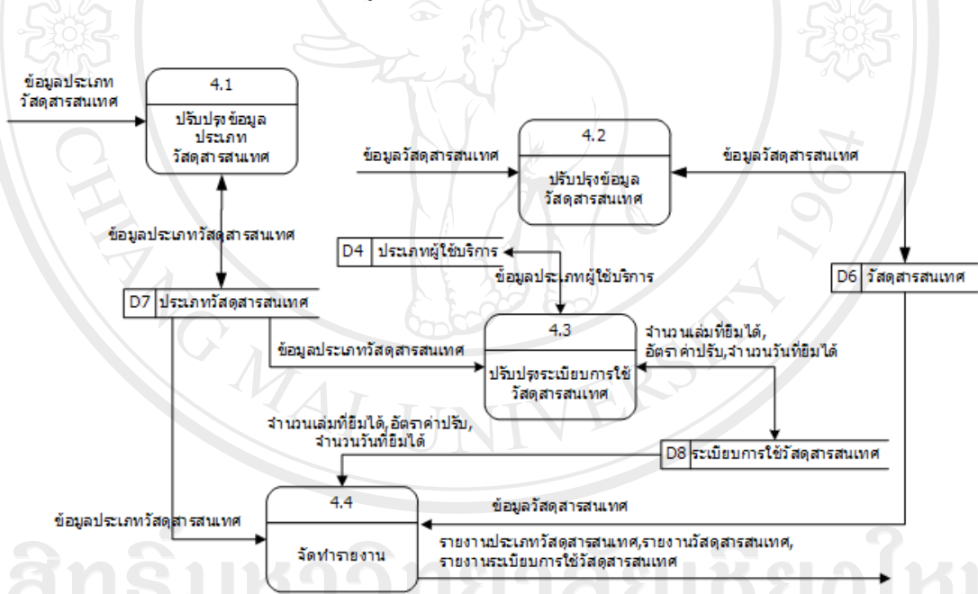
รูป 3.11 แผนผังกระแสข้อมูลระดับที่ 1 ของกระบวนการที่ 4.0 ลงทะเบียนวัสดุสารสนเทศ
